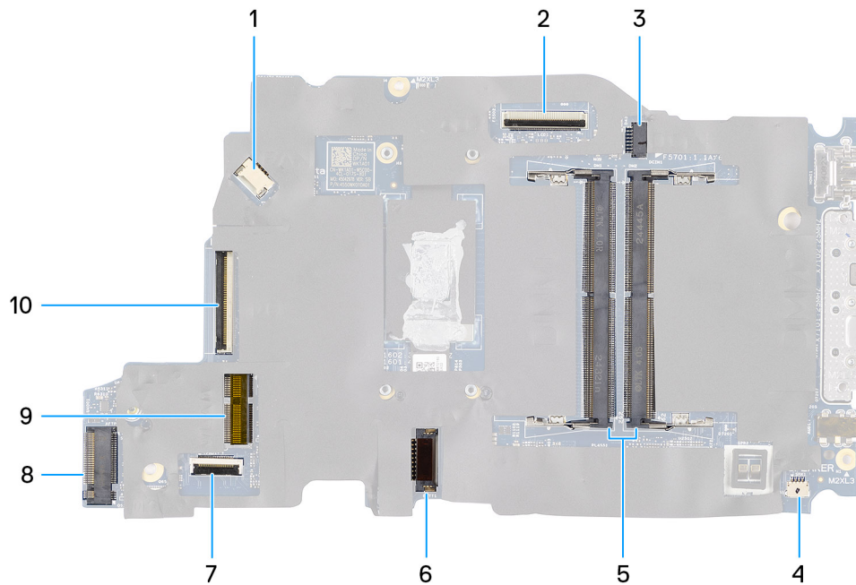
Abbildung 42. Hauptplatinenanschlüsse
