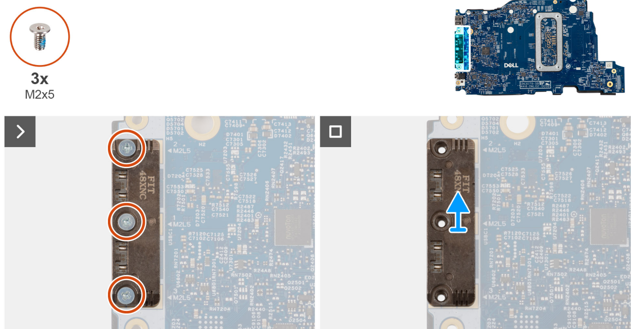
Abbildung 48. Entfernen des USB-Type-C-Moduls
