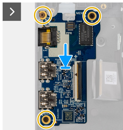
Abbildung 37. Installieren der I/O-Platine
