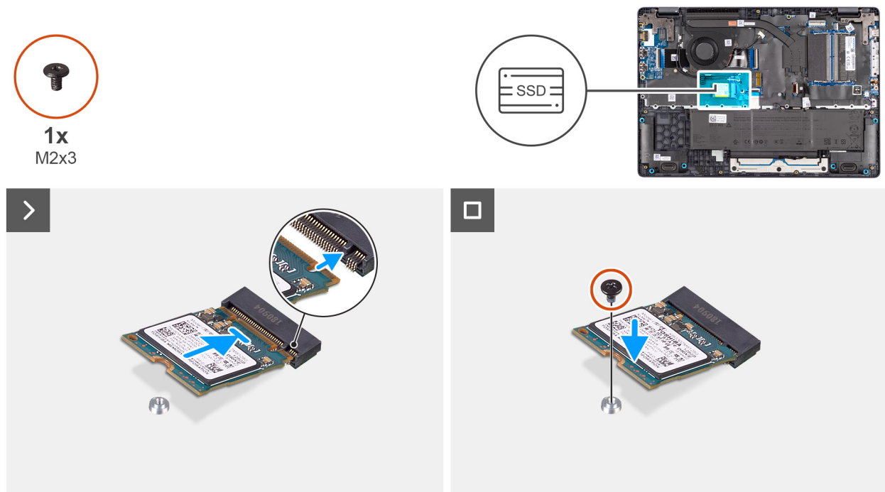
Abbildung 24. Einbauen der SSD-Karte
