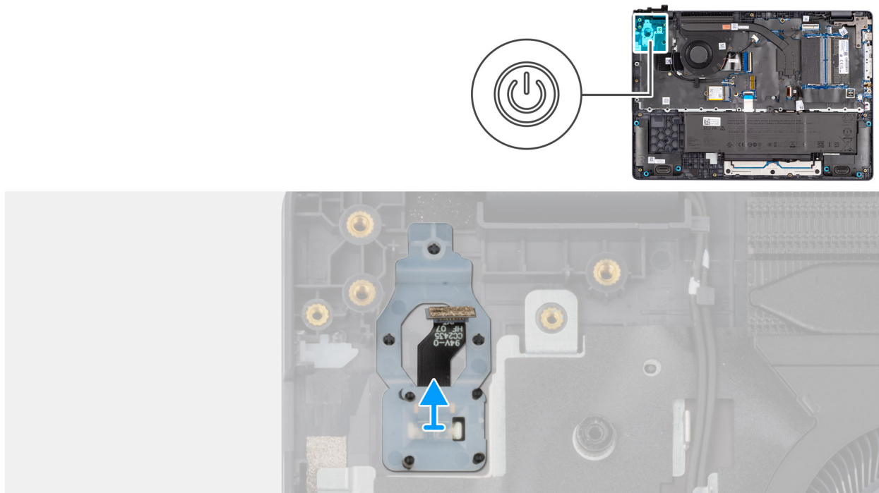
Abbildung 40. Entfernen des Netzschalters mit Fingerabdruck-Lesegerät
