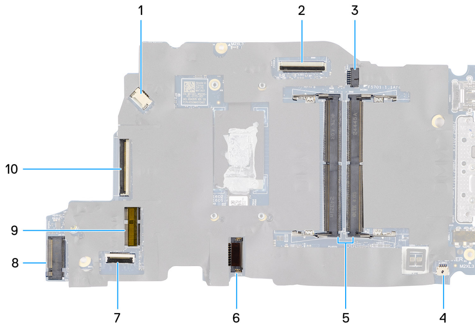
Abbildung 45. Hauptplatinenanschlüsse
