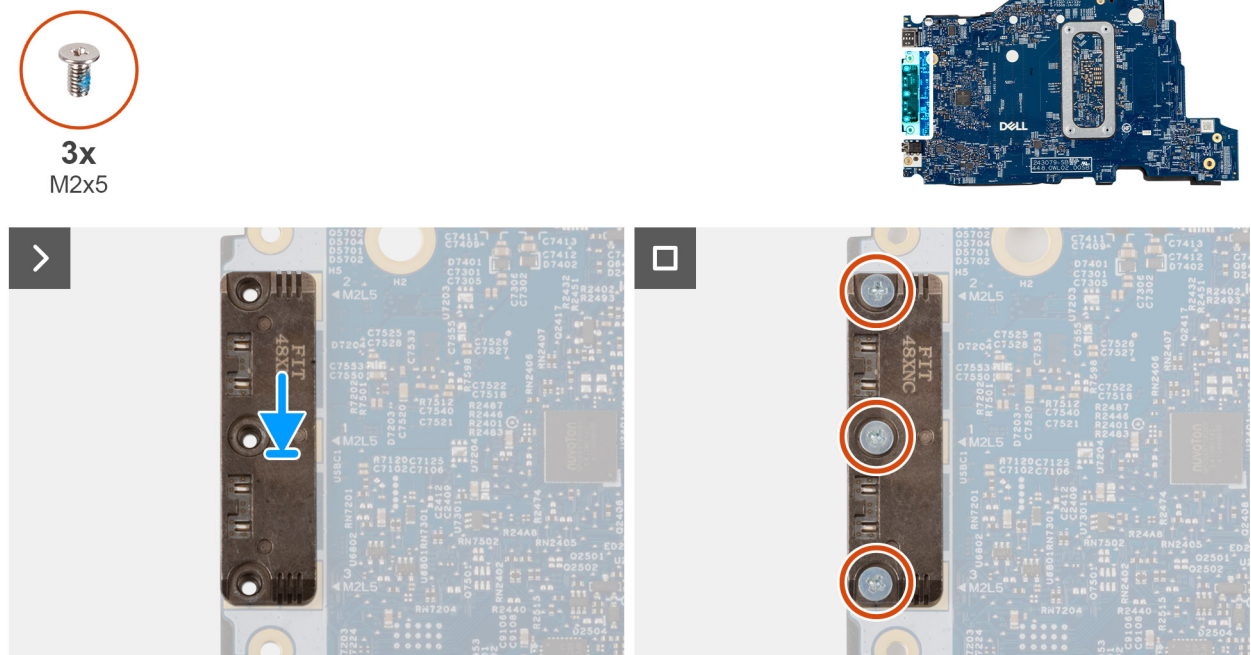
Abbildung 49. Installieren des USB-Type-C-Moduls
