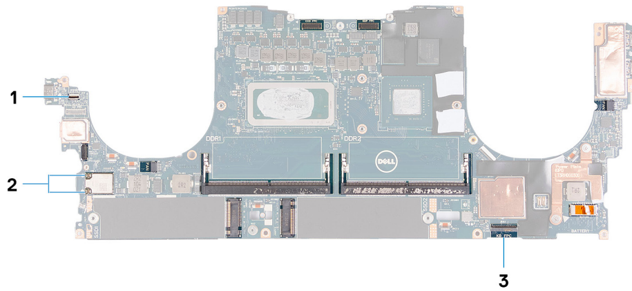
Abbildung 2. Systemplattenanschlüsse
