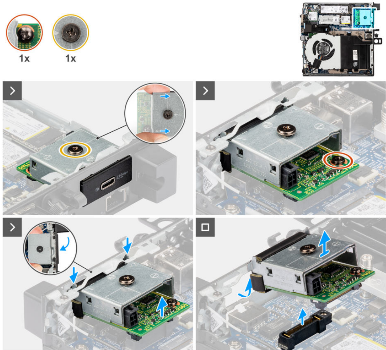
Abbildung 41. Installieren des USB-Typ-C-Anschlussmoduls
