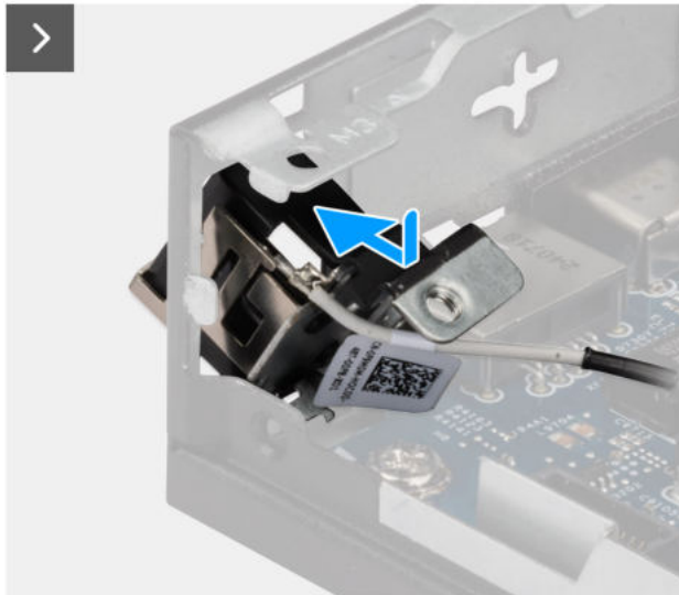
Abbildung 74. Einbauen des Antennenmoduls (weißes Kabel)
