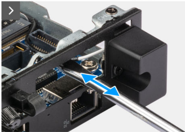
Abbildung 39. Installieren des dualen USB-3.2-Gen2-Anschlussmoduls
