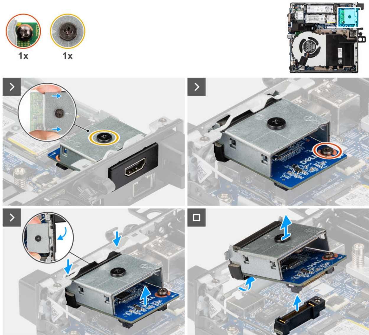
Abbildung 50. Entfernen des HDMI-Anschlussmoduls
