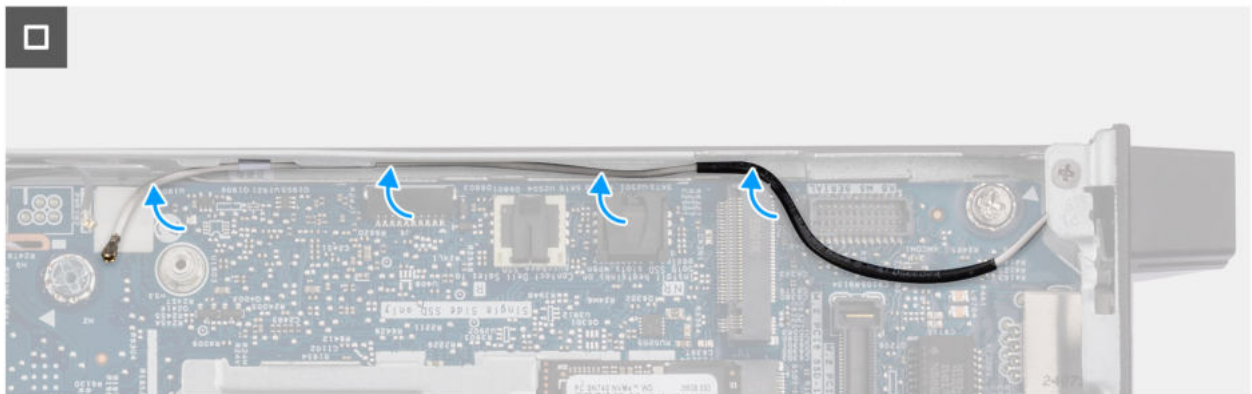
Abbildung 75. Einbauen des Antennenmoduls (weißes Kabel)
