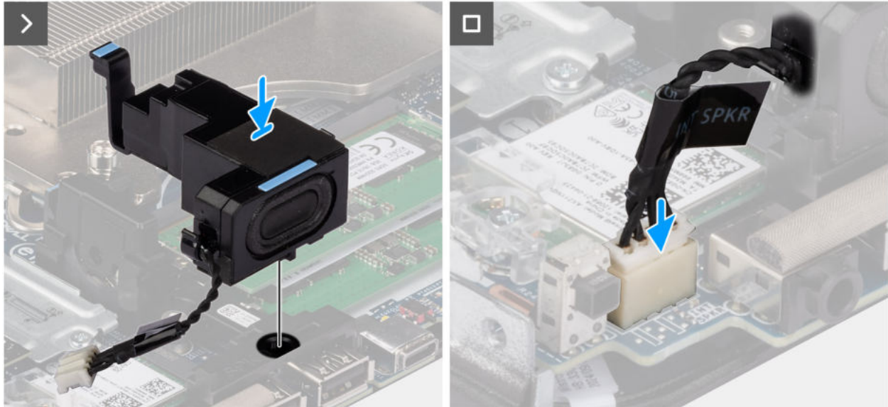
Abbildung 15. Einbauen des Lautsprechers
