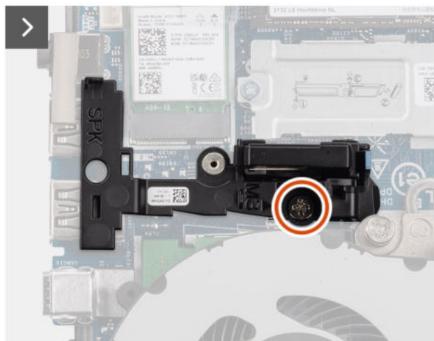
Abbildung 78. Entfernen der Lautsprecherhalterung
