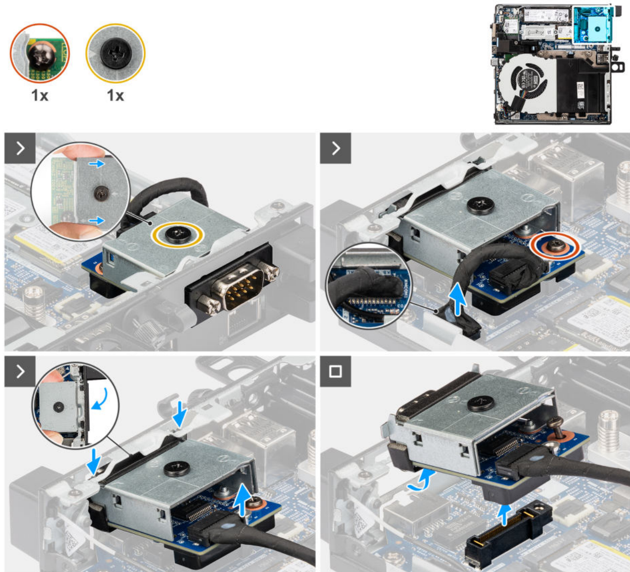
Abbildung 59. Entfernen des seriellen Anschlussmoduls
