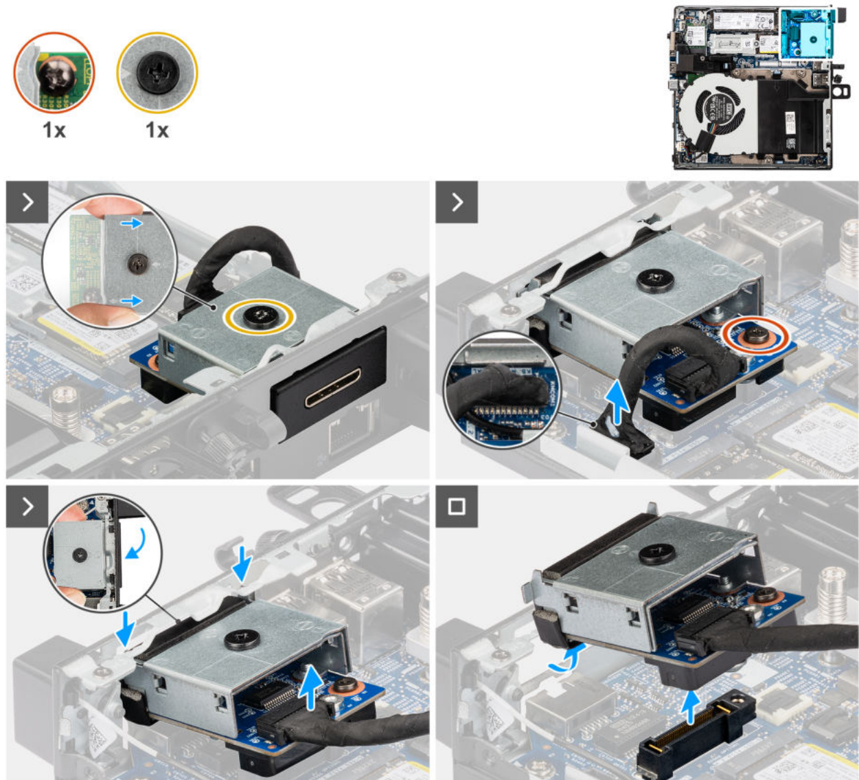
Abbildung 56. Entfernen des PS2-Anschlussmoduls
