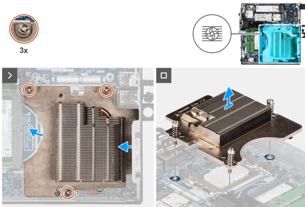
Abbildung 68. Kühlkörper entfernen
