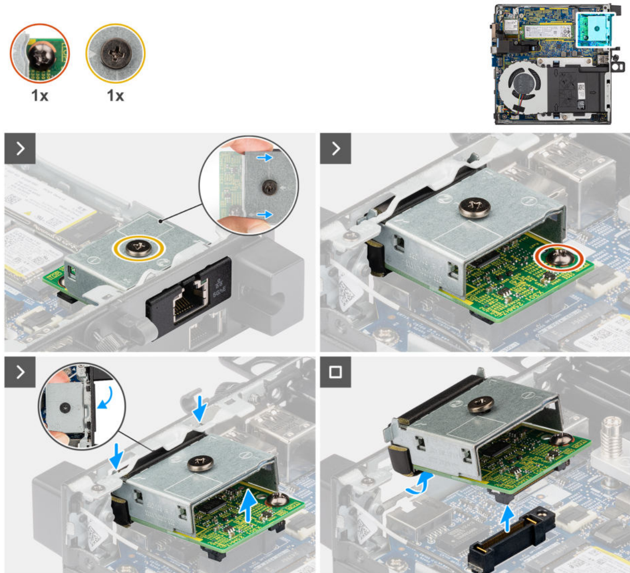
Abbildung 65. Entfernen des RJ45-Ethernet-Anschlussmoduls
