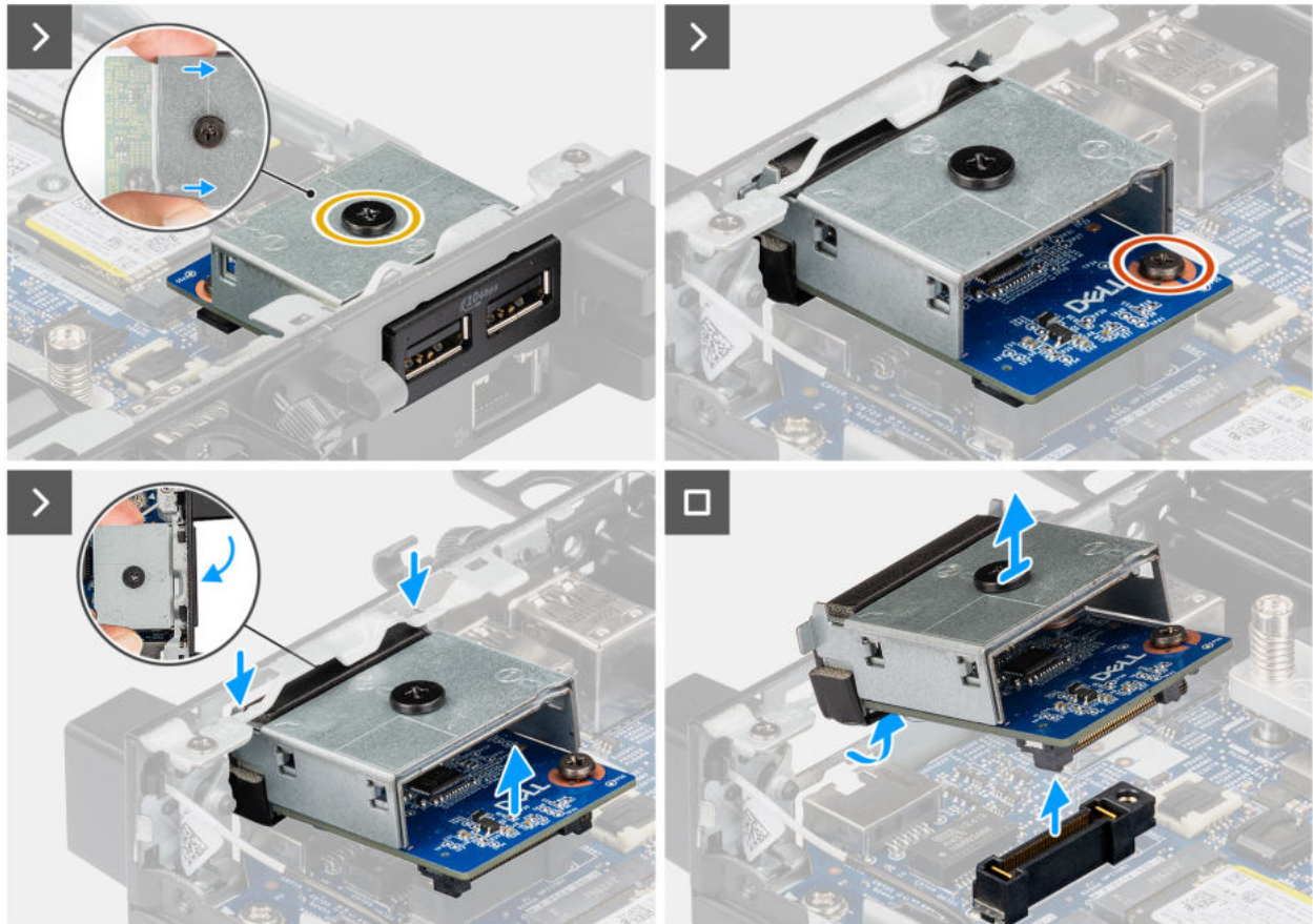
Abbildung 38. Entfernen des dualen USB-3.2-Gen2-Anschlussmoduls
