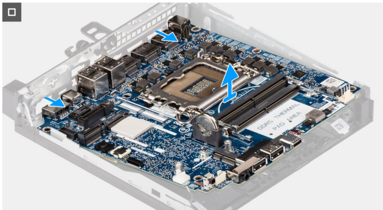
Abbildung 82. Entfernen der Systemplatine
