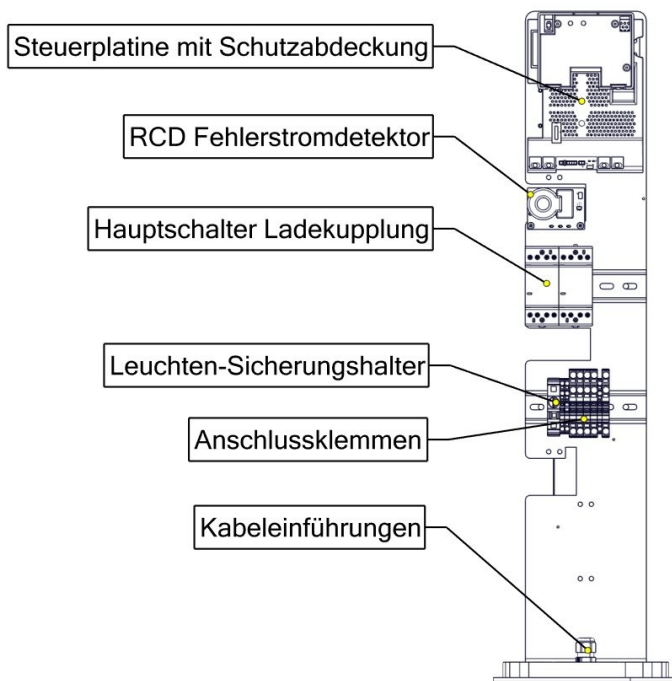
Abbildung 1. Vorderseite des Geräteträgerblech
