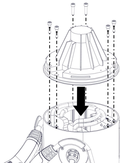
Abbildung 19. Montage Leuchtaufnahme
