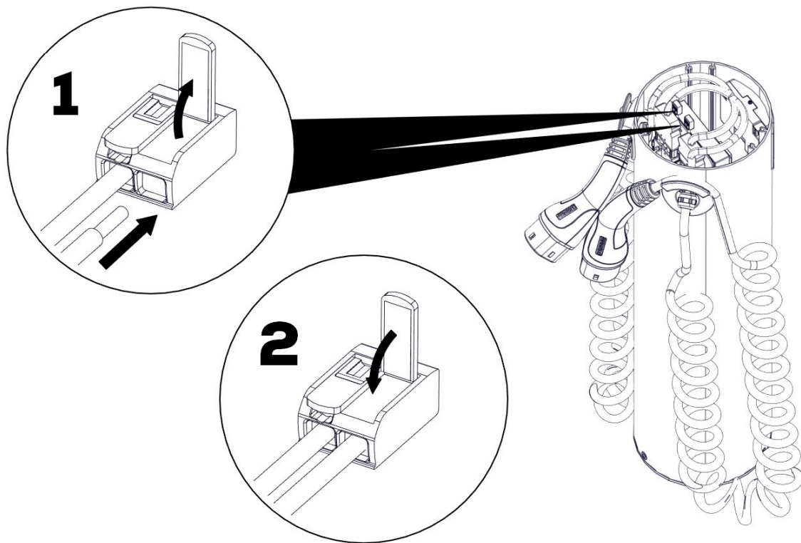
Abbildung 15. Anschluss der CP-Leitung
