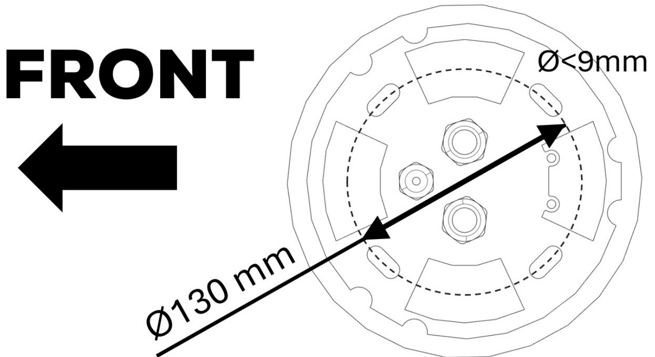
Abbildung 4. Fundamentausrüstung
