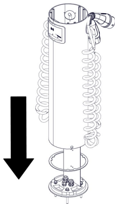
Abbildung 11. Montage des Dichtungsringes
