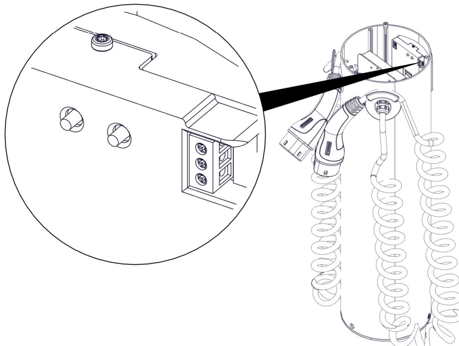
Abbildung 8. Anschluss der Modbusleitung
