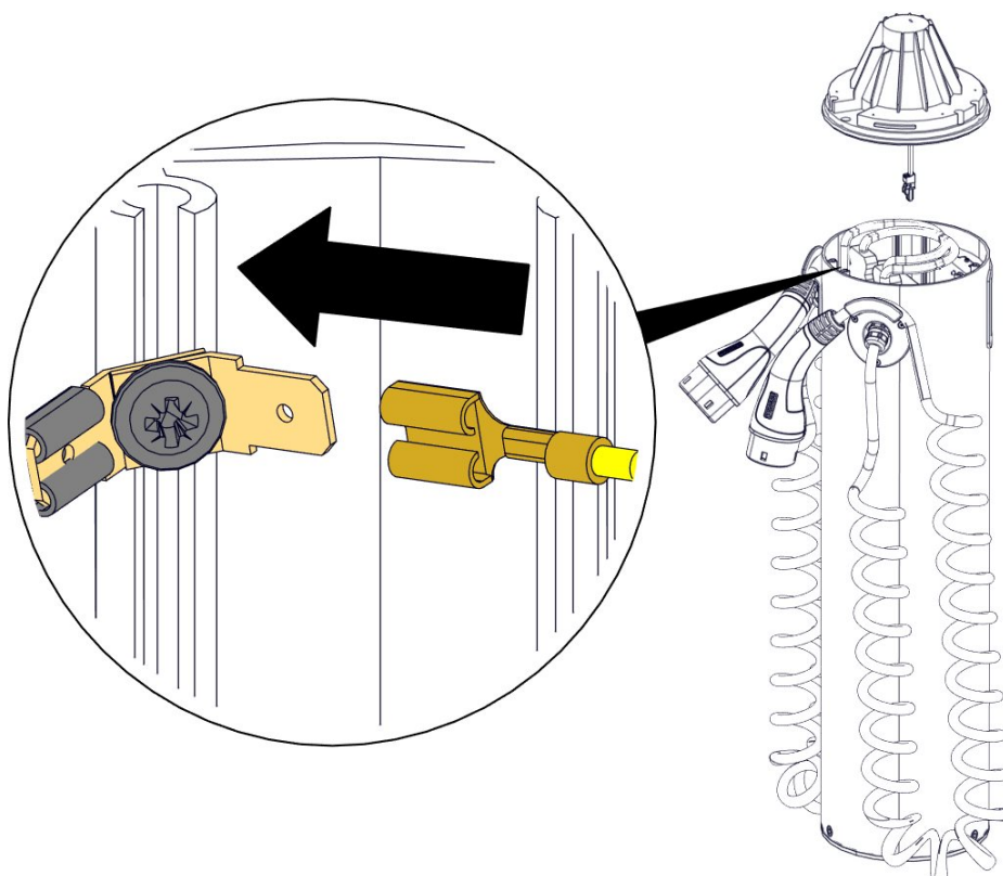
Abbildung 18. Erdung der Leuchtenaufnahme
