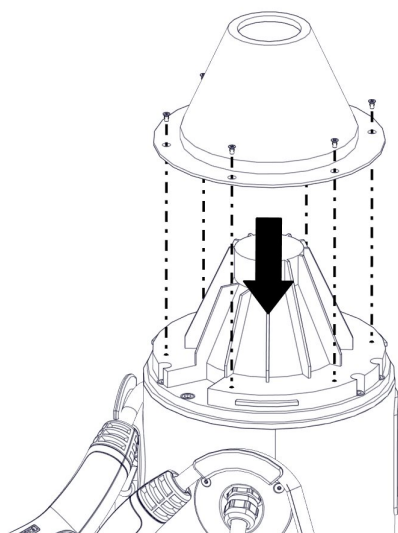
Abbildung 20. Montage Leuchten-Blende
