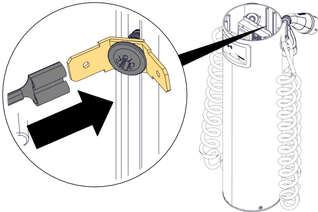
Abbildung 13. Erdungslasche des Rohres aufstecken
