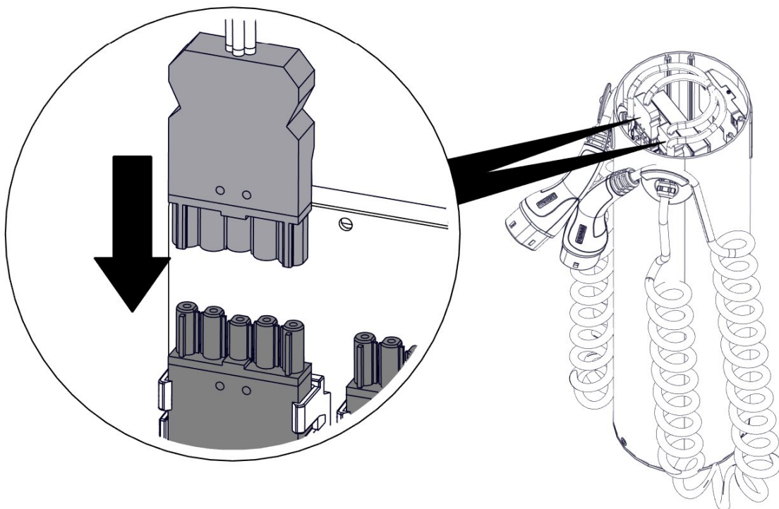
Abbildung 16. Anschluss der Ladeleitungen
