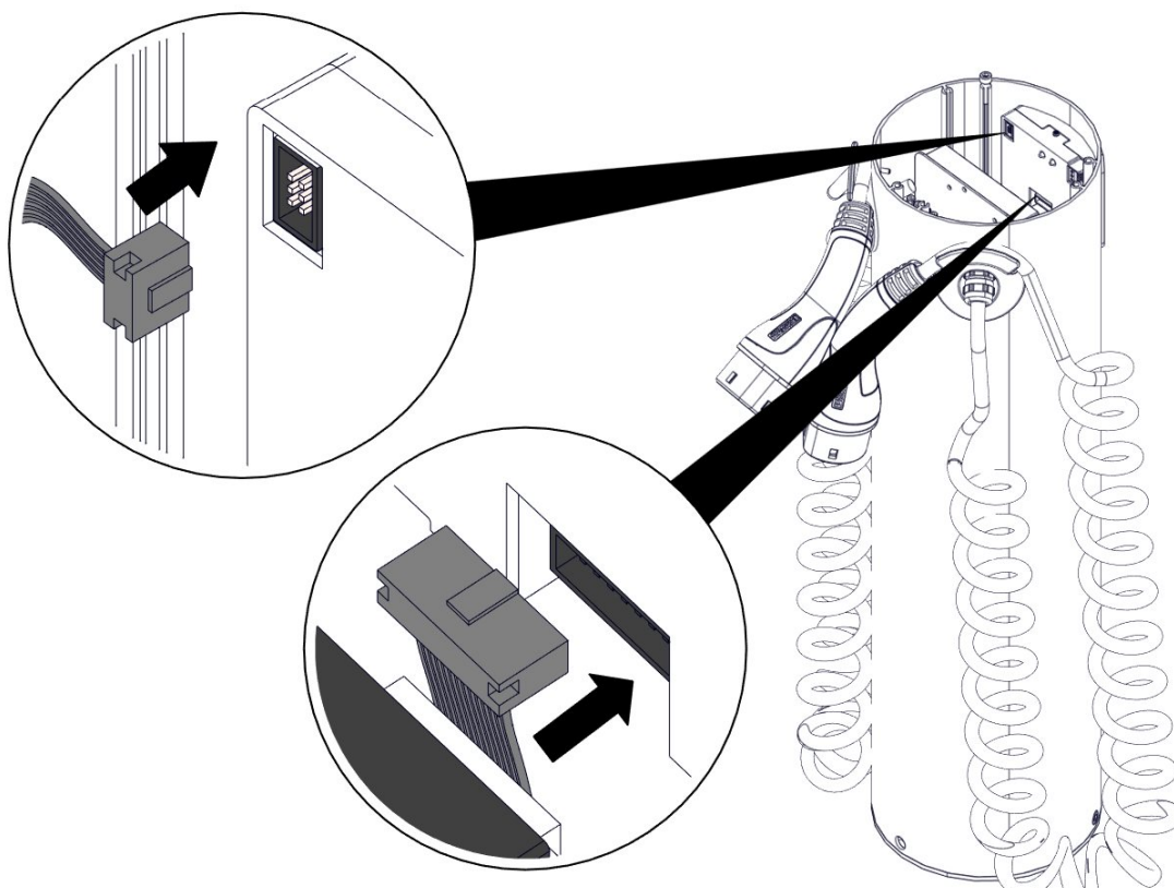
Abbildung 14. Anschluss RFID-Modul
