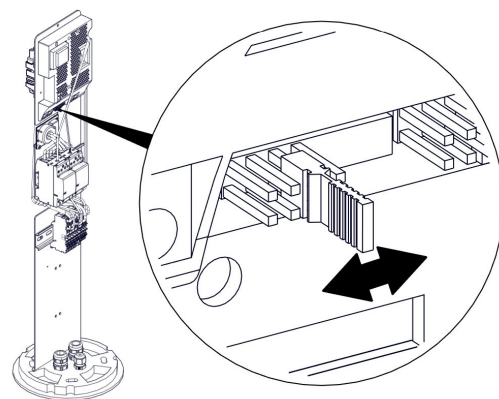
Abbildung 10. Position der Steckbrückenpins
