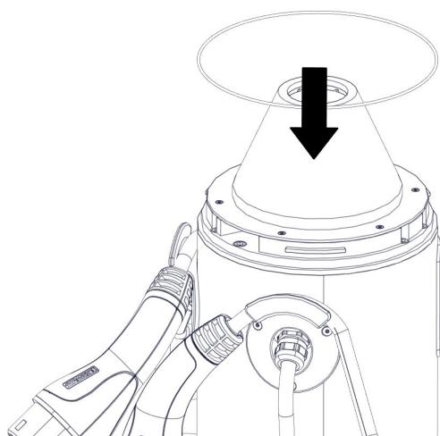
Abbildung 21. Auflage Dichtschnur
