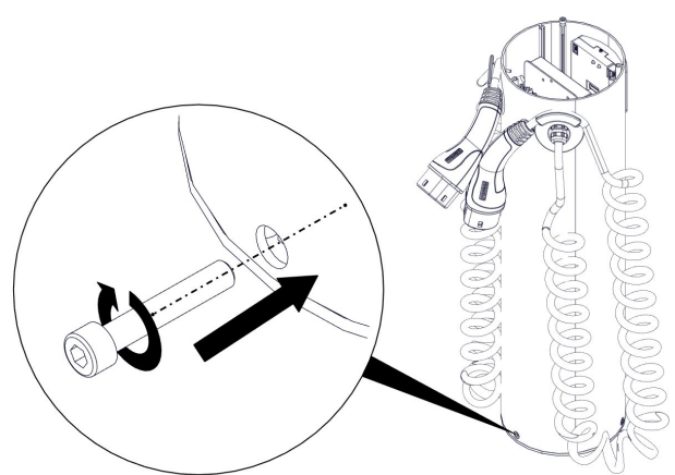
Abbildung 12. Untere Verschraubung des Gehäuses
