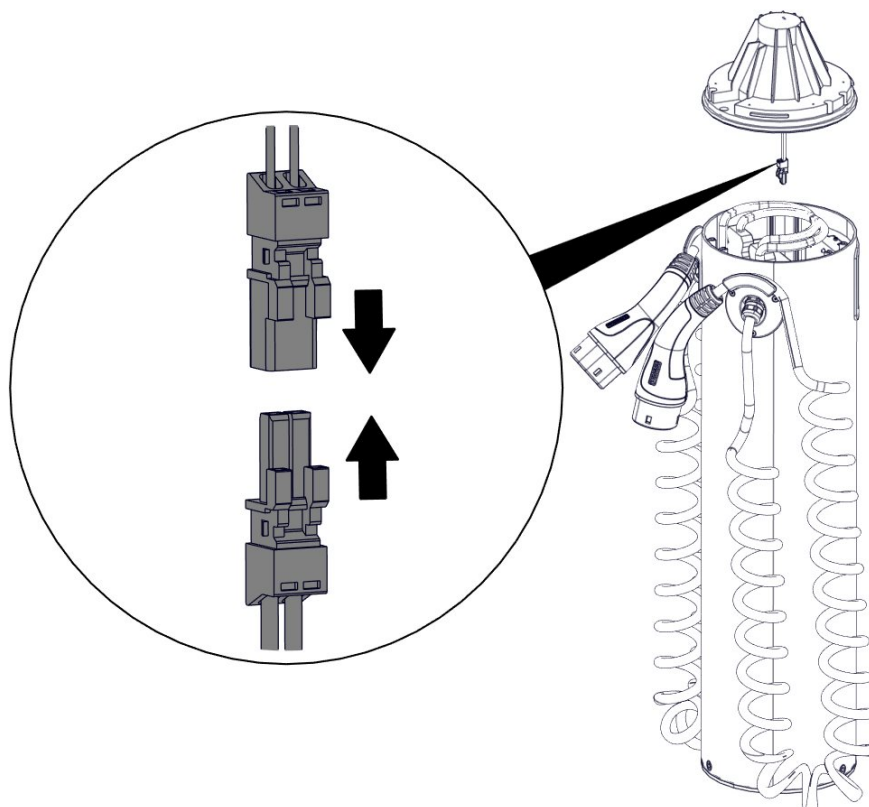
Abbildung 17. Anschluss der Leuchtenleitung
