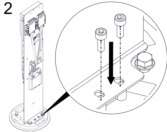
Abbildung 6. Montage des Geräteträgerblechs
