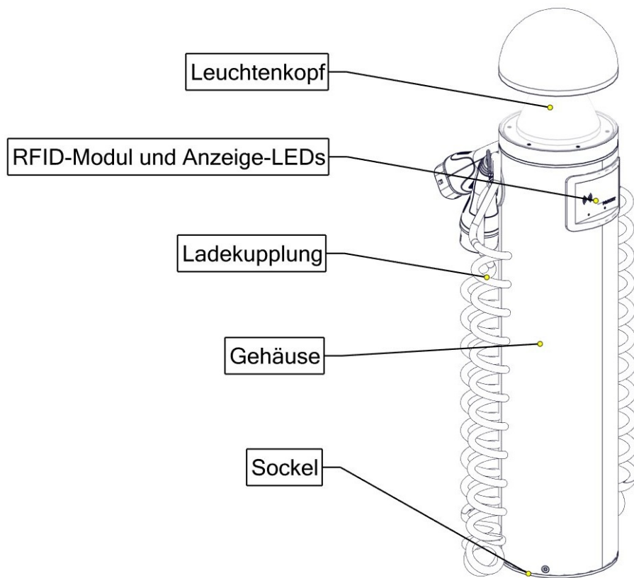
Abbildung 3. Komponenten der GAMMA
