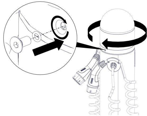
Abbildung 23. Fixierung Leuchtenabdeckung
