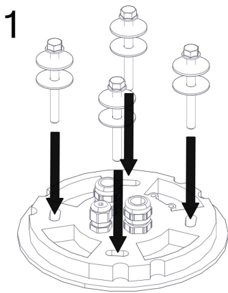
Abbildung 5. Montage der Bodenplatte
