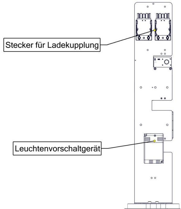
Abbildung 2. Rückseite des Geräteträgerblech
