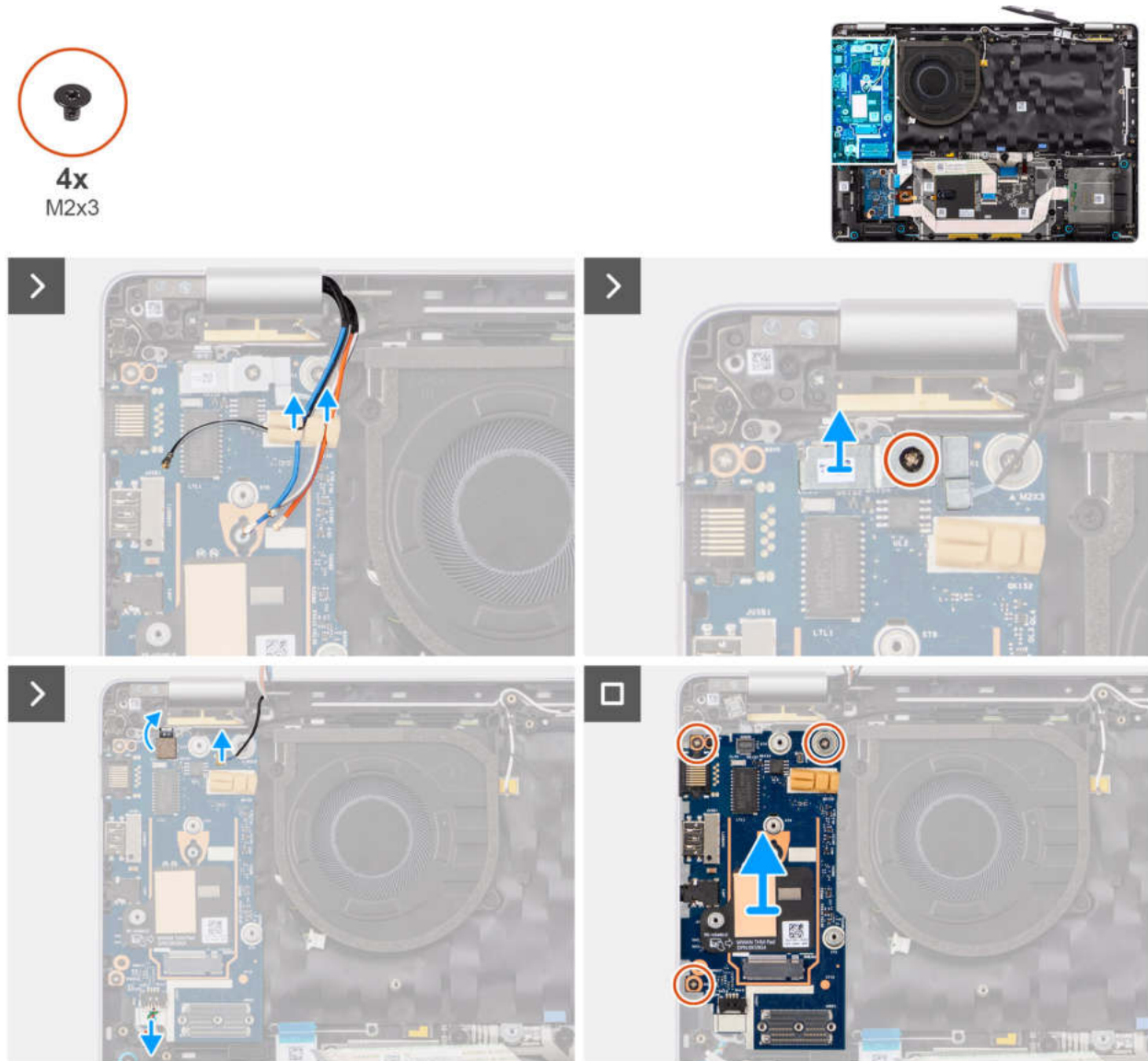
Abbildung 53. Entfernen der E/A-Platine
