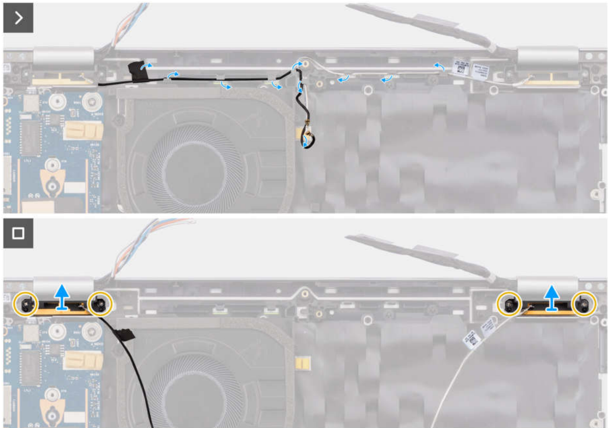
Abbildung 48. Entfernen der WLAN-Antennenmodule
