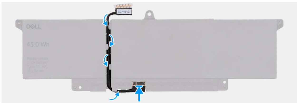
Abbildung 24. Austauschen des Akkukabels
