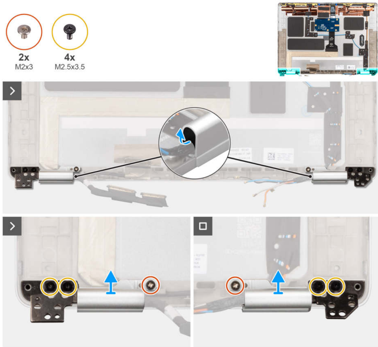
Abbildung 73. Entfernen der Bildschirmscharniere
