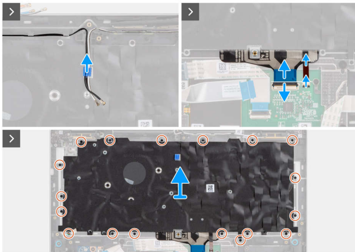
Abbildung 93. Entfernen der Tastatur
