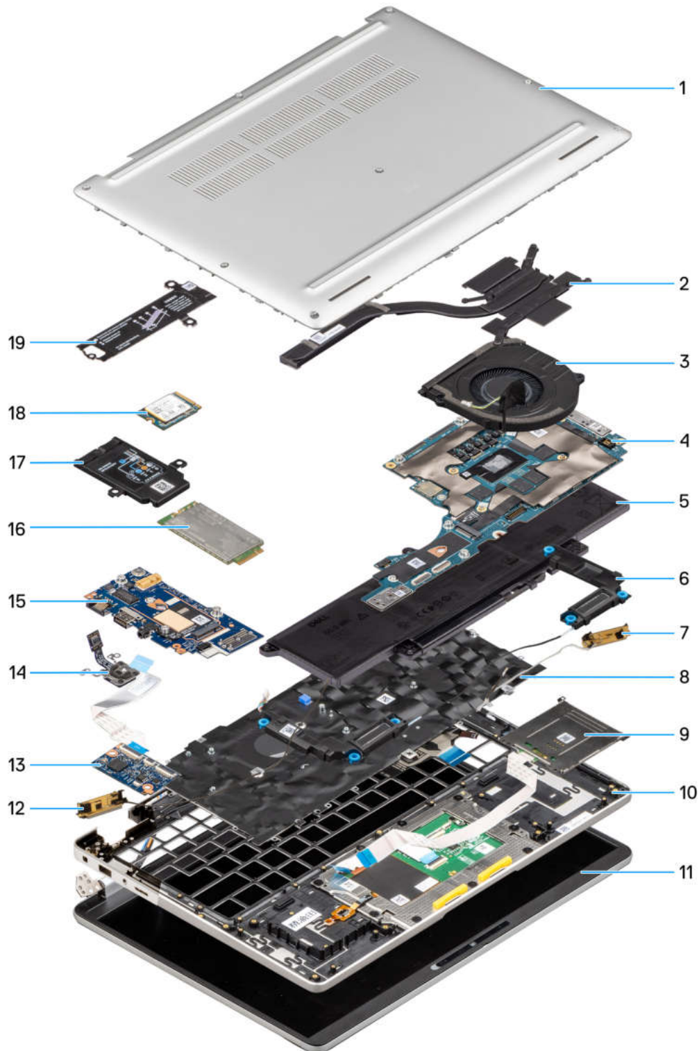
Abbildung 14. Hauptkomponenten des Dell Pro 14 Plus/Dell Pro 14 Plus 2-in-1
