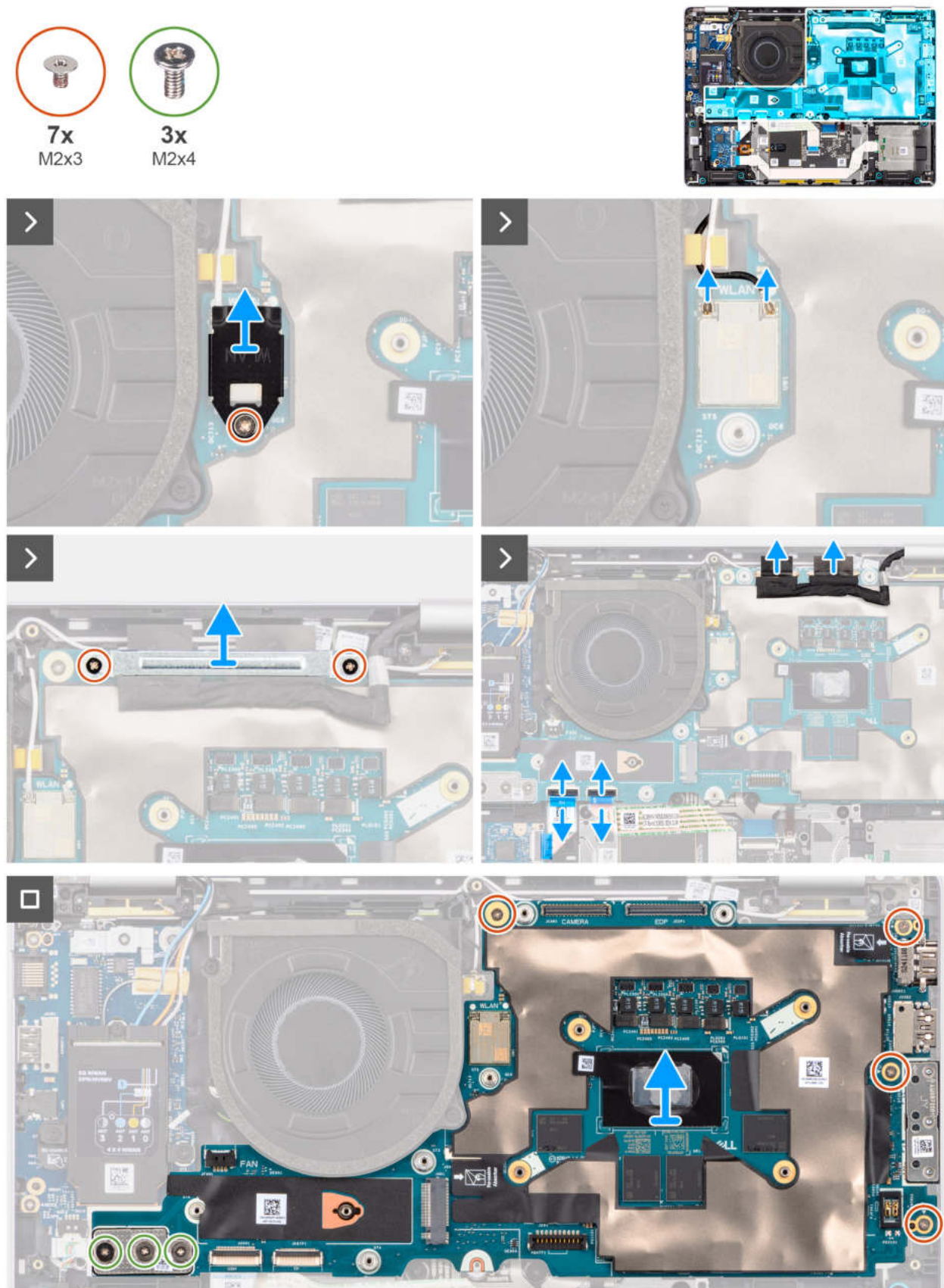
Abbildung 43. Entfernen der Systemplatine
