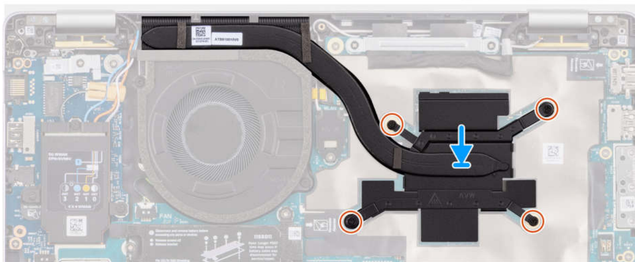
Abbildung 37. Einsetzen des Kühlkörpers
