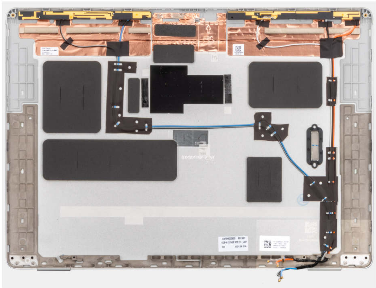
Abbildung 91. Entfernen der Baugruppe aus hinterer Bildschirmabdeckung und Antennen
