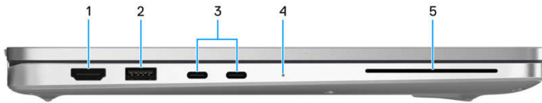
Abbildung 2. Linke Seitenansicht des Dell Pro 14 Plus/Dell Pro 14 Plus 2-in-1
