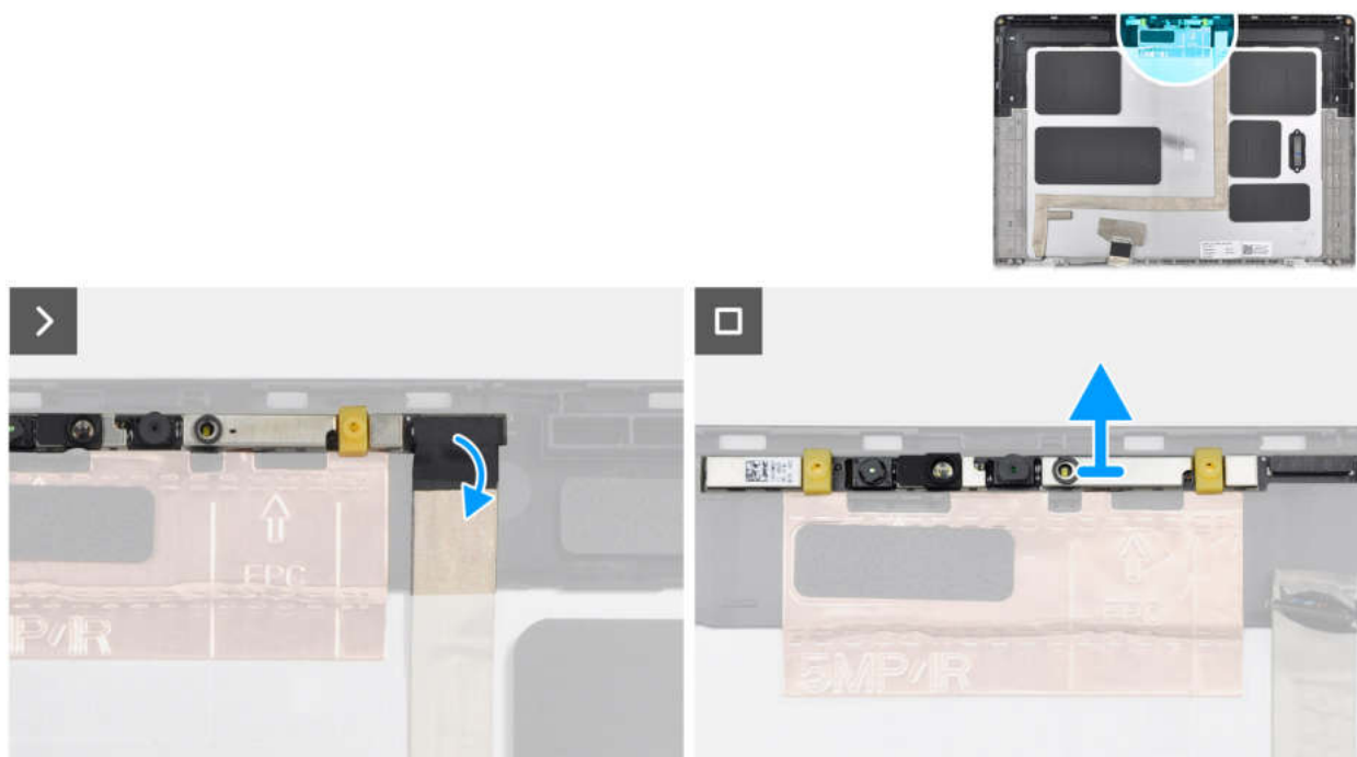
Abbildung 75. Entfernen der IR-Kamera
