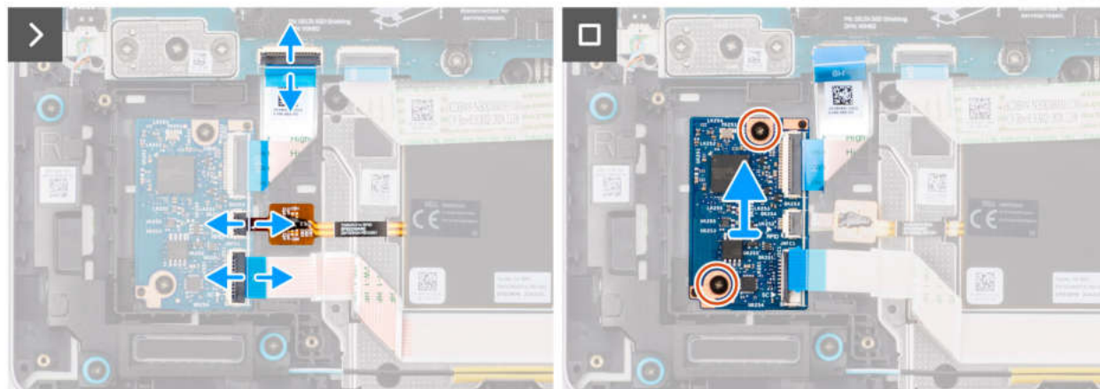
Abbildung 38. Entfernen der USH-Zusatzplatine
