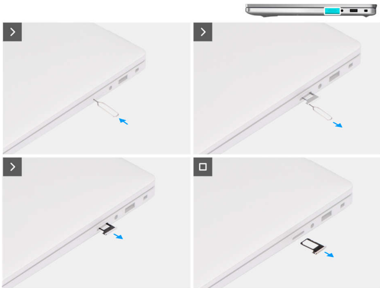
Abbildung 15. Entfernen des SIM-Kartenfachs
