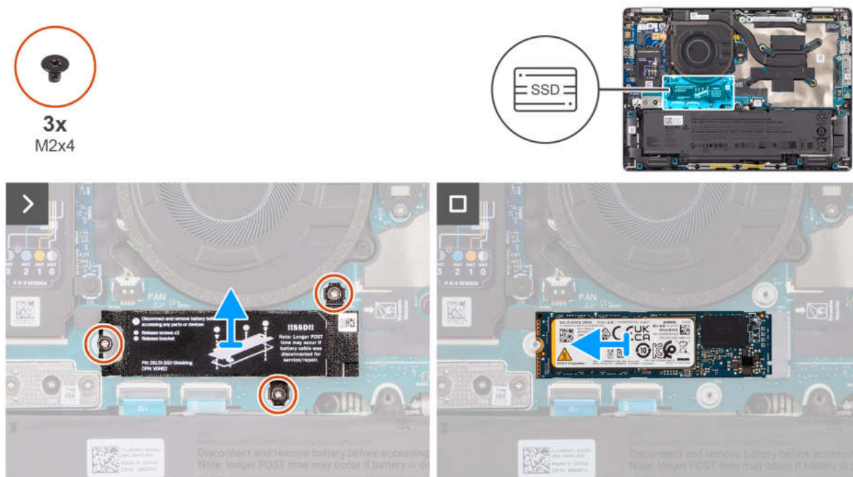
Abbildung 29. Entfernen der M.2-2280-SSD
