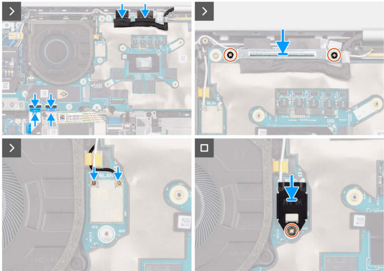
Abbildung 46. Einbauen der Systemplatine
