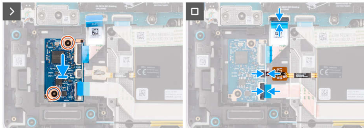
Abbildung 39. Installieren der USH-Zusatzplatine
