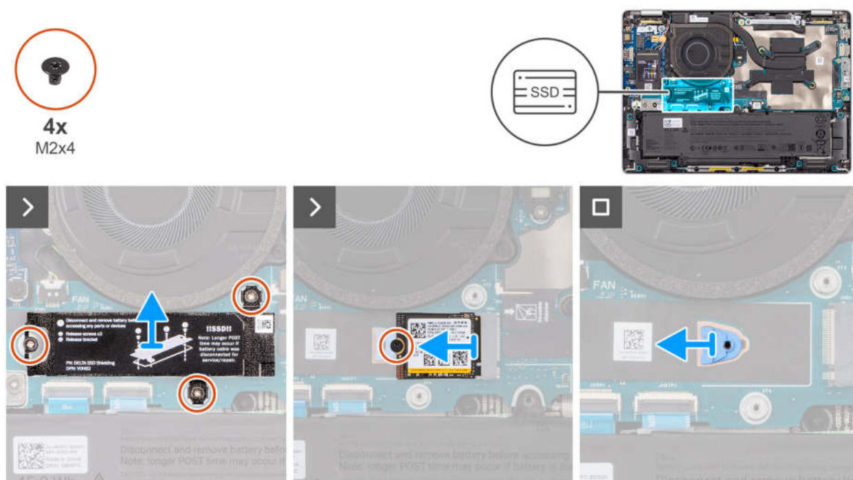
Abbildung 27. Entfernen des M.2-2230-Solid-State-Laufwerks
