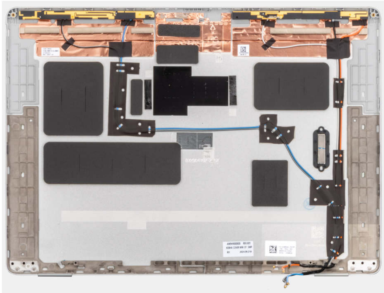
Abbildung 92. Bildschirmrückwand-Antennen-Baugruppe
