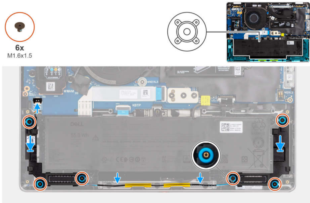
Abbildung 32. Installieren der Lautsprecher
