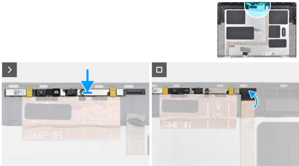
Abbildung 77. Installieren der IR-Kamera
