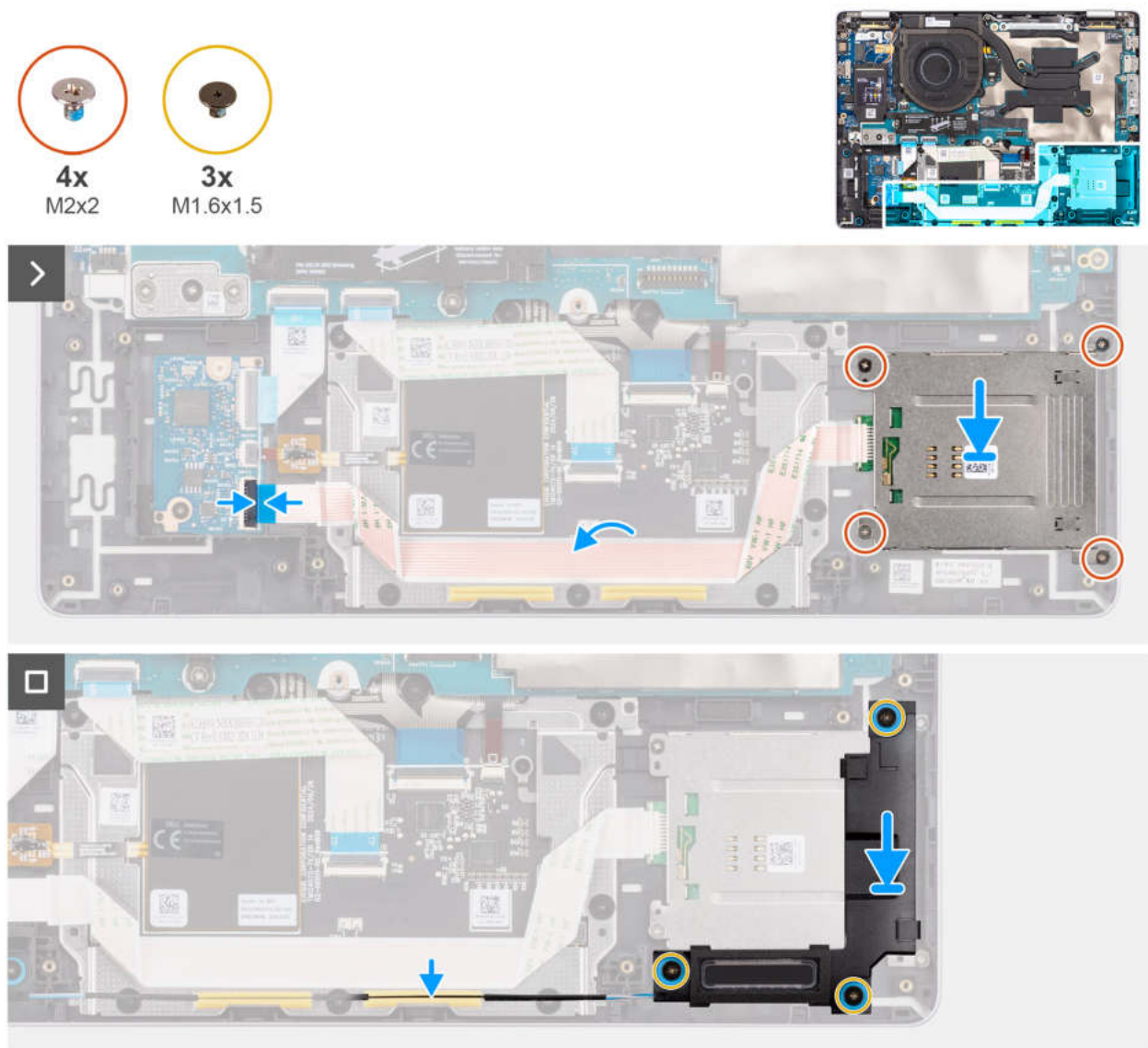
Abbildung 41. Installieren des Smartcardlesegeräts
