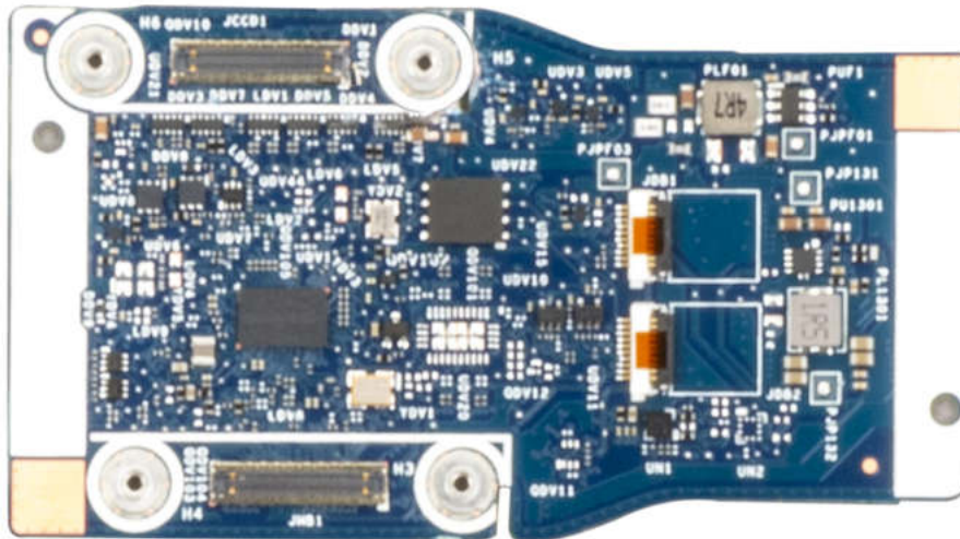
Abbildung 89. Mittlere Zusatzplatine
