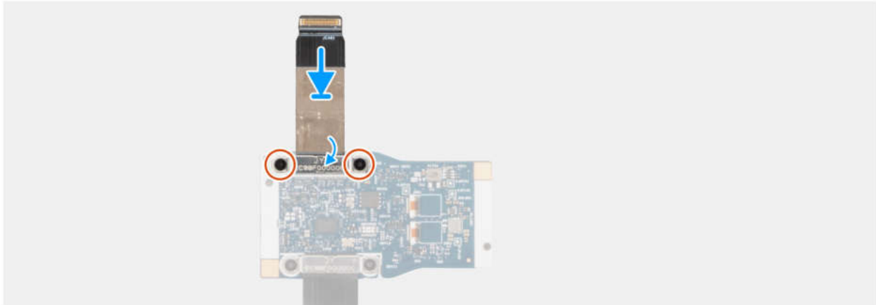
Abbildung 88. Installieren des Kabels der mittleren Zusatzplatine
