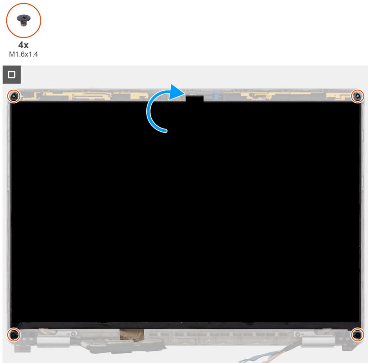
Abbildung 72. Einbauen des Bildschirms
