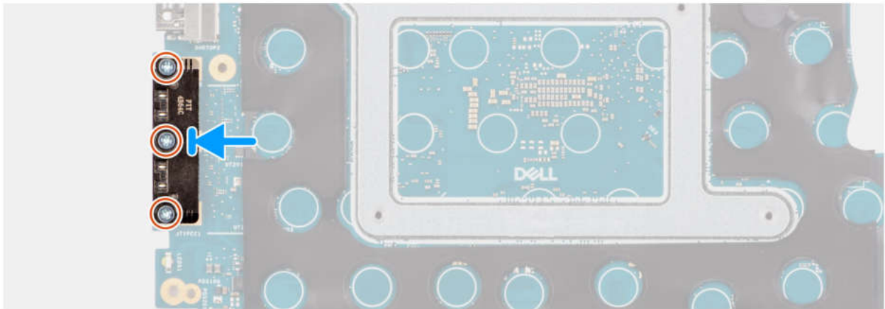
Abbildung 52. Installieren des USB-Type-C-Anschlussmoduls
