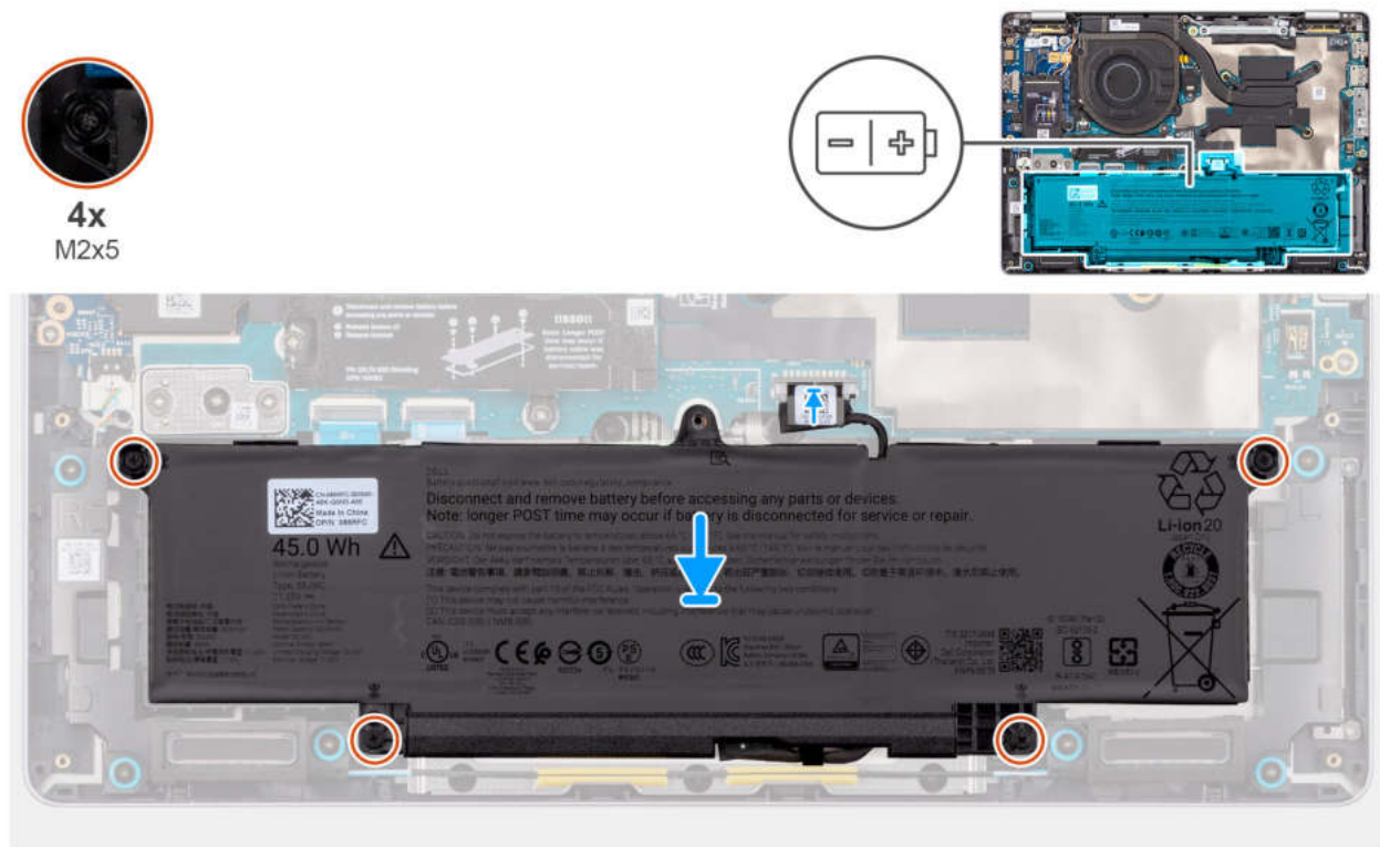
Abbildung 22. Einsetzen des Akkus
