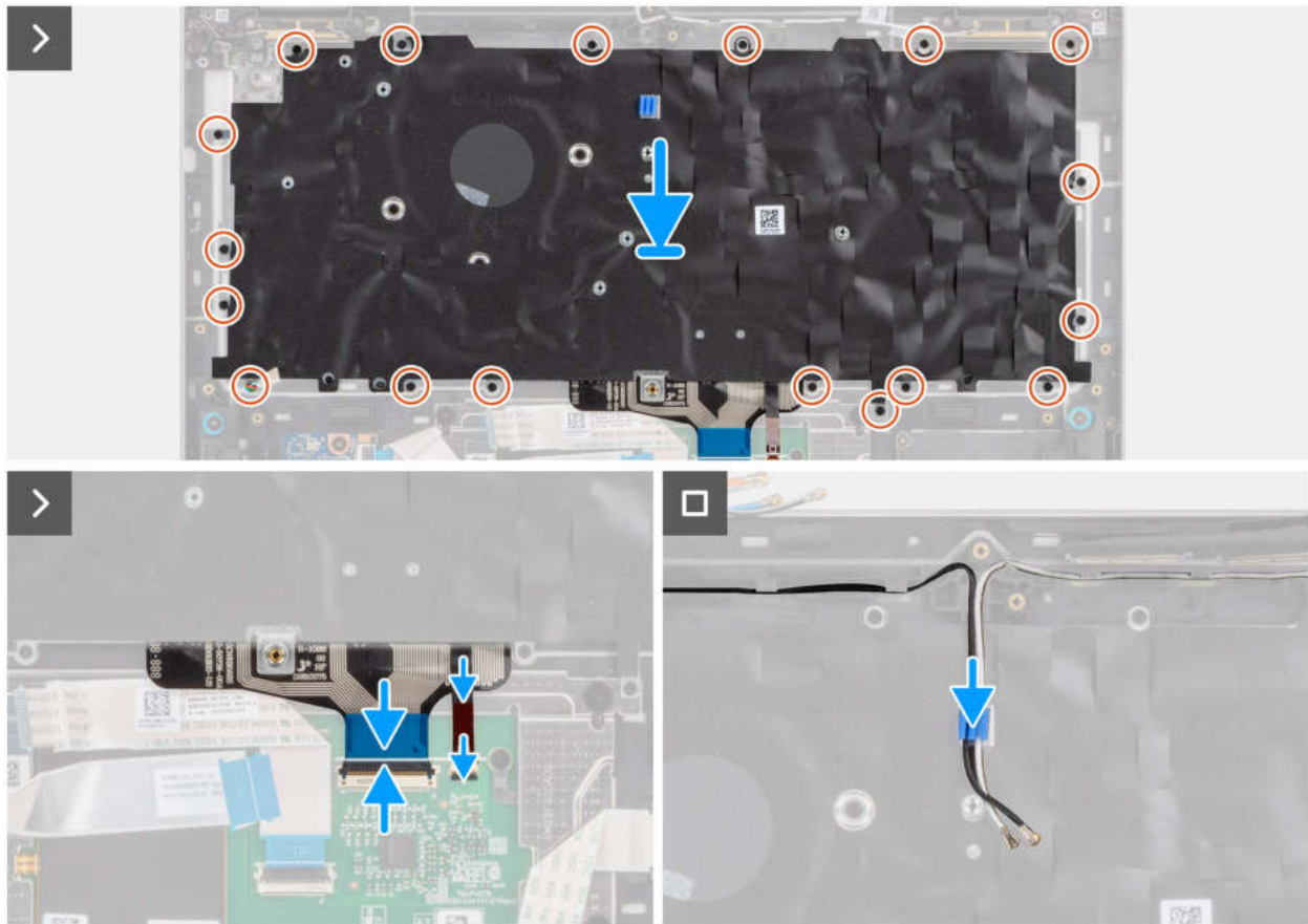
Abbildung 96. Einbauen der Tastatur
