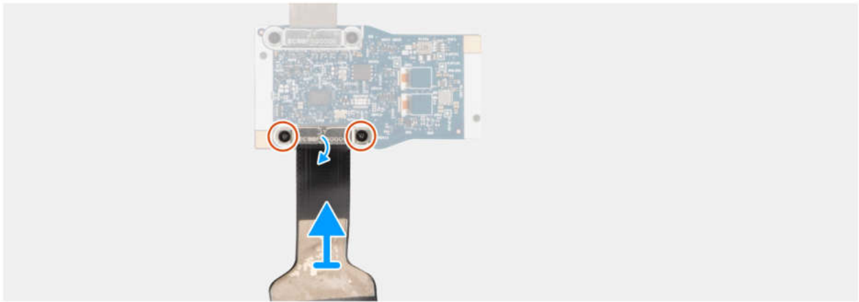
Abbildung 85. Entfernen des Bildschirmkabels für die MIPI-Kamera an der mittleren Zusatzplatine
