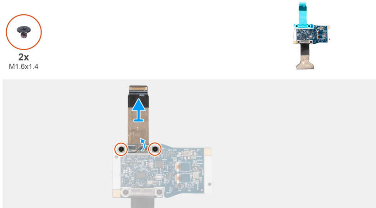
Abbildung 87. Entfernen des Kabels der mittleren Zusatzplatine
