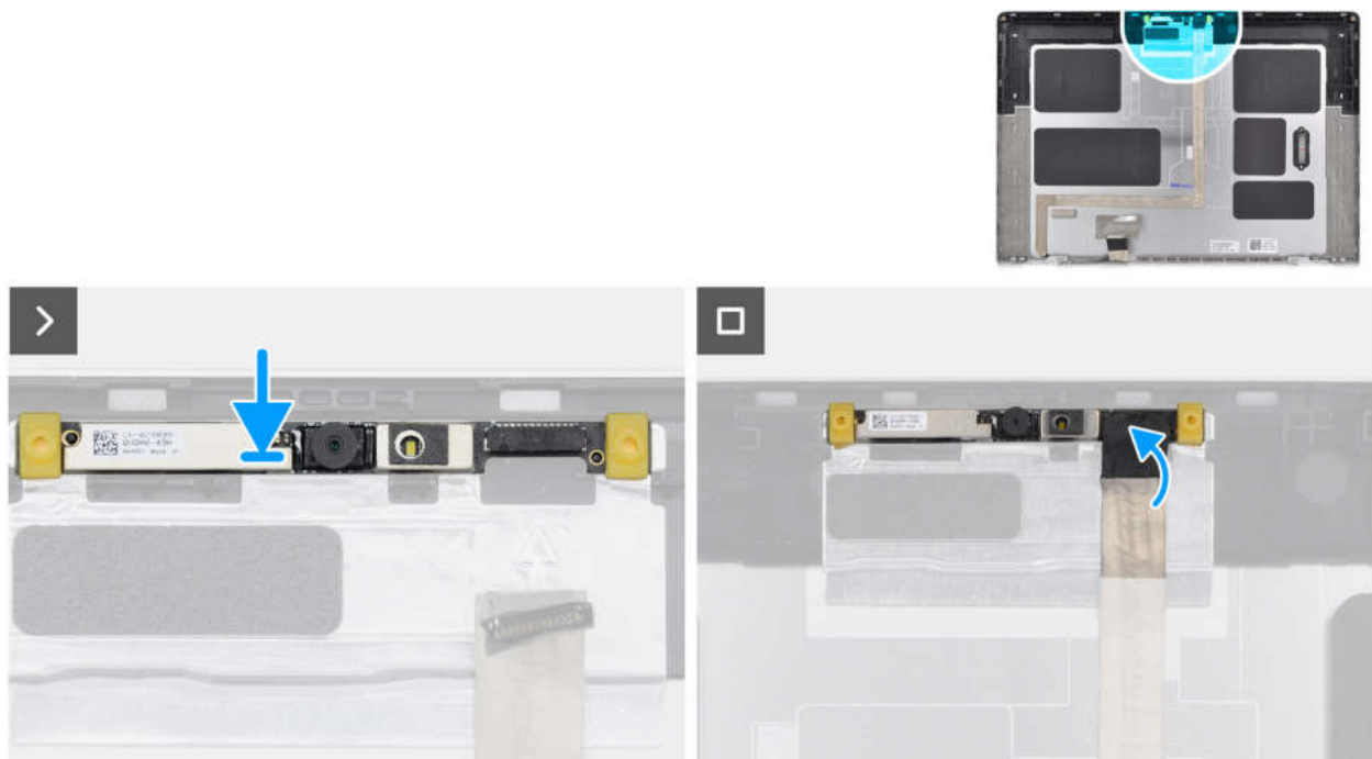
Abbildung 78. Installieren der RGB-Kamera
