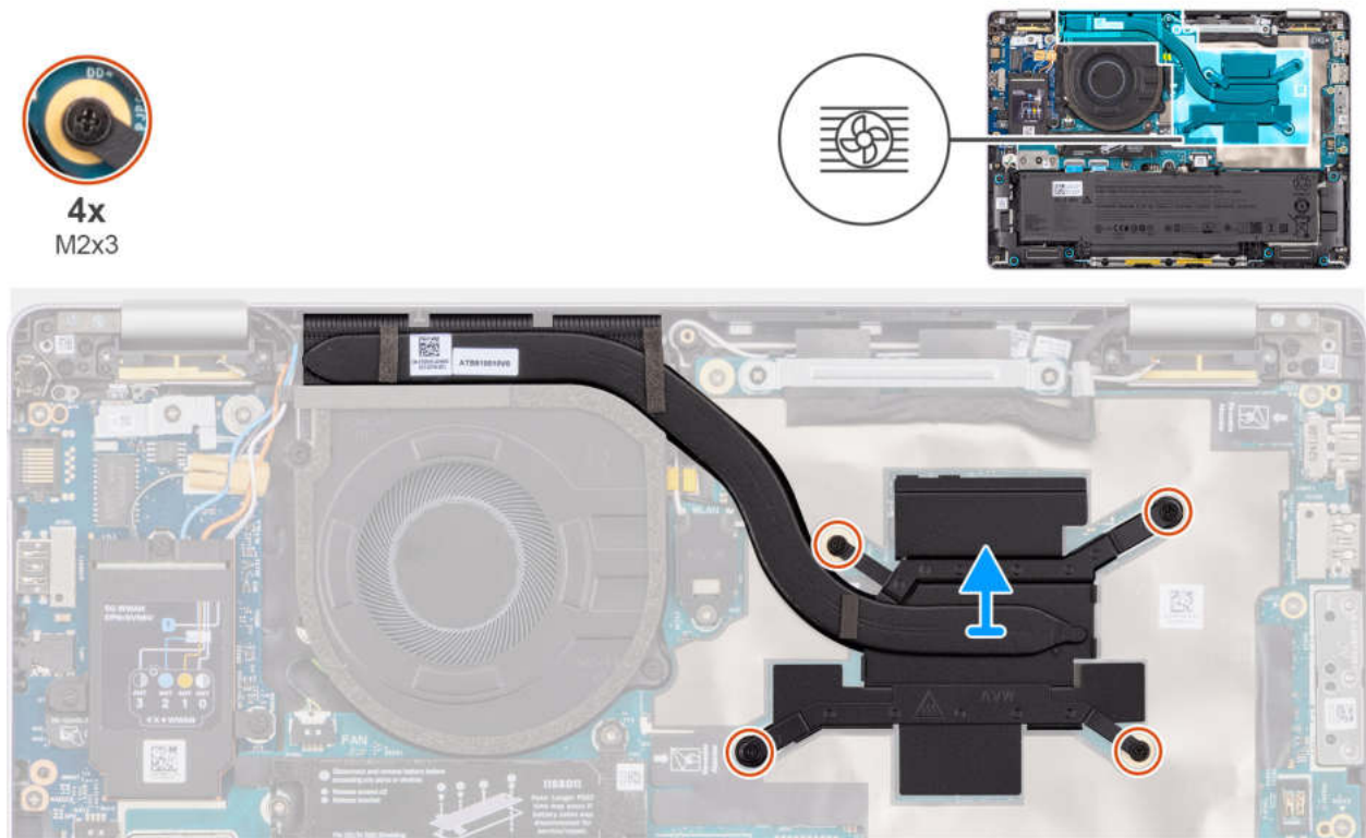
Abbildung 36. Kühlkörper entfernen
