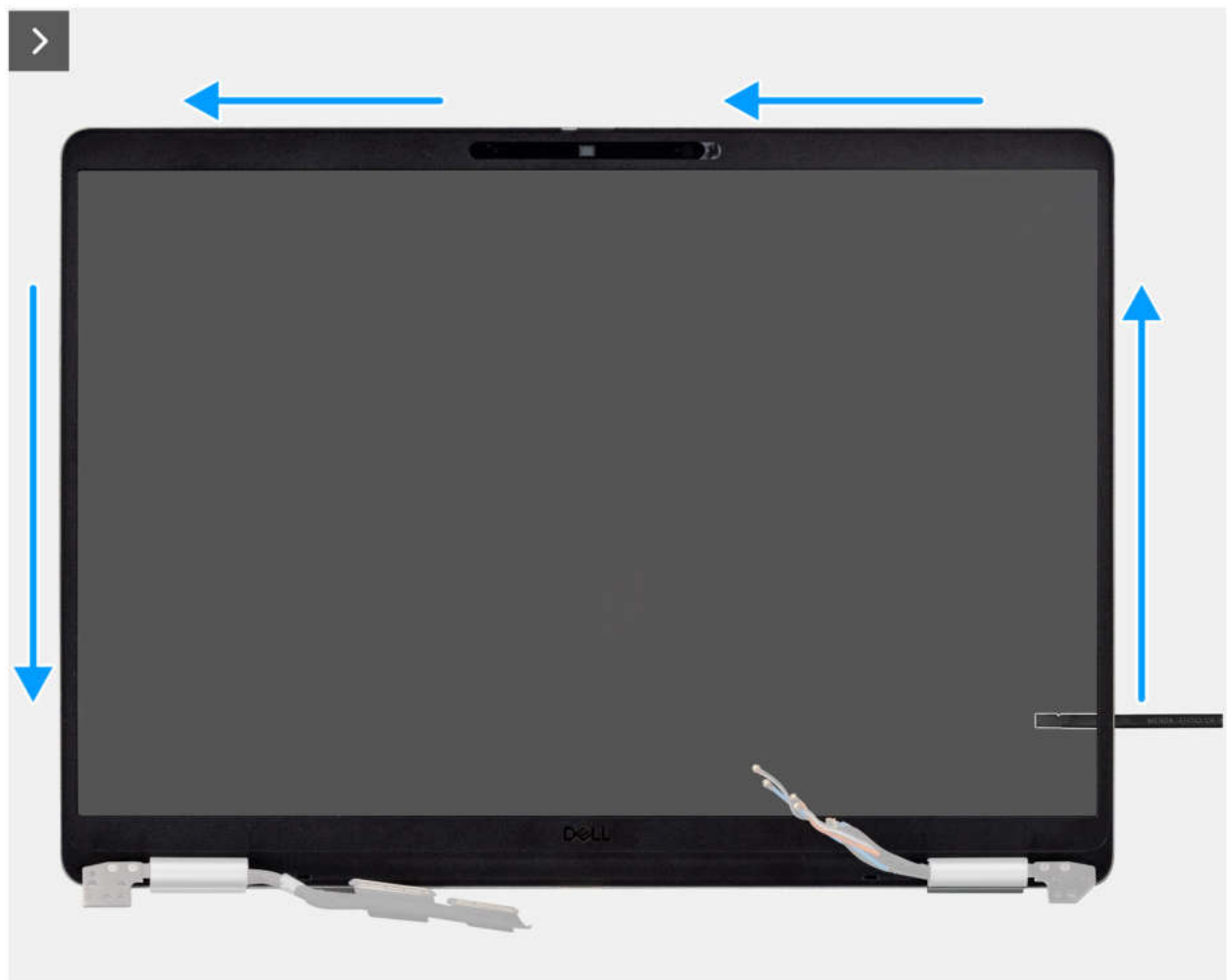
Abbildung 64. Abhebeln der Blende an den Seiten
