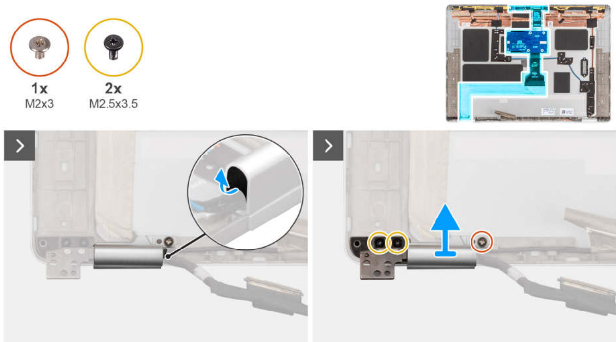
Abbildung 81. Entfernen des Bildschirmkabels der RGB/IR-Kamera
