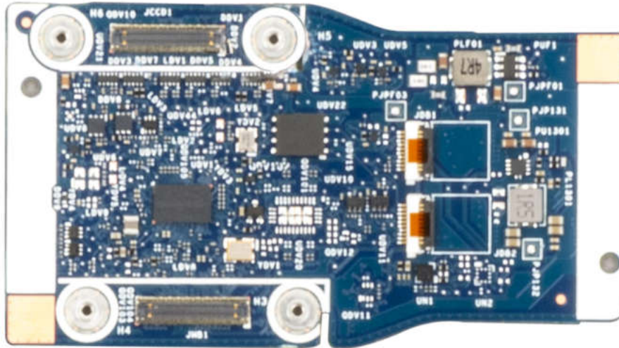
Abbildung 90. Mittlere Zusatzplatine
