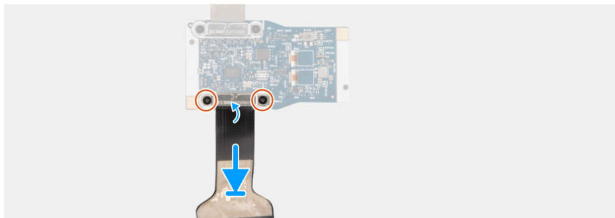
Abbildung 86. Installieren des Bildschirmkabels für die MIPI-Kamera an der mittleren Zusatzplatine
