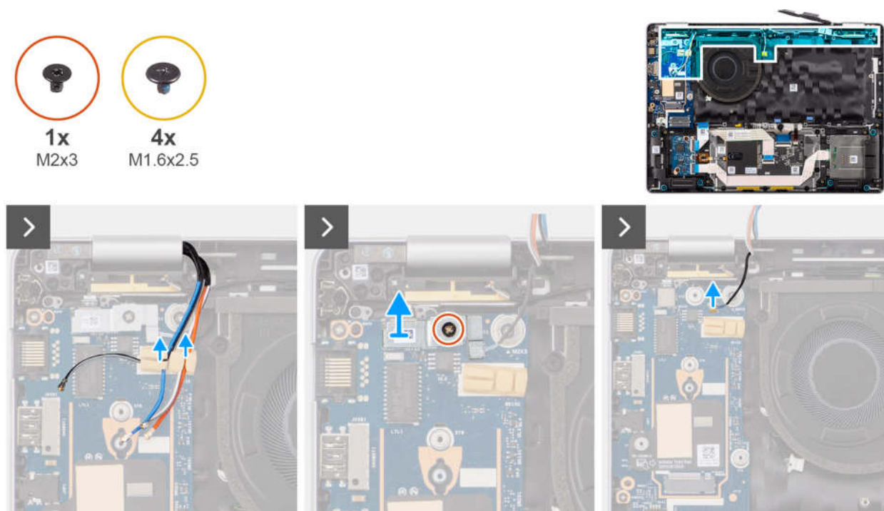
Abbildung 47. Entfernen der WLAN-Antennenmodule
