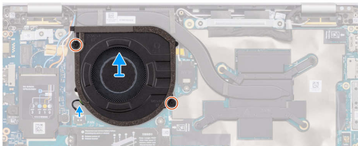
Abbildung 34. Entfernen des Lüfters
