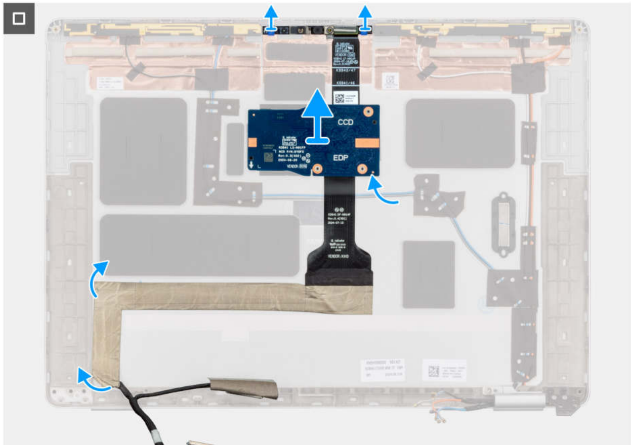
Abbildung 82. Entfernen des Bildschirmkabels der RGB/IR-Kamera
