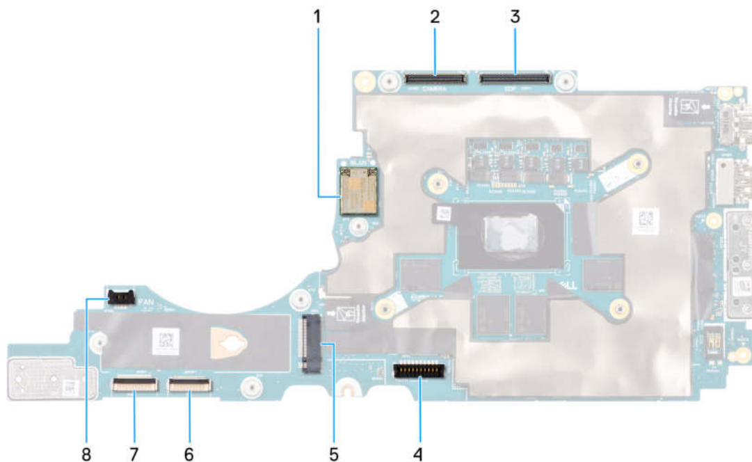
Abbildung 44. Steckplätze und Anschlüsse der Hauptplatine
