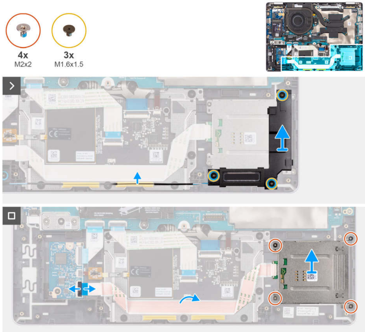
Abbildung 40. Entfernen des Smartcardlesegeräts
