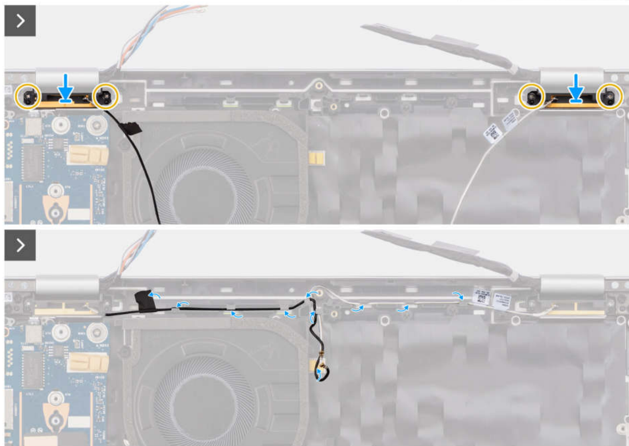
Abbildung 49. Einbauen der WLAN-Antennenmodule
