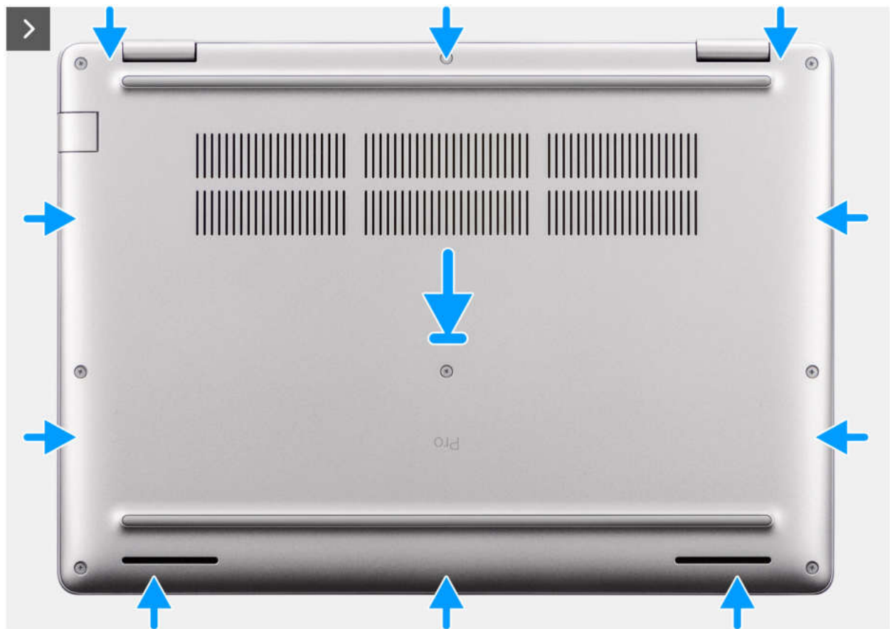
Abbildung 19. Anbringen der Bodenabdeckung
