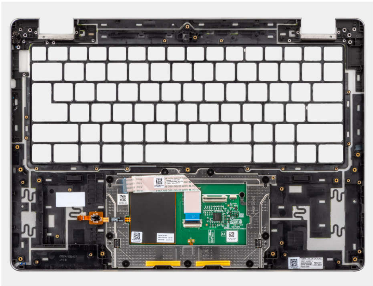
Abbildung 97. Handauflagenbaugruppe
