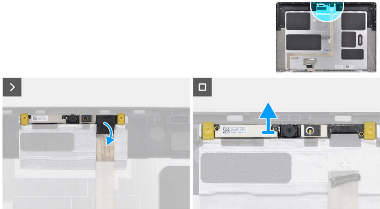
Abbildung 76. Entfernen der RGB-Kamera
