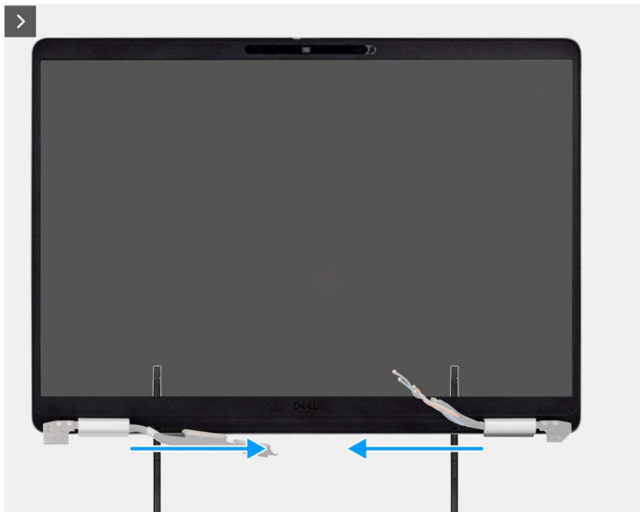
Abbildung 62. Abhebeln der Blende entlang der Scharniere
