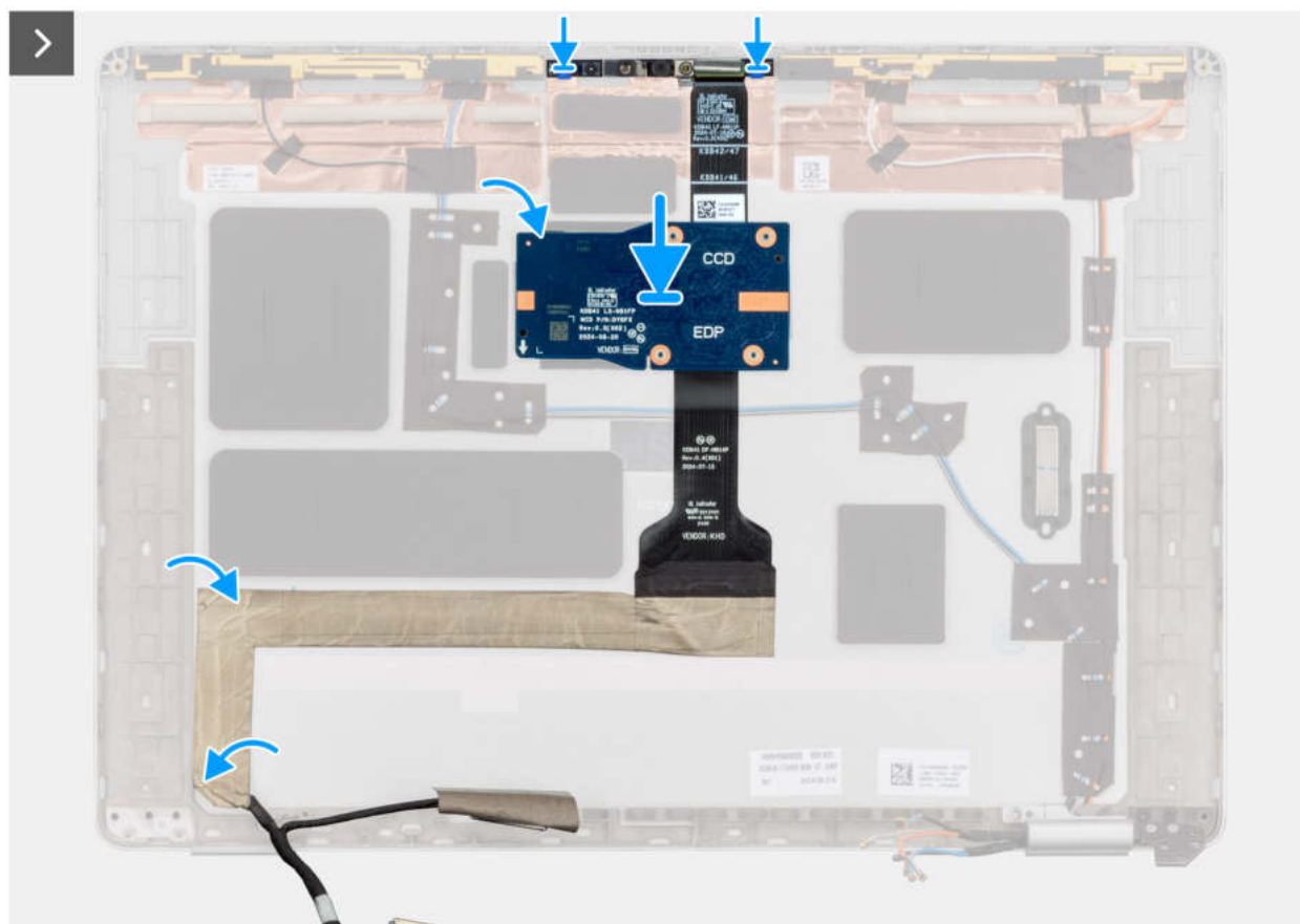
Abbildung 83. Installieren des Bildschirmkabels der RGB/IR-Kamera
