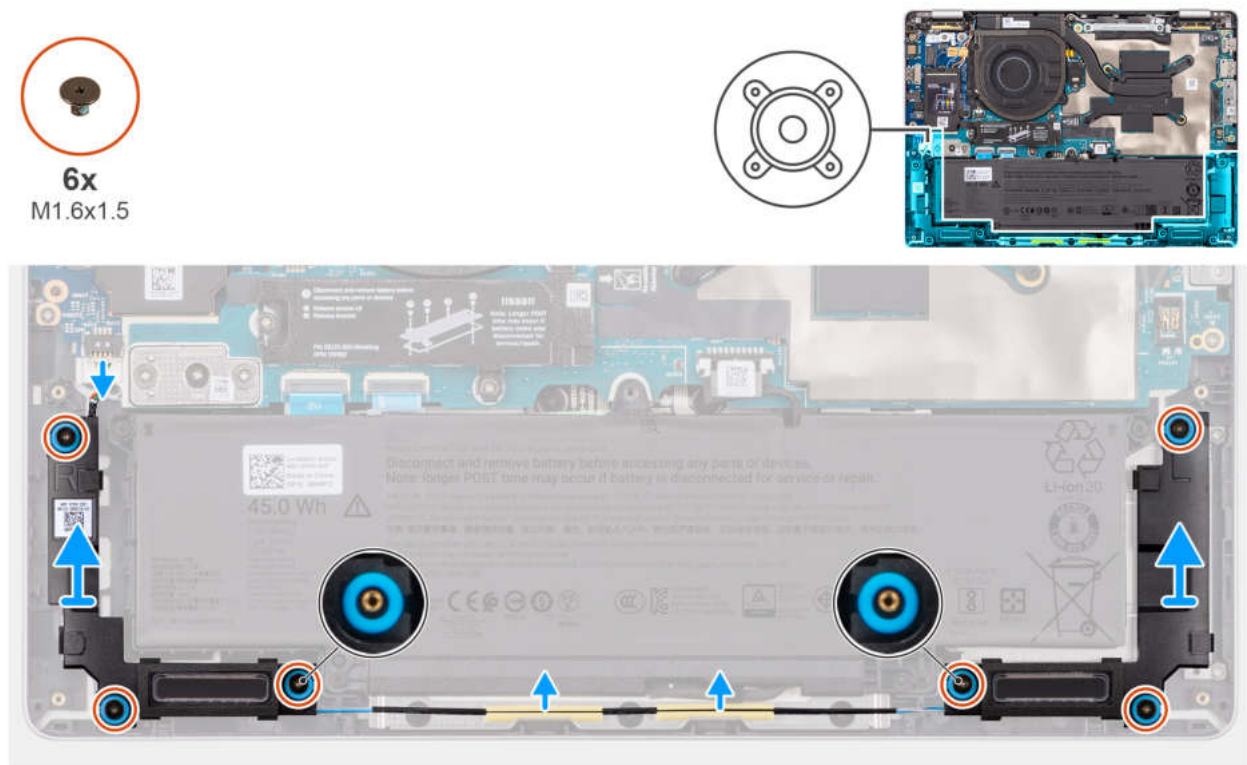
Abbildung 31. Entfernen der Lautsprecher
