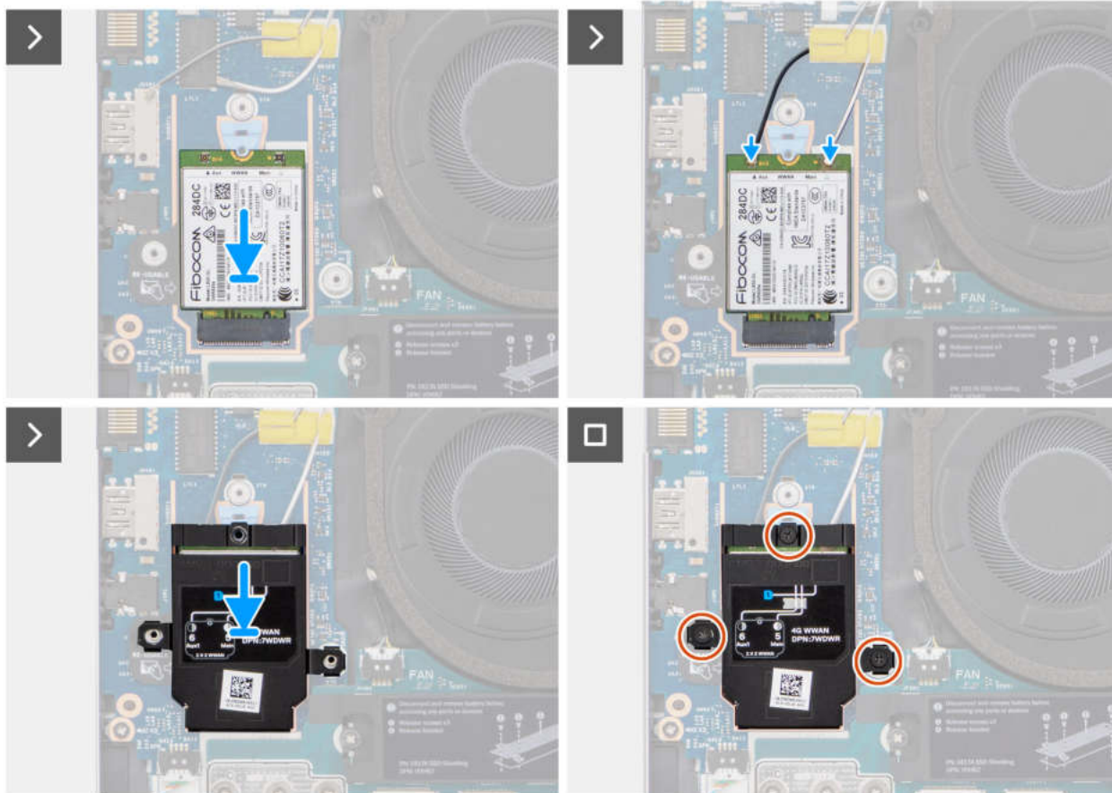
Abbildung 26. Installieren der 4G-WWAN-Karte
