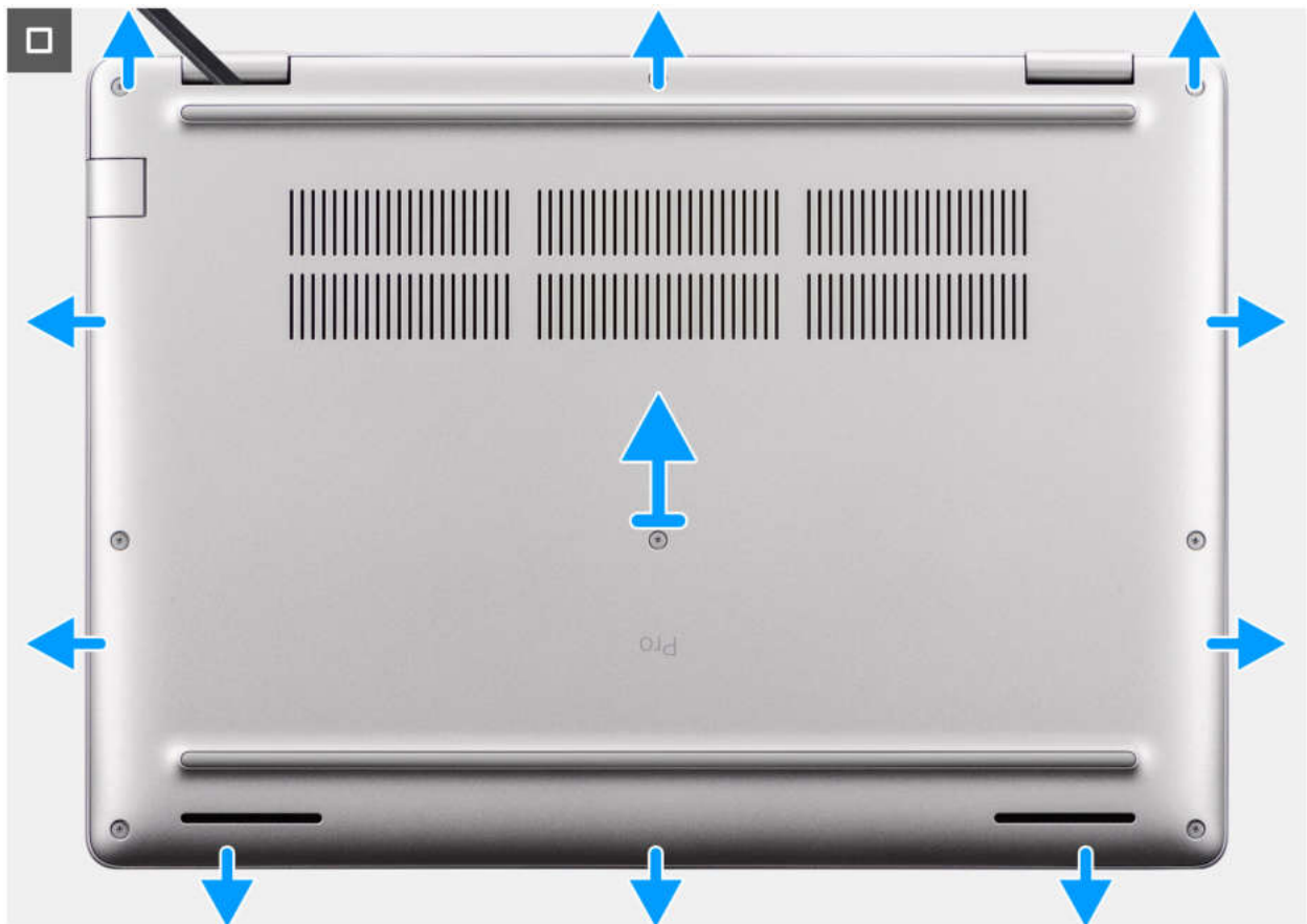
Abbildung 18. Entfernen der Bodenabdeckung
