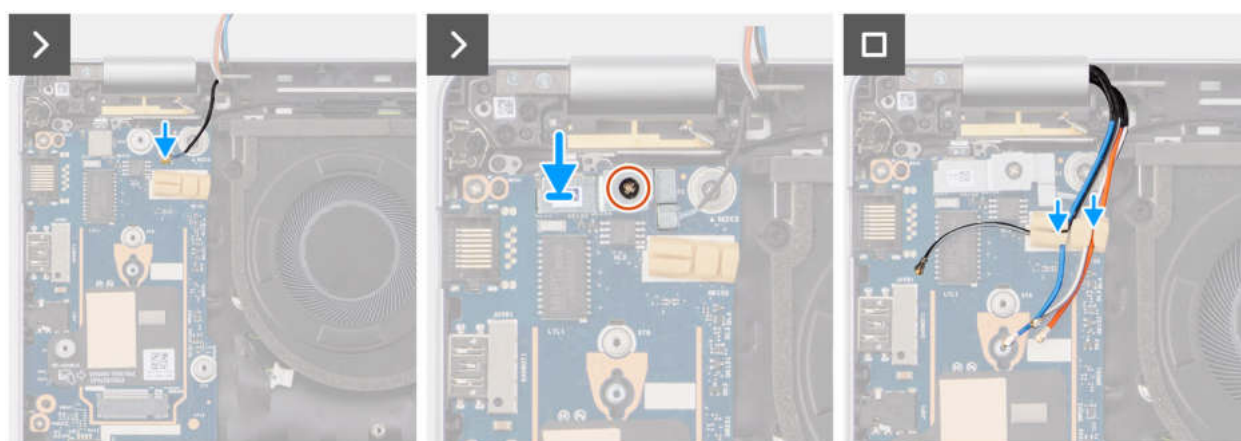
Abbildung 50. Einbauen der WLAN-Antennenmodule
