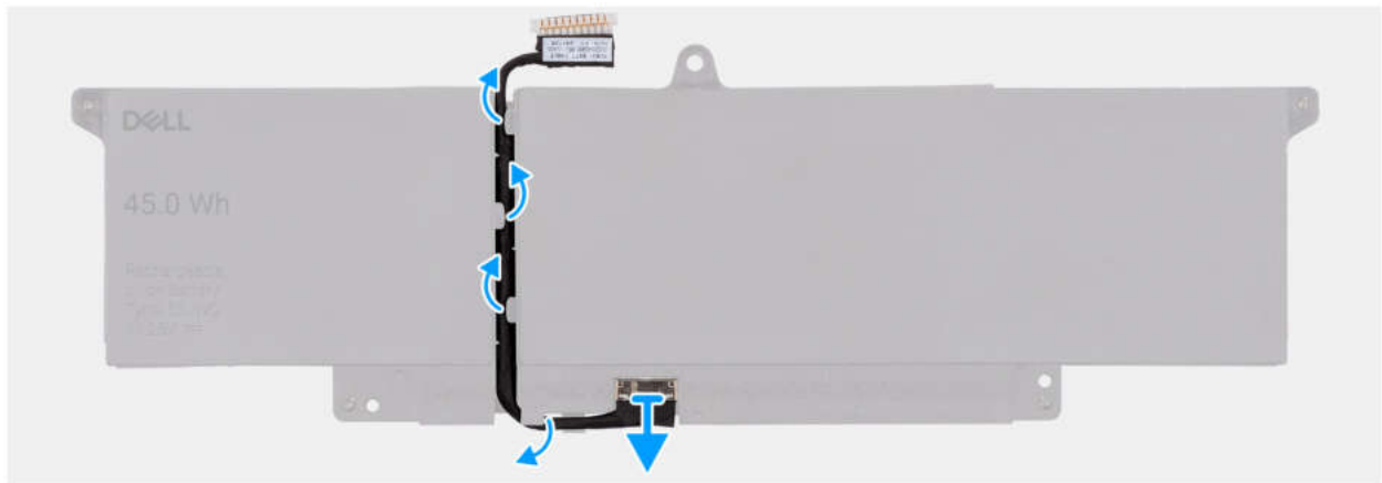
Abbildung 23. Entfernen des Akkukabels
