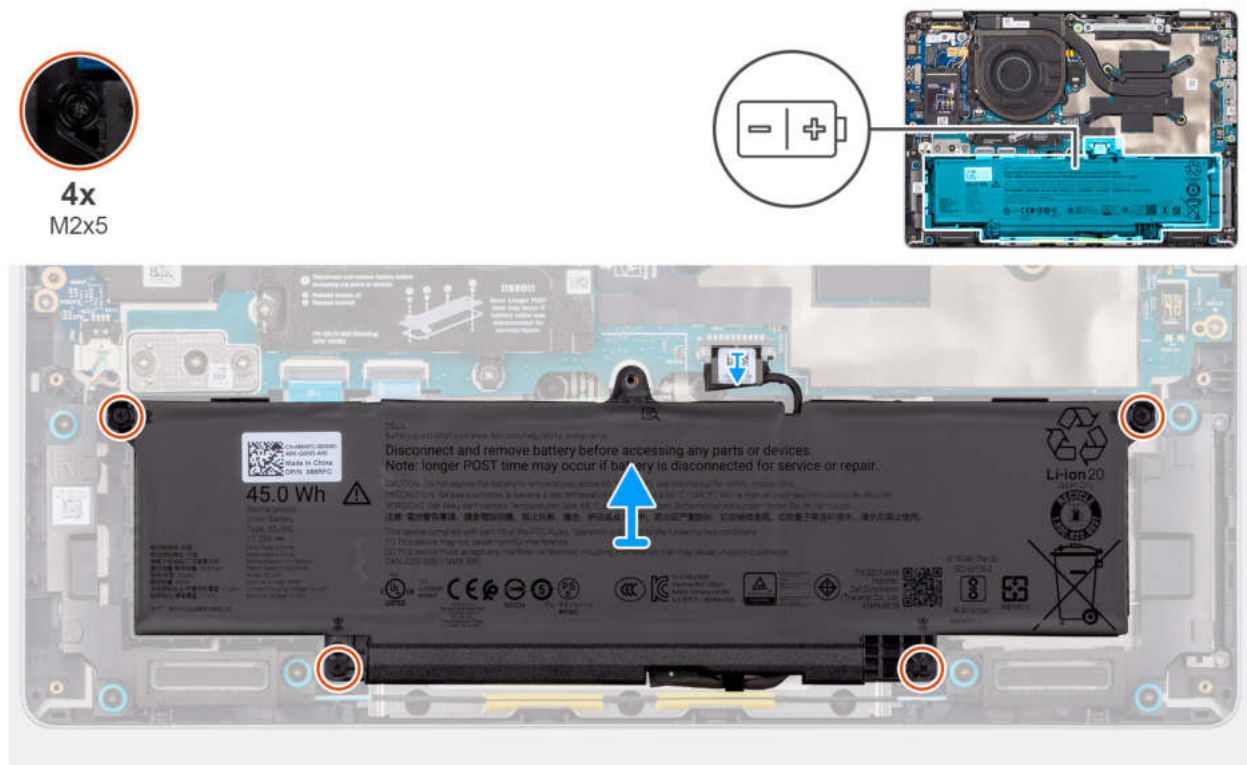
Abbildung 21. Entfernen des Akkus
