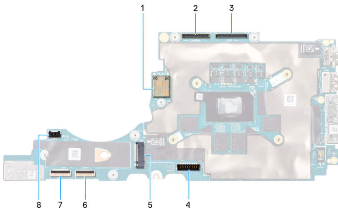
Abbildung 42. Steckplätze und Anschlüsse der Hauptplatine
