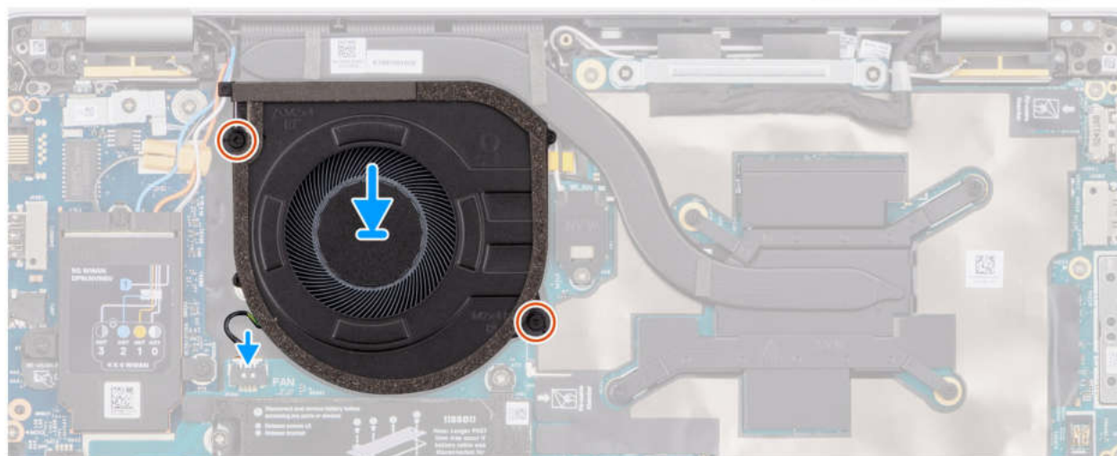
Abbildung 35. Einbauen des Lüfters
