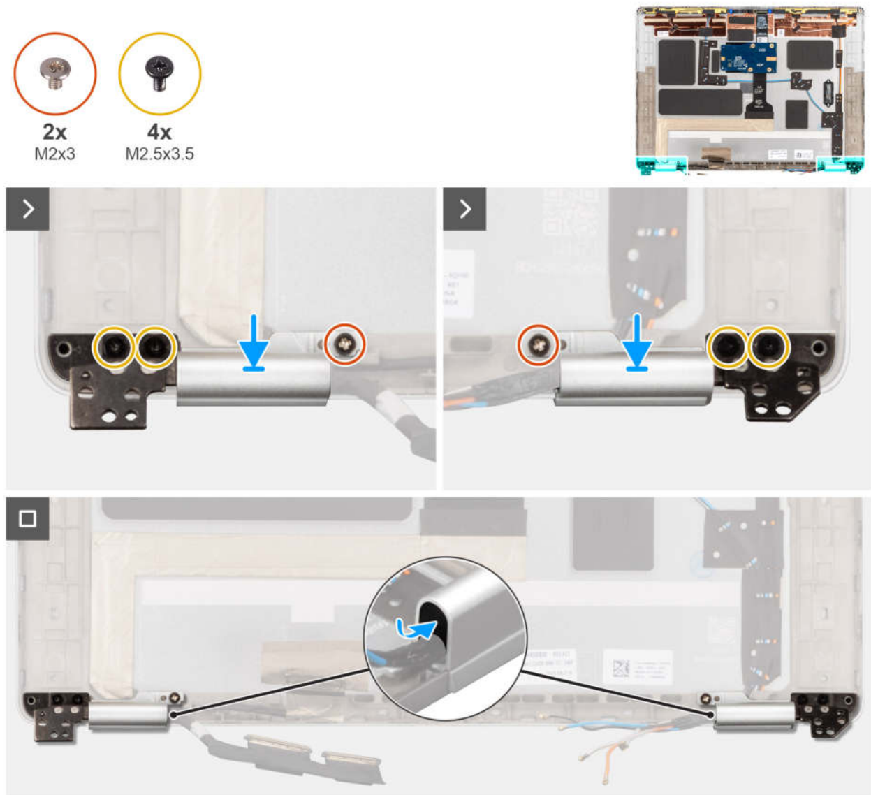
Abbildung 74. Einbauen der Scharnierabdeckungen
