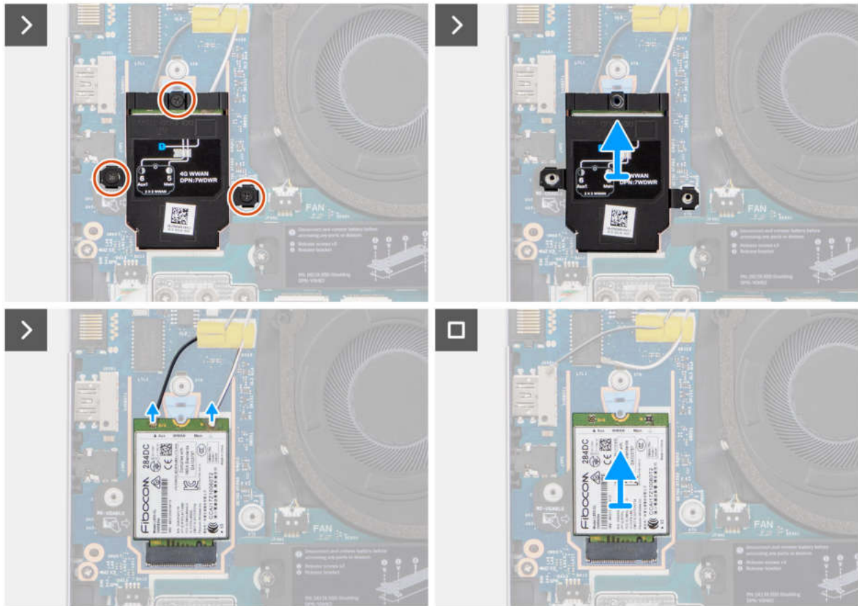
Abbildung 25. Entfernen der 4G-WWAN-Karte
