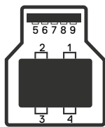
Figure 6. Connecteur USB type B en amont
