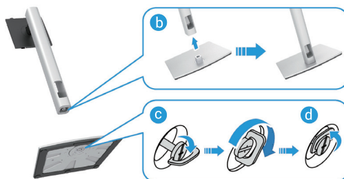
Figure 14. Installez la colonne de support et le socle
