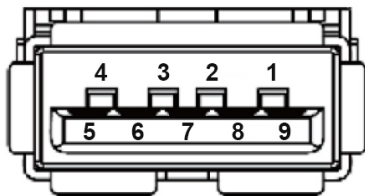
Figure 7. Connecteur USB type A 9 broches
