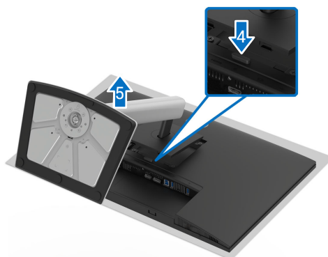
Figure 24. Enlever le socle du moniteur
