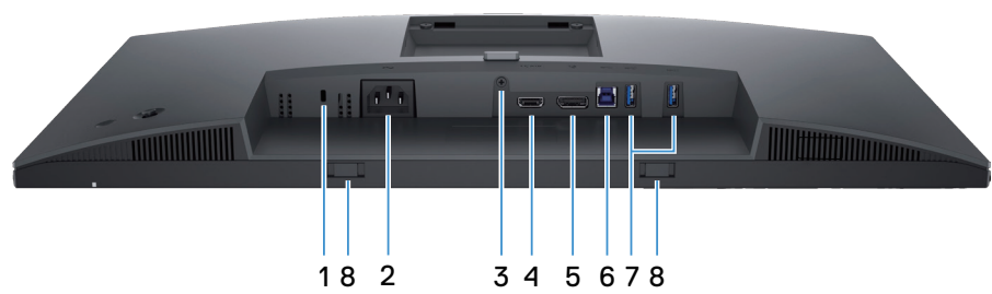
Figure 3. Vue de dessous
