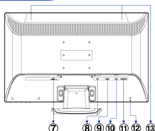
<Rückseite1 (PLE2407HDS) >
