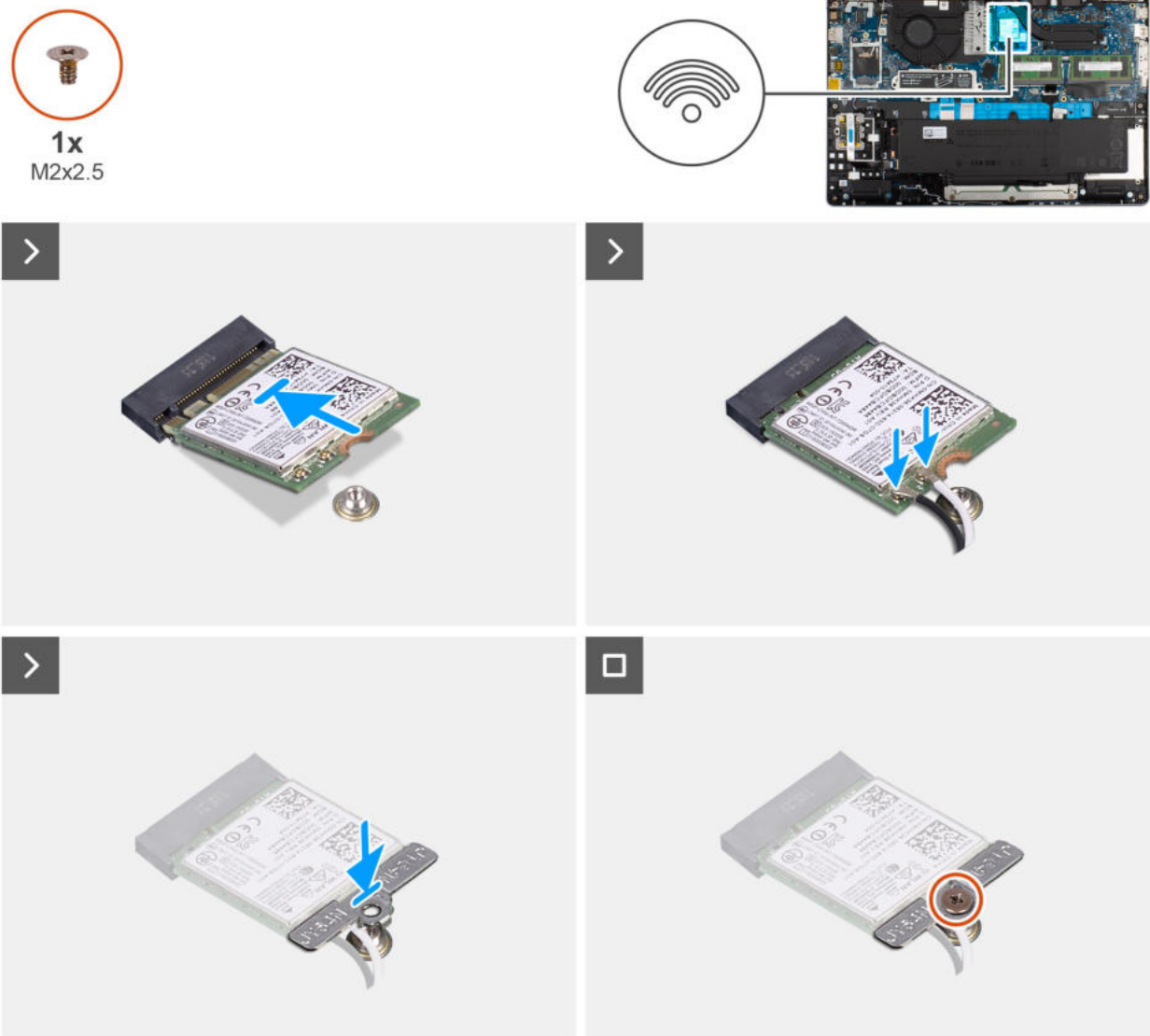
Abbildung 36. Einbauen der WLAN-Karte
