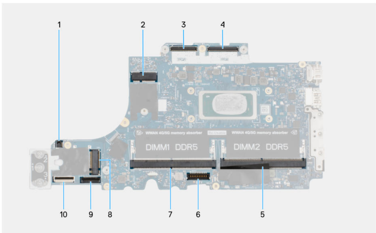
Abbildung 54. Hauptplattenanschluss
