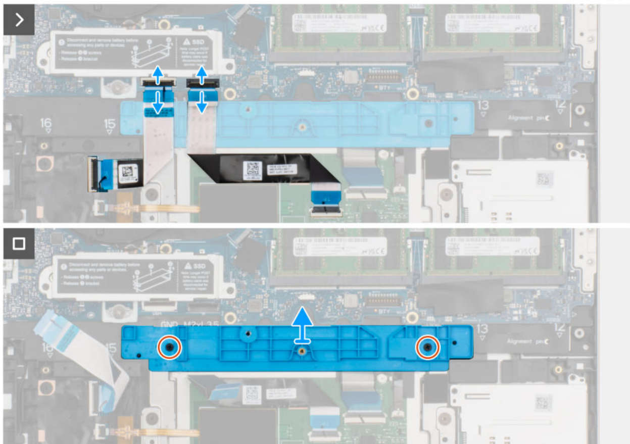
Abbildung 47. Entfernen der Akkuhalterung
