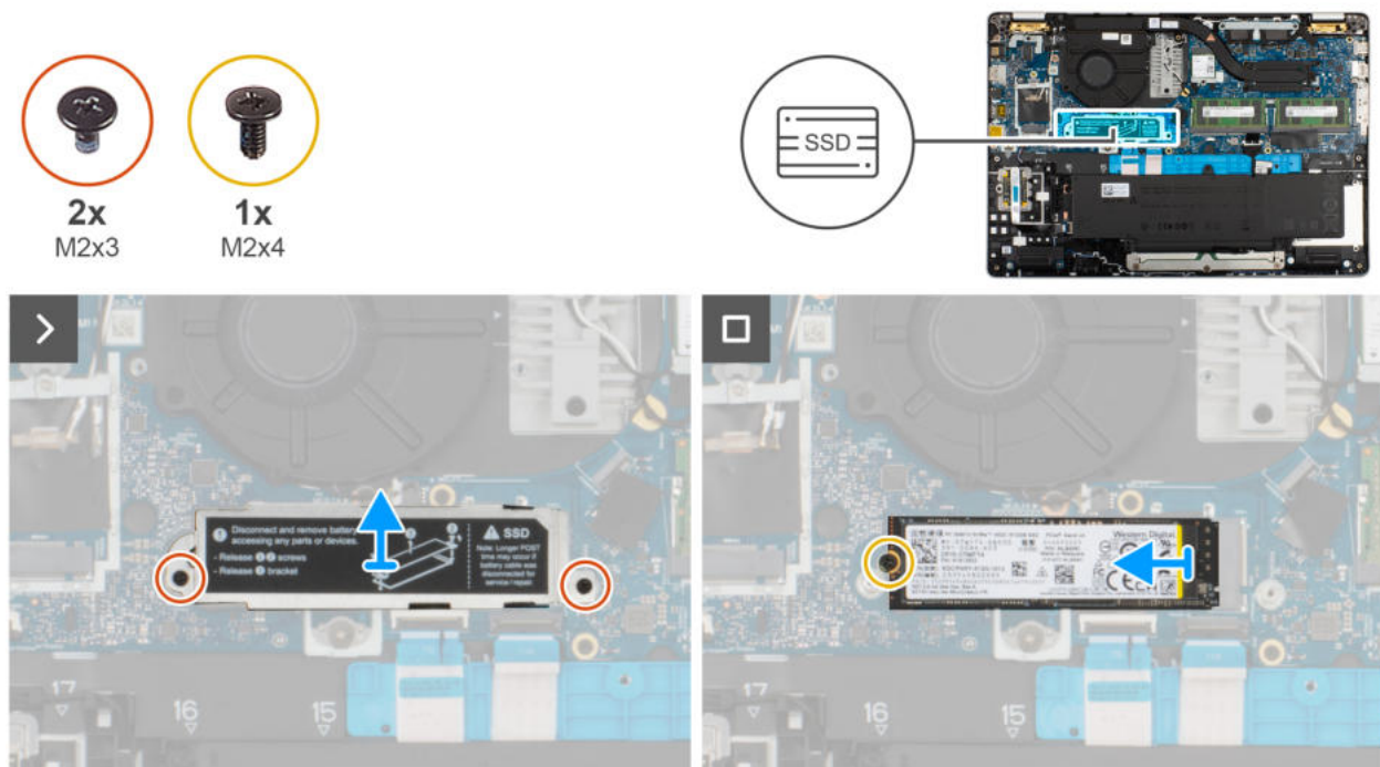
Abbildung 26. Entfernen des M.2-2280-SSD-Laufwerks
