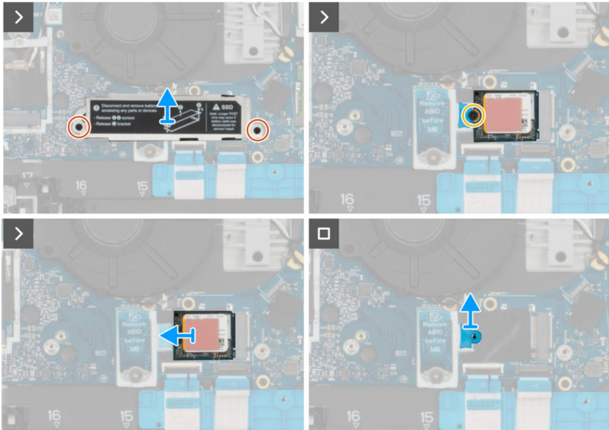
Abbildung 24. Entfernen des M.2-2230-Solid-State-Laufwerks
