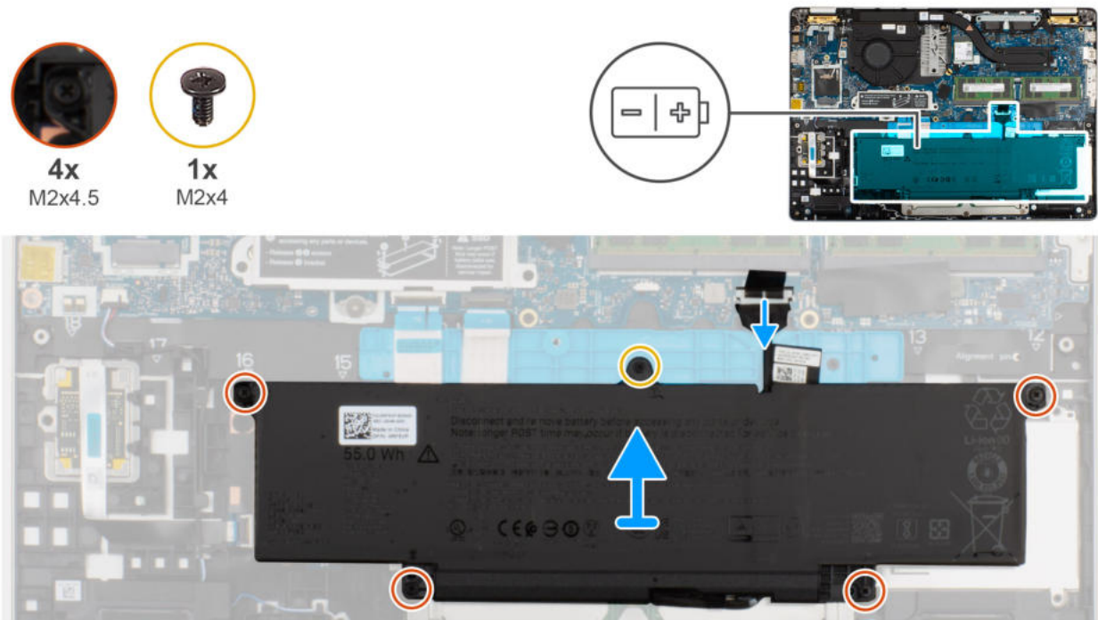
Abbildung 18. Entfernen des Akkus
