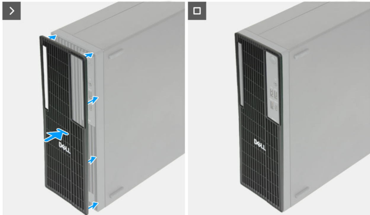
Abbildung 15. Installieren des Staubfilters
