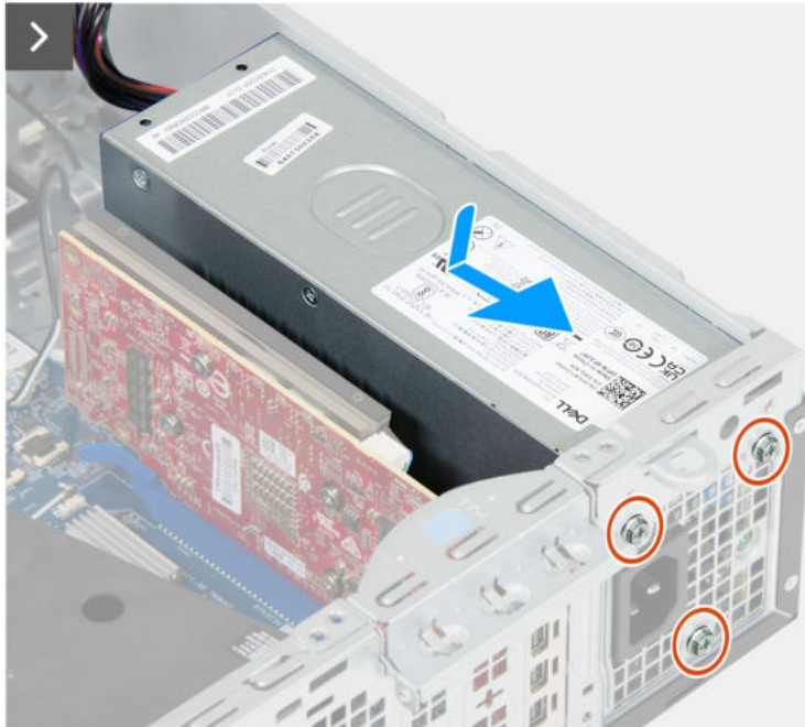
Abbildung 49. Installieren der Stromversorgungseinheit
