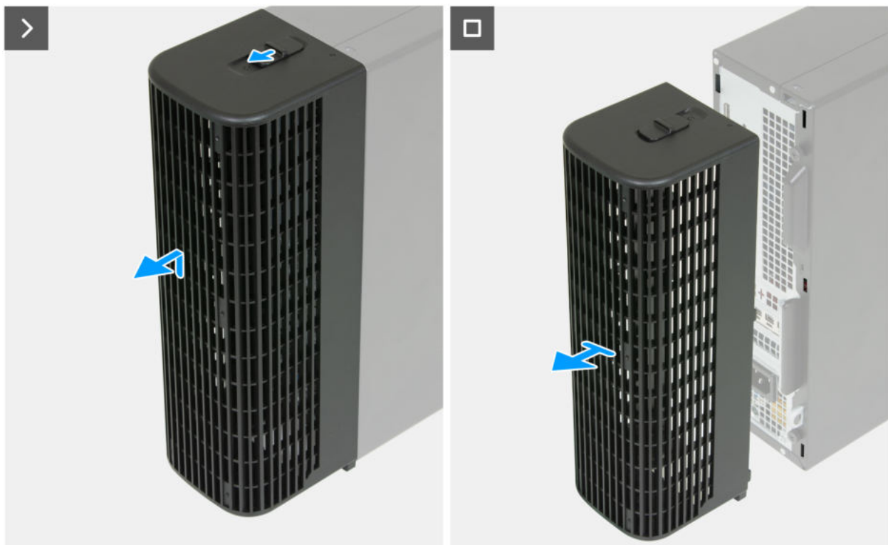
Abbildung 4. Entfernen der Kabelabdeckung
