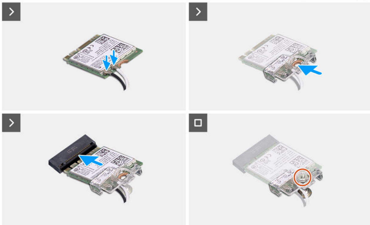
Abbildung 30. Installieren der Wireless-Karte
