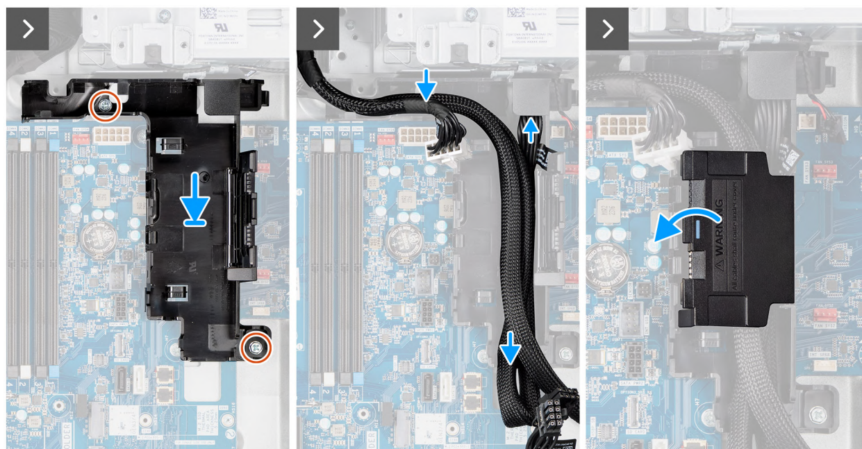
Afbeelding 96. De systeemkaart installeren
