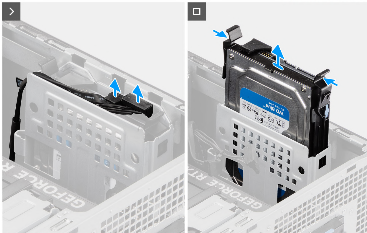
Afbeelding 26. De 3,5-inch harde-schijf eenheid verwijderen (bay-2)
