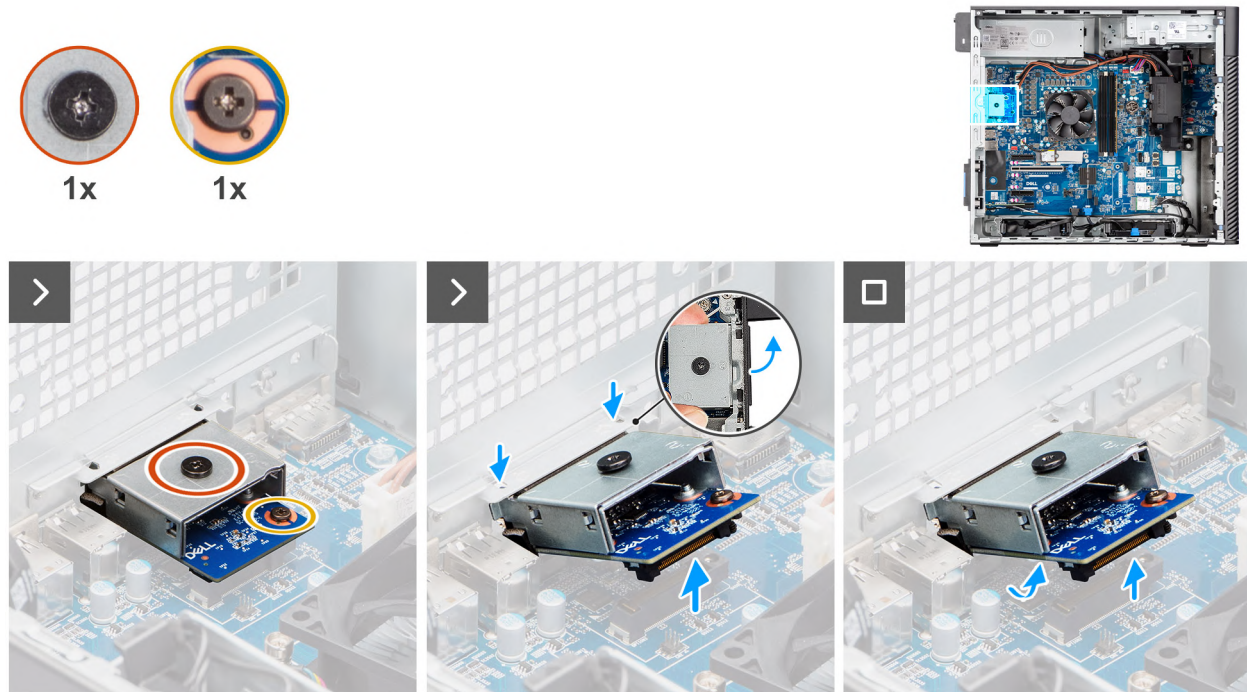
Afbeelding 85. De optionele VGA-module verwijderen
