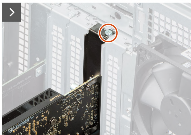
Afbeelding 38. De grafische kaart plaatsen
