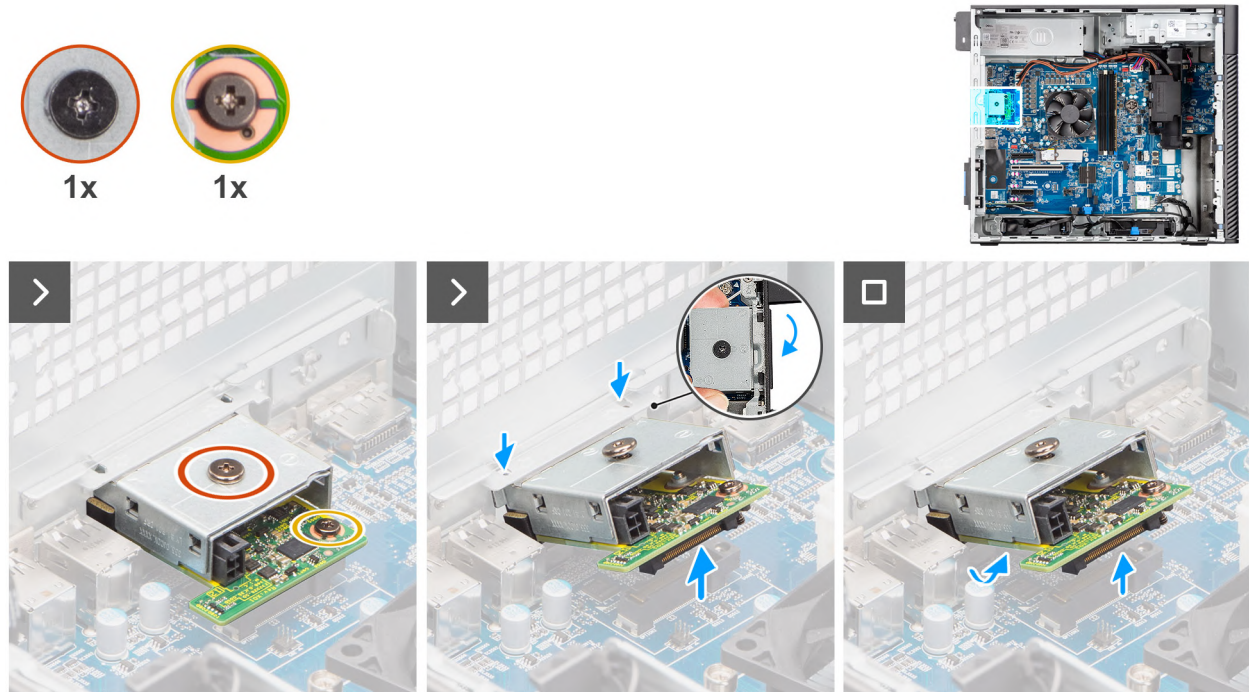
Afbeelding 79. De optionele Thunderbolt-module verwijderen
