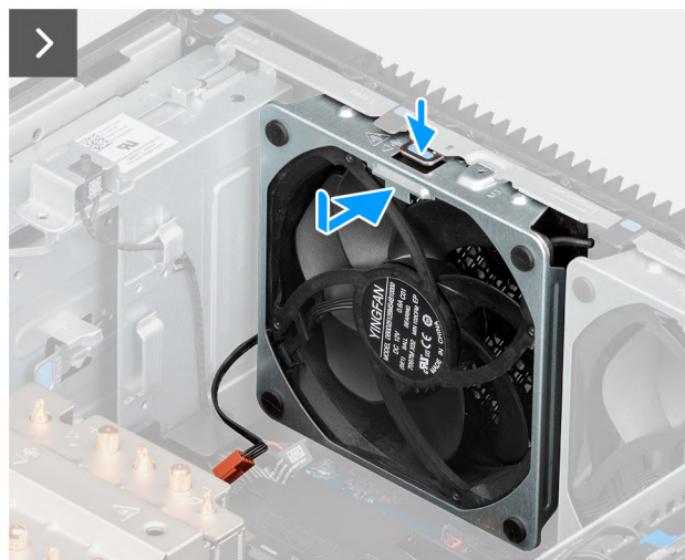
Afbeelding 47. Voorste ventilator 1
