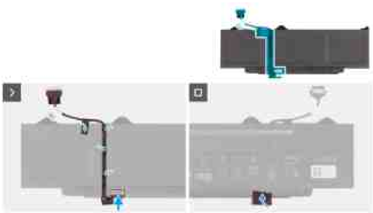
Abbildung 44. Einsetzen des Akkukabels
