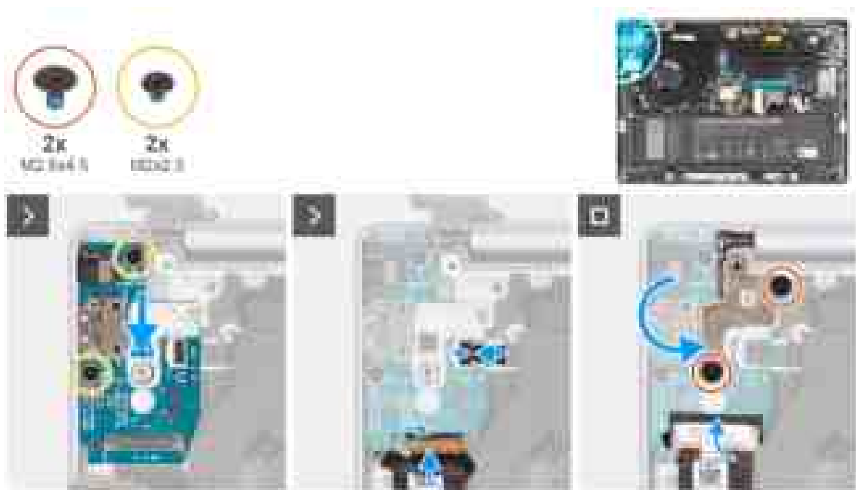
Abbildung 84. Installation der I/O-Platine (bei Computern nur mit WLAN-Unterstützung)
