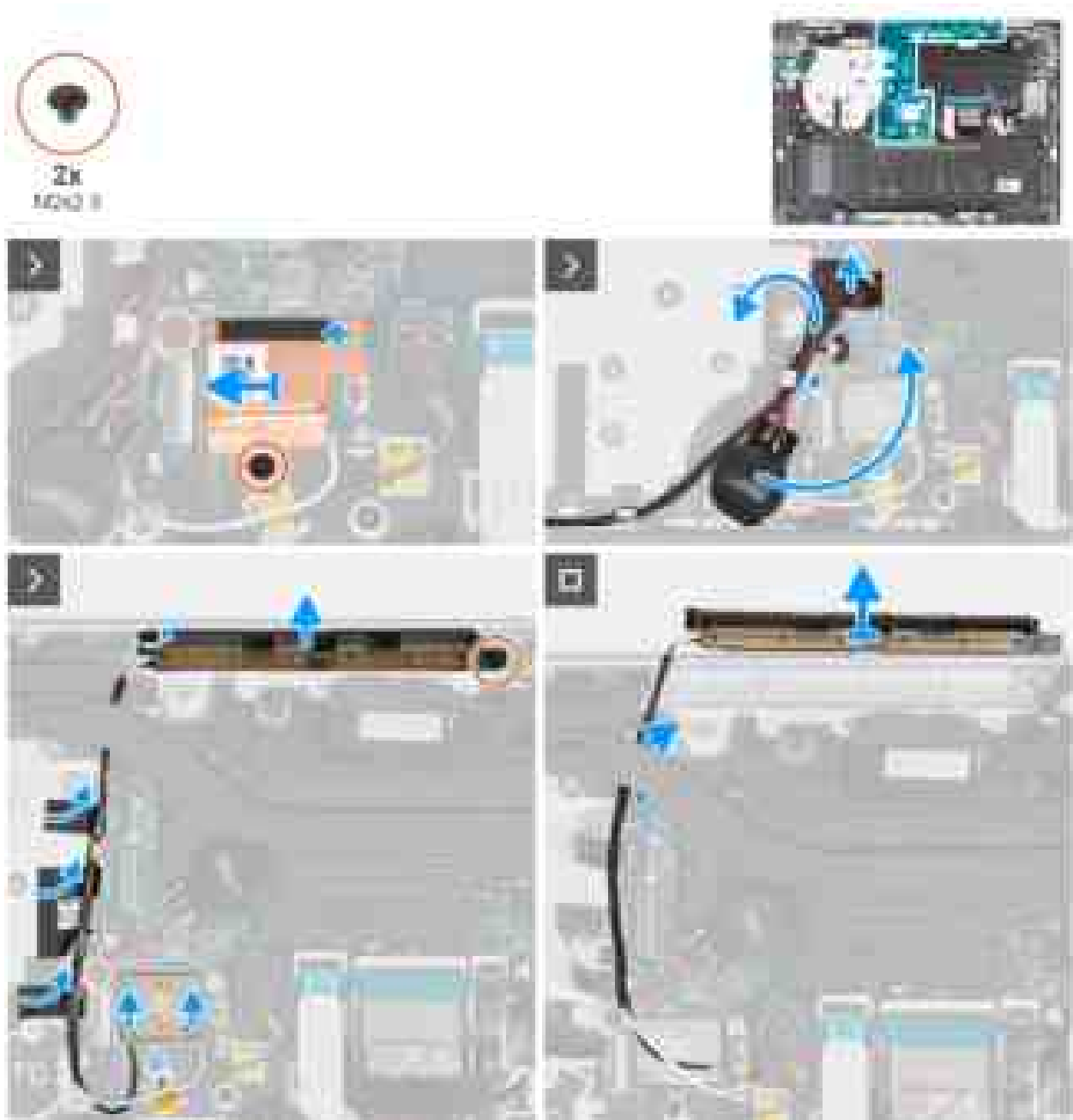
Abbildung 59. Entfernen des WLAN-Antennenmoduls (bei Computern nur mit WLAN-Unterstützung)
