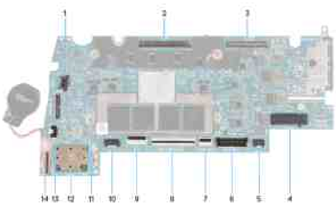
Abbildung 94. Hauptplattenanschlüsse
