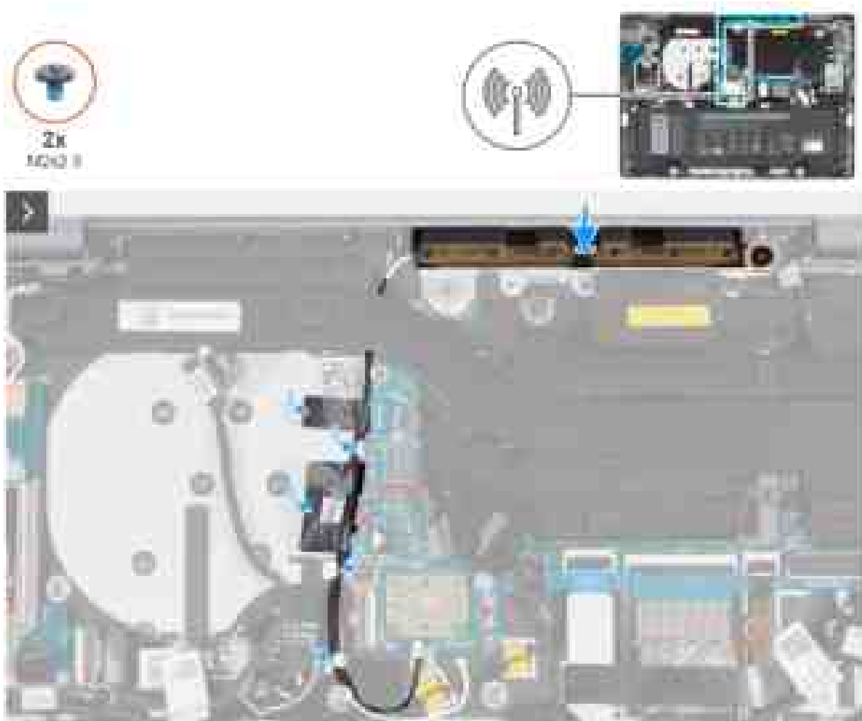
Abbildung 70. Installieren des WLAN-Antennenmoduls (bei Computern mit WWAN-Unterstützung)
