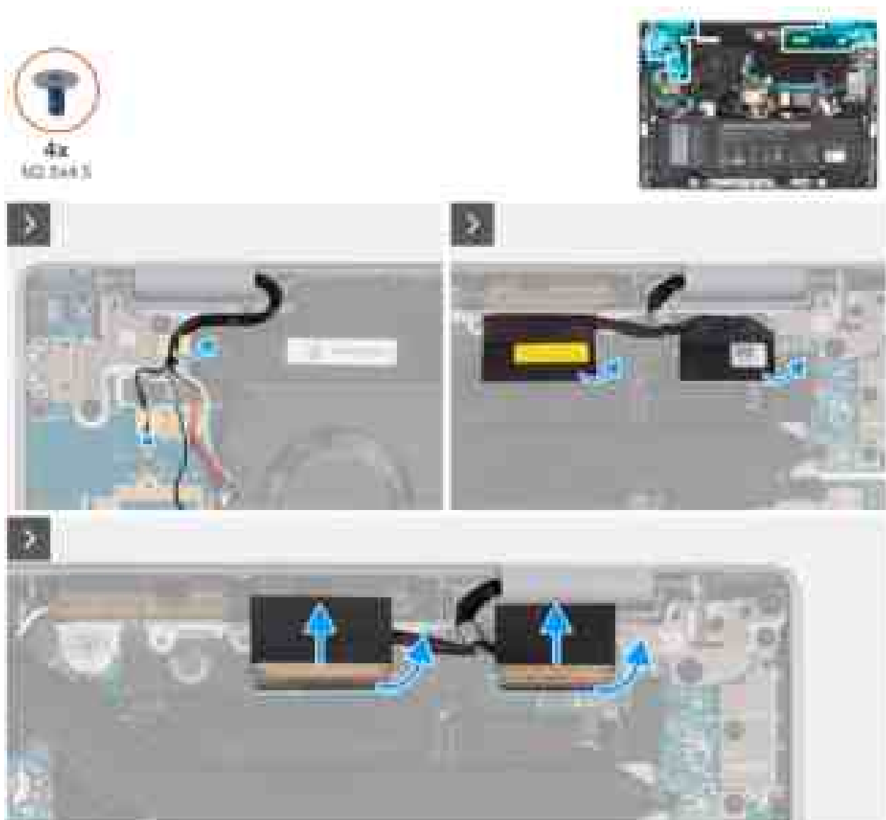
Abbildung 78. Entfernen der Bildschirmbaugruppe (bei Computern mit WWAN-Unterstützung)
