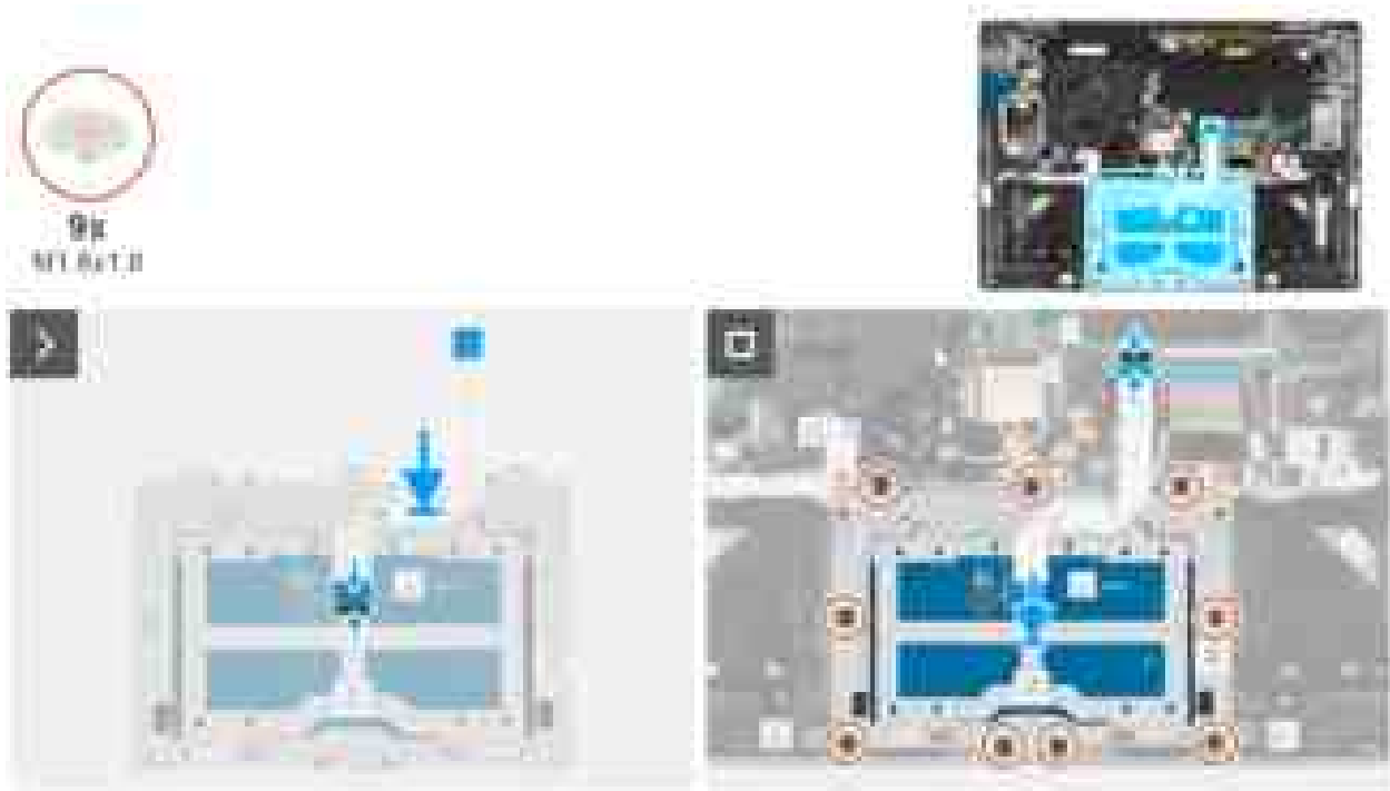
Abbildung 88. Installieren der Touchpad-Baugruppe
