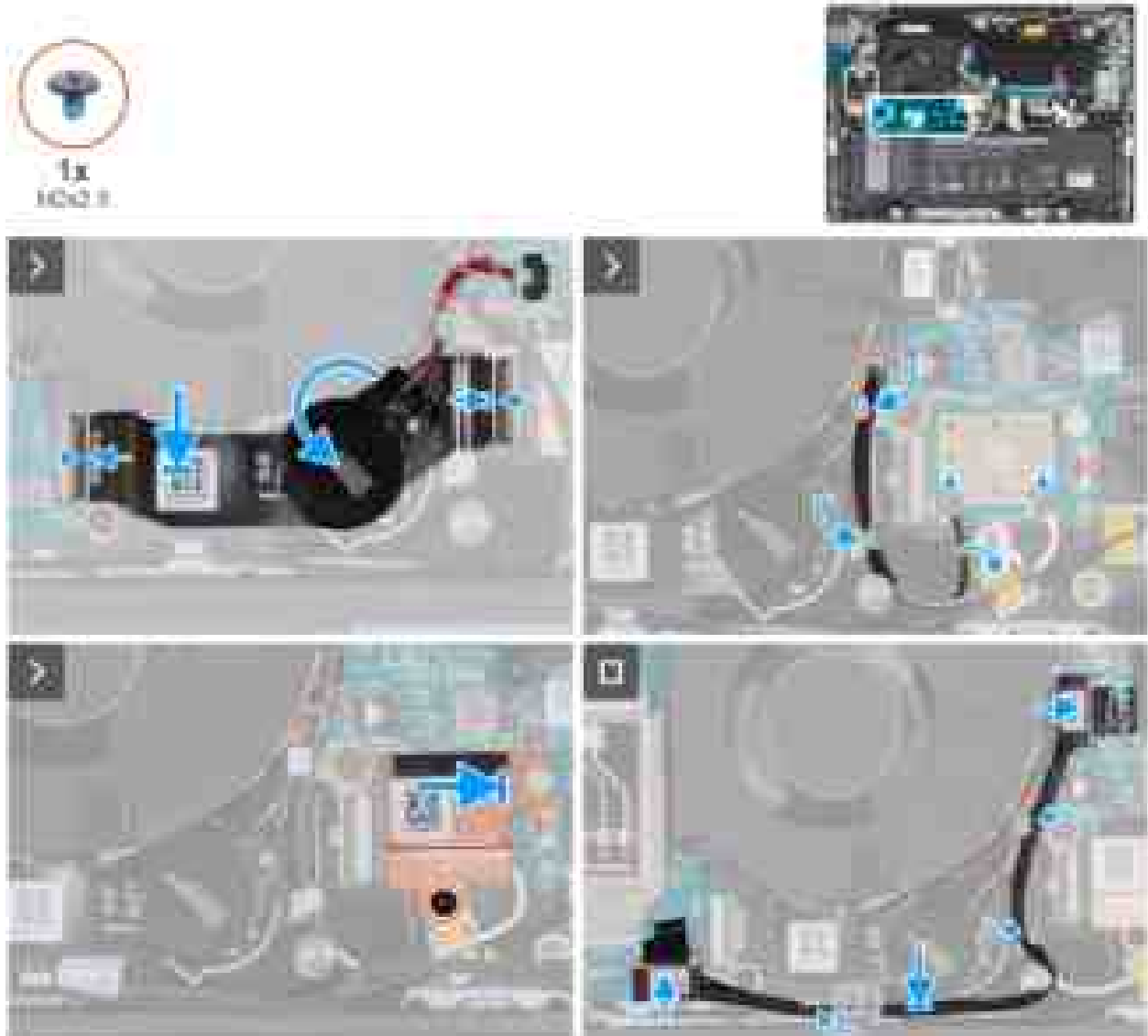
Abbildung 58. Installieren des FPC-Kabels der I/O-Platine
