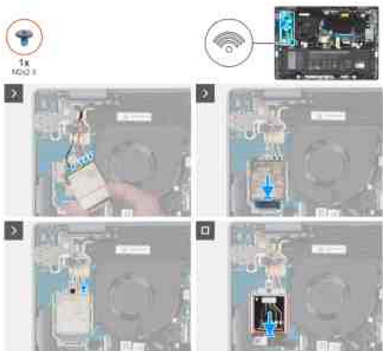
Abbildung 29. Einbauen der 5G-WWAN-Karte
