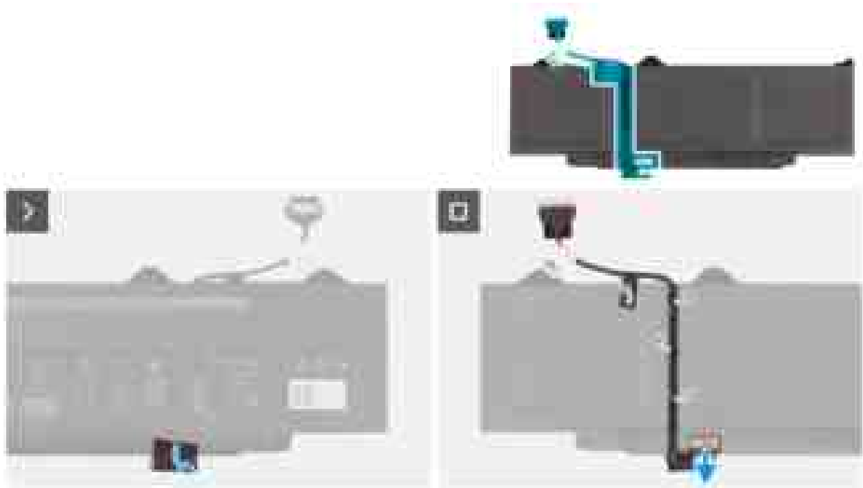
Abbildung 42. Entfernen des Akkukabels
