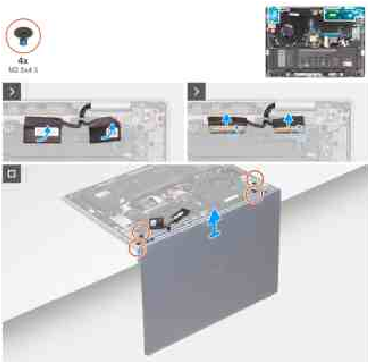
Abbildung 75. Entfernen der Bildschirmbaugruppe (bei Computern nur mit WLAN-Unterstützung)
