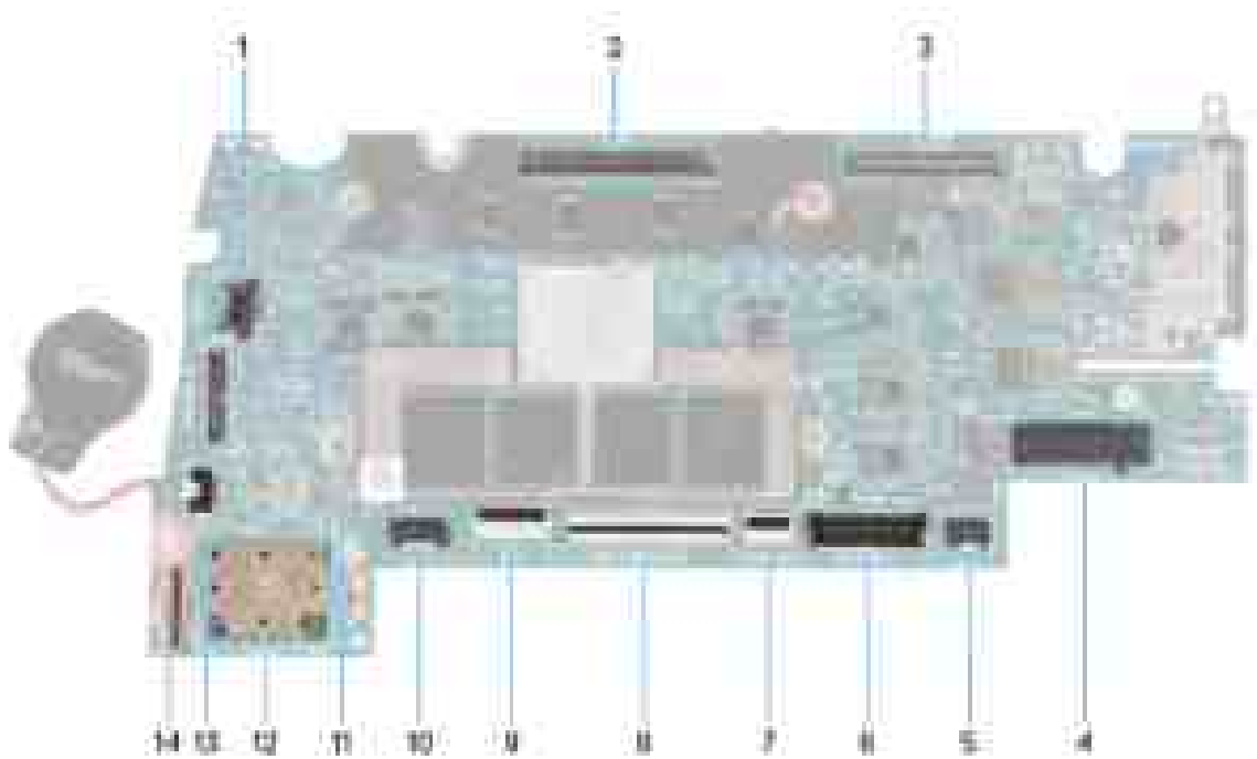
Abbildung 98. Hauptplattenanschlüsse
