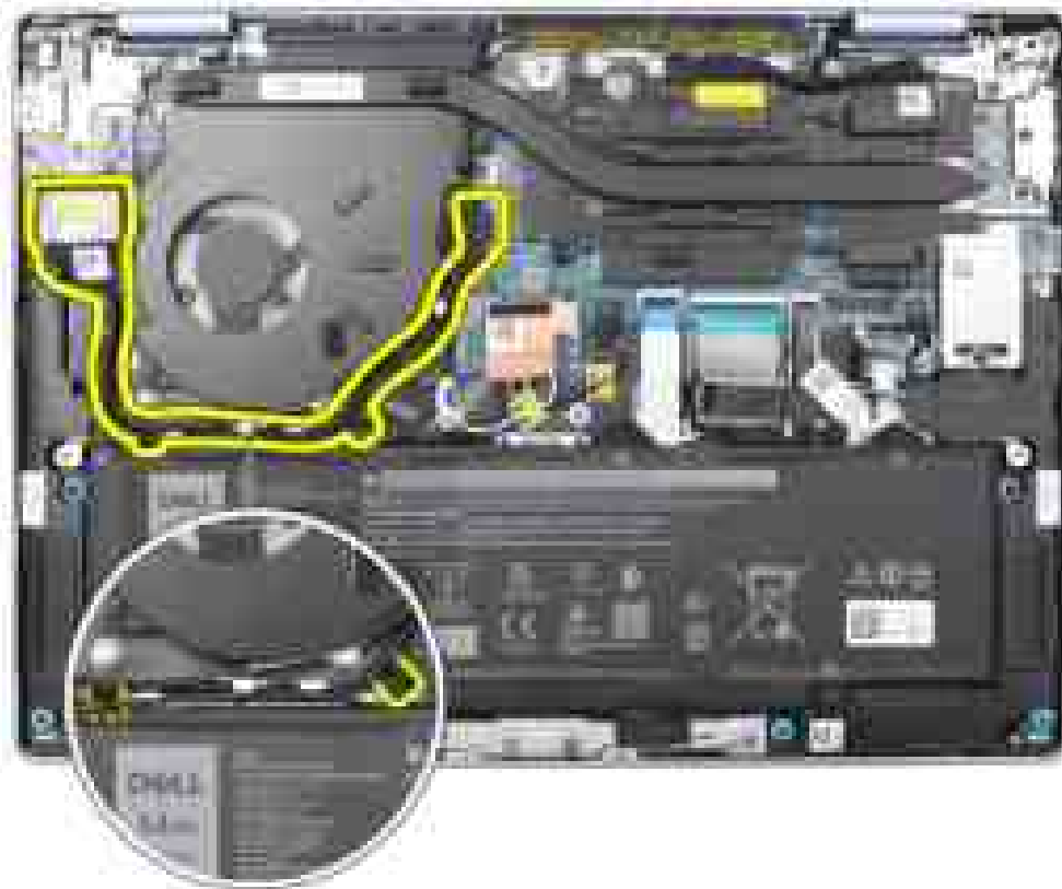
Abbildung 51. Position des I/O-Platinkabels
