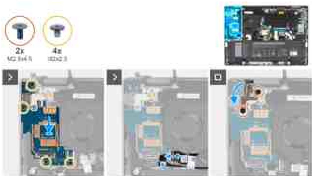
Abbildung 86. Installieren der I/O-Platine Entfernen der I/O-Platine (Computer mit WWAN-Unterstützung)
