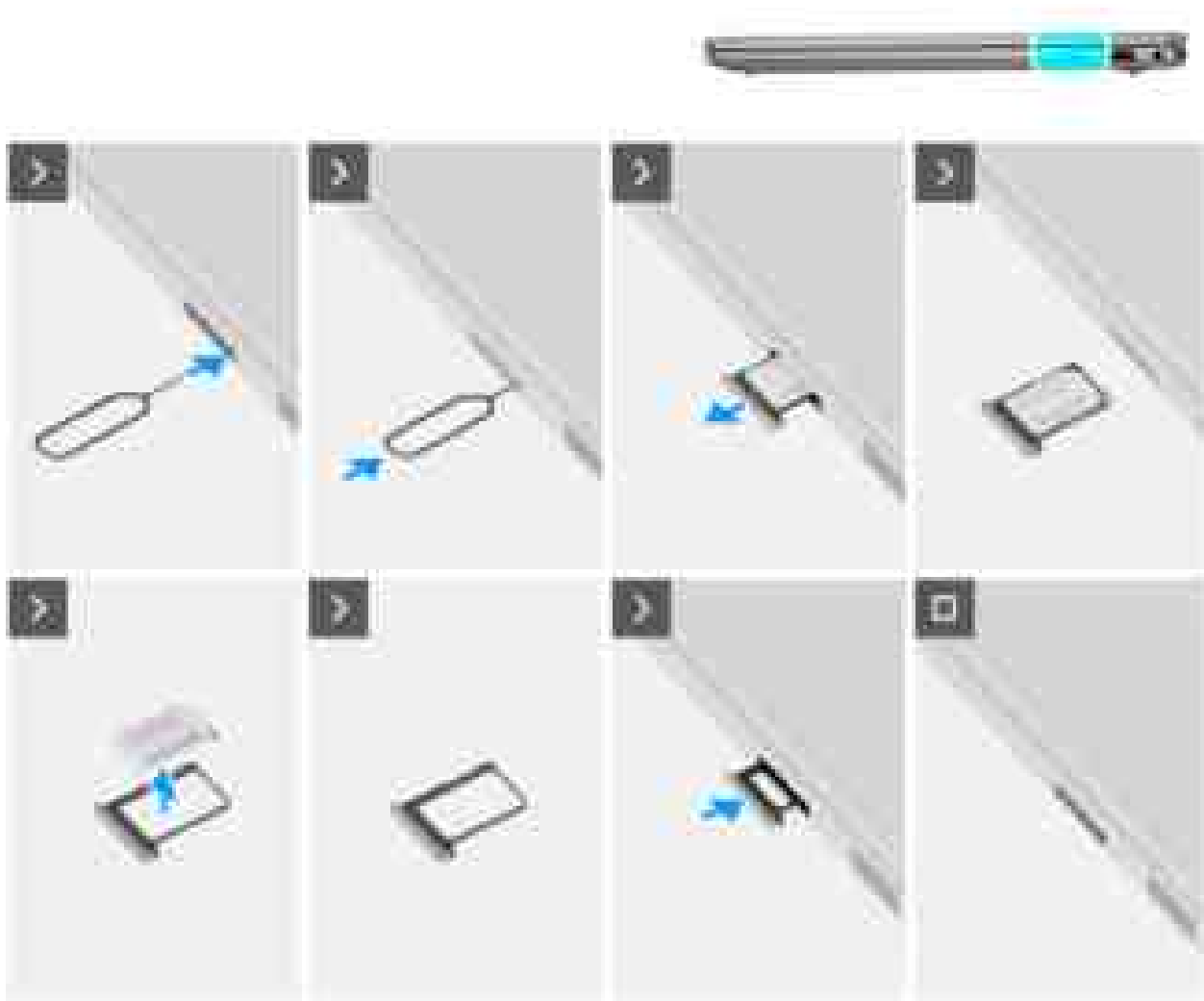
Abbildung 12. Entfernen der SIM-Karte
