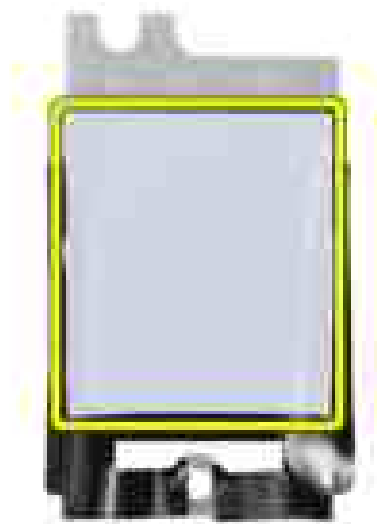
Abbildung 26. Wärmeleitpad unter der SSD-Kühlabdeckung
