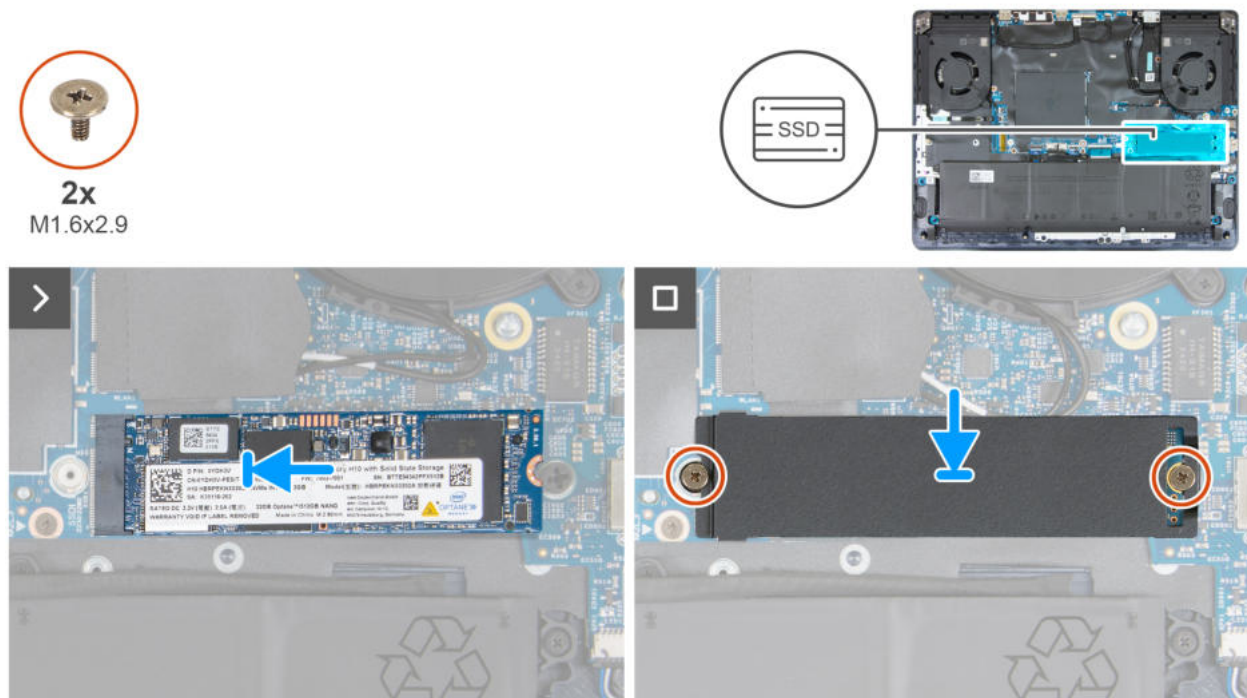
Abbildung 29. Installieren des M.2 2280-SSD-Laufwerks im Steckplatz SSD1
