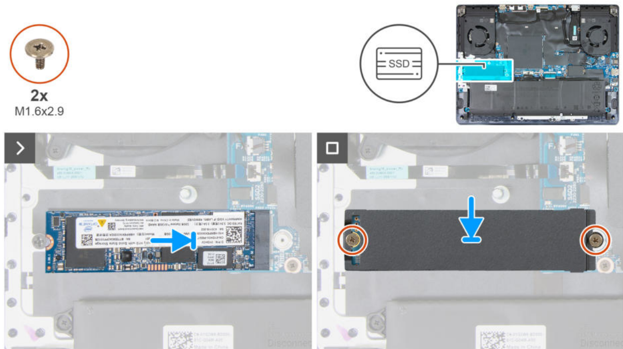
Abbildung 31. Installieren des M.2 2280-SSD-Laufwerks im Steckplatz SSD2
