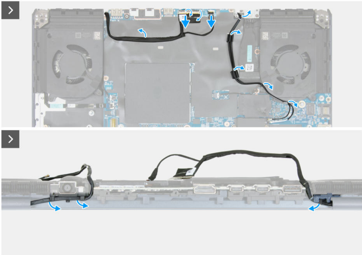
Abbildung 72. Entfernen der Bildschirmbaugruppe
