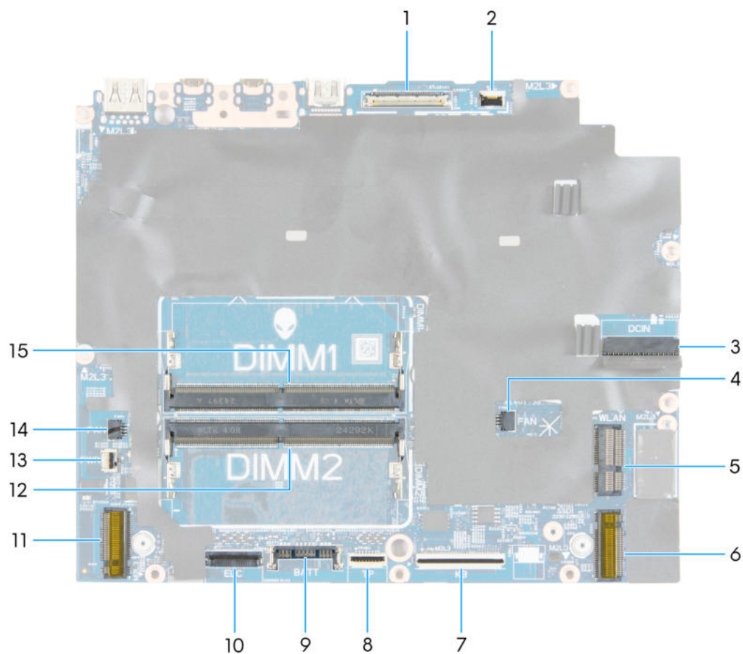
Abbildung 53. Hauptplattenanschlüsse
