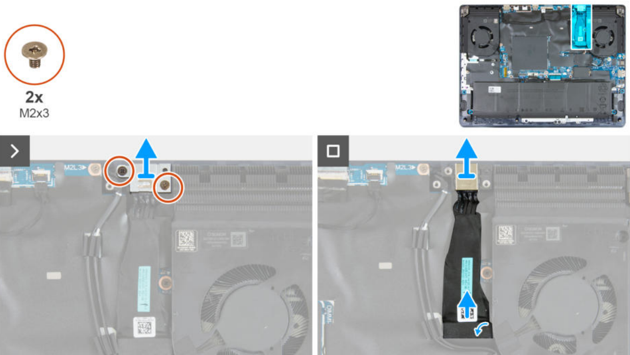
Abbildung 38. Entfernen des Netzadapteranschlusses
