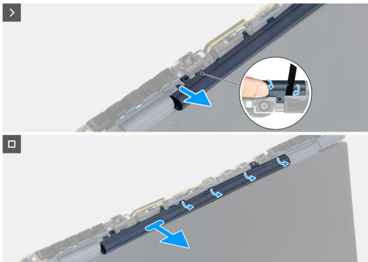
Abbildung 69. Entfernen der Mittelleiste
