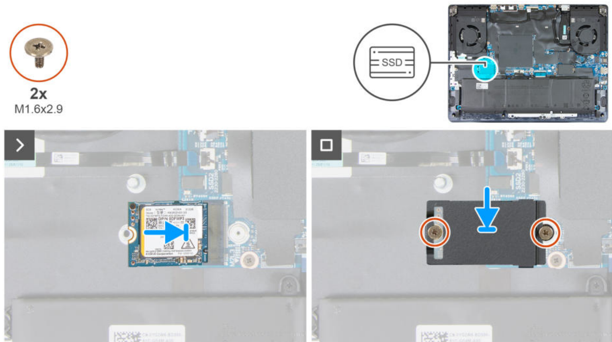
Abbildung 27. Installieren des M.2 2230-SSD im Steckplatz SSD2
