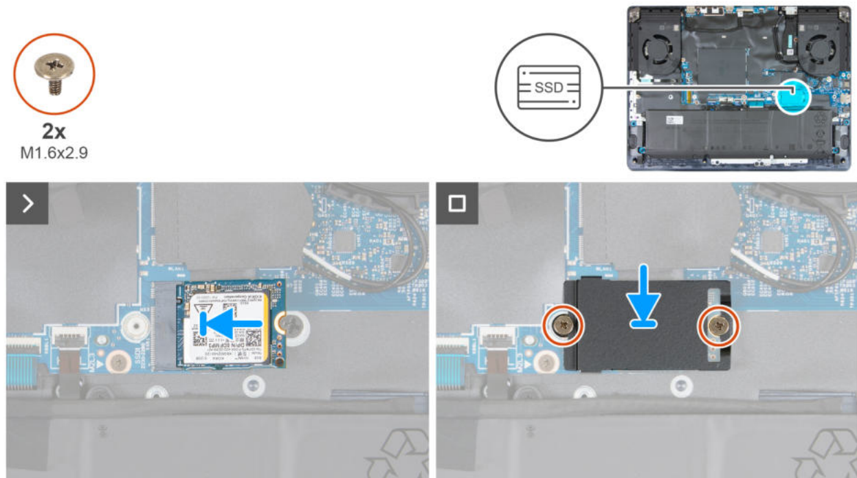
Abbildung 25. Installieren des M.2 2230-SSD im Steckplatz SSD1
