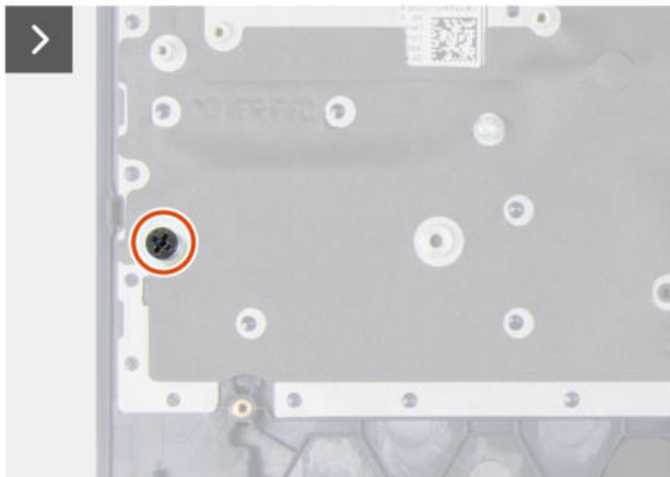
Abbildung 78. SSD-Schraubenhalterungen entfernen
