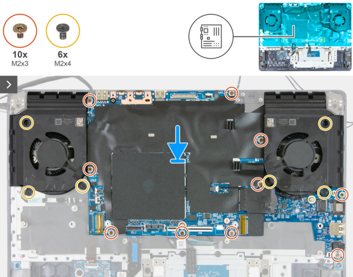
Abbildung 56. Einbauen der Systemplatine
