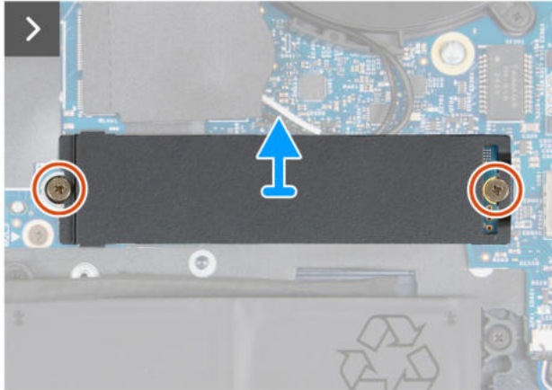
Abbildung 28. Entfernen des M.2 2280-SSD-Laufwerks aus dem Steckplatz SSD1
