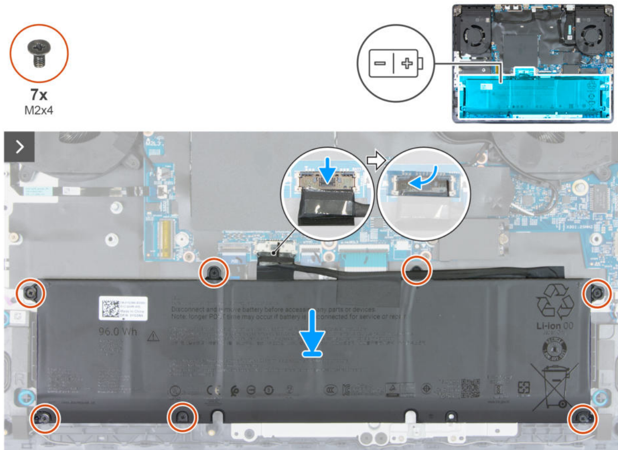
Abbildung 19. Einsetzen des Akkus
