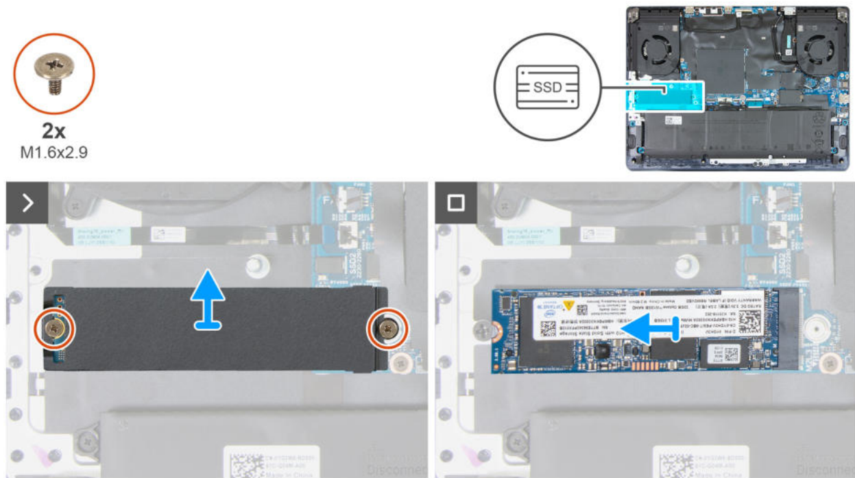
Abbildung 30. Entfernen des M.2 2280-SSD-Laufwerks aus dem Steckplatz SSD2
