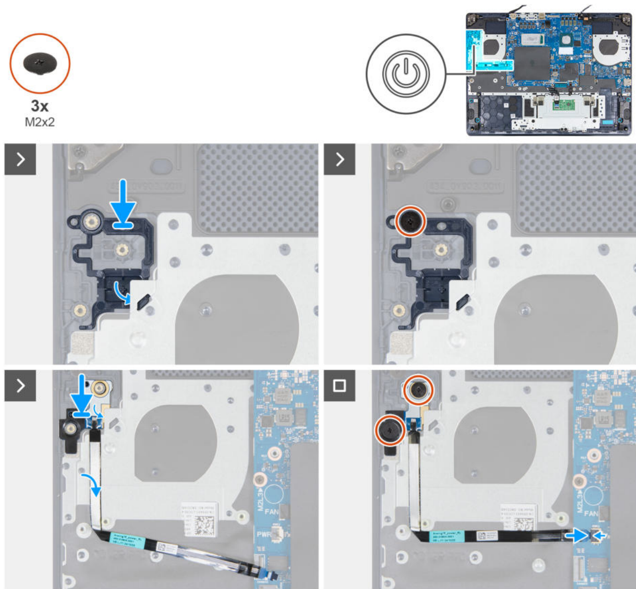
Abbildung 60. Einbauen des Netzschalters und der Netzschalterplatine
