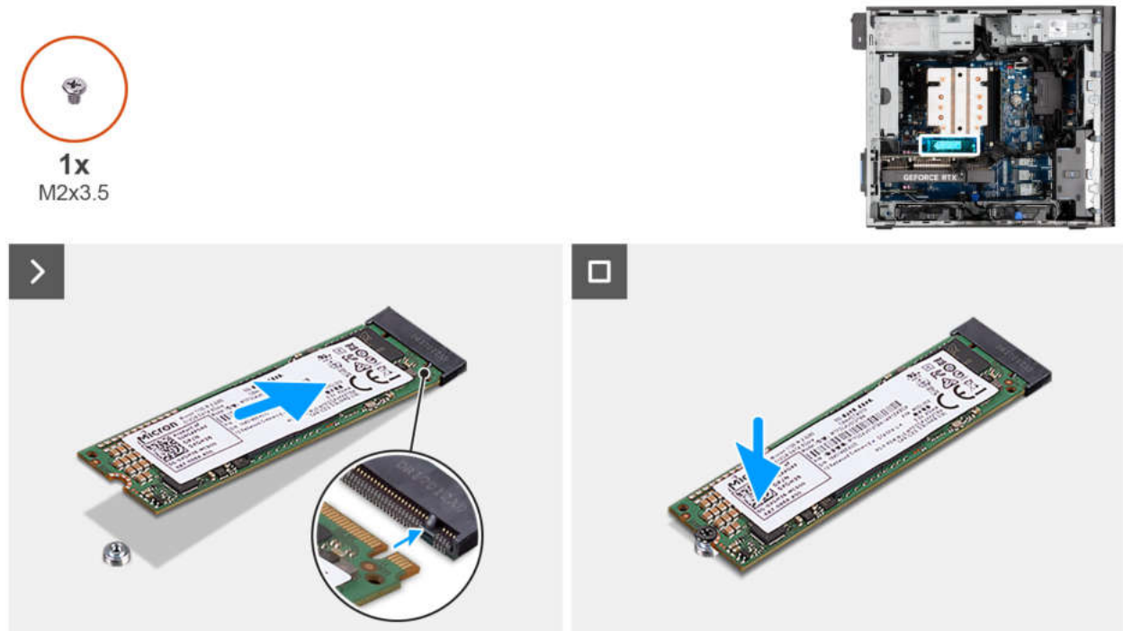
Abbildung 34. Einbauen des M.2 2280-PCIe-SSD-Laufwerks
