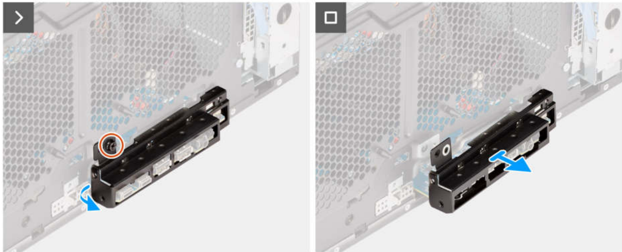
Abbildung 19. Entfernen der vorderen E/A-Halterung
