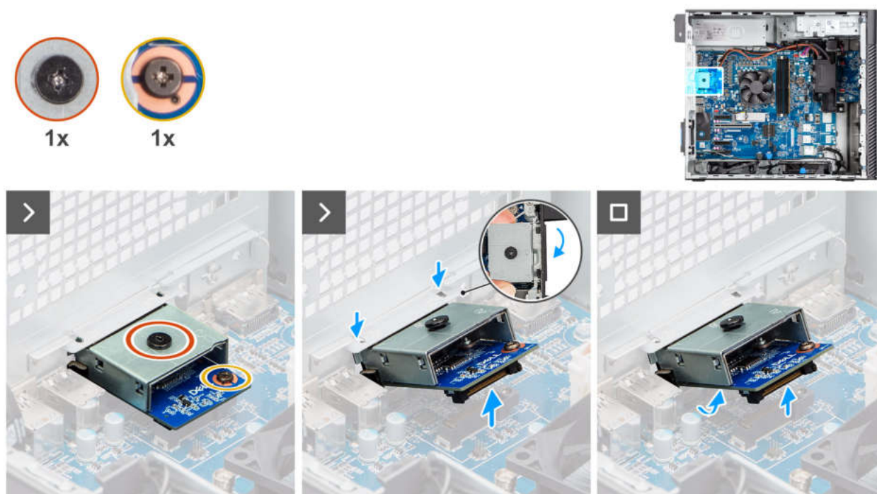
Abbildung 70. Entfernen des optionalen HDMI-Moduls
