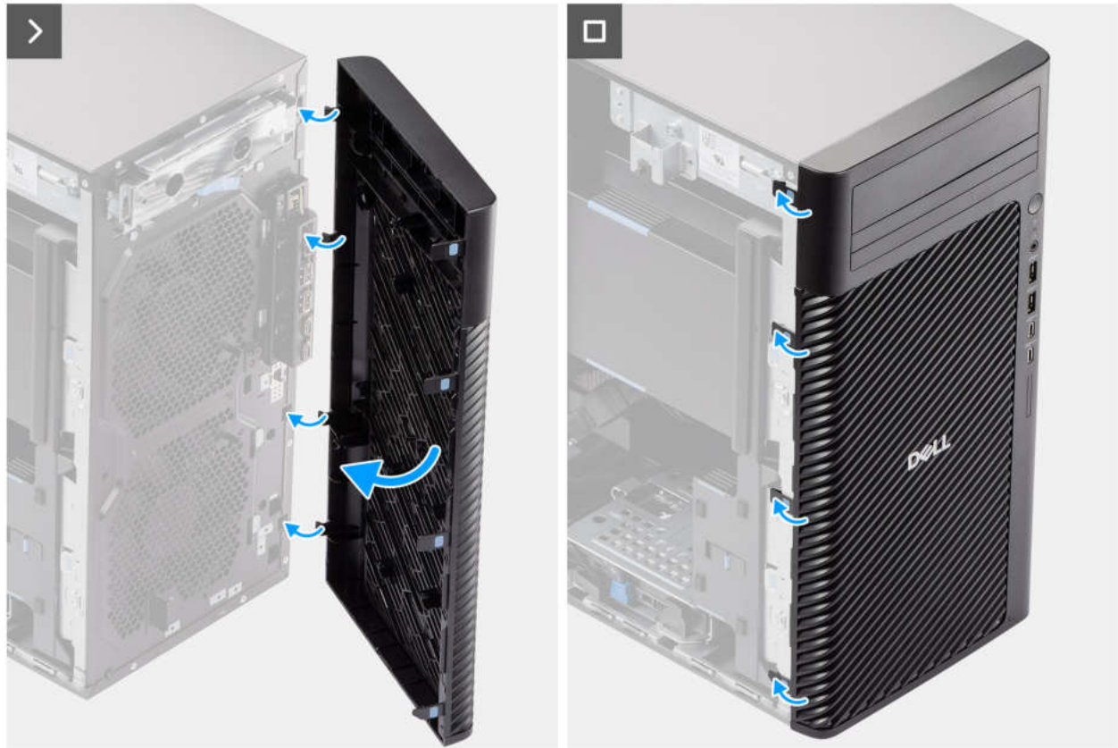
Abbildung 18. Installieren der Frontverkleidung
