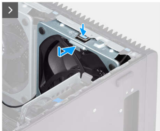
Abbildung 48. Vorderer Lüfter 2
