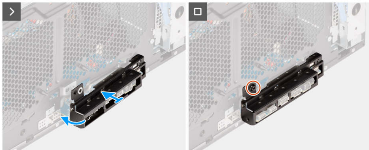
Abbildung 20. Anbringen der vorderen E/A-Halterung
