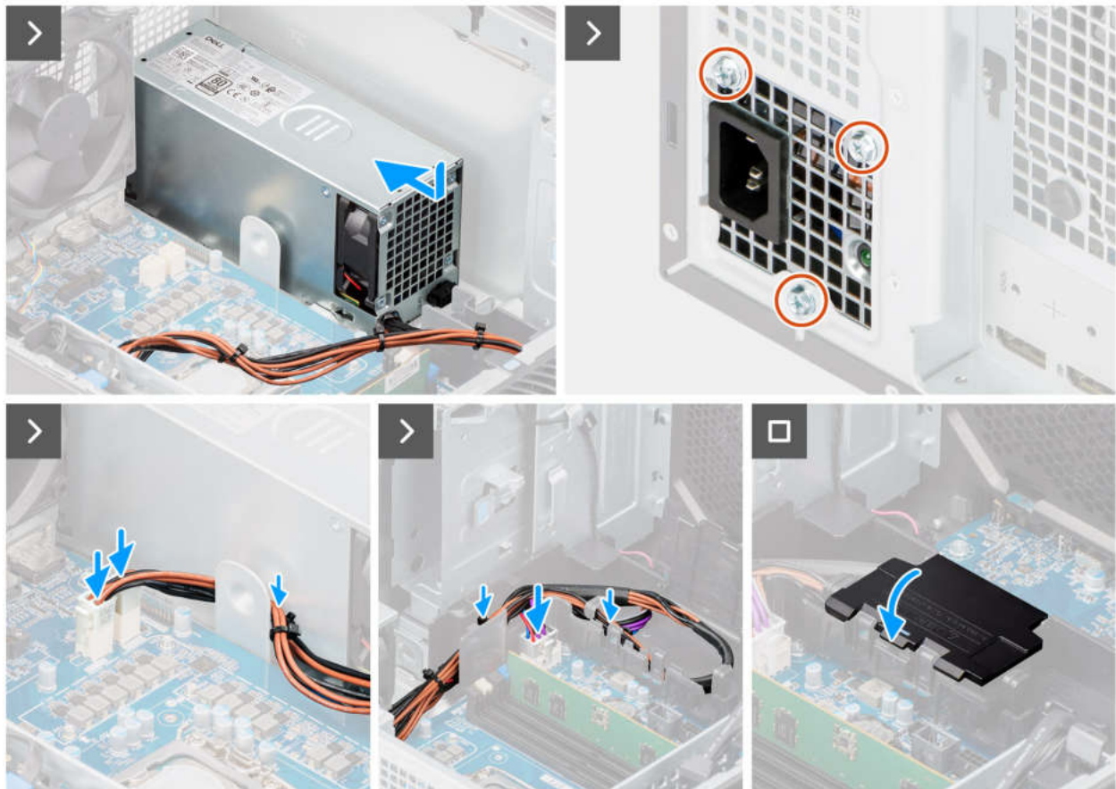
Abbildung 58. Installieren der 360-W-Stromversorgungseinheit
