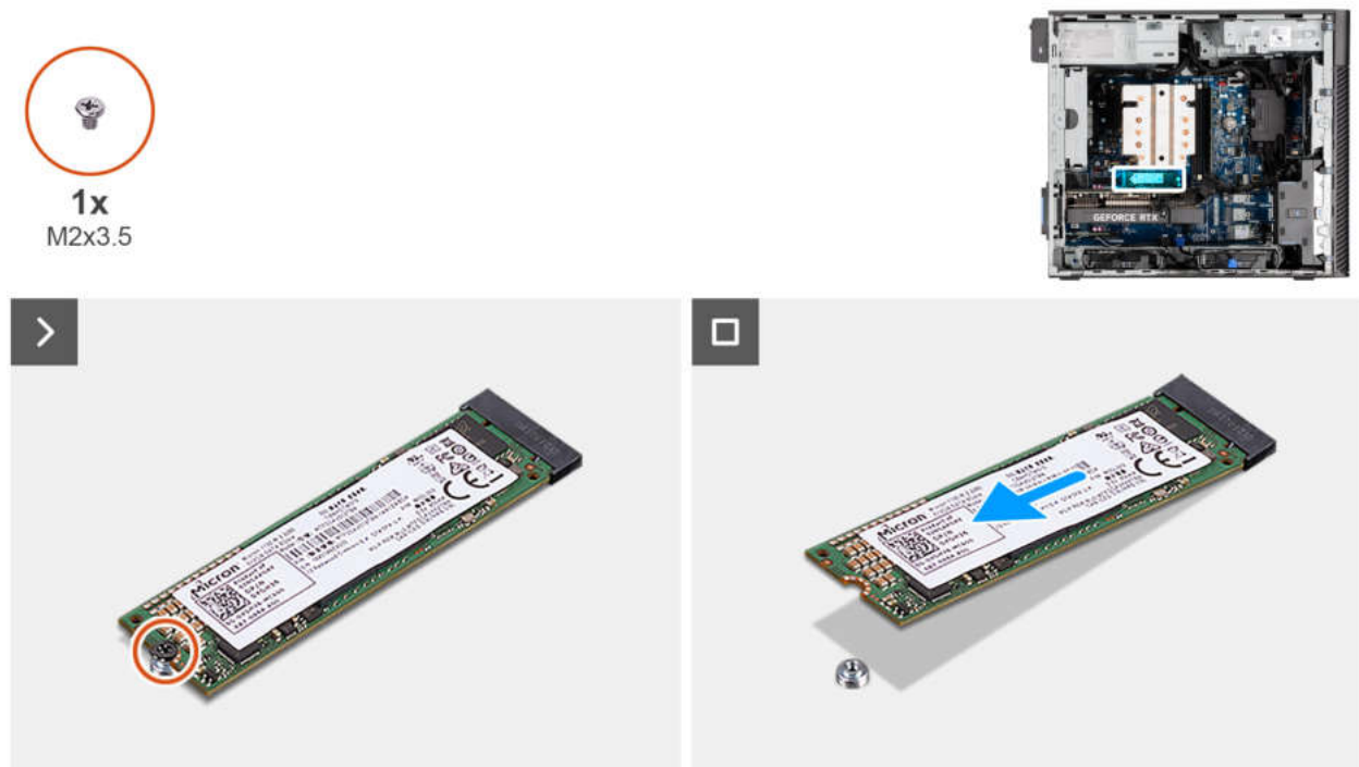
Abbildung 33. Entfernen des M.2 2280-PCIe-SSD-Laufwerks
