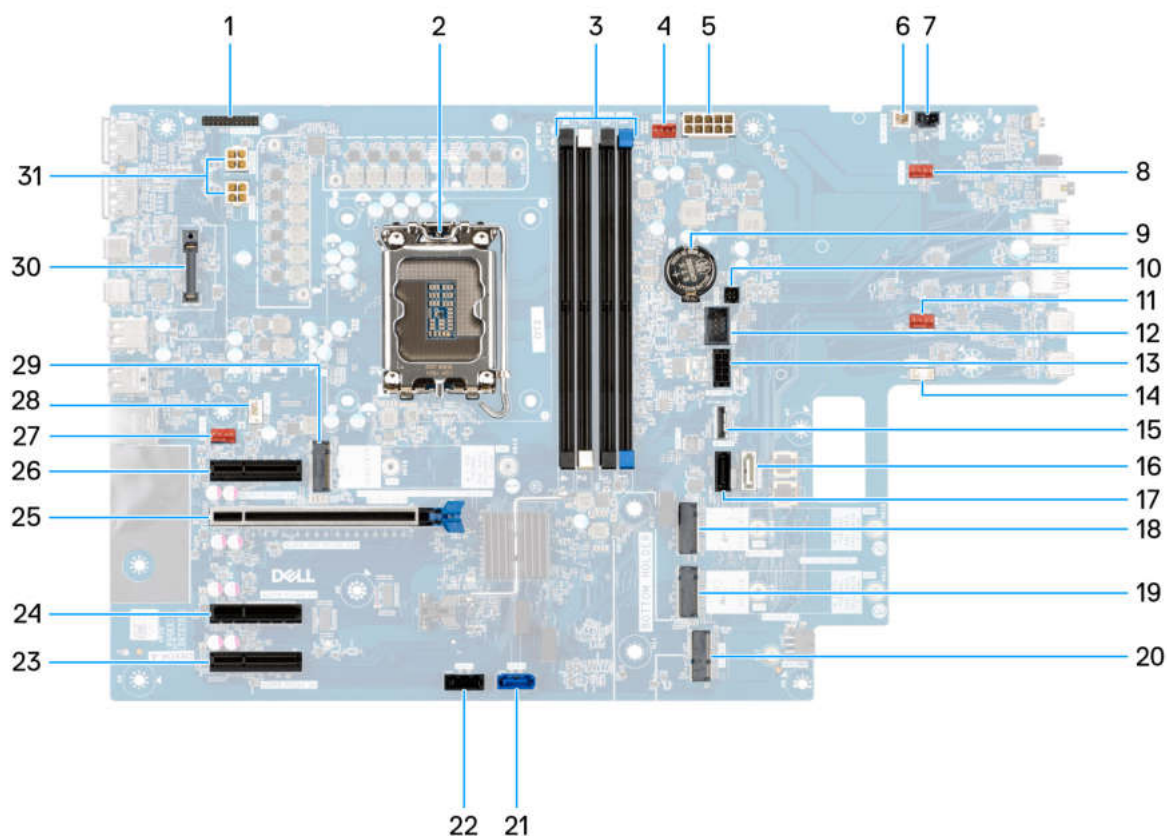
Abbildung 93. Systemplatinenbeschriftung
