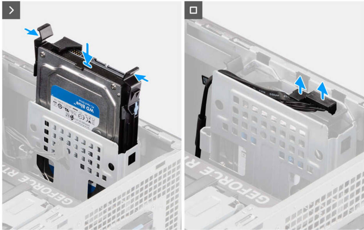
Abbildung 29. Installieren der 3,5-Zoll-Festplattenbaugruppe (Schacht 2)
