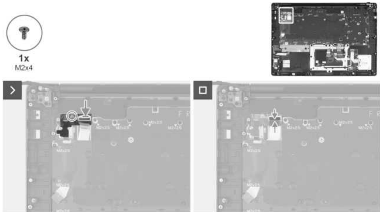
Abbildung 126. Einbauen der Netzschalterplatine
