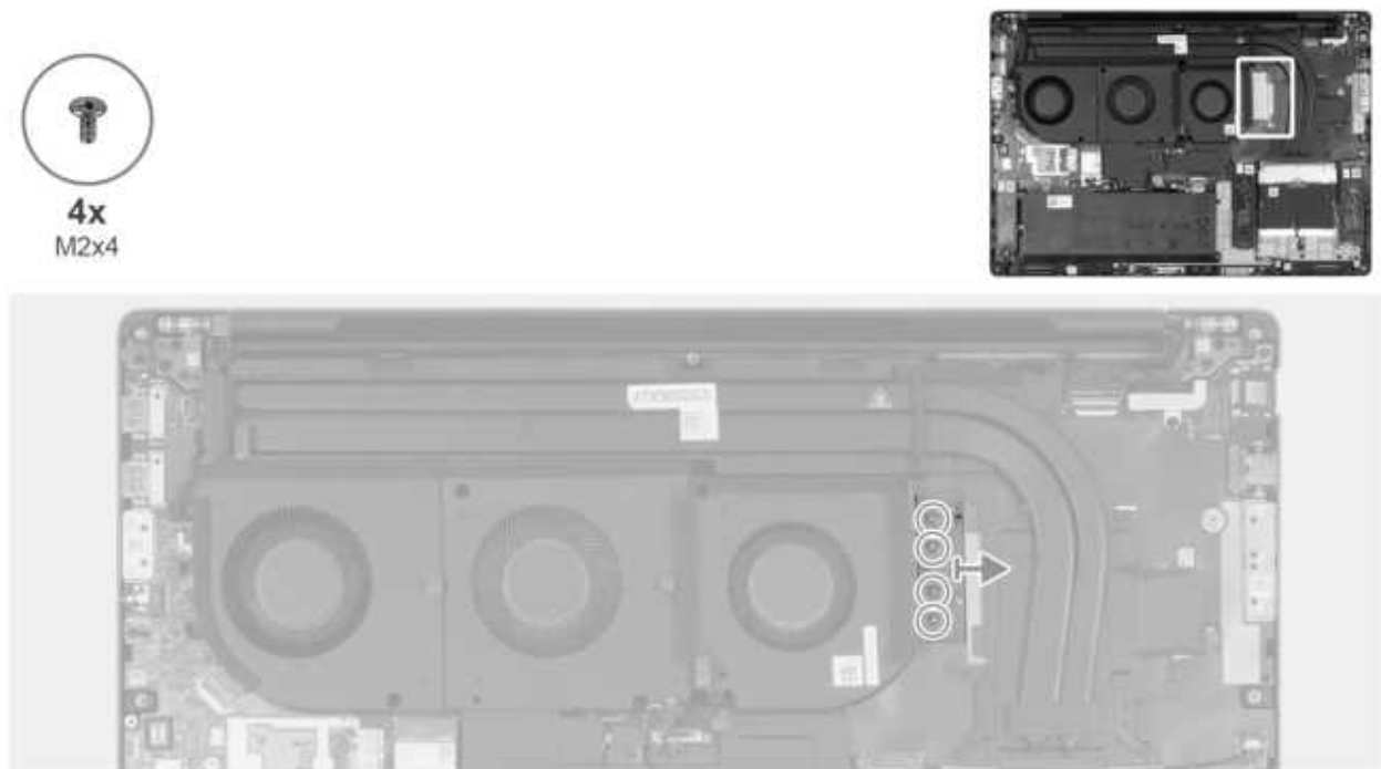
Abbildung 57. Entfernen des integrierten FPC-Trägerverbinders
