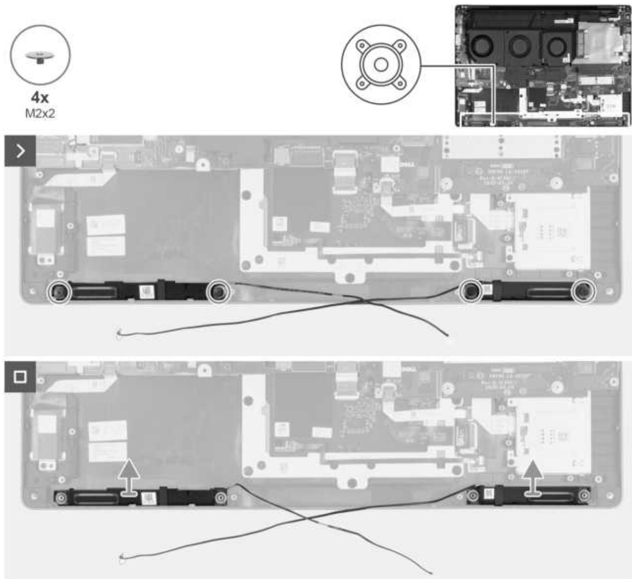
Abbildung 81. Entfernen der Lautsprecher
