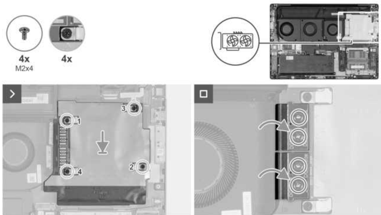
Abbildung 56. Einbauen der GPU-Karte
