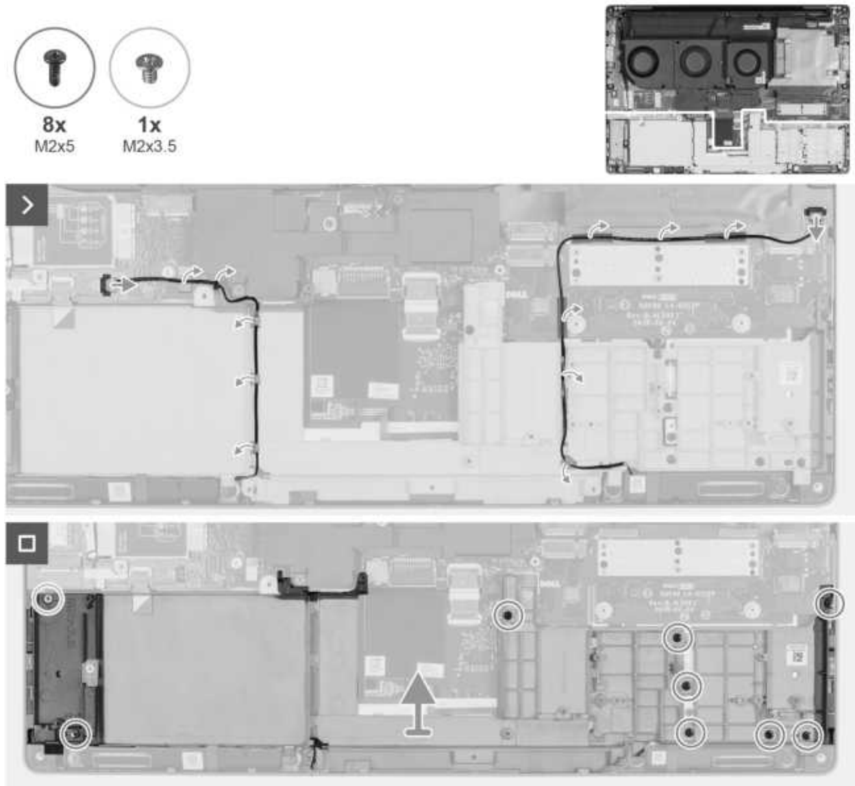
Abbildung 79. Entfernen des inneren Rahmens
