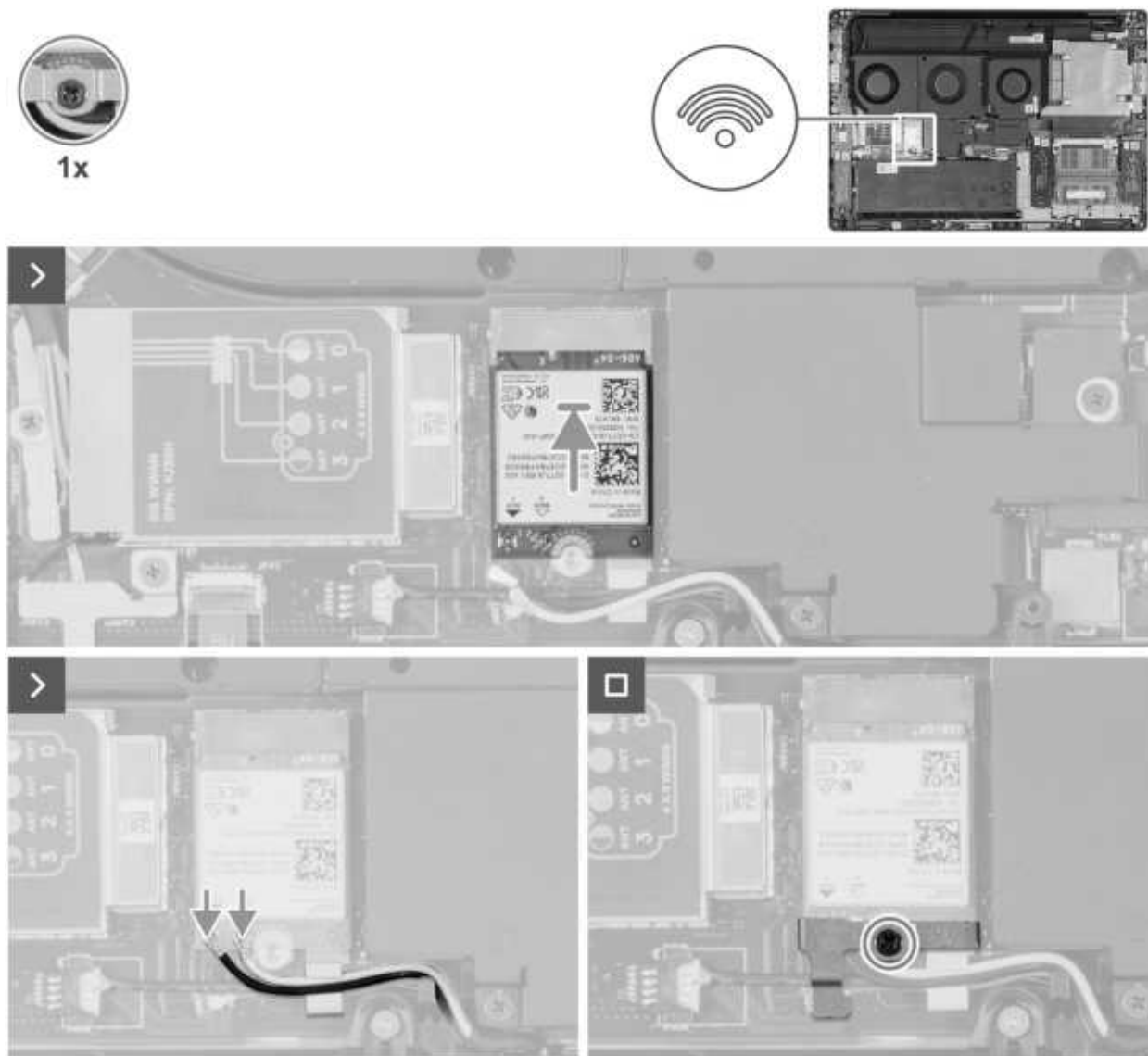
Abbildung 49. Einbauen der WLAN-Karte
