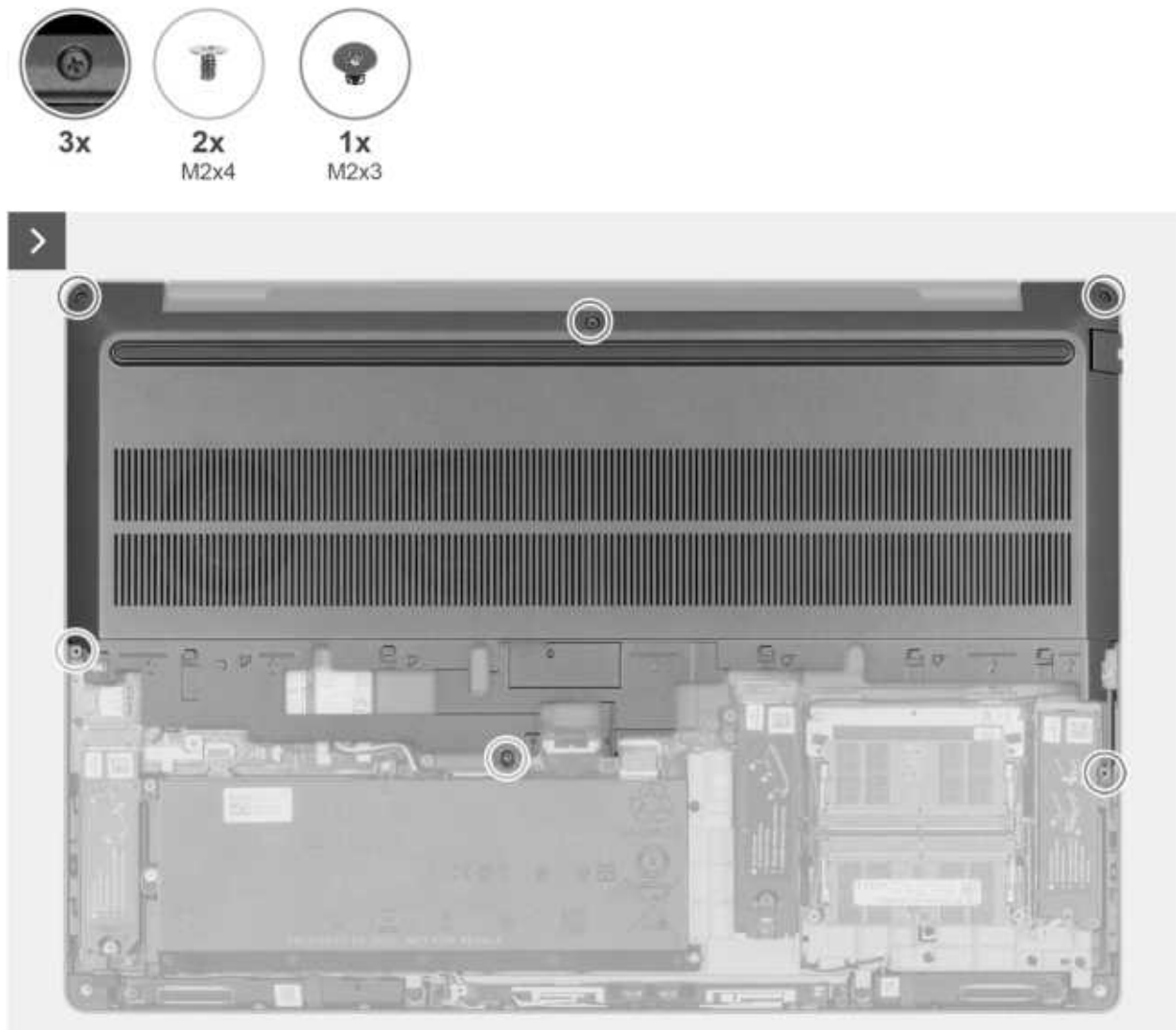
Abbildung 18. Lösen der drei unverlierbaren Schrauben und Entfernen der drei Schrauben
