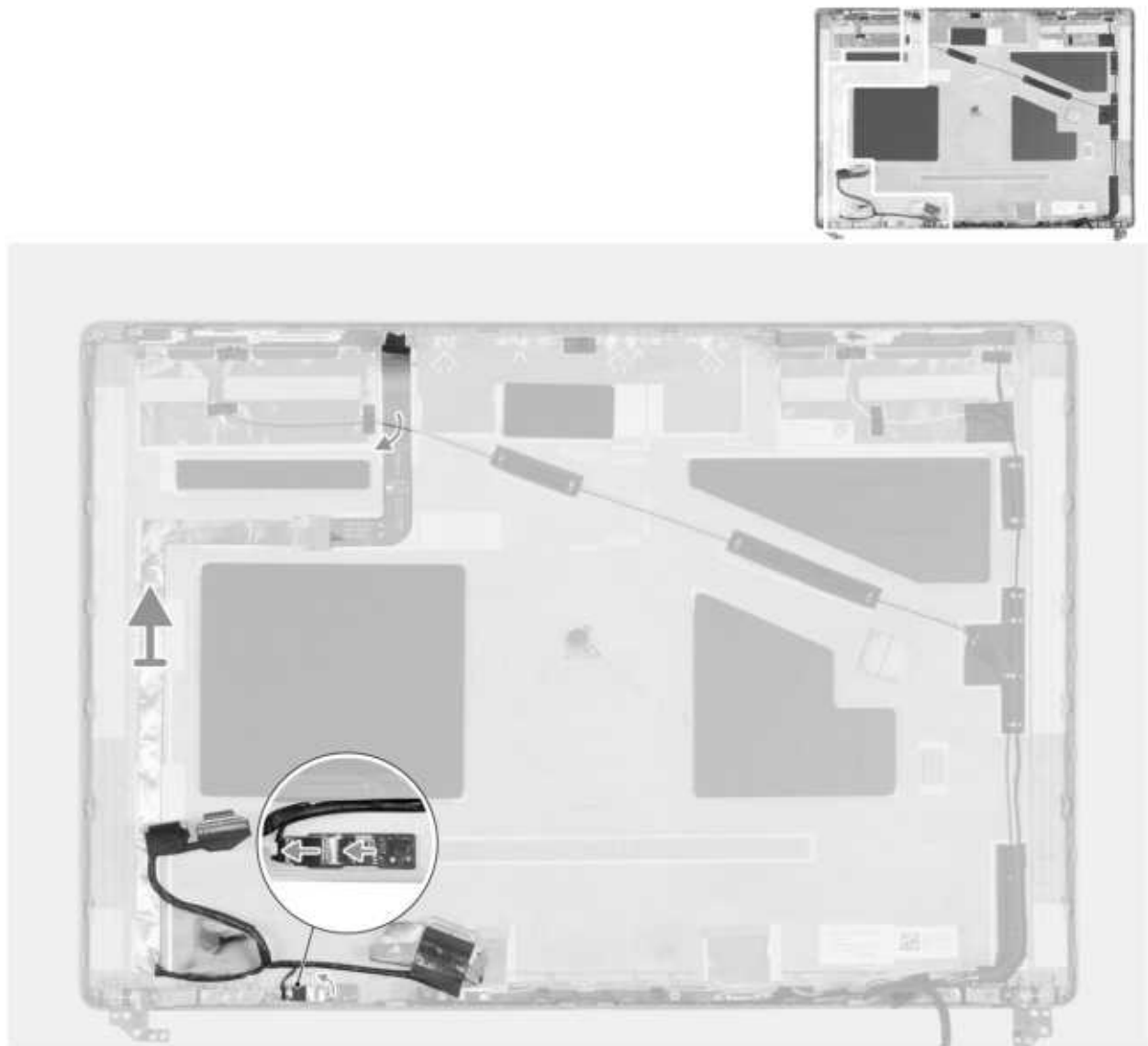
Abbildung 102. Entfernen des Bildschirmkabels
