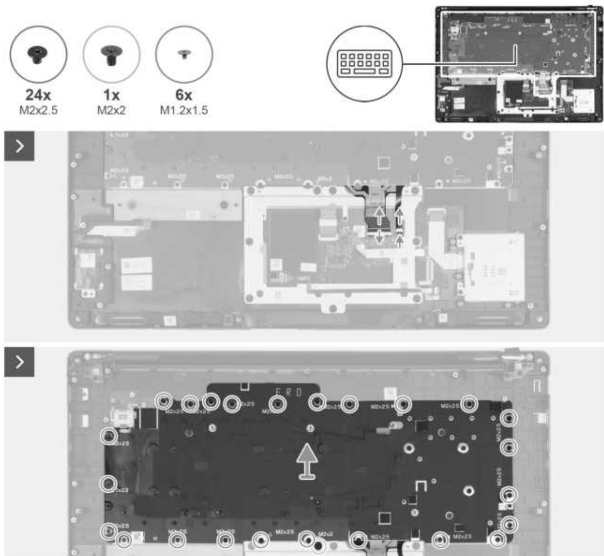
Abbildung 117. Entfernen der Tastatur
