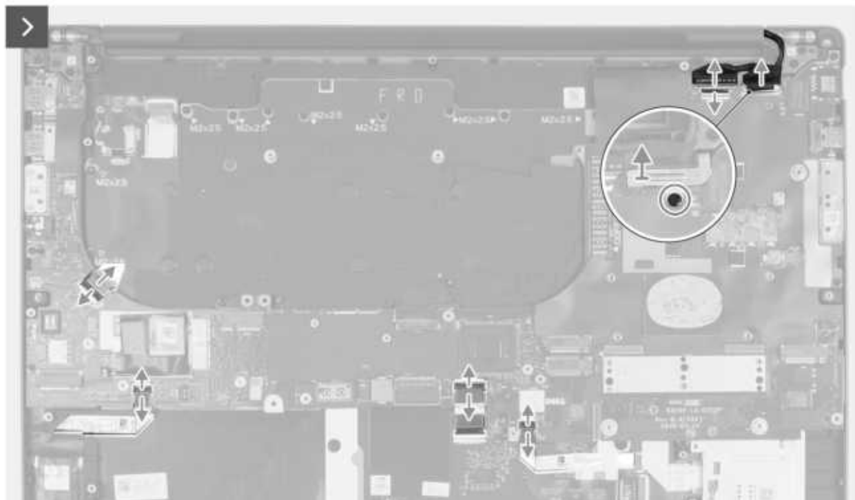
Abbildung 107. Entfernen der Systemplatine
