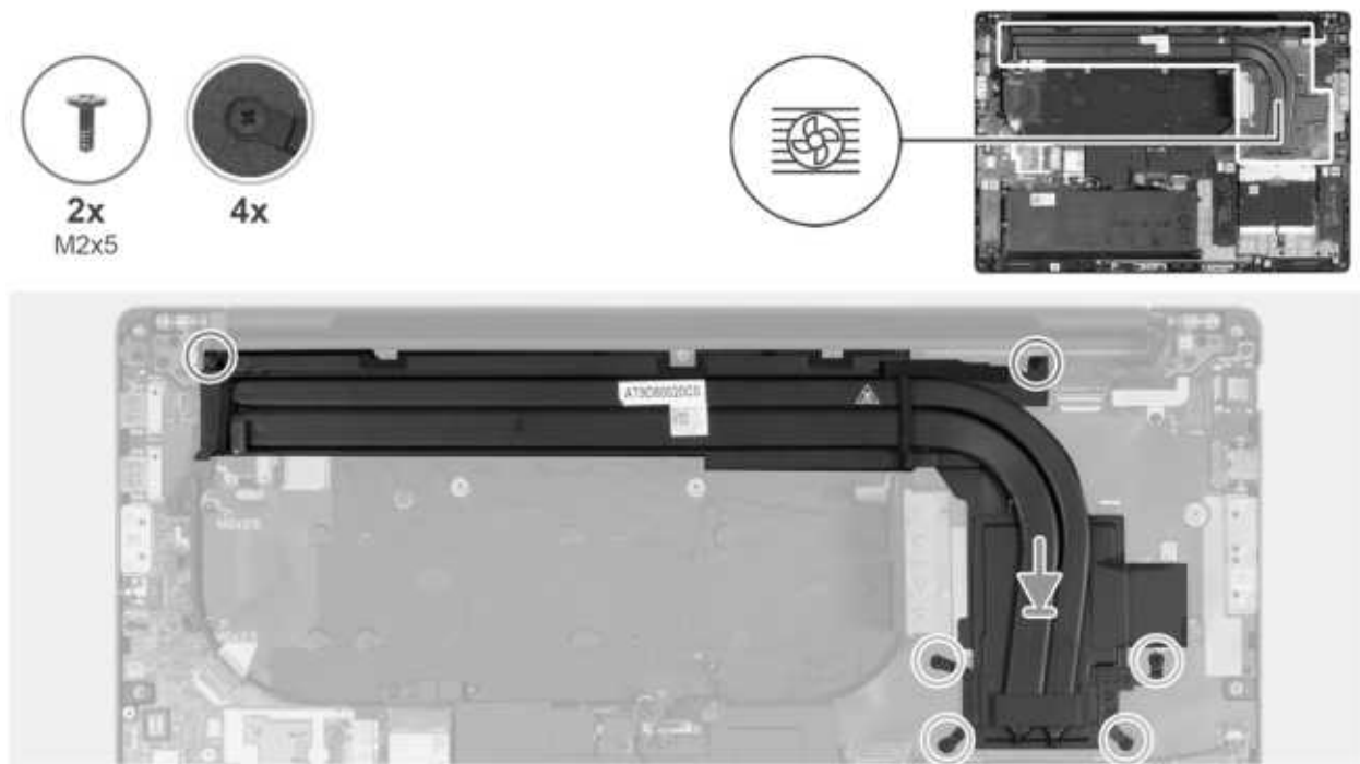
Abbildung 74. Installieren des Kühlkörpers bei Computern mit integrierter Grafikkarte
