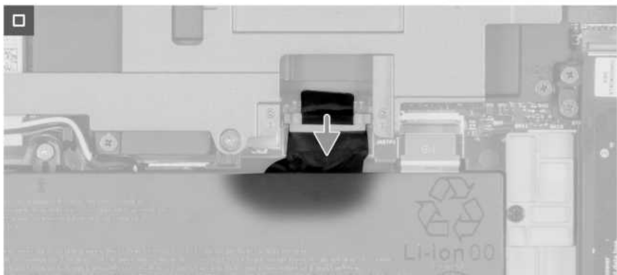
Abbildung 20. Trennen des Akkukabels
