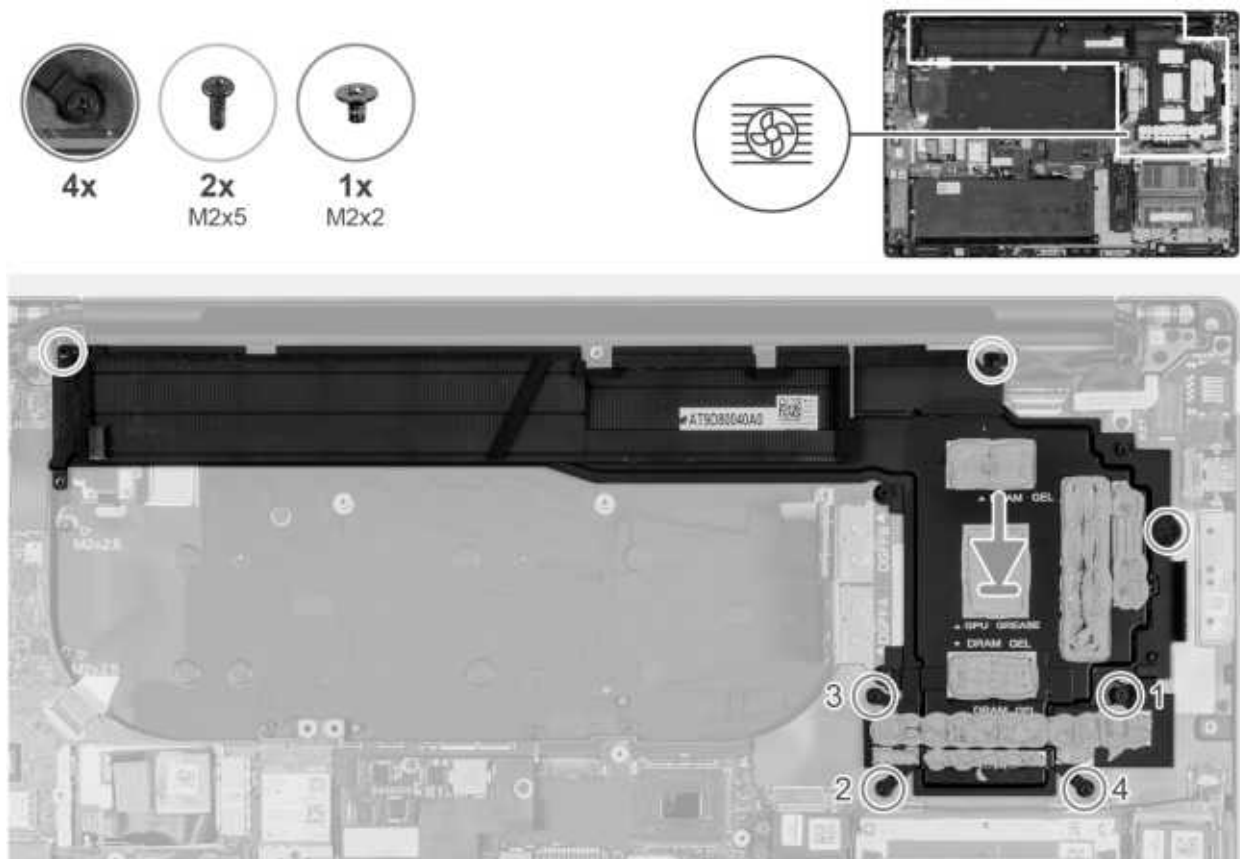
Abbildung 76. Installieren des Kühlkörpers bei Computern mit separater Grafikkarte
