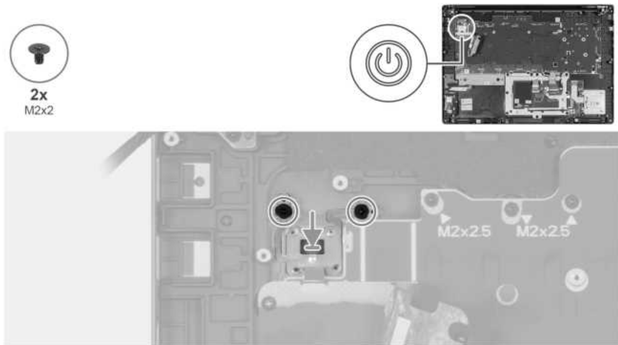
Abbildung 128. Installieren des Netzschalters
