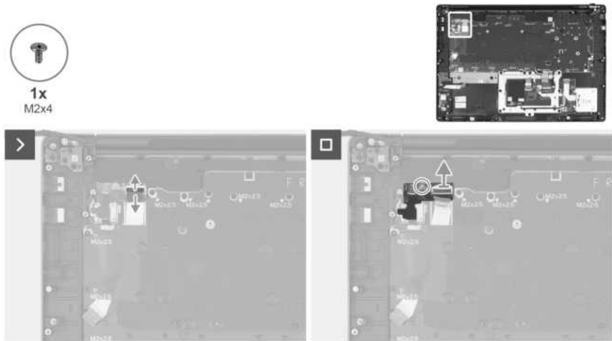
Abbildung 125. Entfernen der Netzschalterplatine
