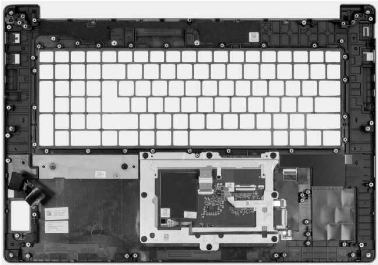
Abbildung 130. Handauflagenbaugruppe
