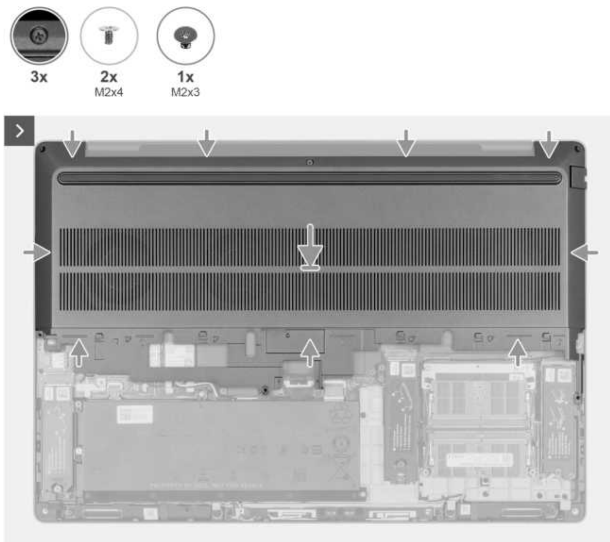
Abbildung 22. Ausrichten der Schraubenbohrungen der Bodenabdeckung an den Schraubenbohrungen der Handballenstützen- und Tastaturbaugruppe
