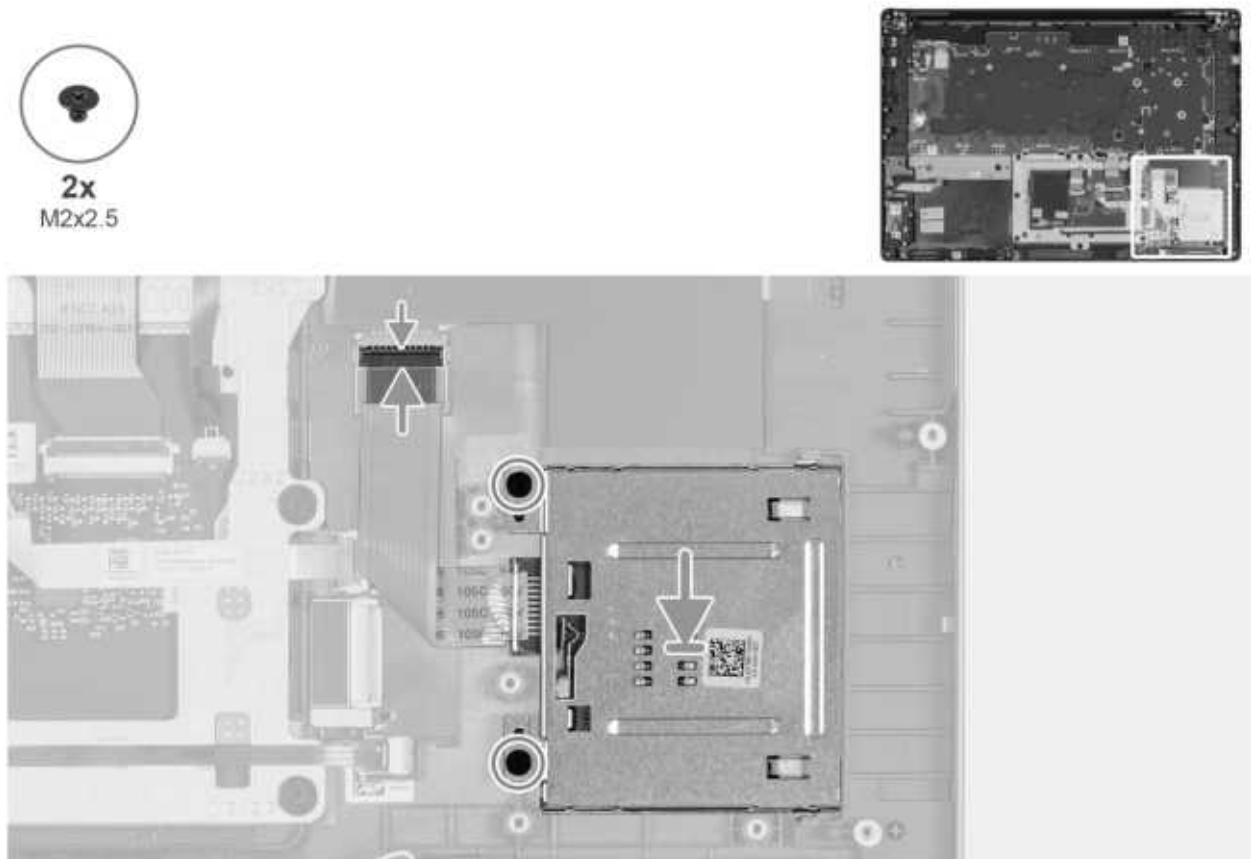
Abbildung 122. Installieren des Smartcardlesegeräts
