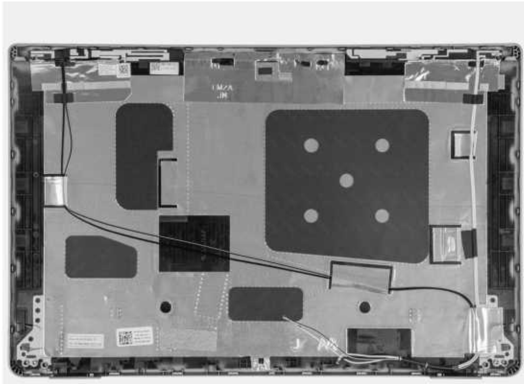
Abbildung 105. Hintere Bildschirmrückabdeckung
