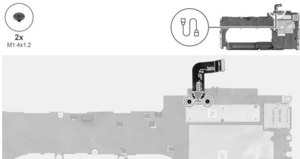
Abbildung 116. Einbauen des USH-Platinenkabels
