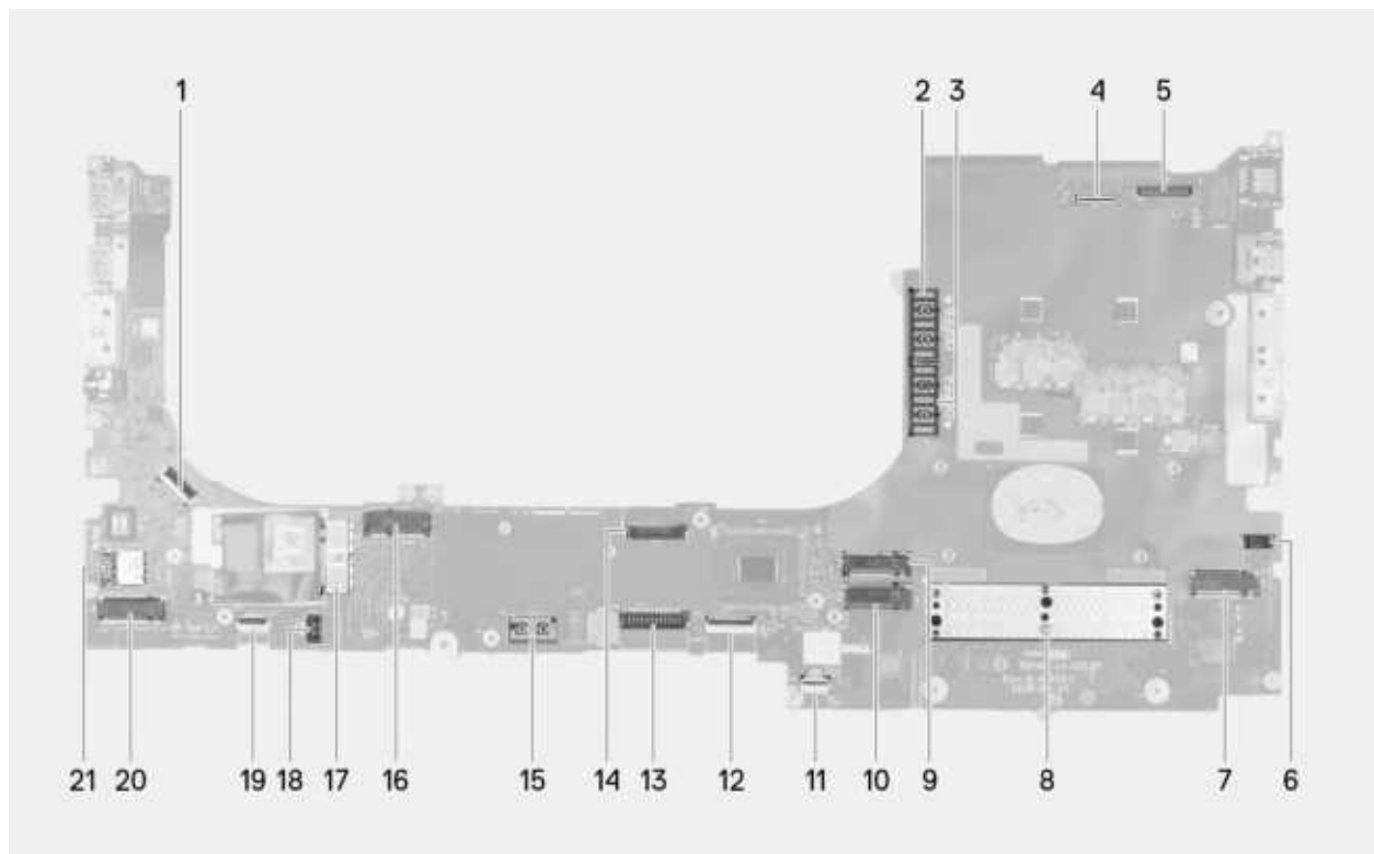
Abbildung 106. Hauptplatinenanschlüsse
