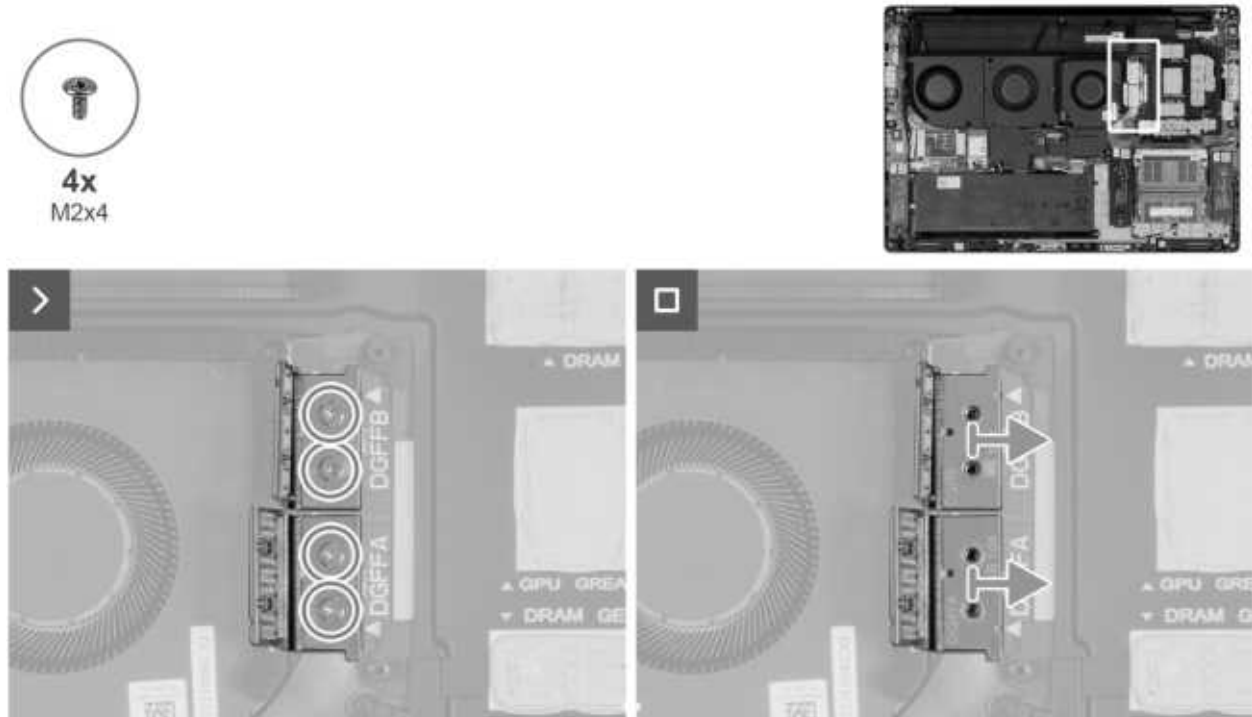
Abbildung 59. Entfernen des separaten FPC-Trägerverbinders
