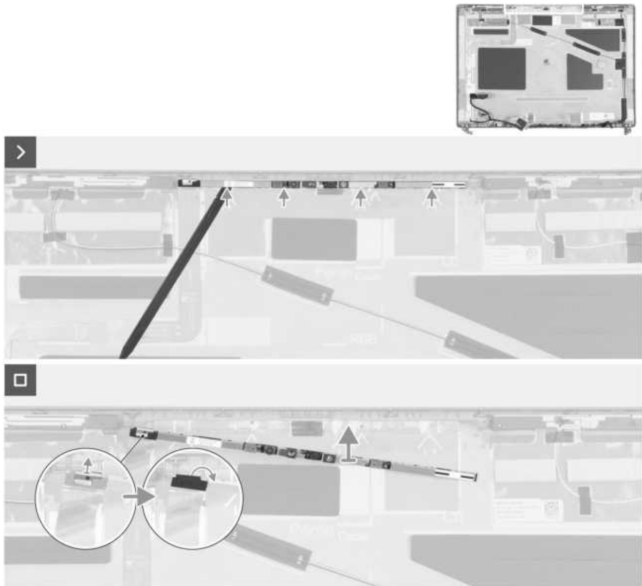
Abbildung 101. Entfernen des Kameramoduls
