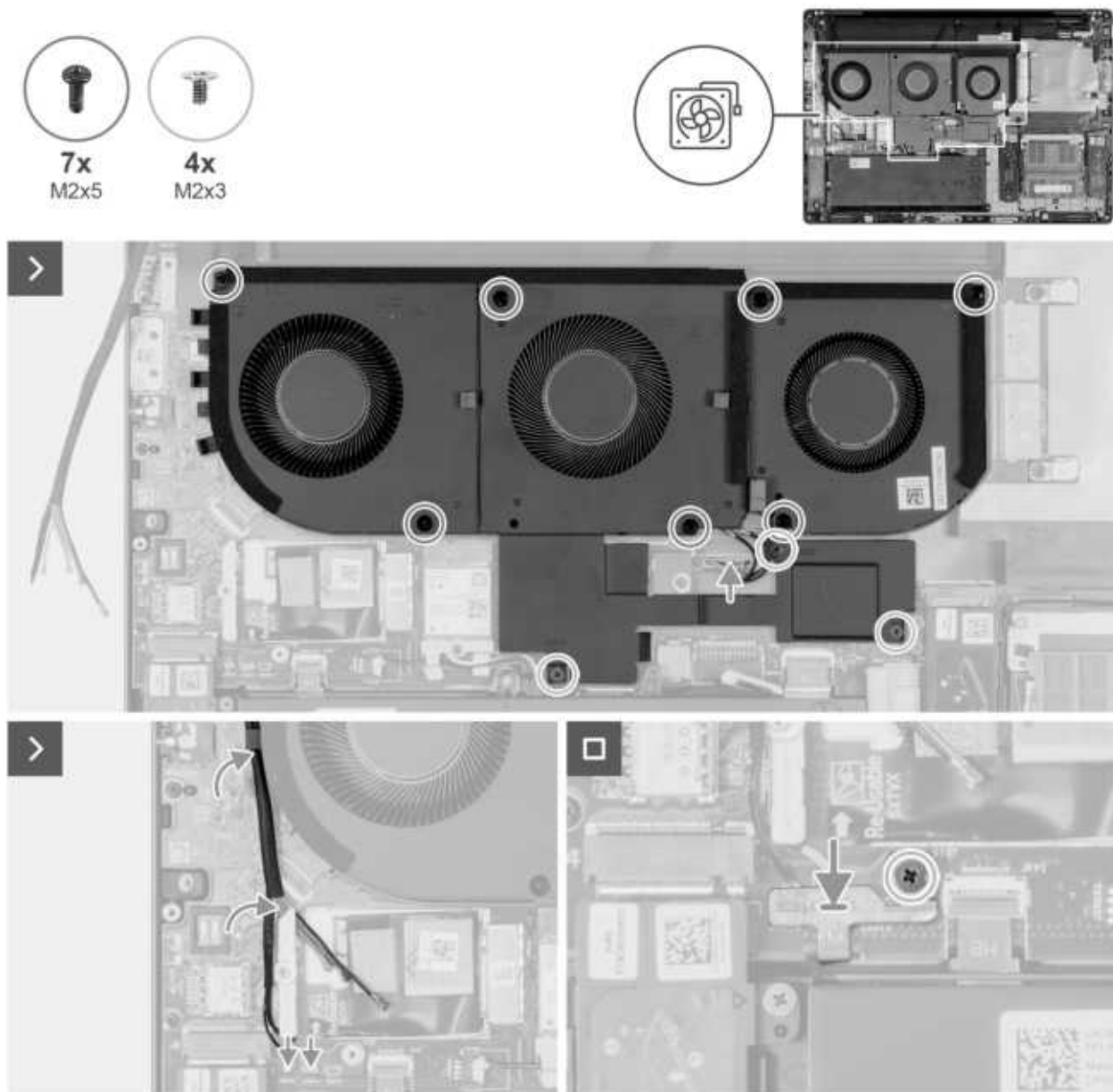
Abbildung 62. Installieren der Lüfterbaugruppe
