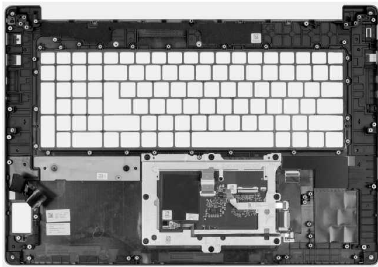
Abbildung 129. Handauflagenbaugruppe
