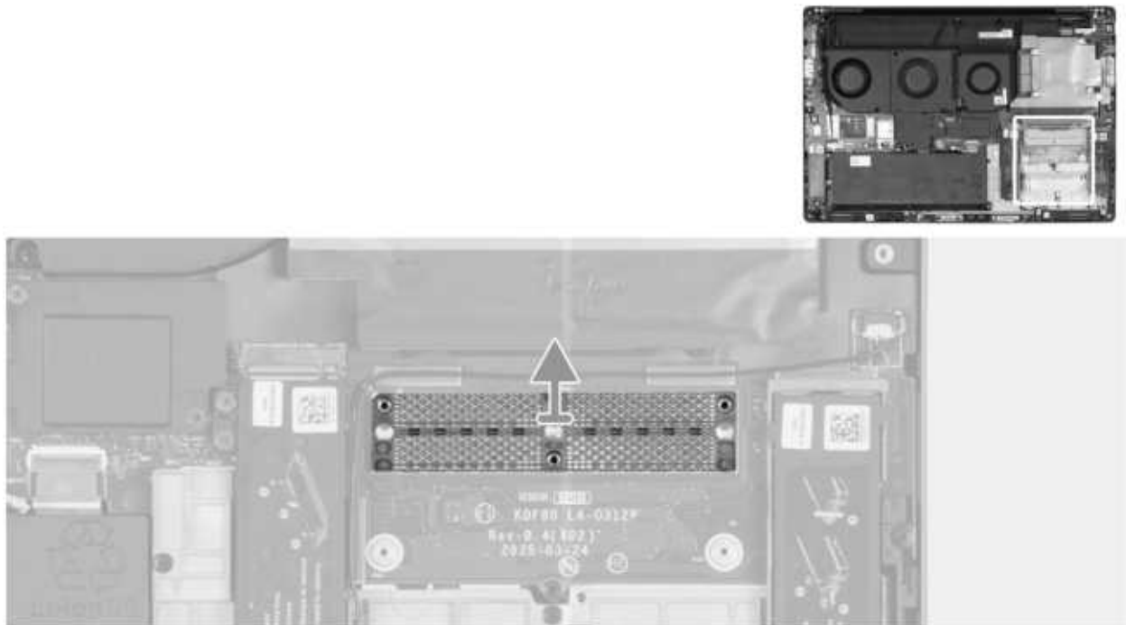
Abbildung 69. Entfernen des Speicheranschlusses
