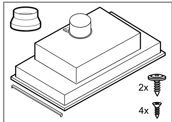
Gerätebreite 730 mm
