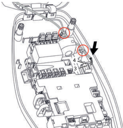
Abb. 19: Anschluss Downgrade-Eingang
