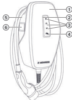
Abb. 3: Außenansicht (Beispiel)
