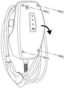
Abb. 8: Produkt öffnen
