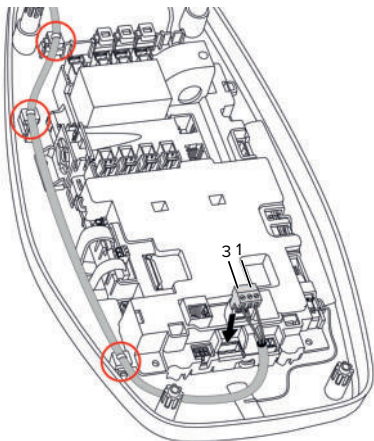
Abb. 12: Anschluss Arbeitsstromauslöser
