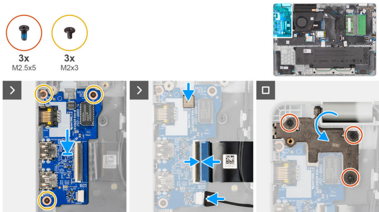
Abbildung 41. Installing the I/O board
