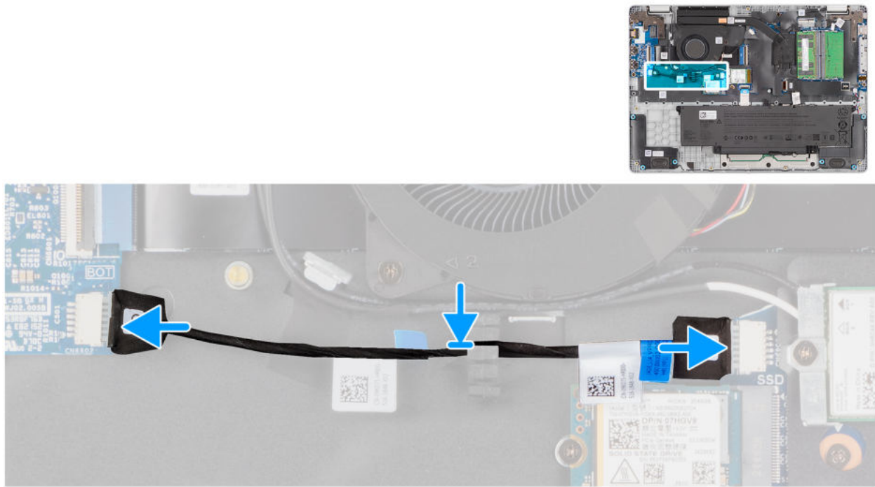
Abbildung 37. Installing the vPro cable
