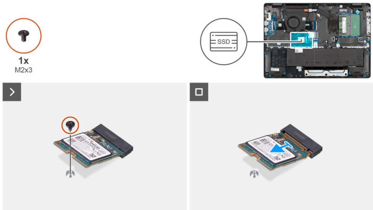
Abbildung 23. Removing the SSD
