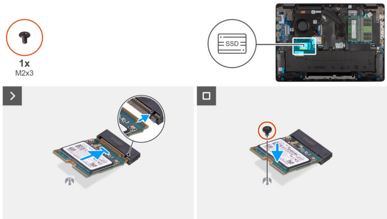
Abbildung 24. Installing the SSD
