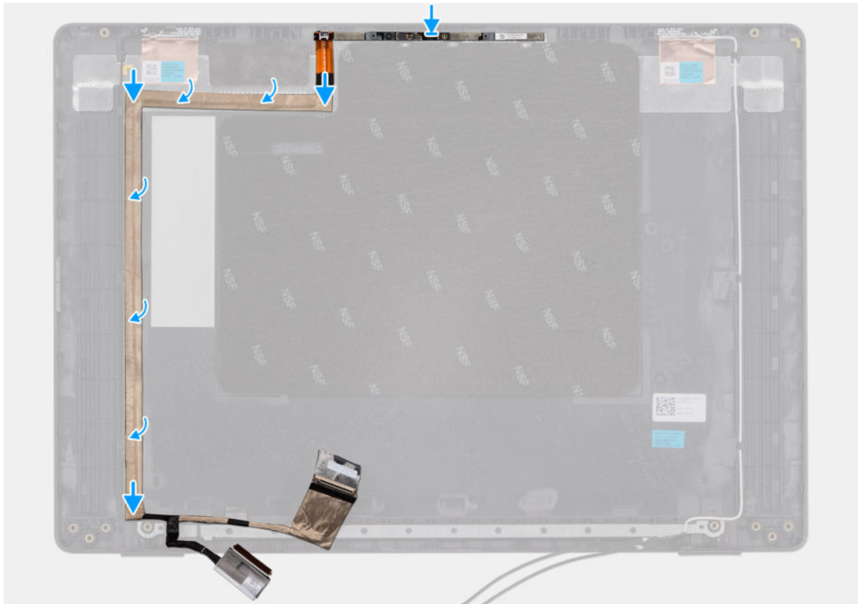
Abbildung 95. Installing the eDP cable
