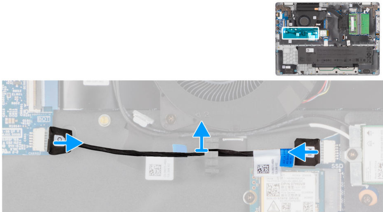
Abbildung 36. Removing the vPro cable
