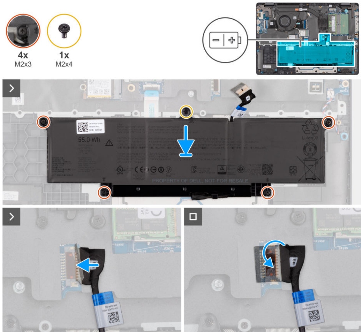
Abbildung 18. Installing the battery
