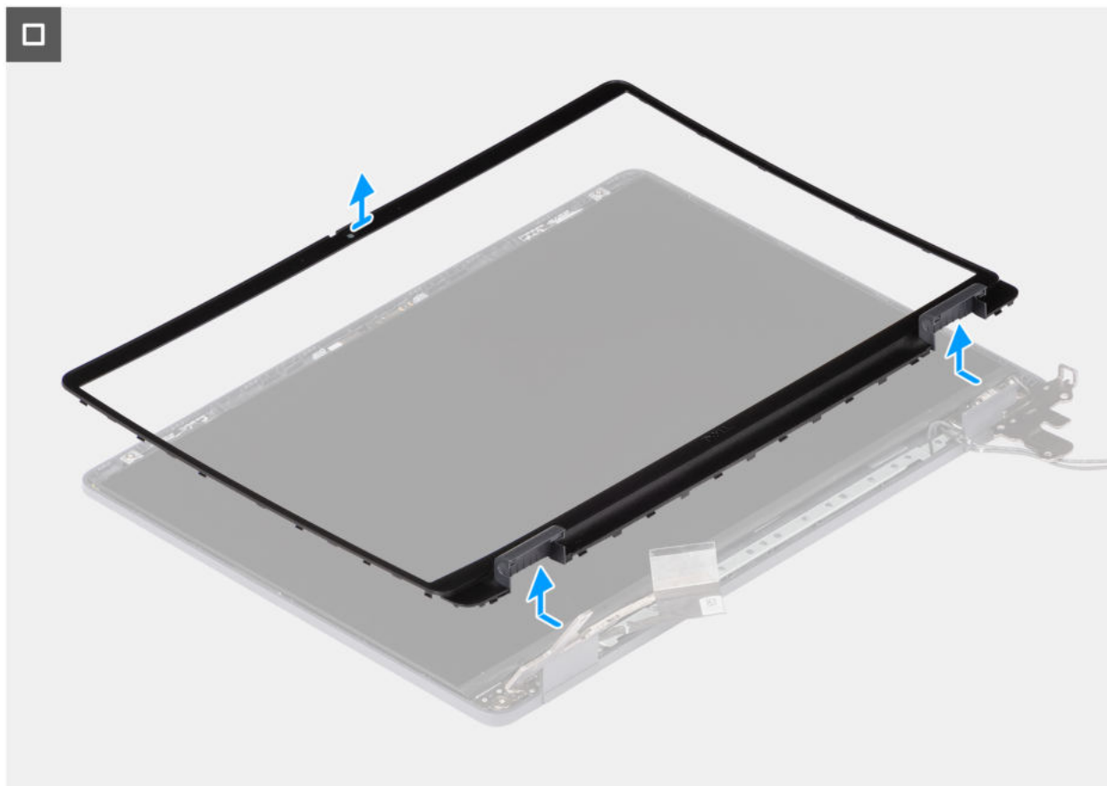
Abbildung 81. Removing the display bezel
