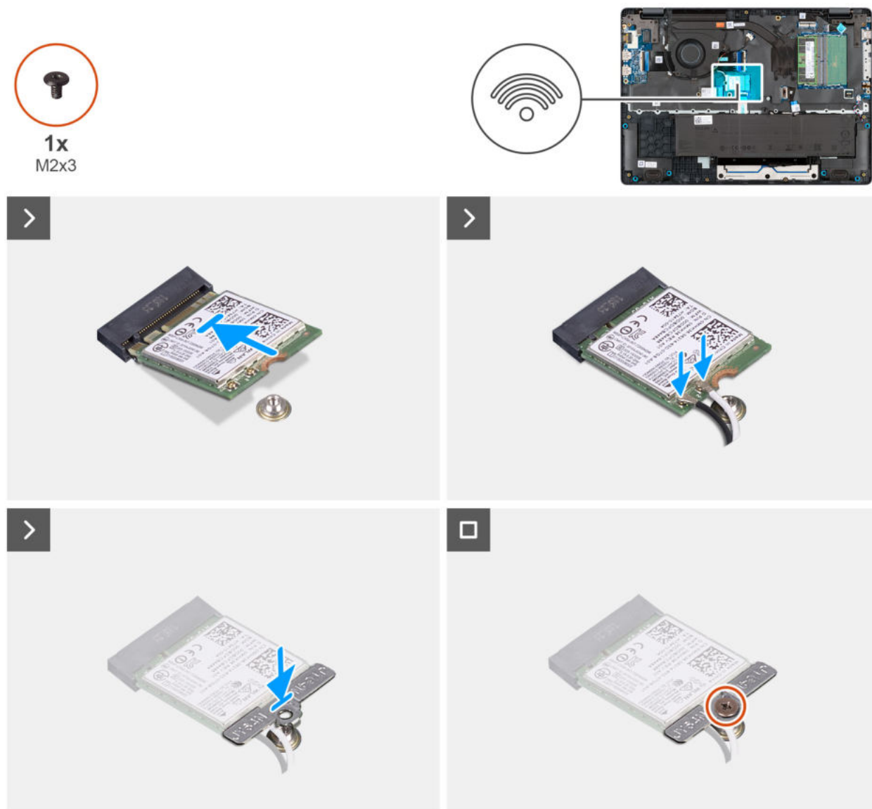
Abbildung 26. Installing the wireless card
