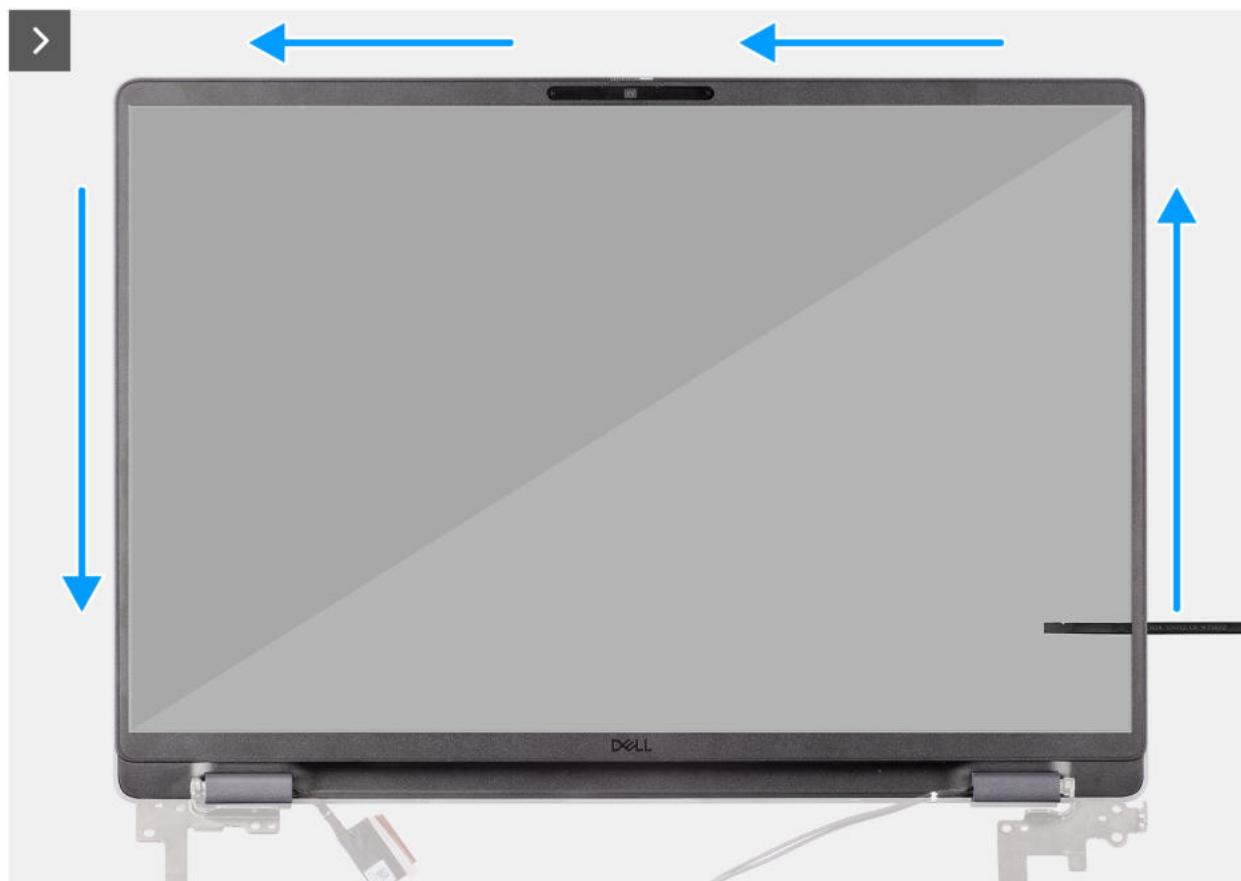
Abbildung 80. Removing the display bezel
