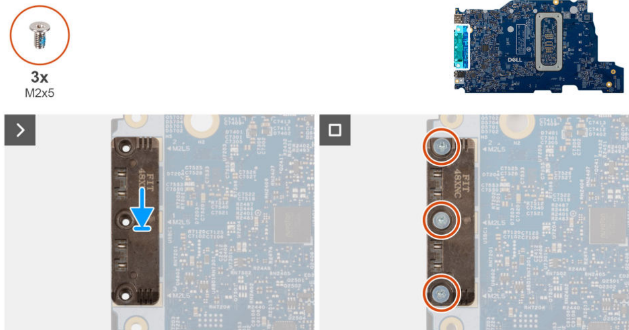
Abbildung 59. Installing the USB Type-C module
