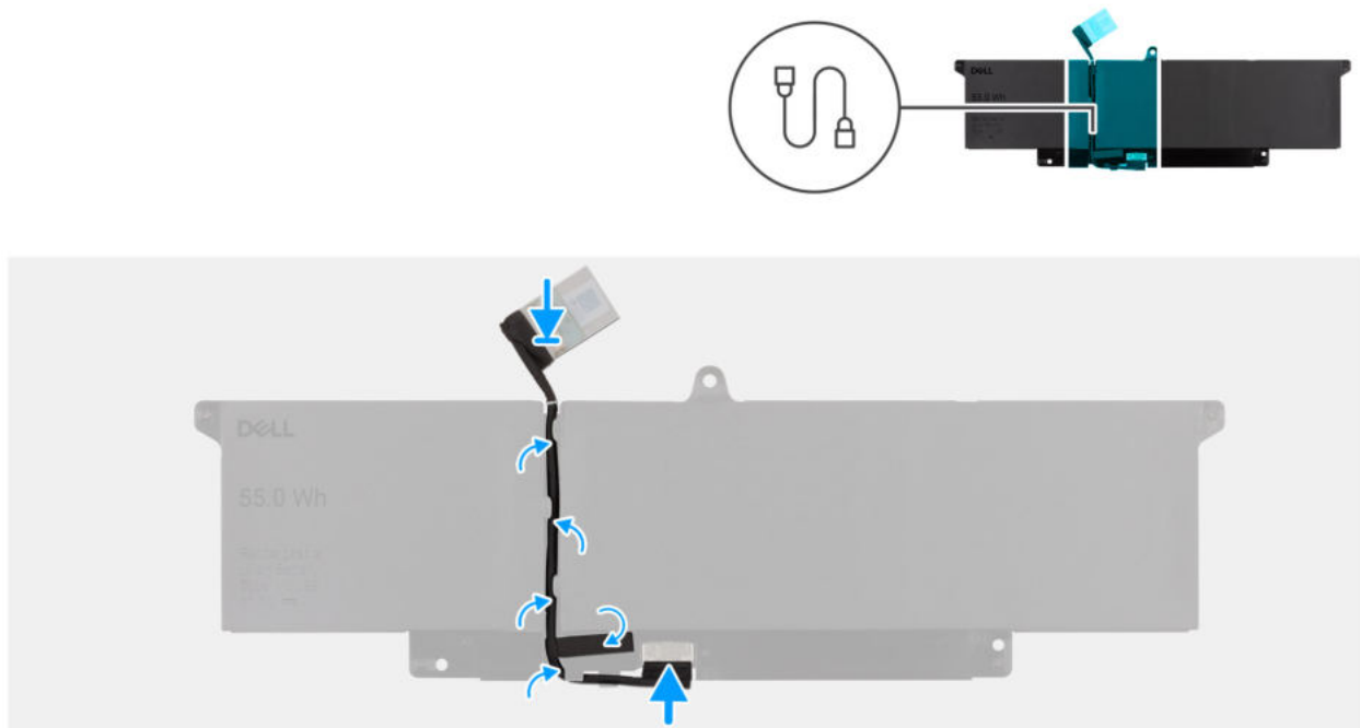
Abbildung 20. Installing the battery cable
