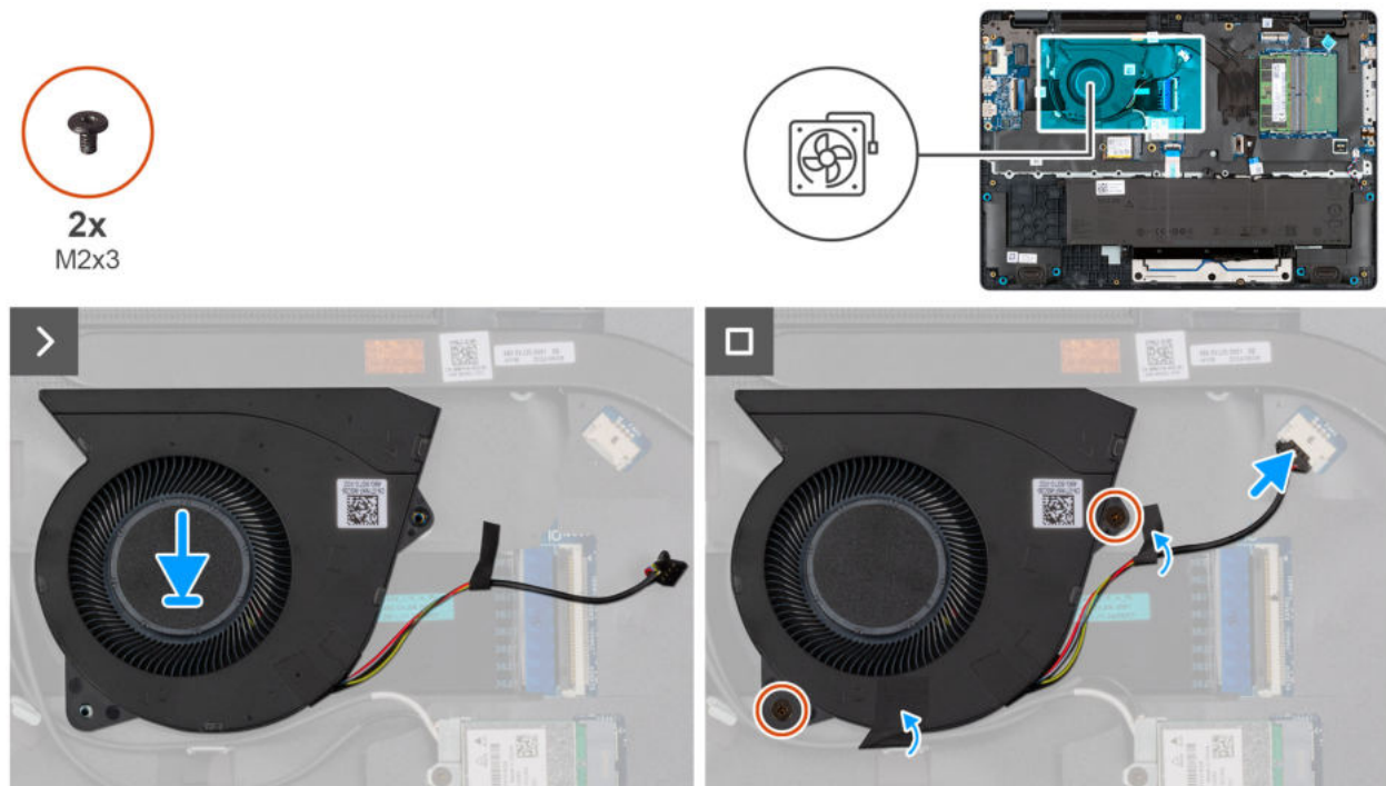
Abbildung 31. Installing the fan
