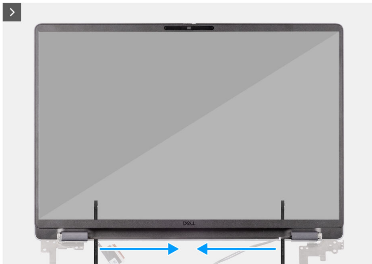
Abbildung 78. Removing the display bezel
