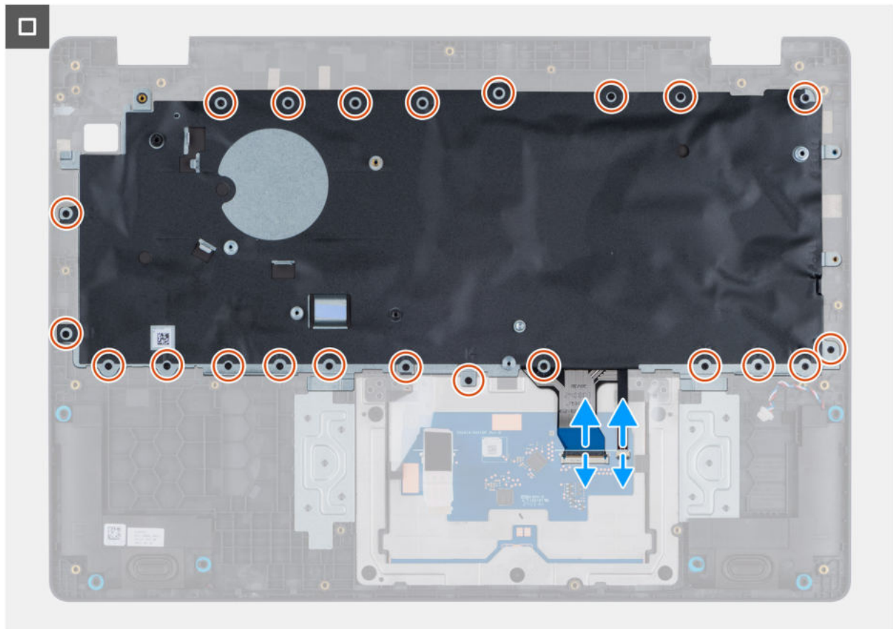
Abbildung 65. Installing the keyboard
