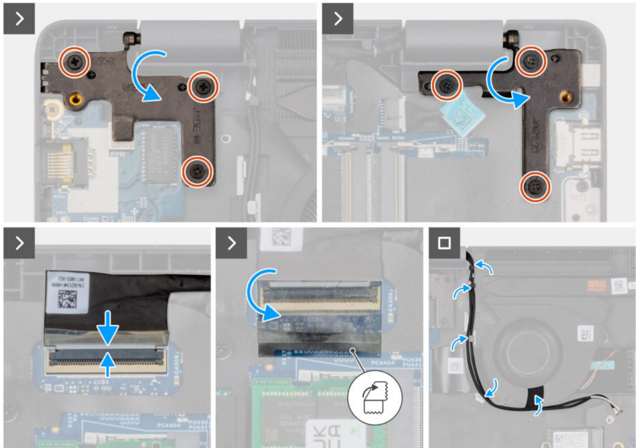
Abbildung 76. Installing the display assembly
