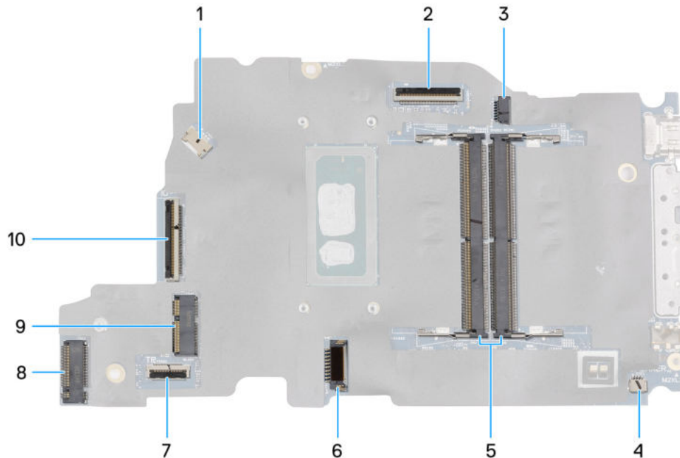
Abbildung 46. System-board connectors
