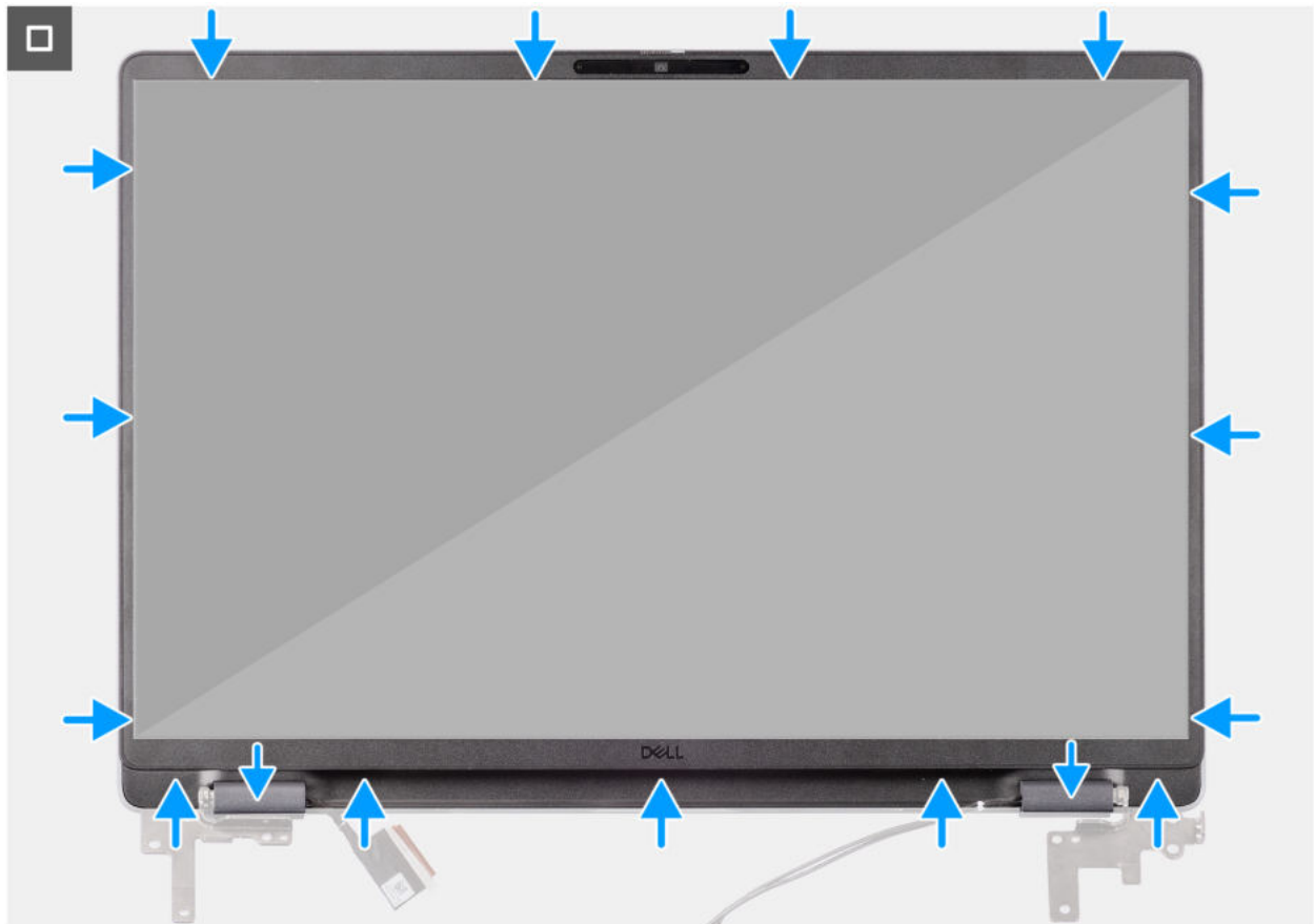
Abbildung 83. Installing the display bezel
