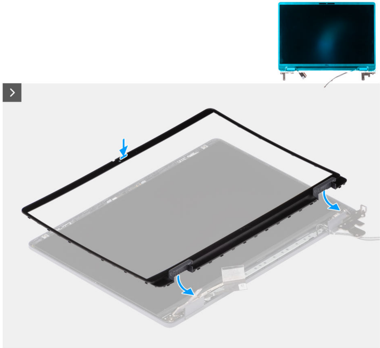
Abbildung 82. Installing the display bezel
