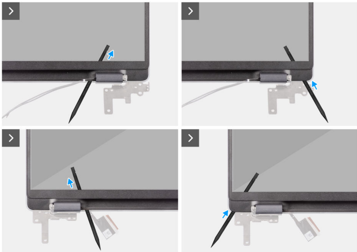
Abbildung 79. Removing the display bezel
