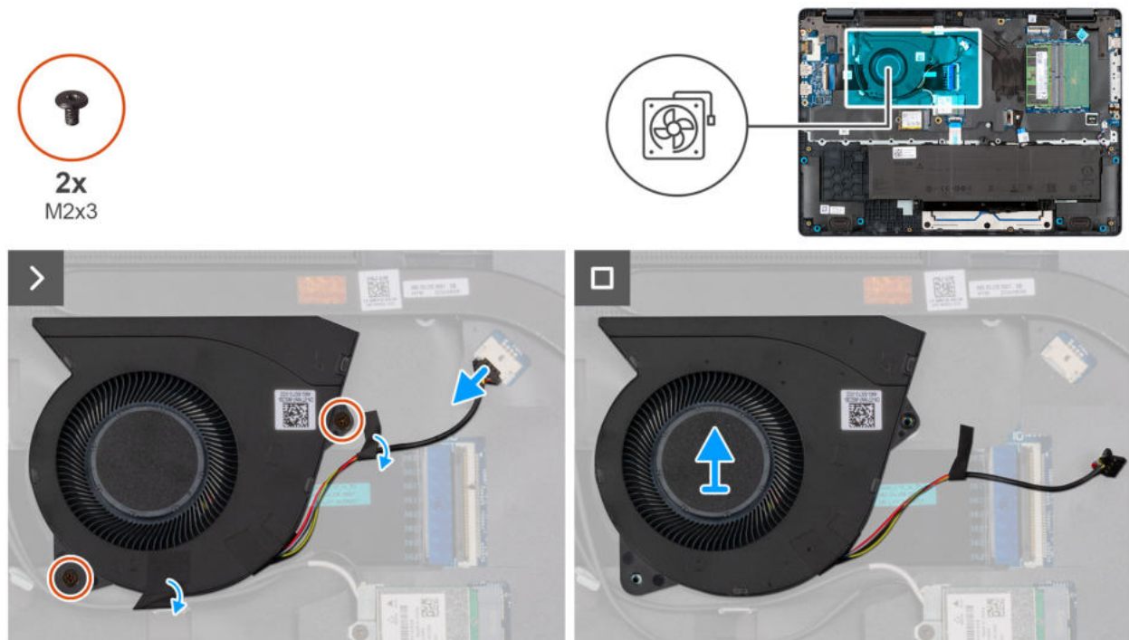
Abbildung 30. Removing the fan
