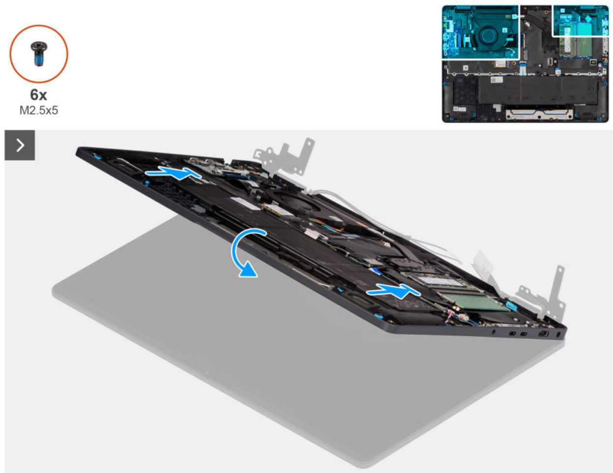
Abbildung 75. Installing the display assembly
