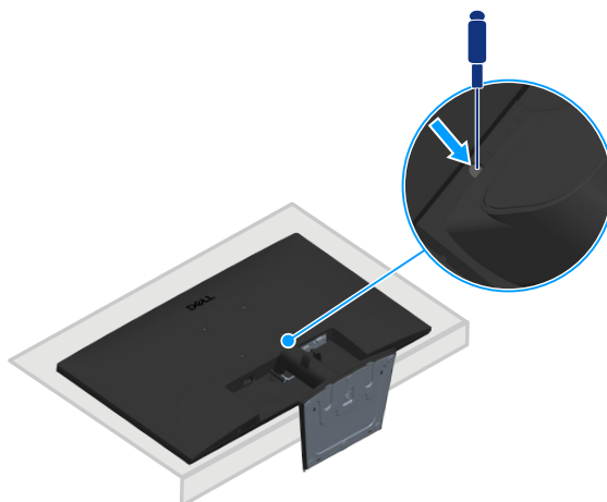
Abbildung 22. Freigabetaste mit einem langen Schraubendreher drücken
