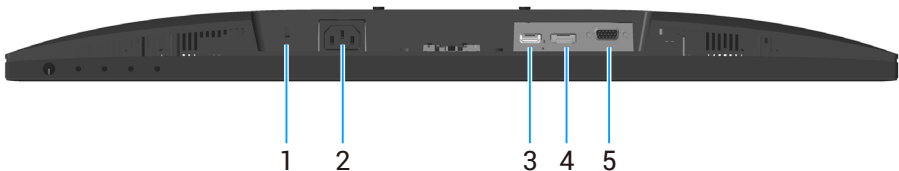
Abbildung 4. Ansicht von unten
