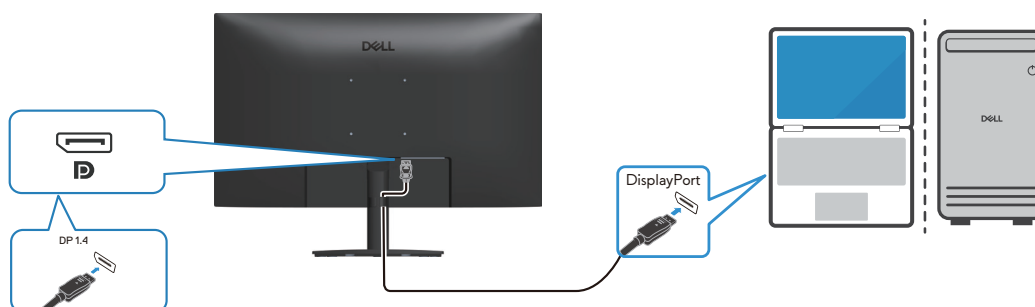
Abbildung 18. DisplayPort-Kabel anschließen
