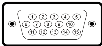
Abbildung 5. VGA-Port
