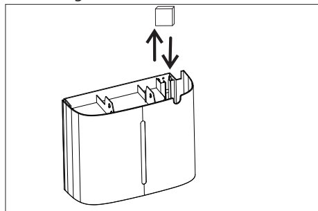
Abb. 6 – Schwimmer einsetzen
