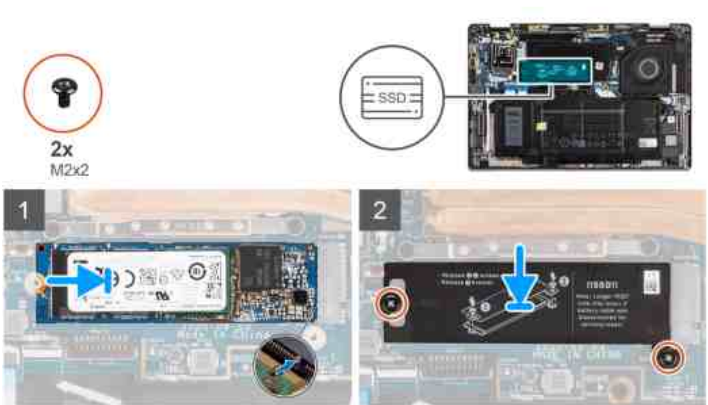
Abbildung 4. Einbauen des SSD (für Computer nur mit WLAN-Unterstützung)
