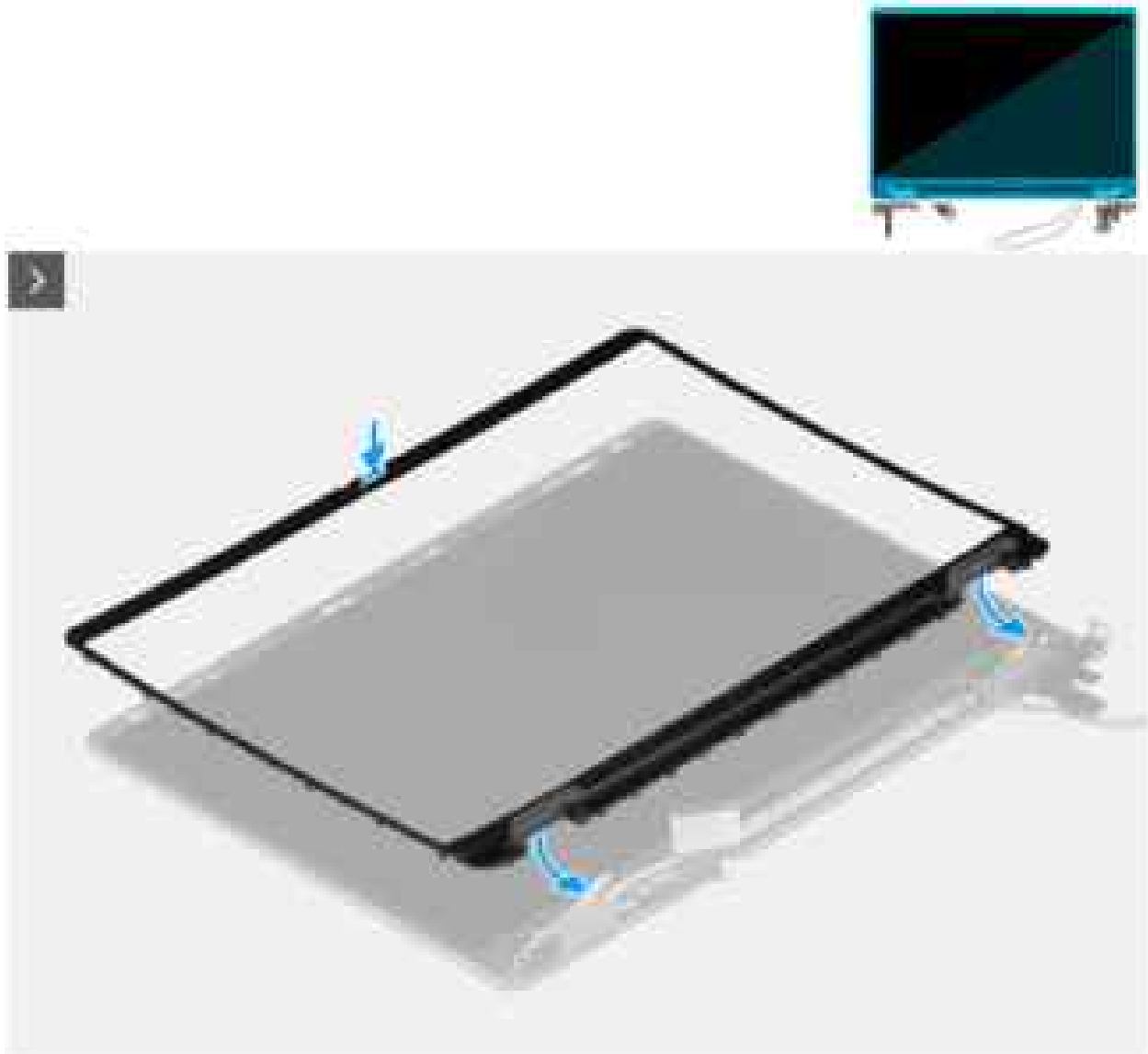
Abbildung 109. Einbauen der Bildschirmblende
