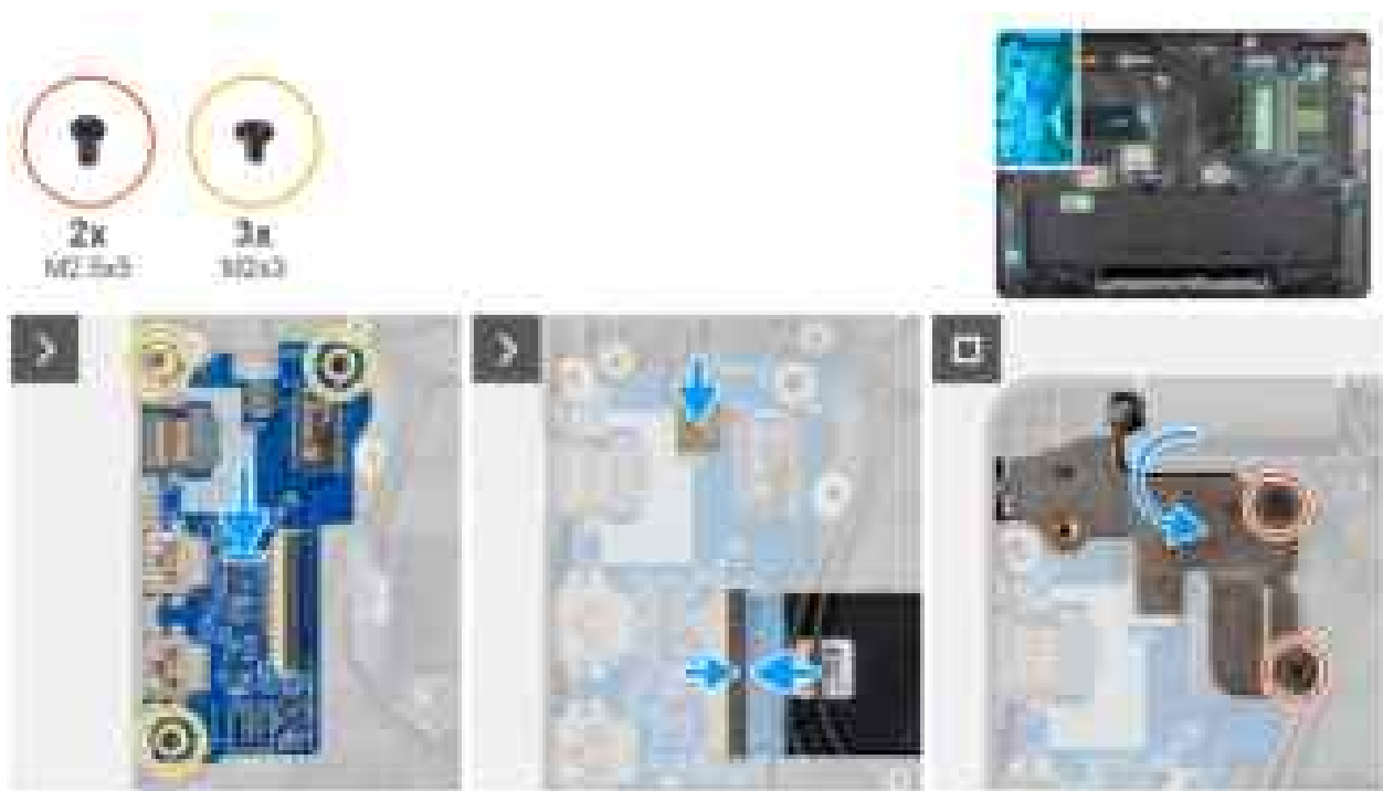
Abbildung 50. Installieren der I/O-Platine
