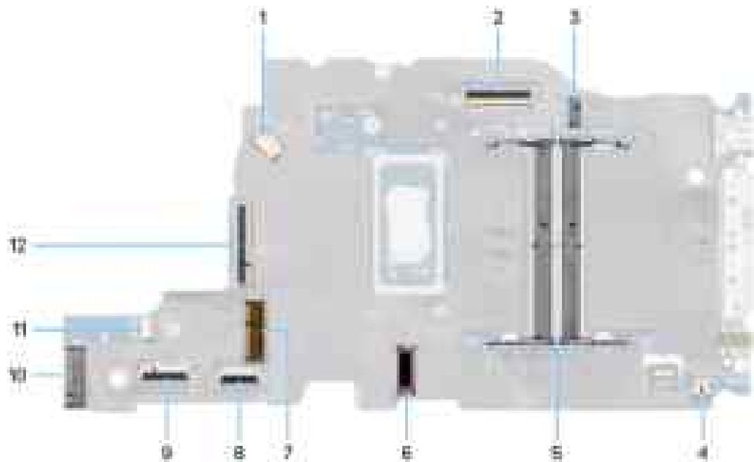
Abbildung 69. Hauptplattenanschlüsse
