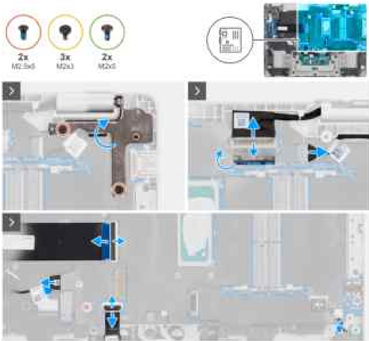
Abbildung 64. Entfernen der Systemplatine
