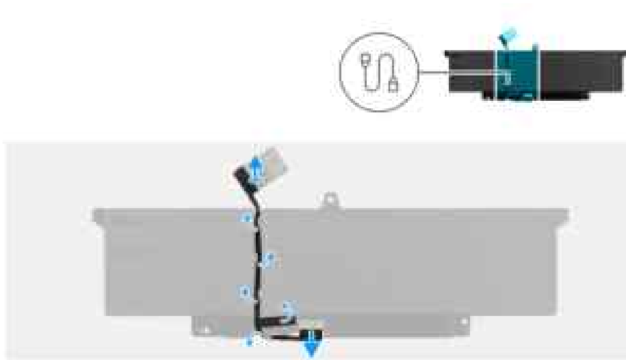
Abbildung 19. Entfernen des Akkukabels
