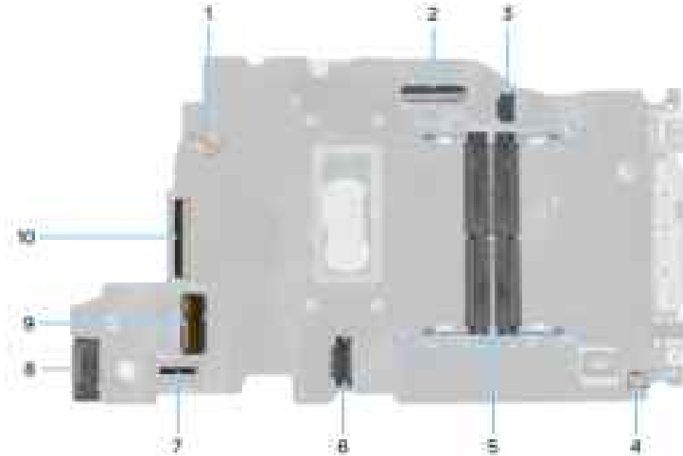
Abbildung 57. Hauptplattenanschlüsse
