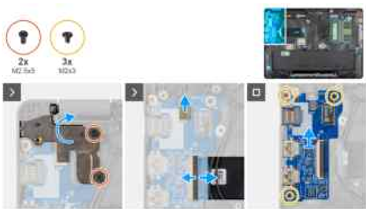
Abbildung 49. Entfernen der E/A-Platine
