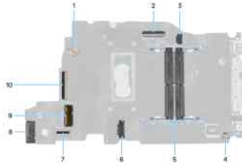
Abbildung 60. Hauptplattenanschlüsse
