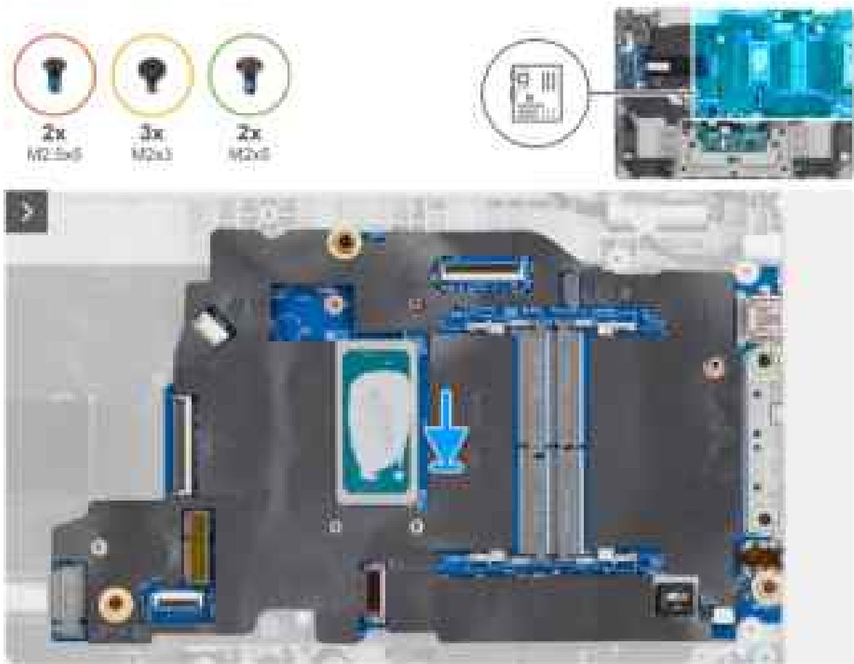
Abbildung 67. Einbauen der Systemplatine
