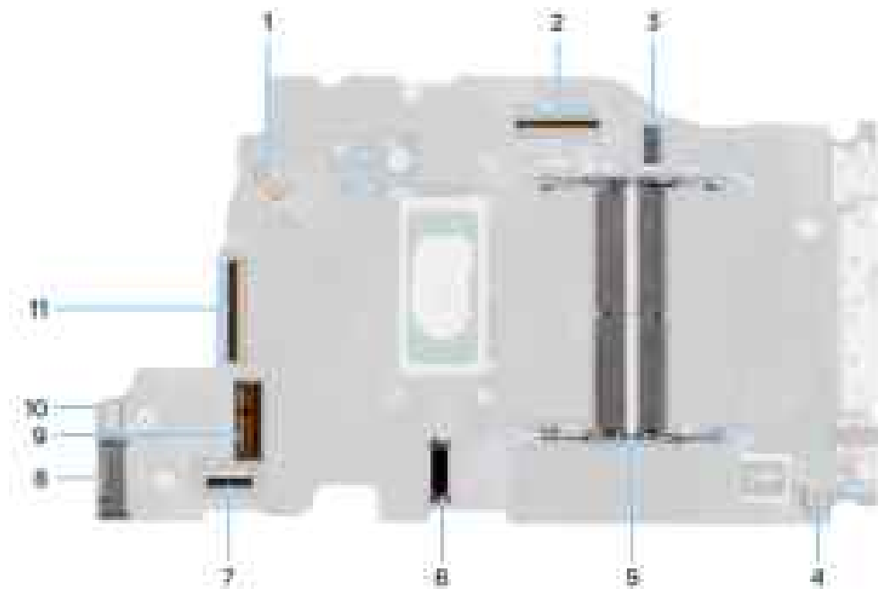
Abbildung 66. Hauptplattenanschlüsse
