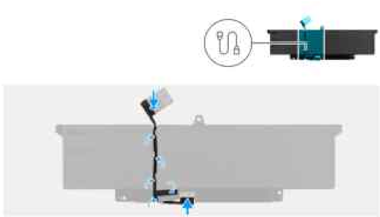
Abbildung 20. Einsetzen des Akkukabels
