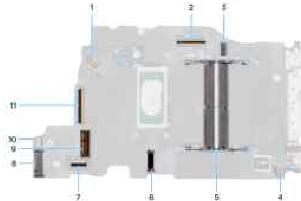
Abbildung 63. Hauptplattenanschlüsse
