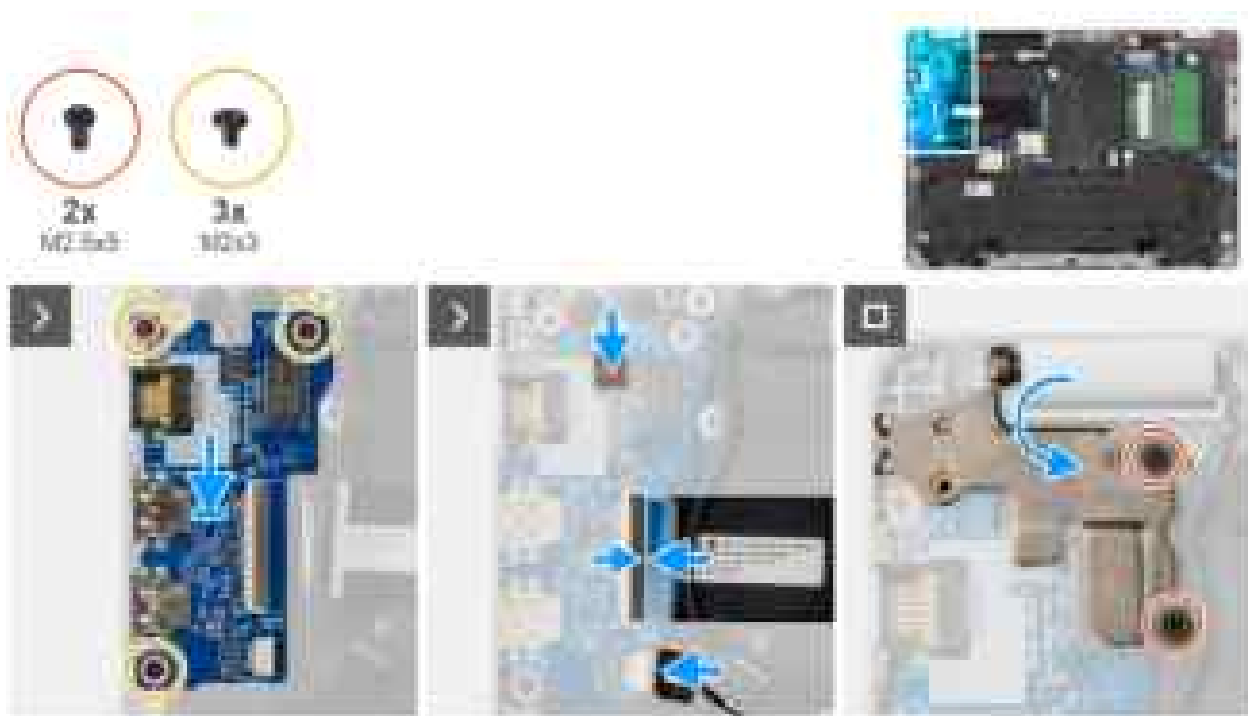
Abbildung 52. Installieren der I/O-Platine
