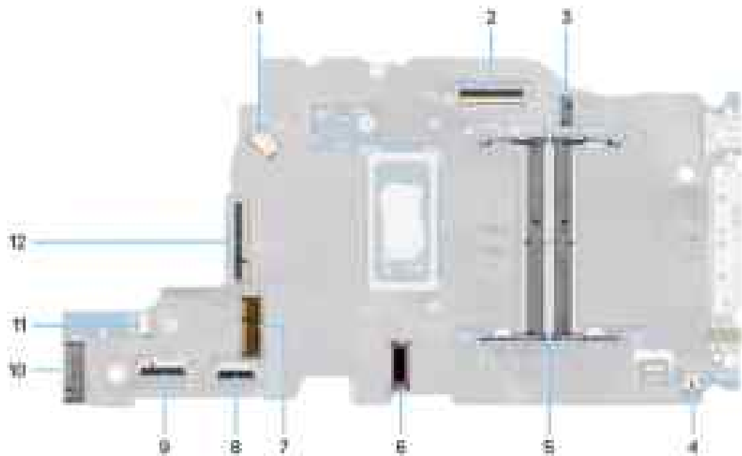
Abbildung 72. Hauptplatinenanschlüsse
