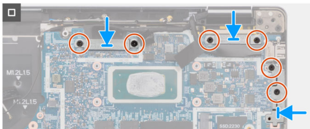
Abbildung 57. Systemplatine
