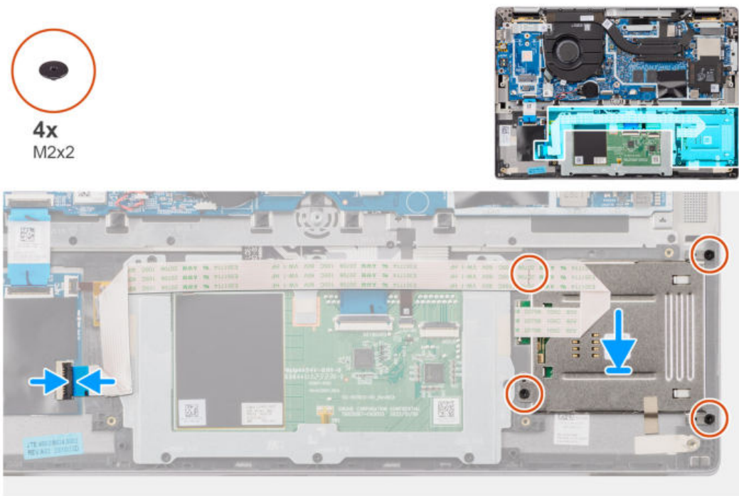
Abbildung 47. Einbauen des Smartcardlesegeräts
