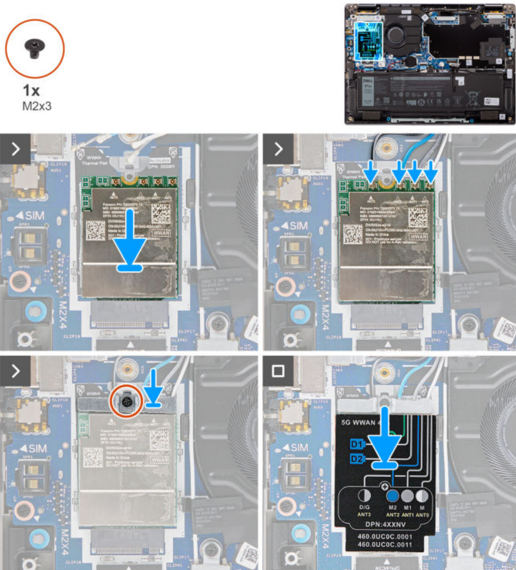
Abbildung 24. Einbauen der WWAN-Karte
