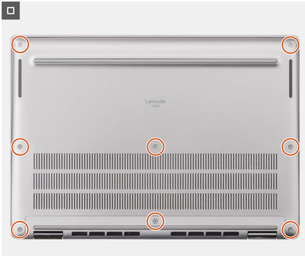
Abbildung 20. Anbringen der Bodenabdeckung
