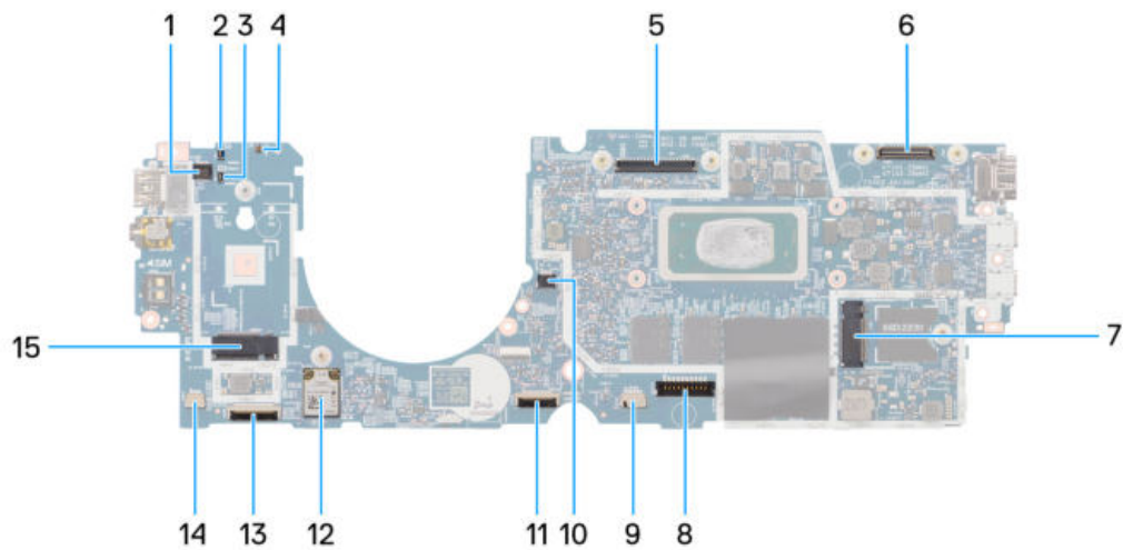
Abbildung 48. Systemplatinenbeschriftung
