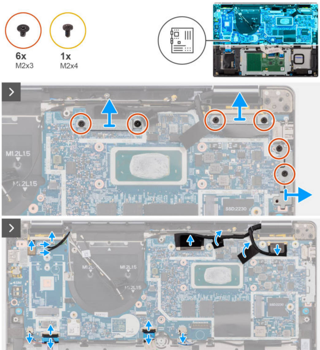
Abbildung 49. Entfernen der Systemplatine
