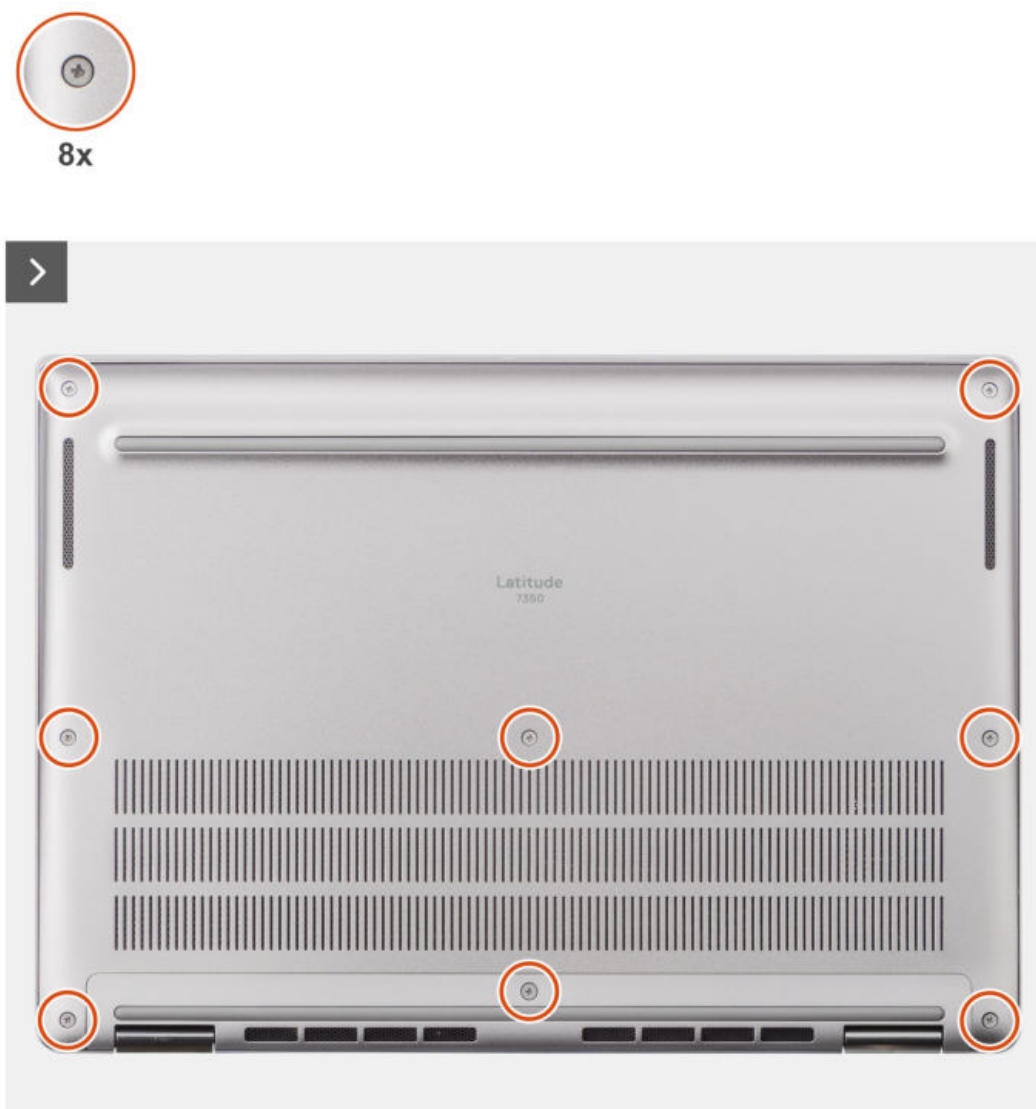
Abbildung 15. Entfernen der Bodenabdeckung
