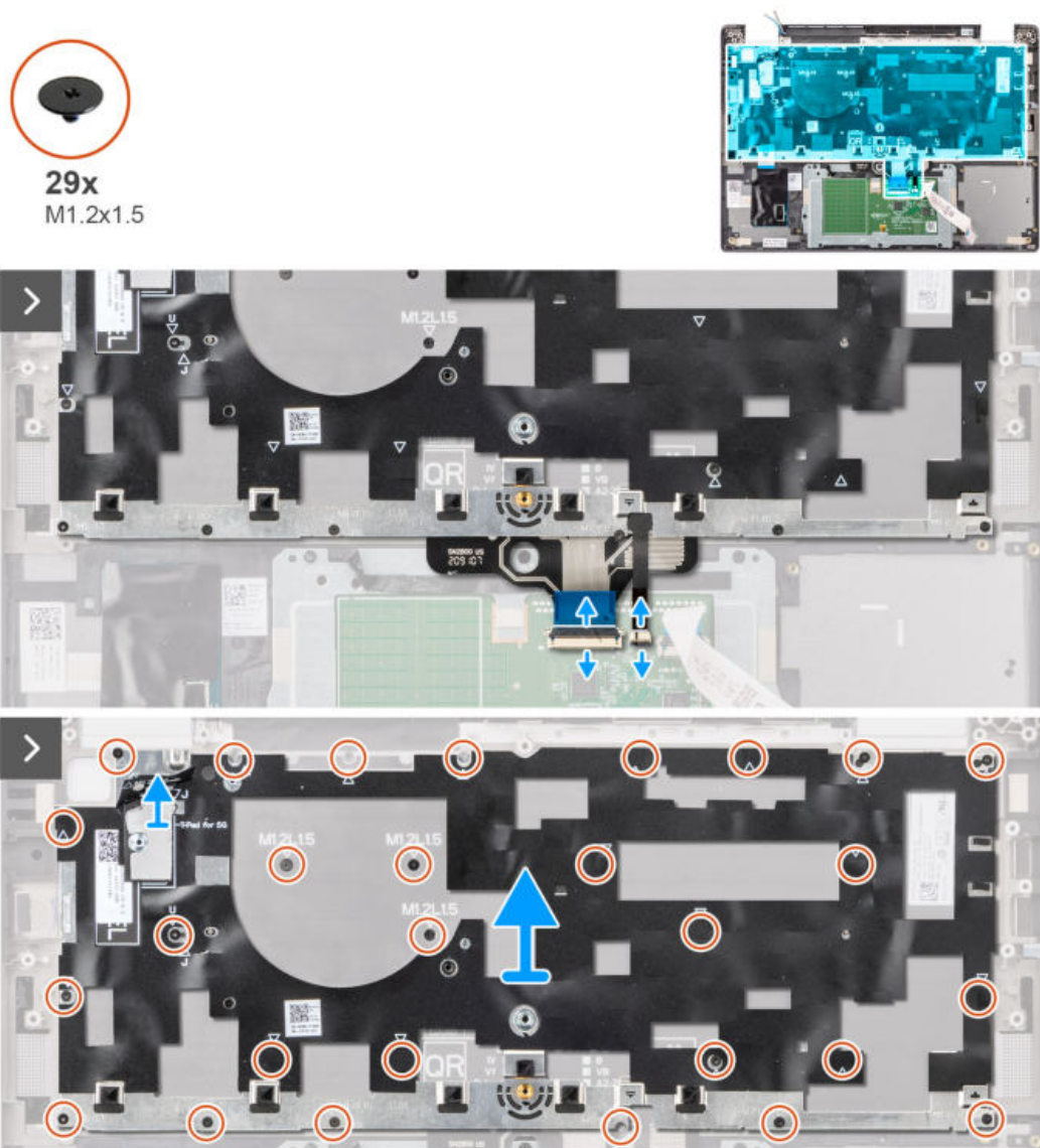
Abbildung 62. Entfernen der Tastatur
