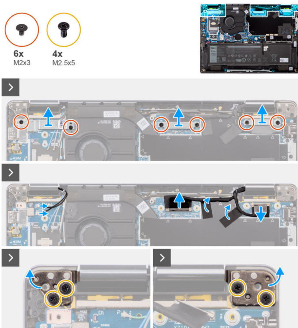
Abbildung 41. Entfernen der Bildschirmbaugruppe
