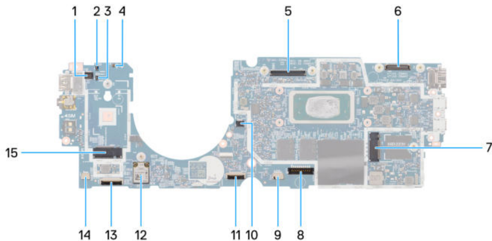
Abbildung 55. Systemplatinebeschriftung
