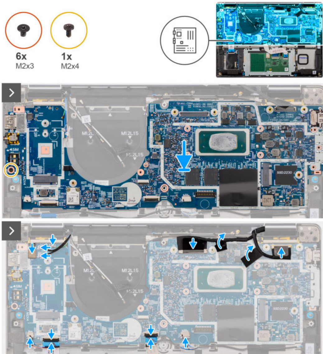
Abbildung 56. Installation der Systemplatine
