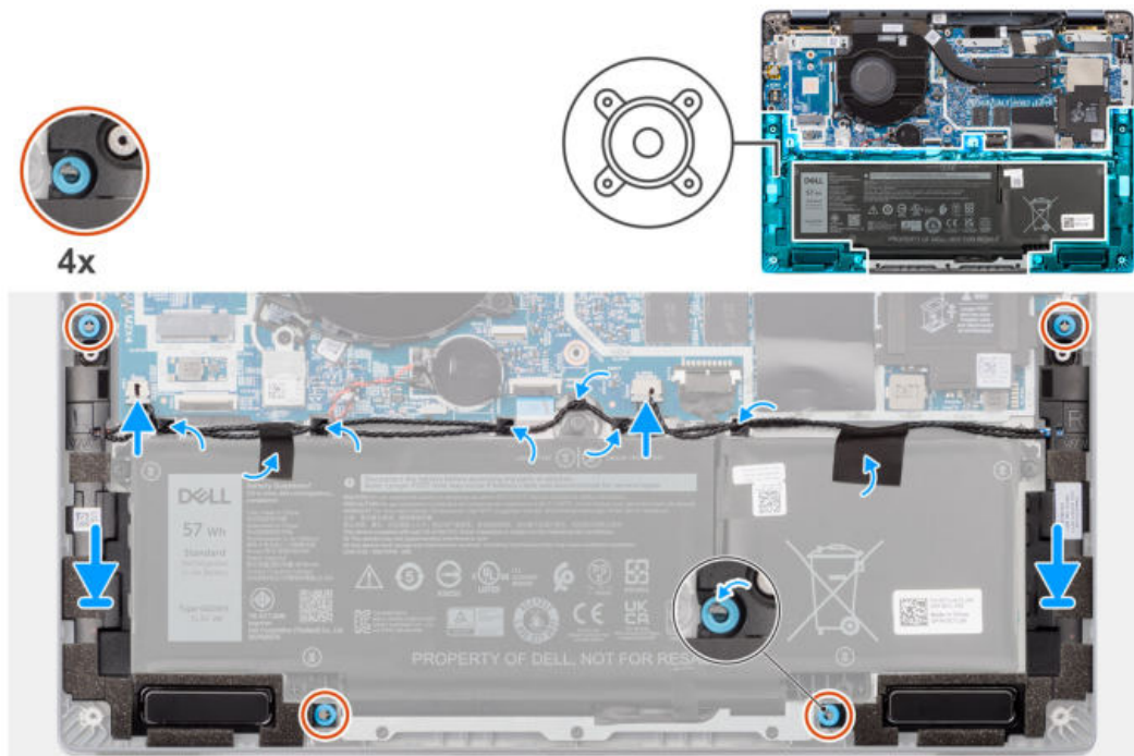
Abbildung 26. Einbauen der Lautsprecher für den Mainstream
