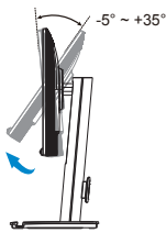
(Neigung)
