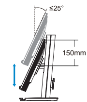
(Höhenverstellung)
