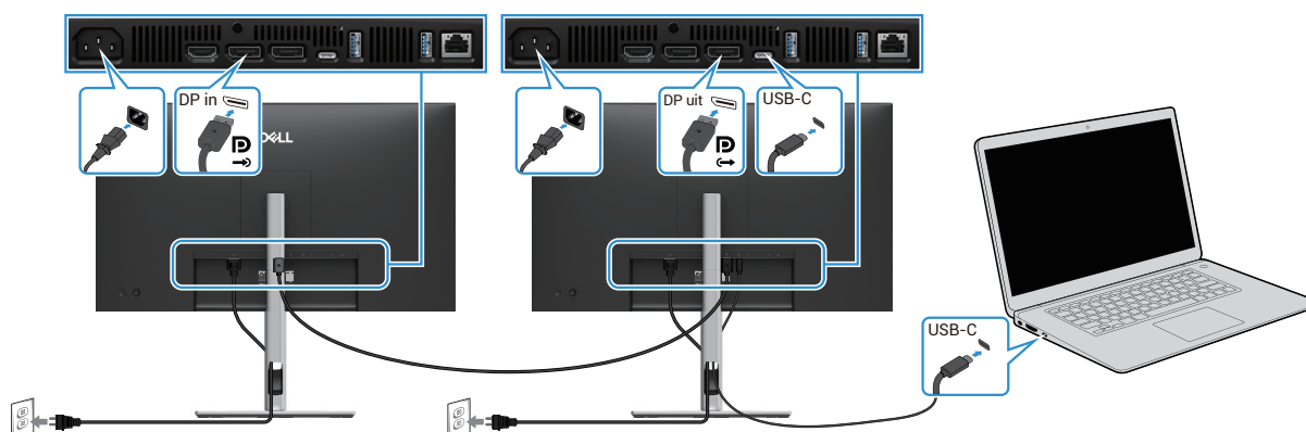
Afbeelding 33. De monitor voor de USB-C MST-functie aansluiten
