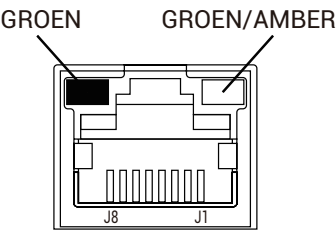
Afbeelding 13. RJ45-poort-connector
