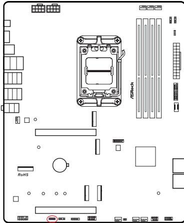
RGB_LED1
