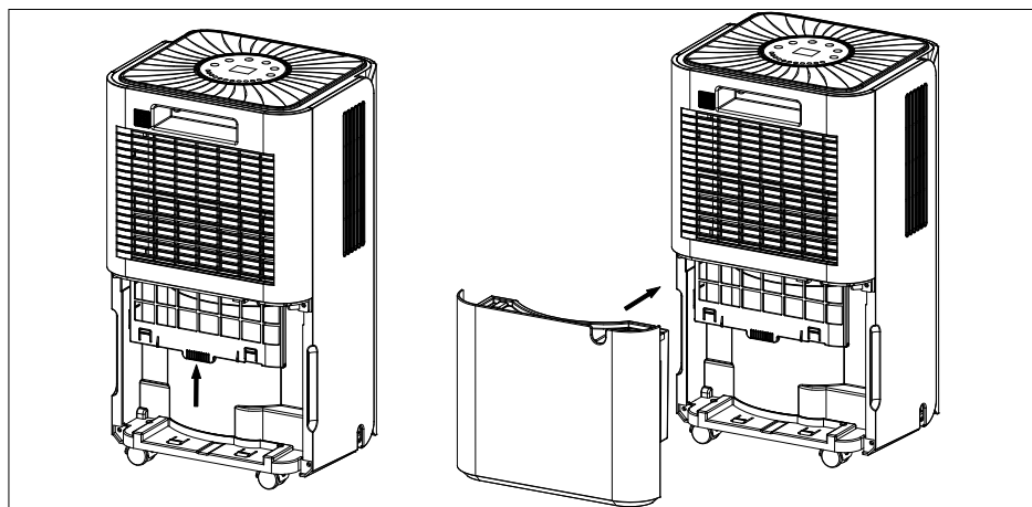
Fig. 10 – Inserimento del filtro
