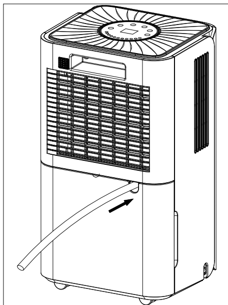
Fig. 5 – Fixer le tuyau de condensat
