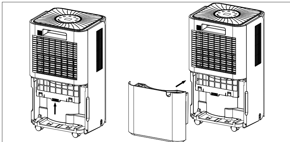
Afb. 10 – Filter plaatsen
