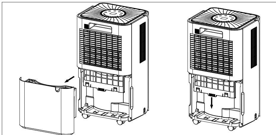
Fig. 8 – Retirer le filtre
