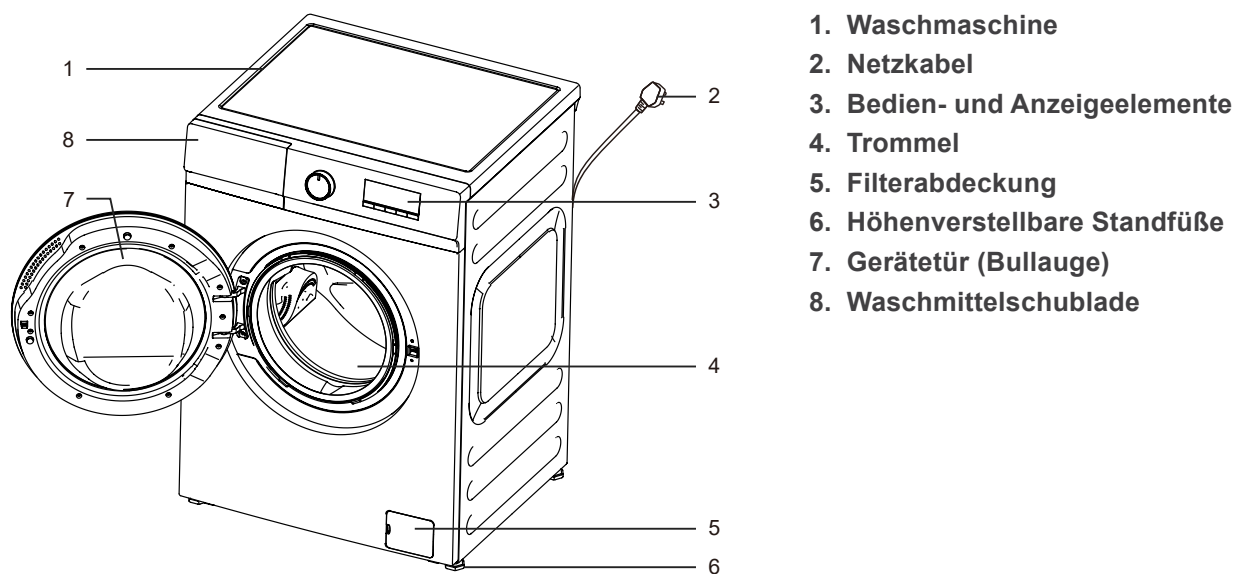
Abb. 2 Waschmaschine
