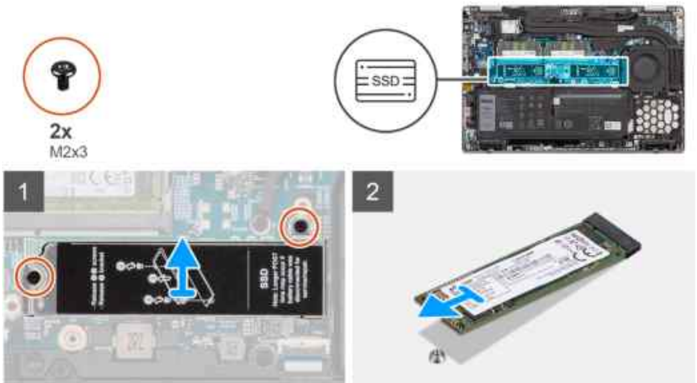
Abbildung 2. M.2-2280-Solid-State-Laufwerk mit Halterung
