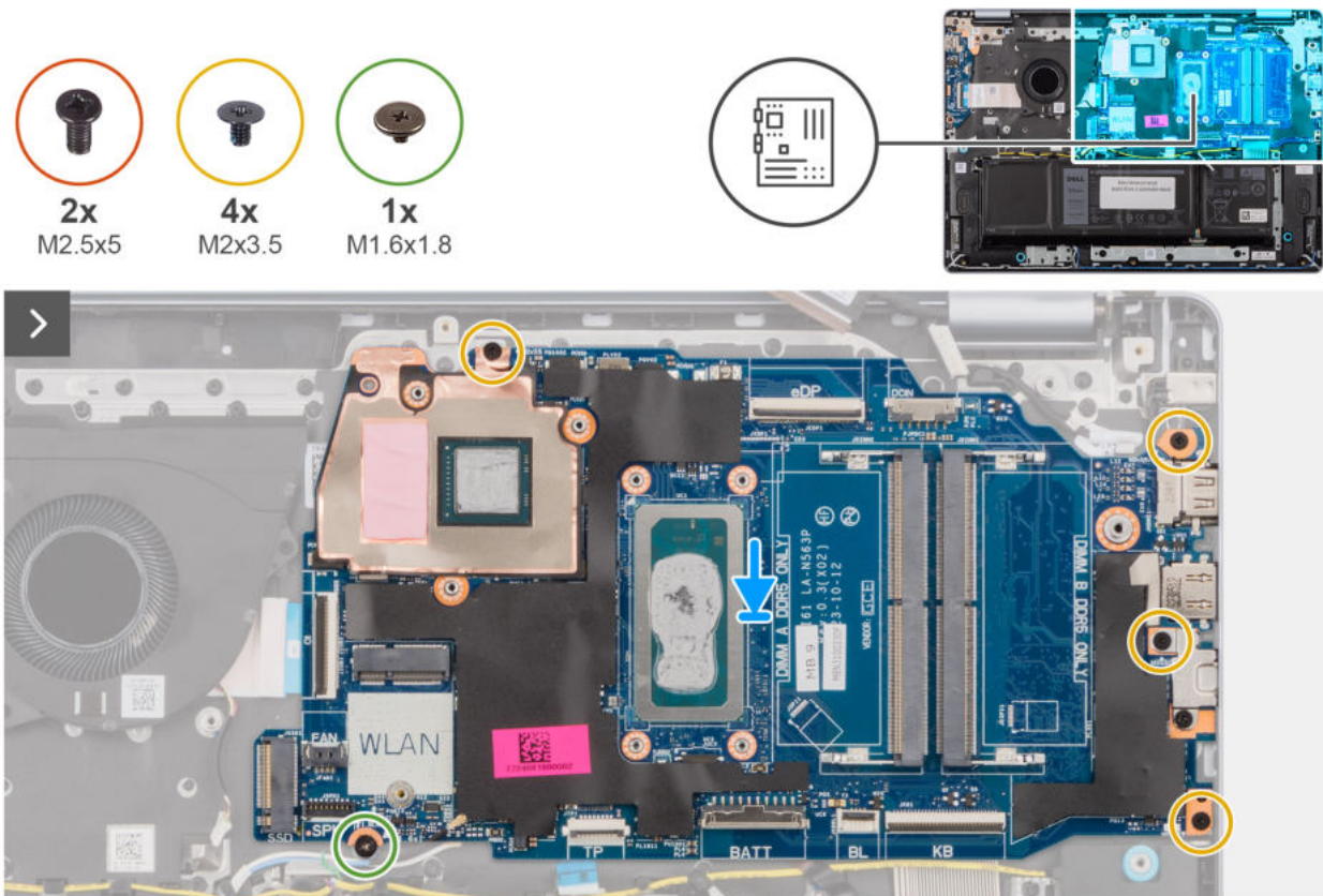
Abbildung 85. Einbauen der Systemplatine
