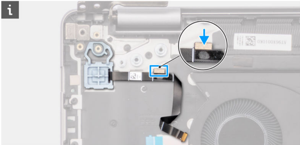
Abbildung 76. Befestigen des Kabels des Fingerabdruck-Lesegeräts an der Handauflagen- und Tastaturbaugruppe
