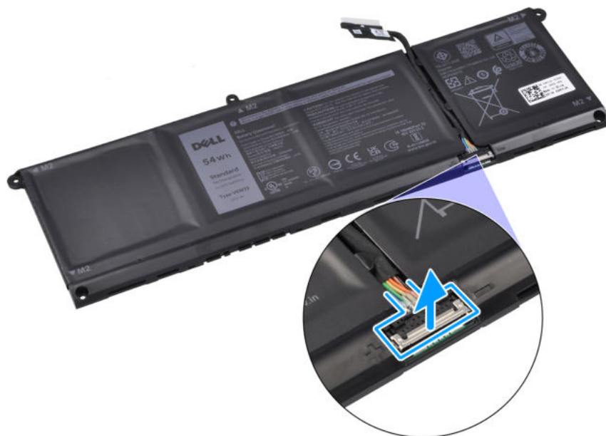
Abbildung 24. Trennen des Akkukabels
