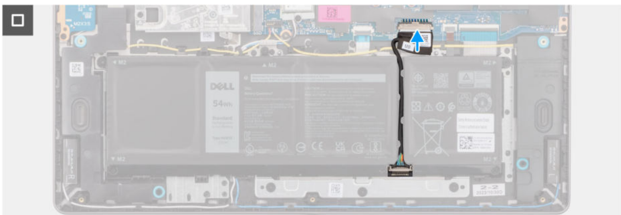
Abbildung 36. Verbinden des Akkukabels
