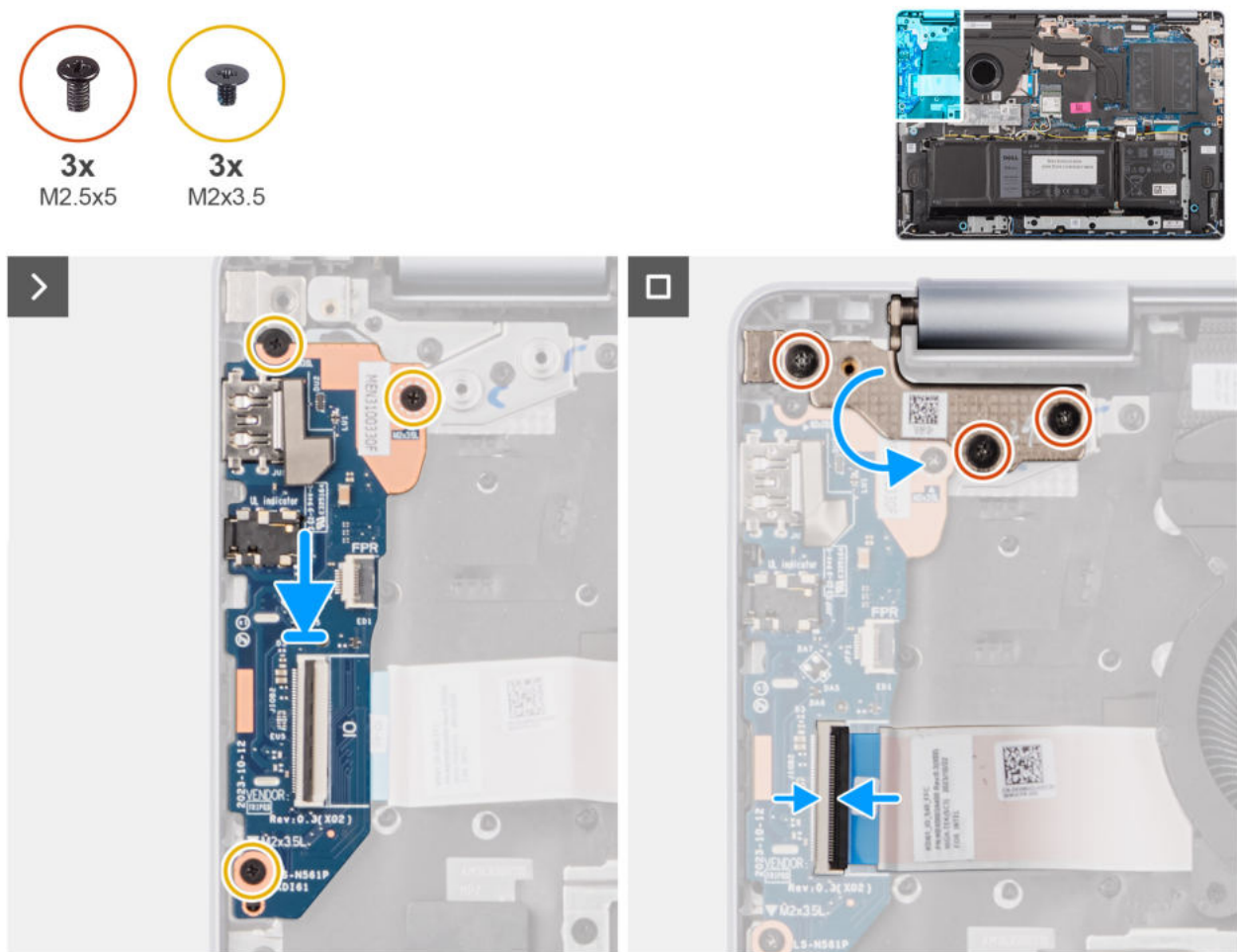
Abbildung 49. Installieren der I/O-Platine
