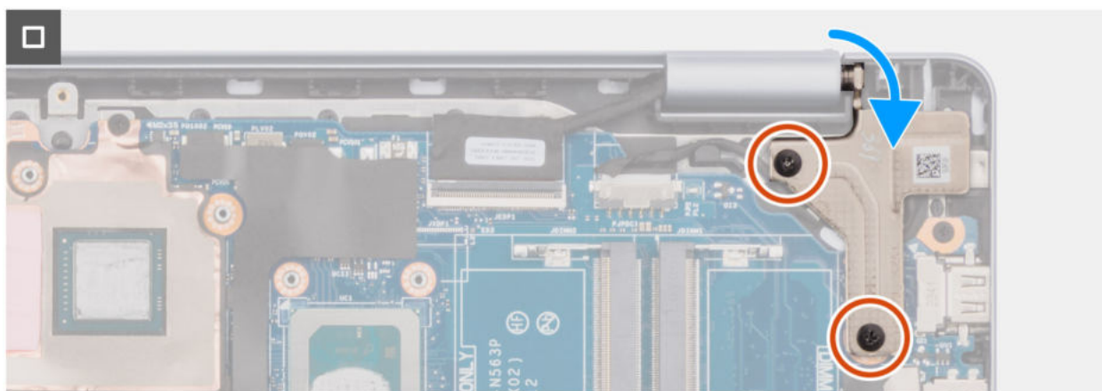
Abbildung 87. Einbauen der Systemplatine
