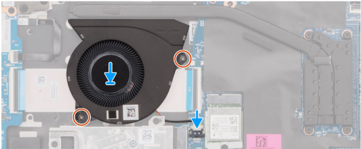
Abbildung 39. Einbauen des Lüfters
