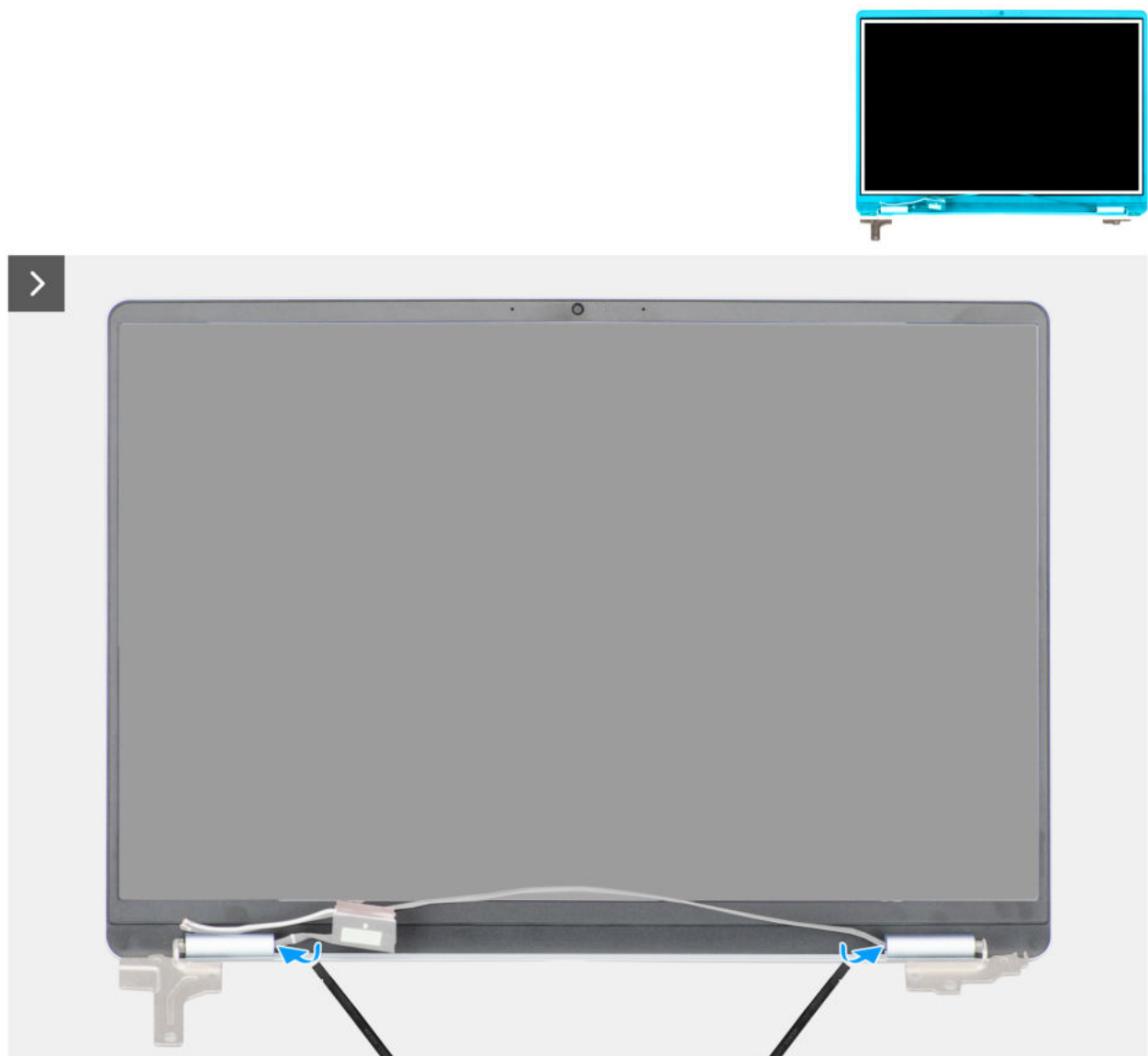
Abbildung 54. Entfernen der Bildschirmblende
