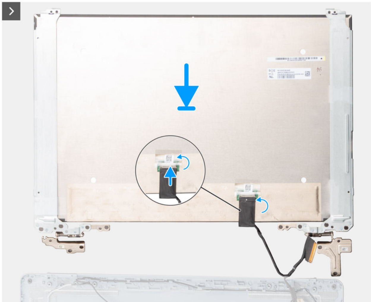
Abbildung 64. Einbauen des Bildschirms
