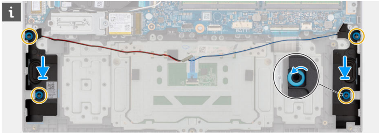
Abbildung 37. Ausrichten der Lautsprecherdichtungen
