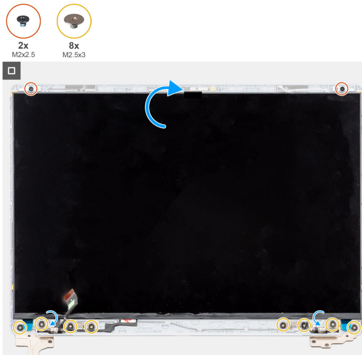
Abbildung 65. Einbauen des Bildschirms
