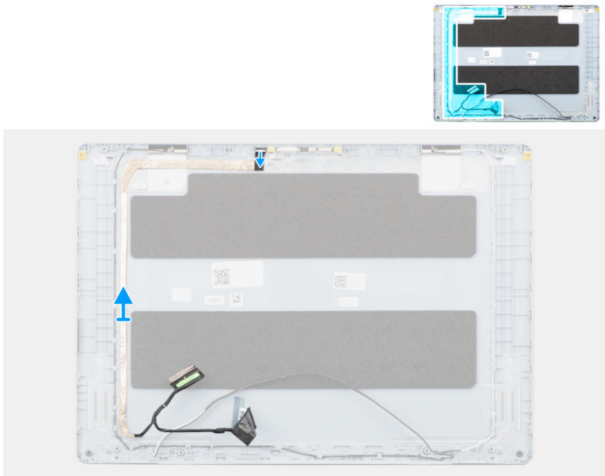
Abbildung 66. Entfernen des Bildschirmkabels
