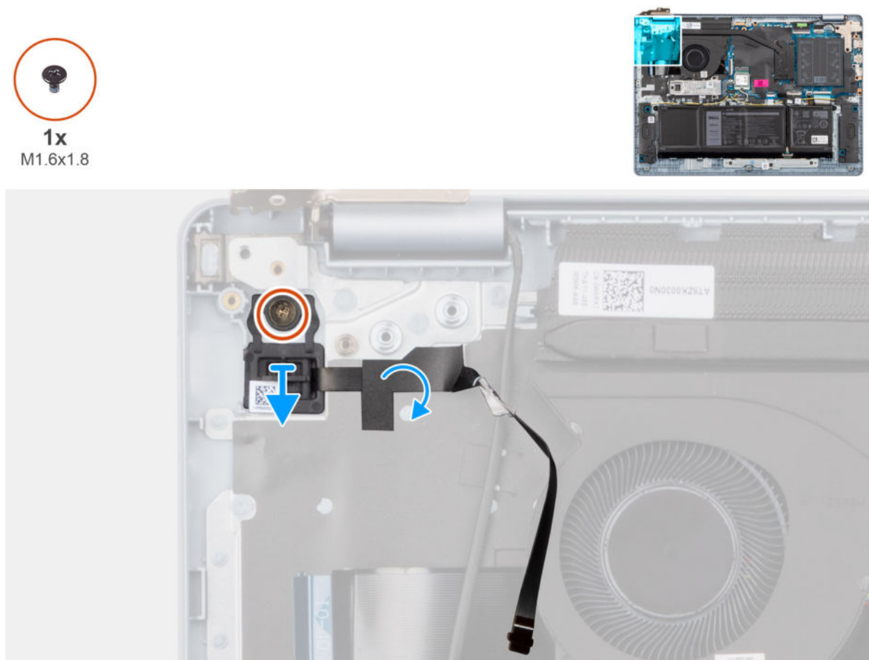
Abbildung 74. Entfernen des Netzschalters mit Fingerabdruck-Lesegerät
