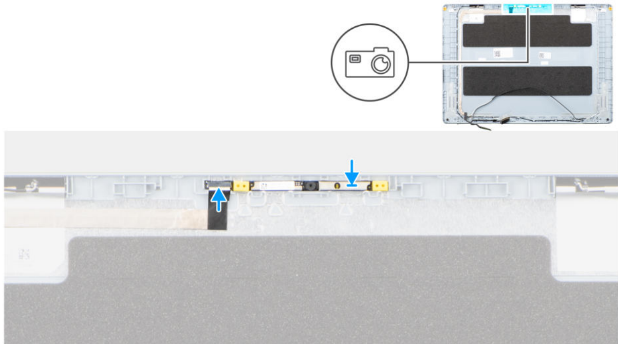
Abbildung 69. Installieren der Kamera
