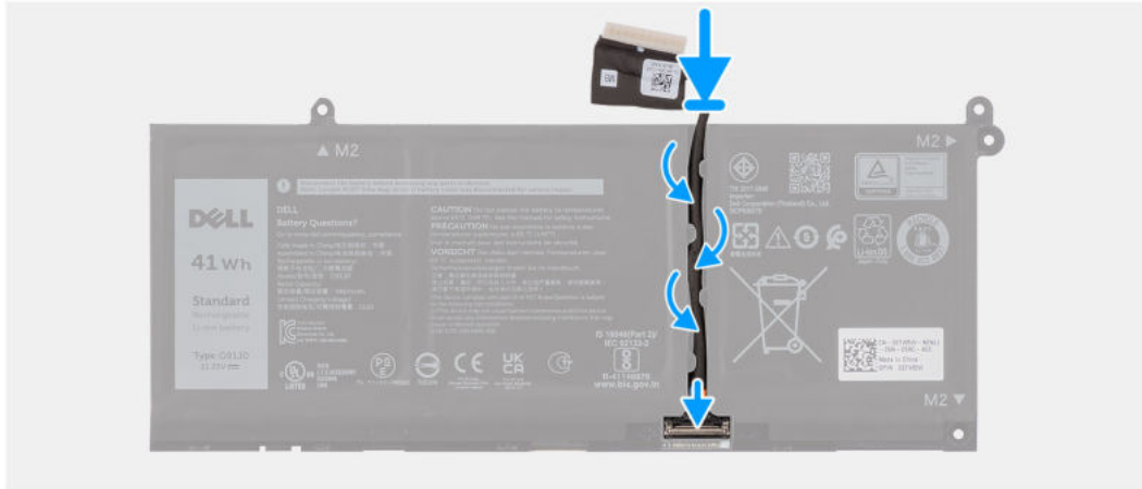
Abbildung 25. Verbinden des Akkukabels
