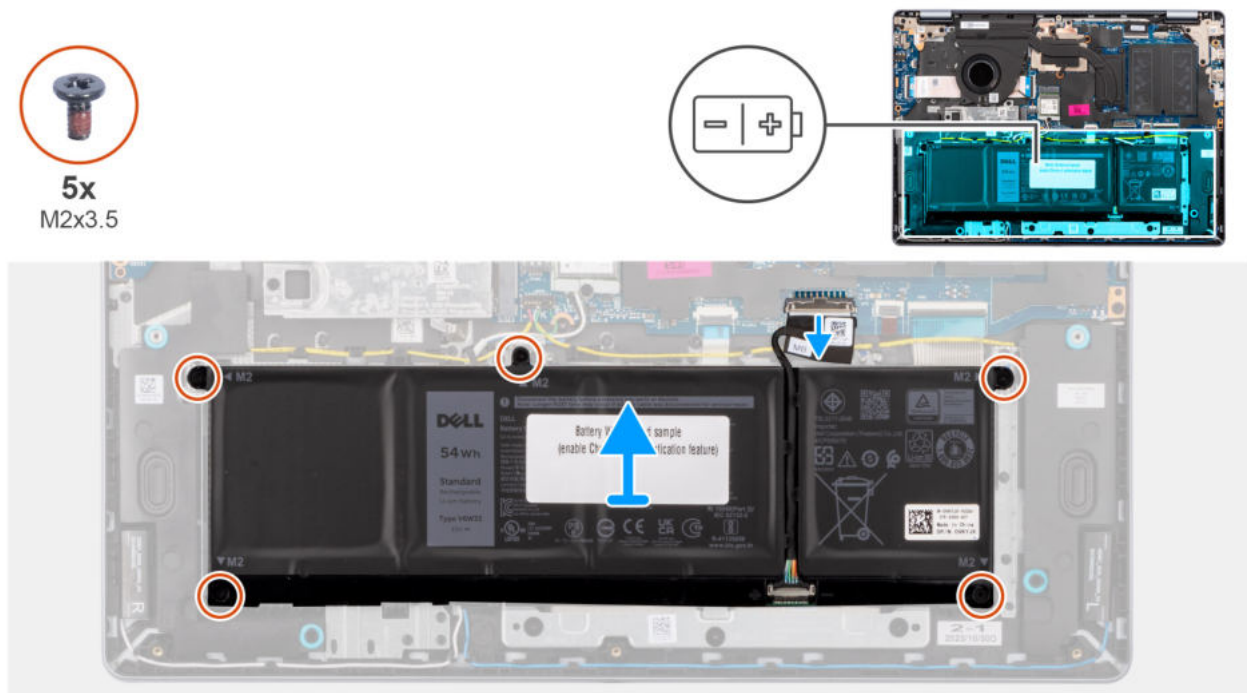
Abbildung 19. Entfernen des 4-Zellen-Akkus
