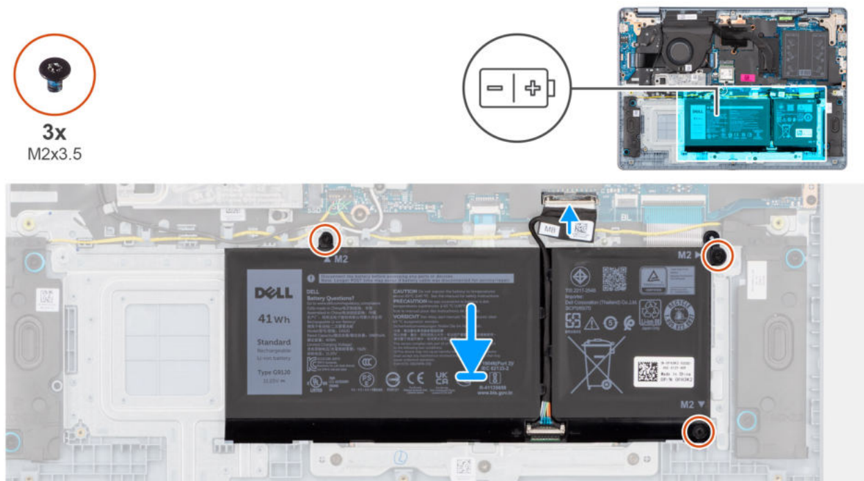
Abbildung 17. Installieren des 3-Zellen-Akkus
