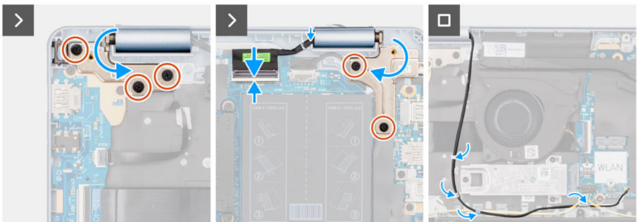
Abbildung 53. Installing the display assembly
