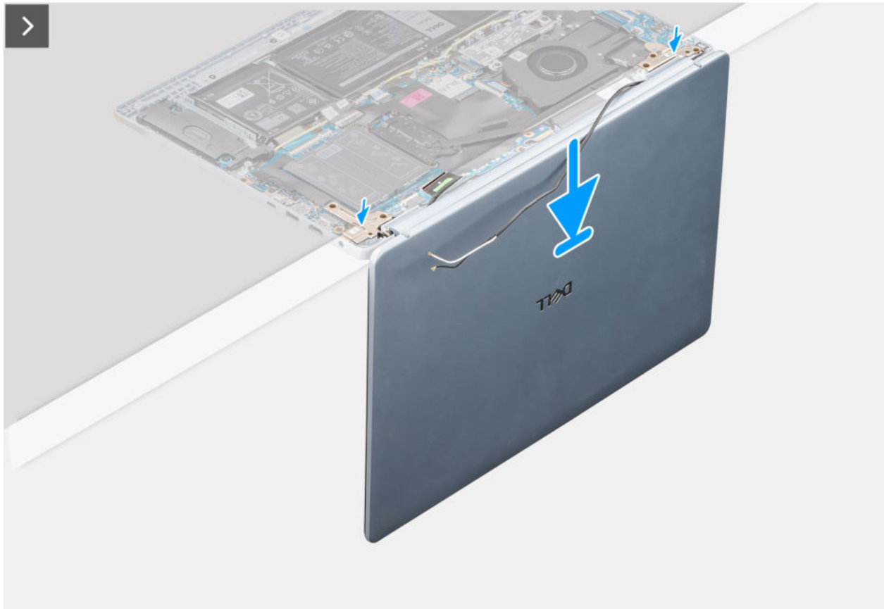
Abbildung 52. Installing the display assembly
