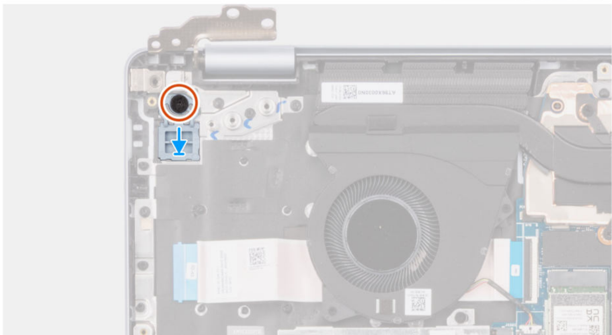
Abbildung 73. Installieren des Netzschalters
