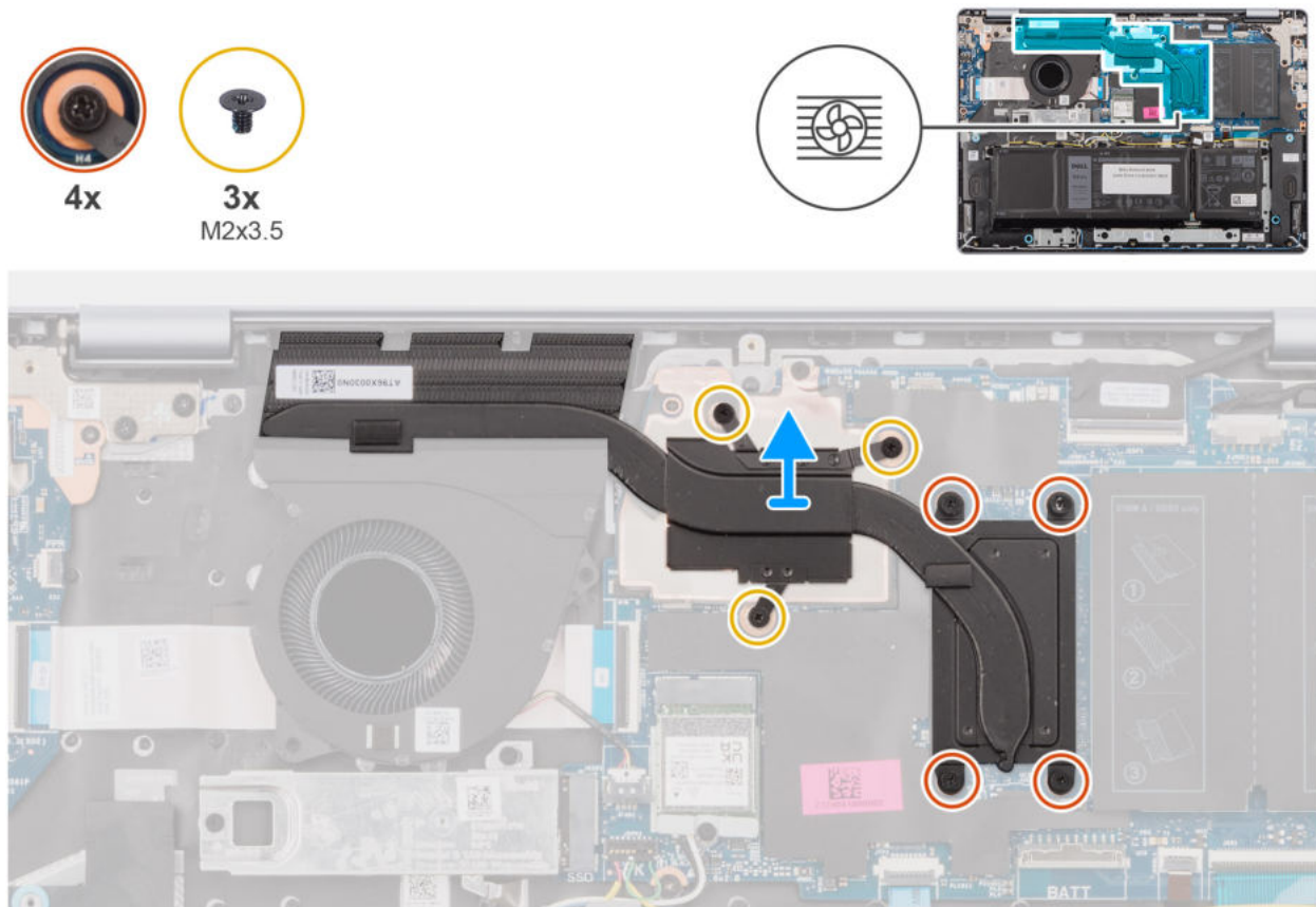
Abbildung 42. Entfernen des Kühlkörpers (bei Computern mit separater Grafikkarte)
