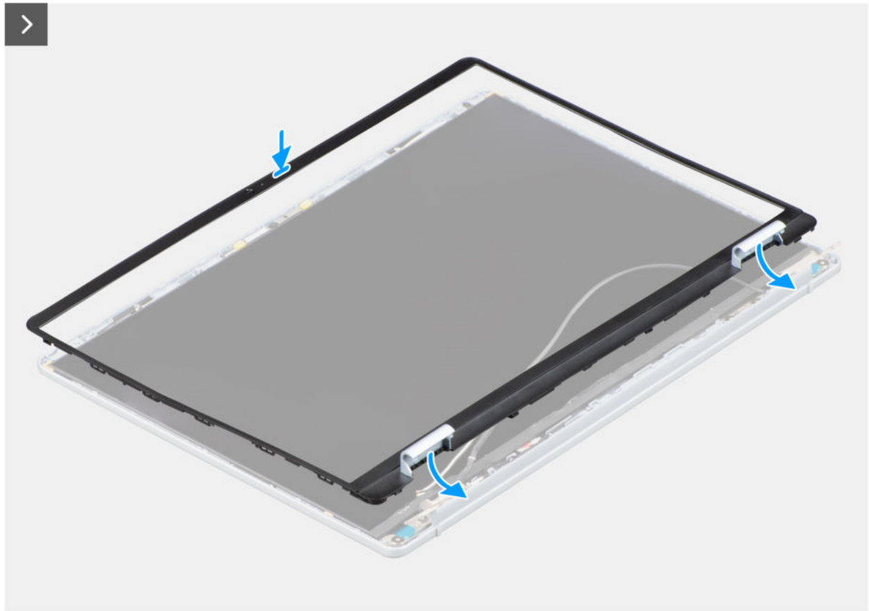
Abbildung 59. Einbauen der Bildschirmblende
