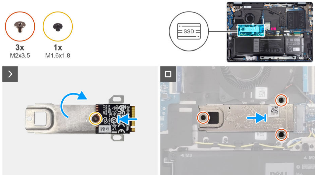
Abbildung 29. Installieren des Solid-State-Laufwerks
