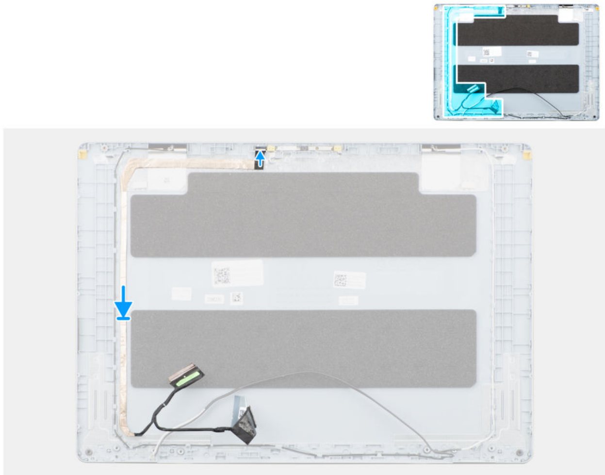
Abbildung 67. Einbauen des Bildschirmkabels
