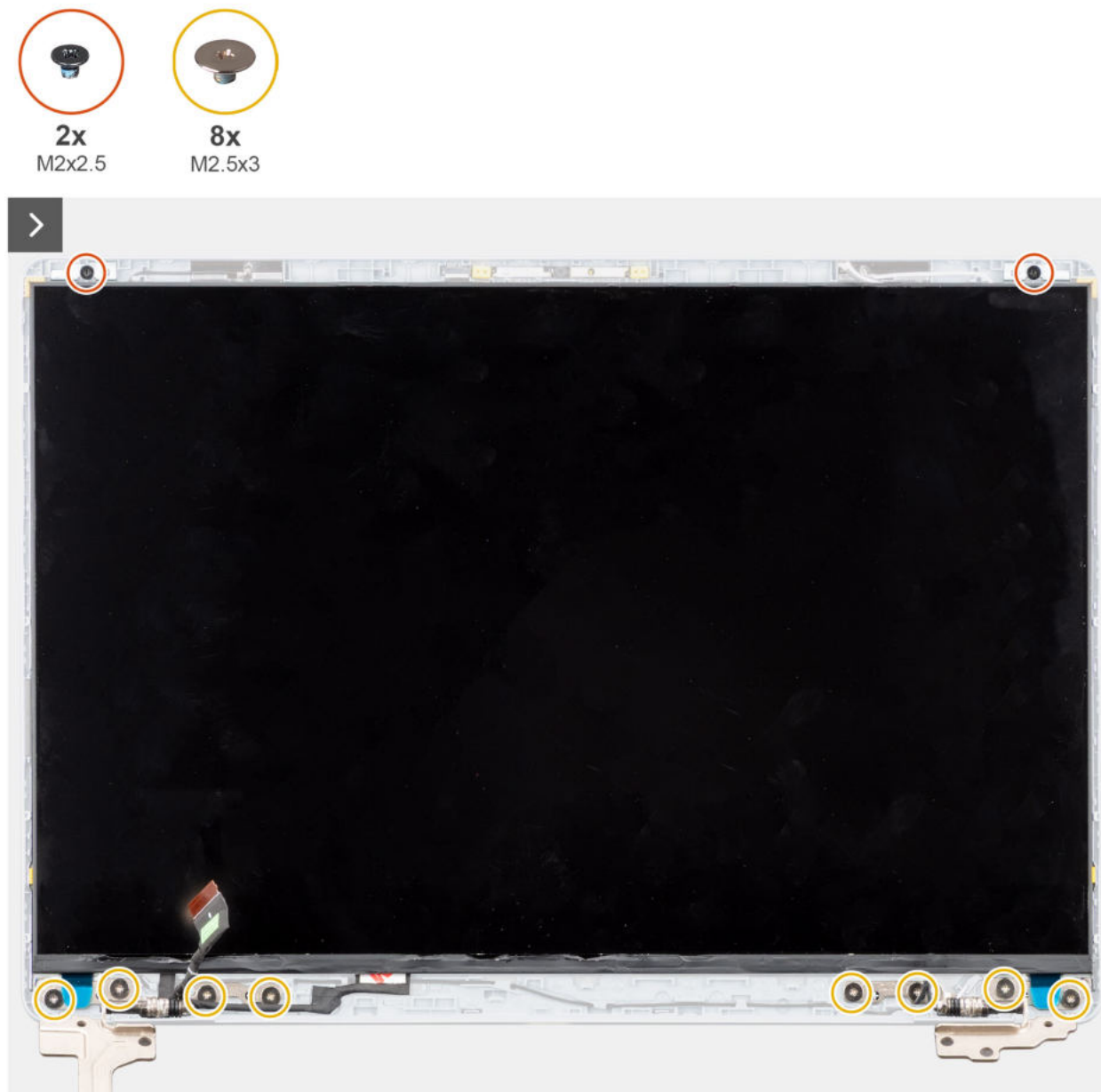
Abbildung 61. Entfernen des Bildschirms
