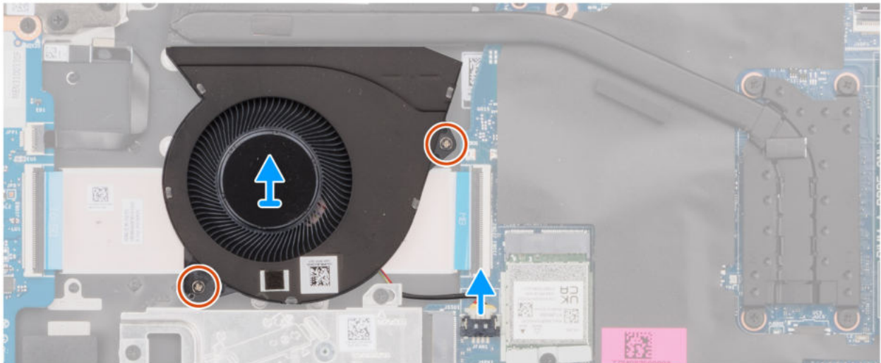
Abbildung 38. Entfernen des Lüfters
