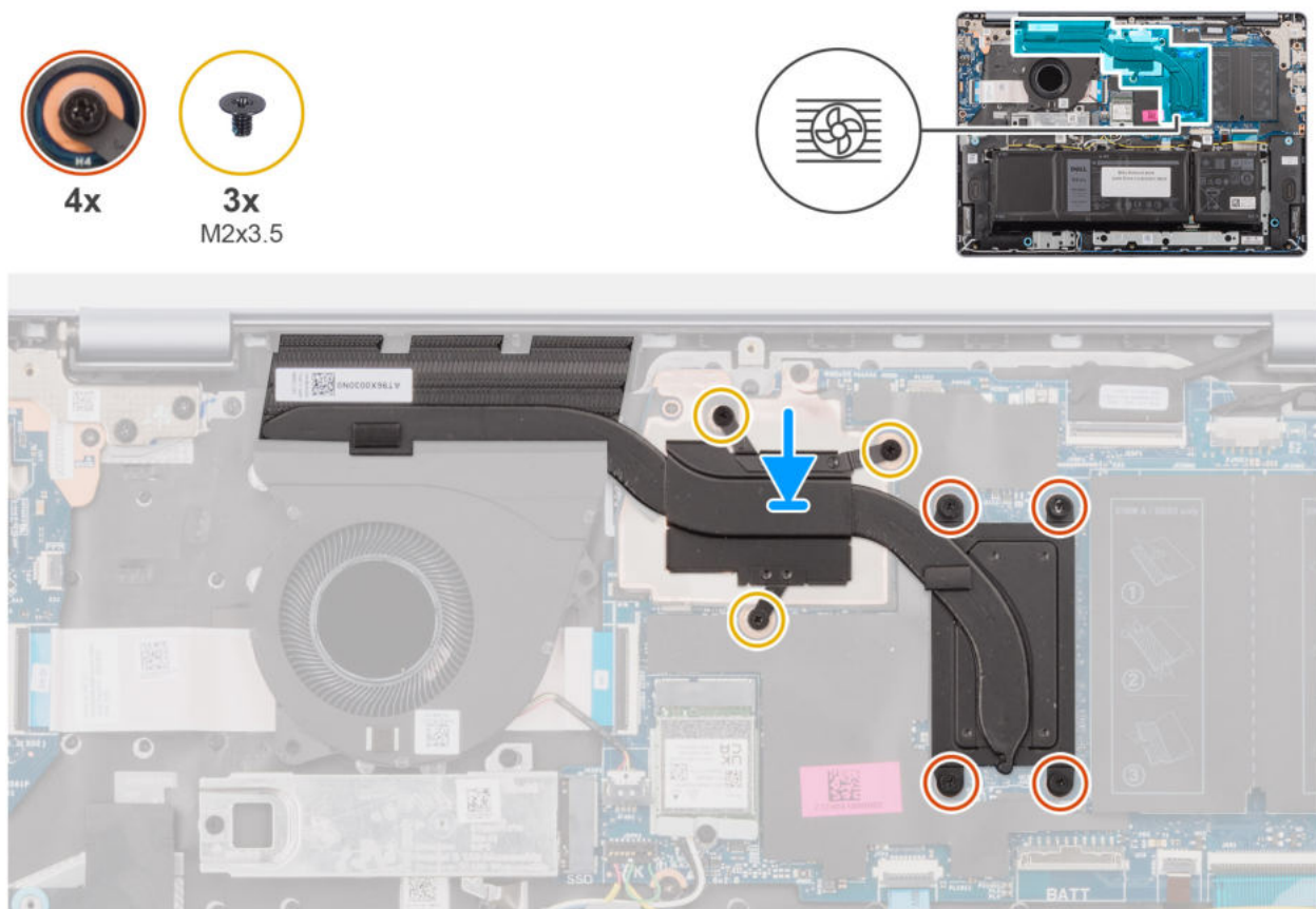
Abbildung 43. Einbauen des Kühlkörpers (bei Computern mit separater Grafikkarte)
