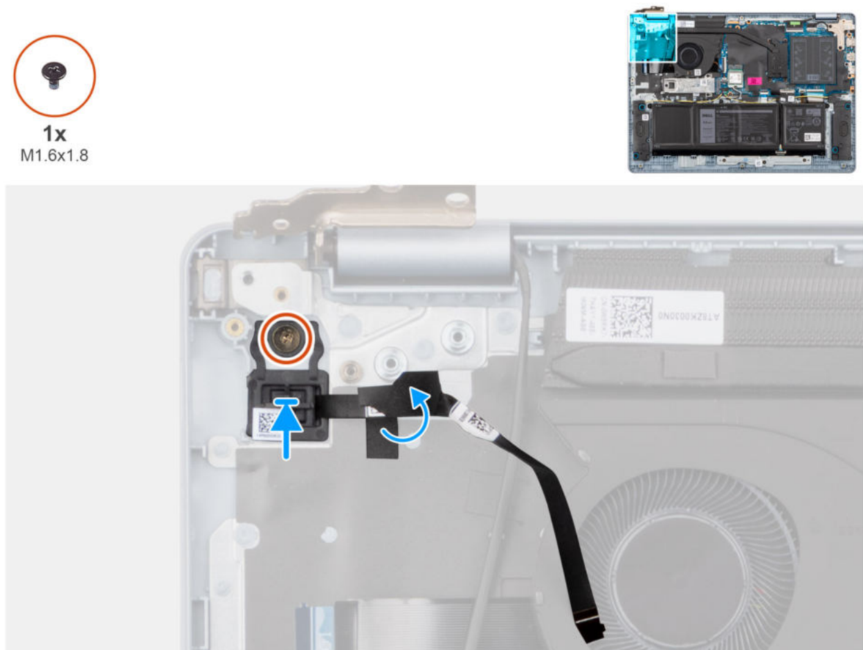
Abbildung 75. Einbauen des Netzschalters mit Fingerabdruck-Lesegerät
