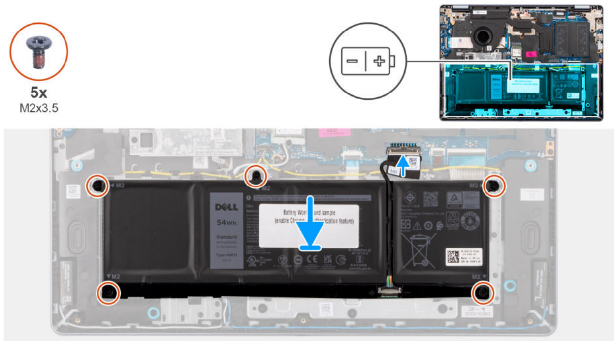
Abbildung 20. Installieren des 4-Zellen-Akkus
