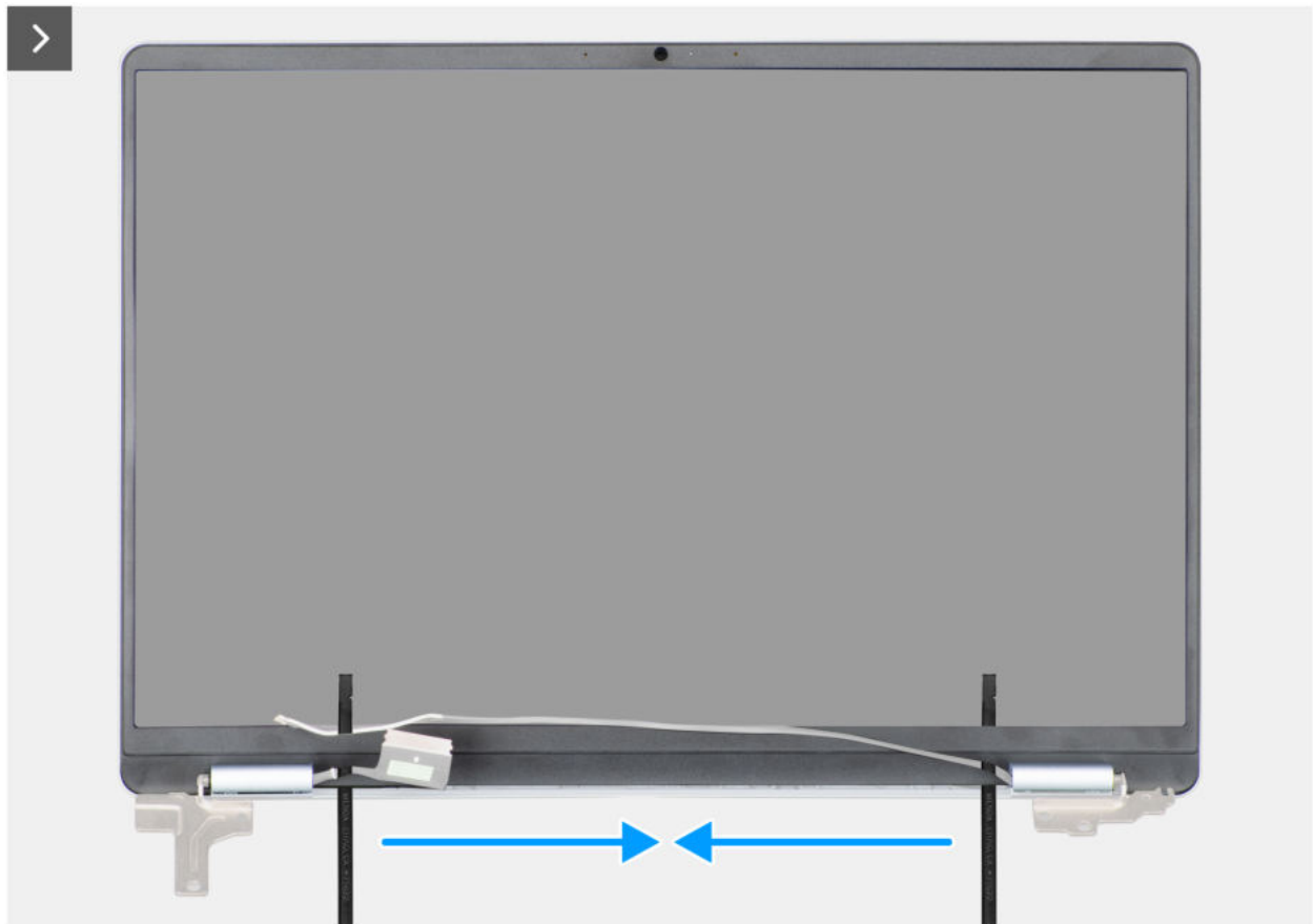
Abbildung 55. Entfernen der Bildschirmblende
