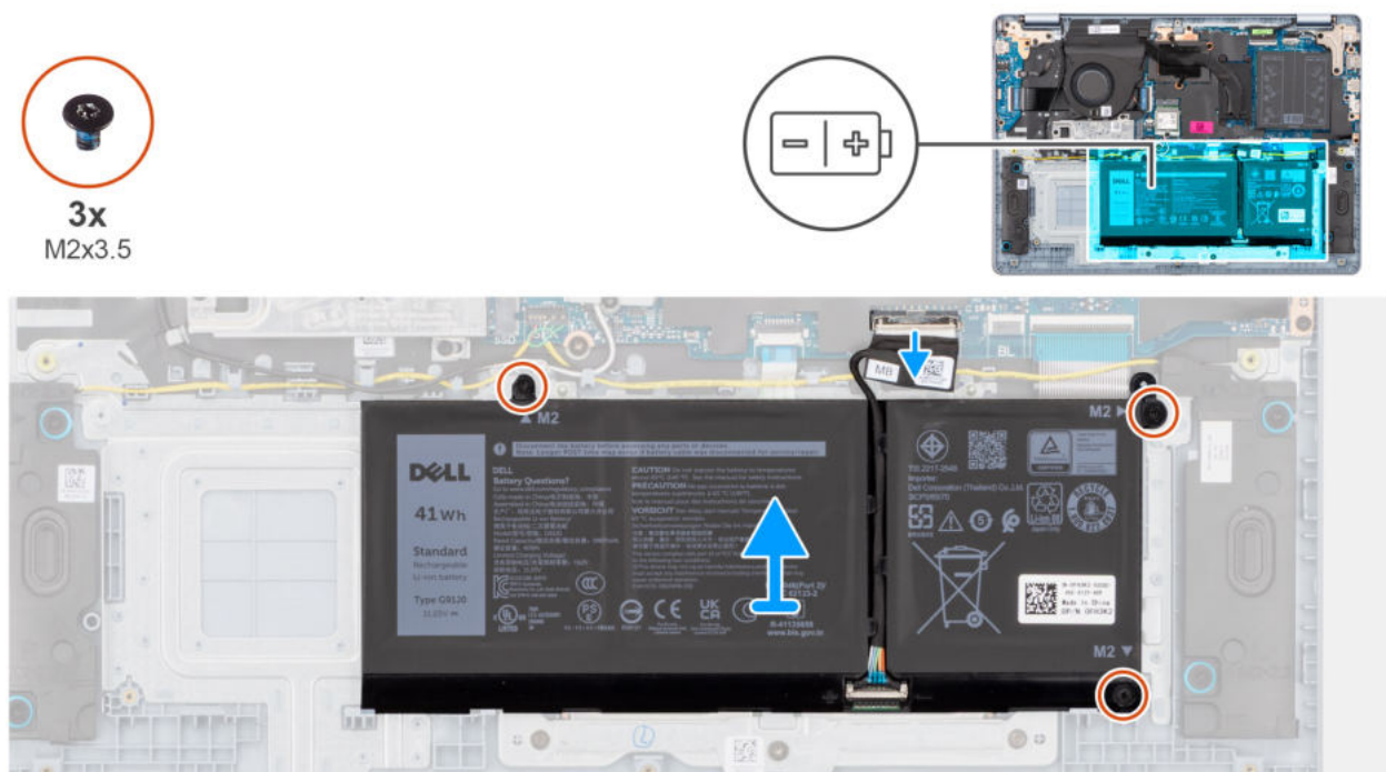
Abbildung 16. Entfernen des 3-Zellen-Akkus
