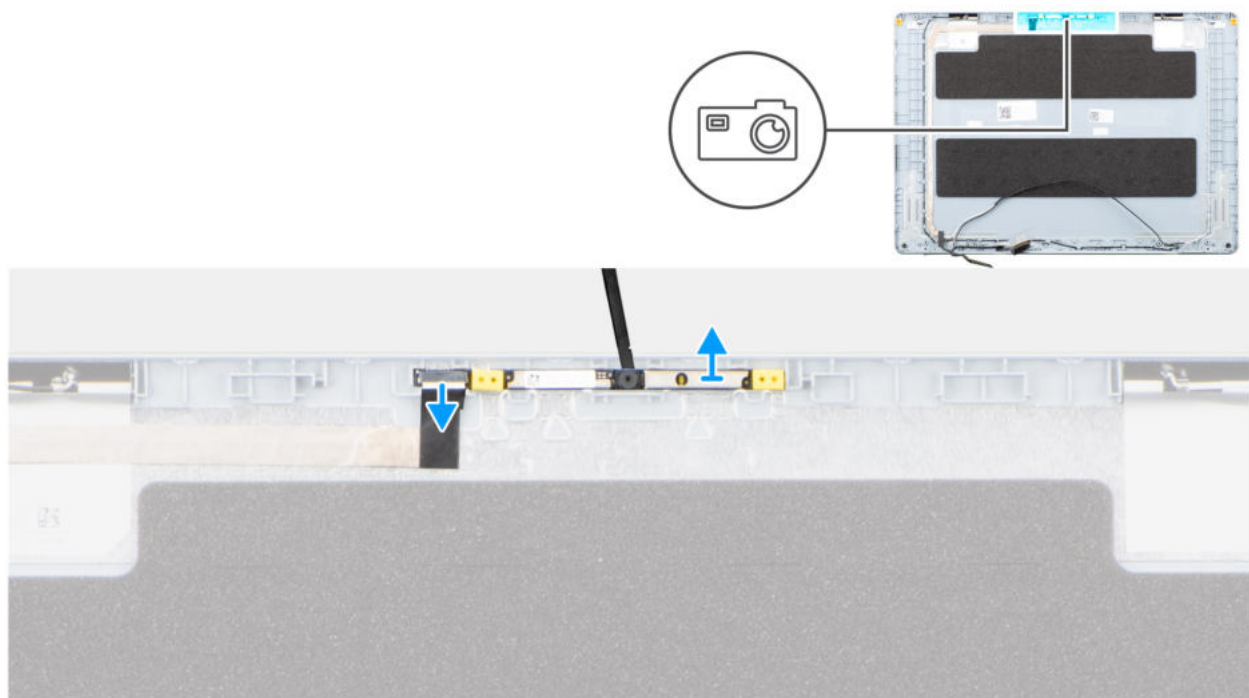
Abbildung 68. Entfernen der Kamera
