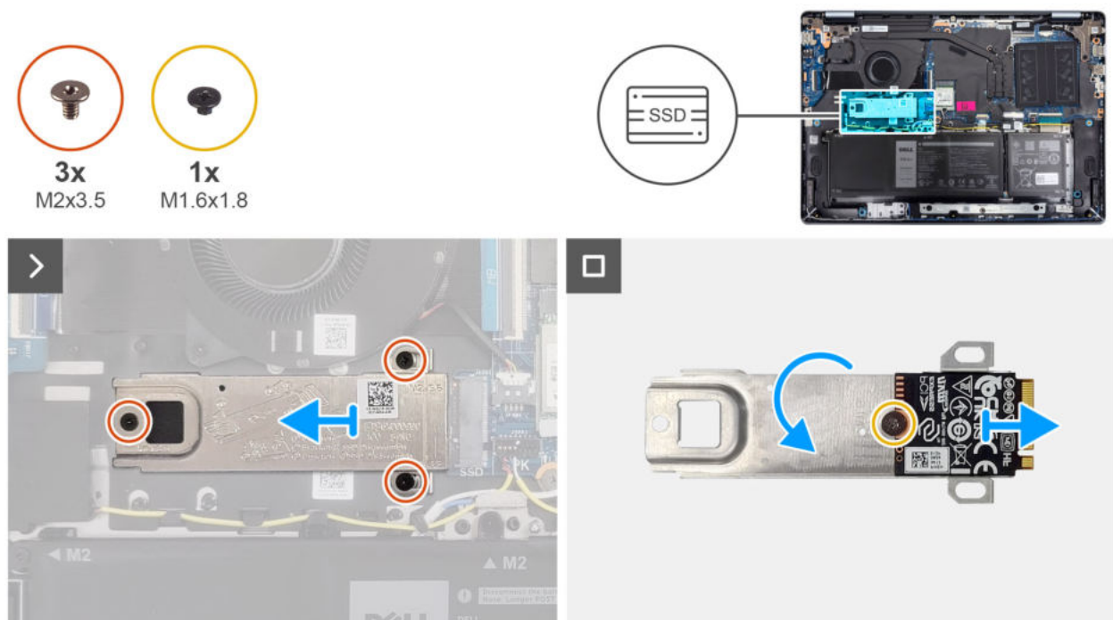
Abbildung 28. Entfernen der Solid-State-Festplatte
