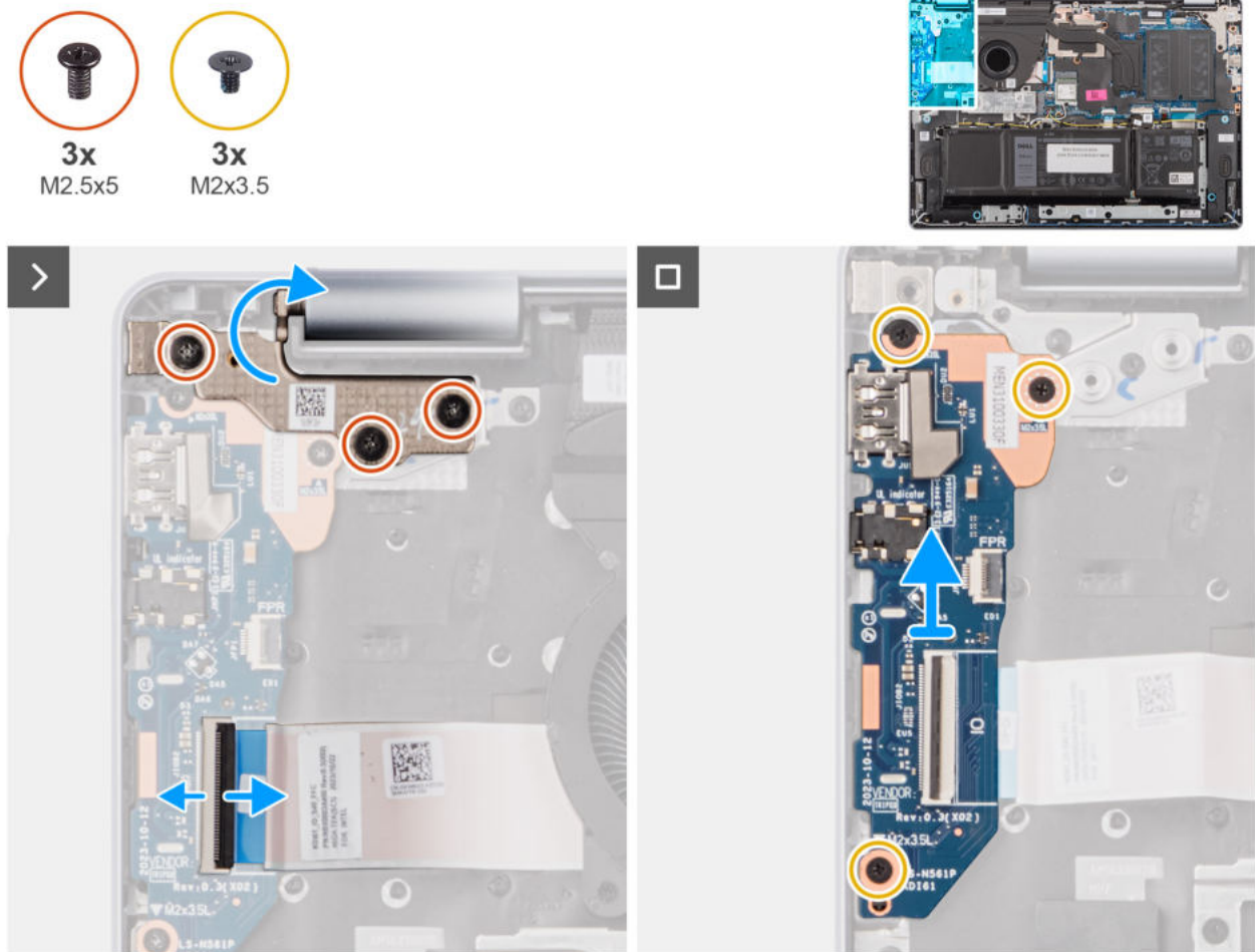
Abbildung 48. Entfernen der E/A-Platine
