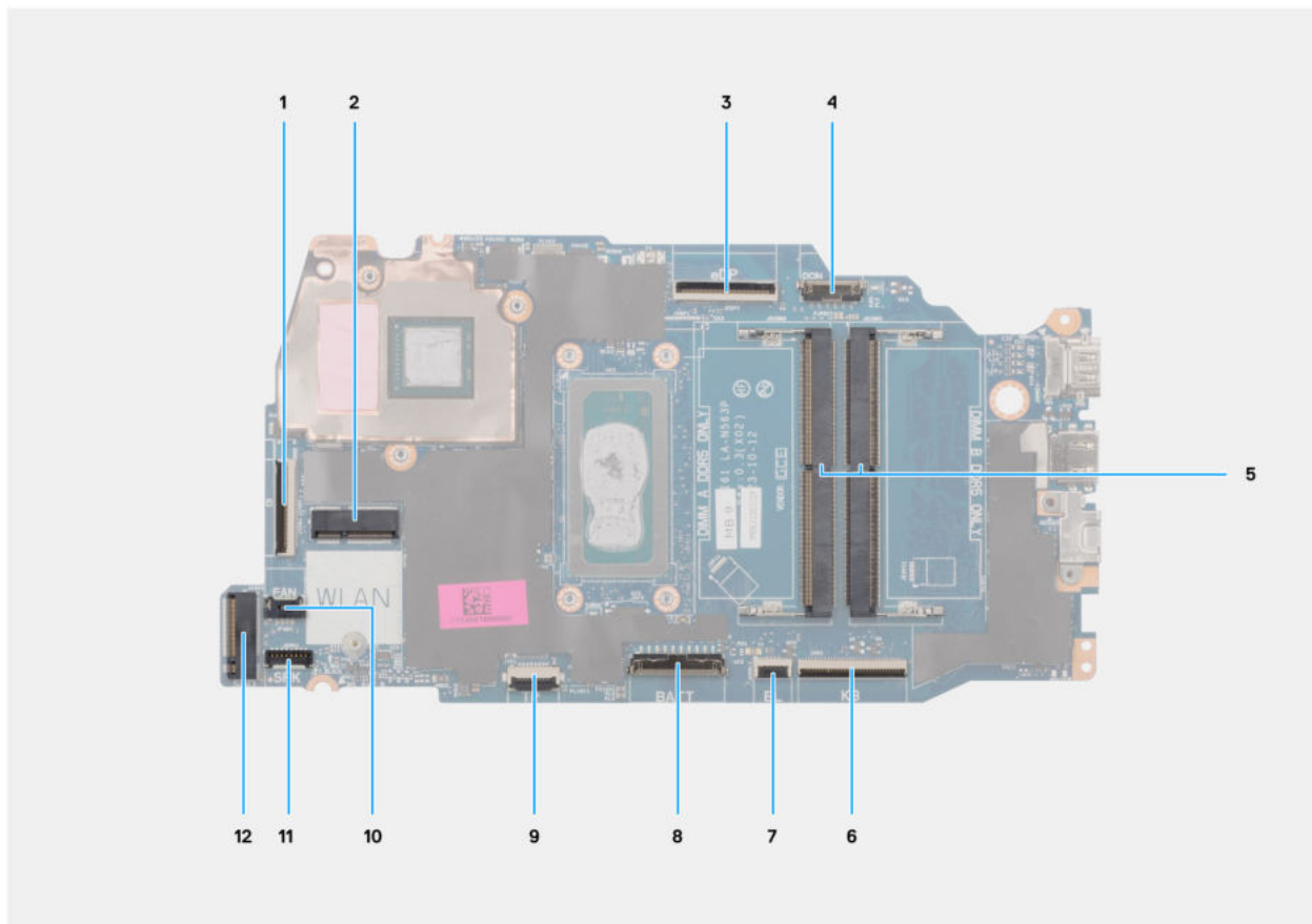
Abbildung 84. Anschlüsse auf der Hauptplatine
