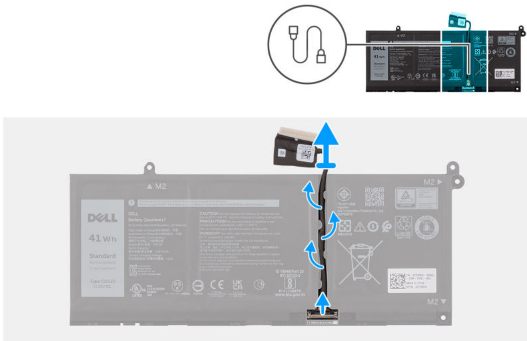
Abbildung 22. Trennen des Akkukabels
