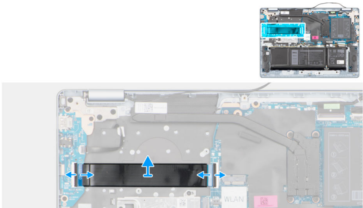
Abbildung 46. Entfernen des I/O-Platinenkabels
