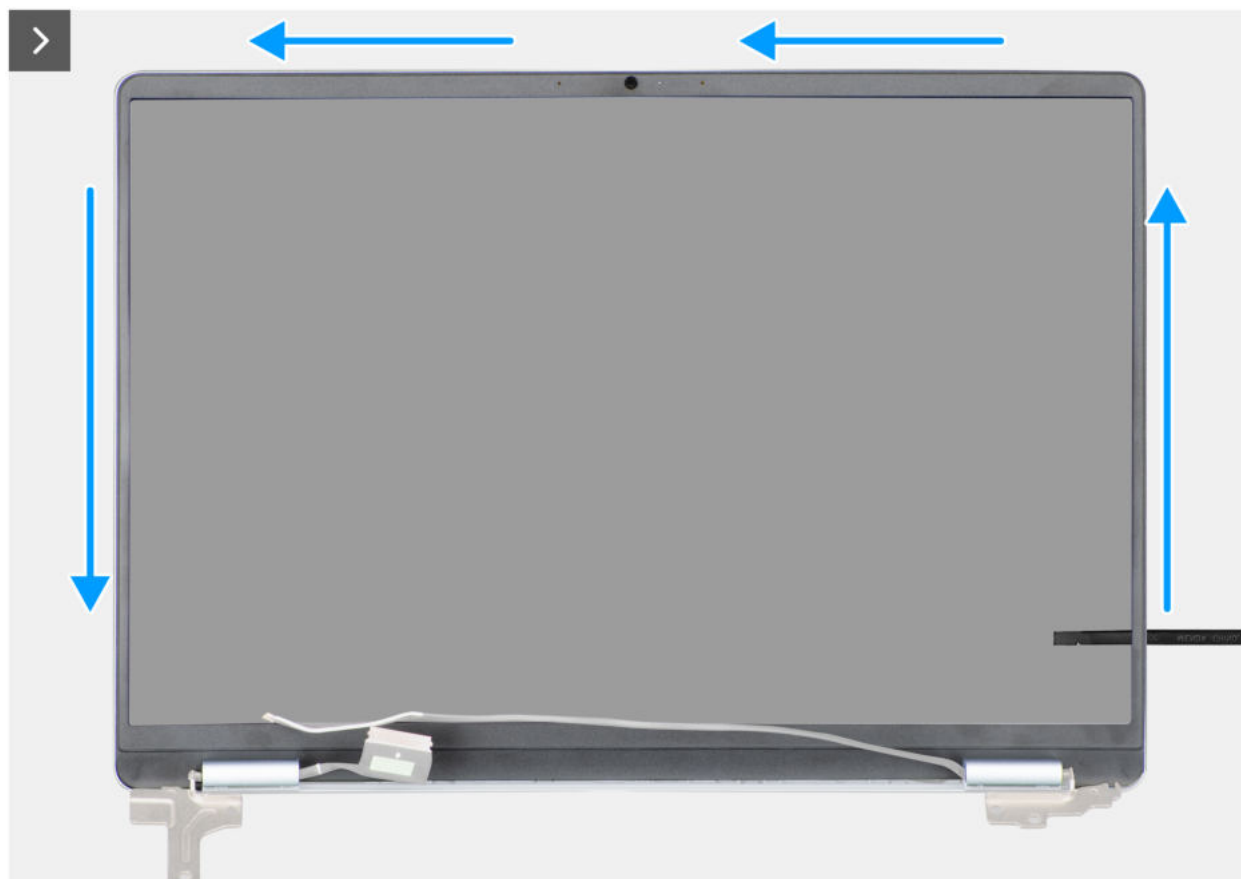
Abbildung 57. Entfernen der Bildschirmblende
