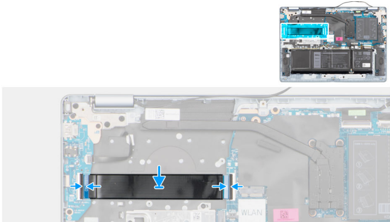
Abbildung 47. Installieren des I/O-Platinenkabels
