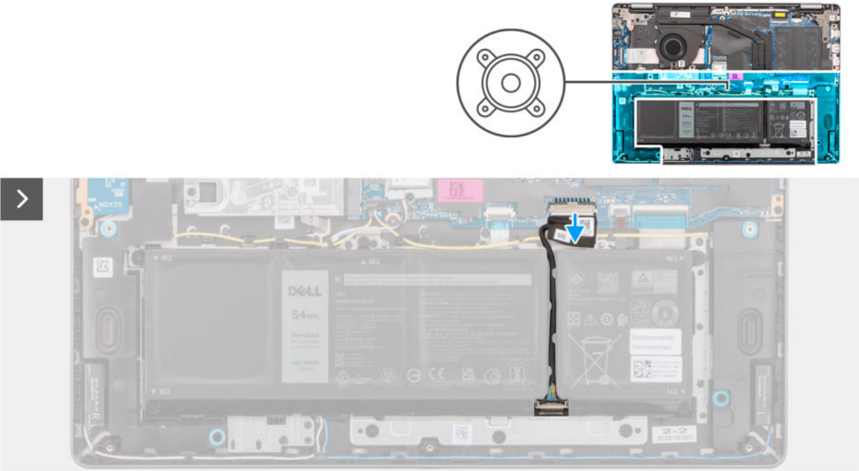
Abbildung 32. Trennen des Akkukabels
