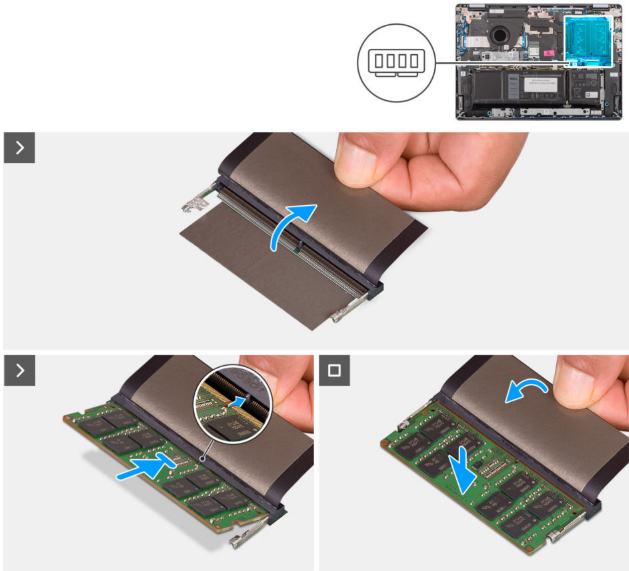
Abbildung 27. Einsetzen des Speichermoduls
