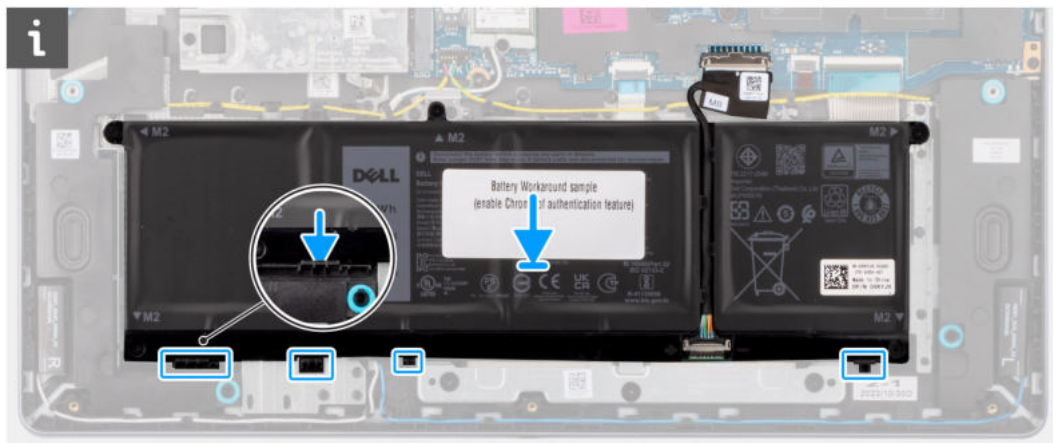
Abbildung 21. Einsetzen des Akkus – Einführen der Laschen in die Haken
