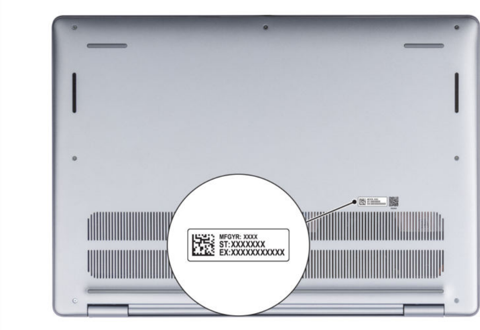
Abbildung 7. Position des Service-Tags/Express-Servicecodes
