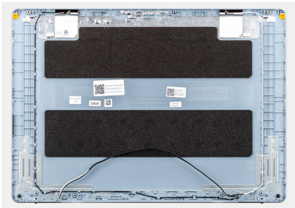
Abbildung 71. Bildschirmrückwand-Antennen-Baugruppe
