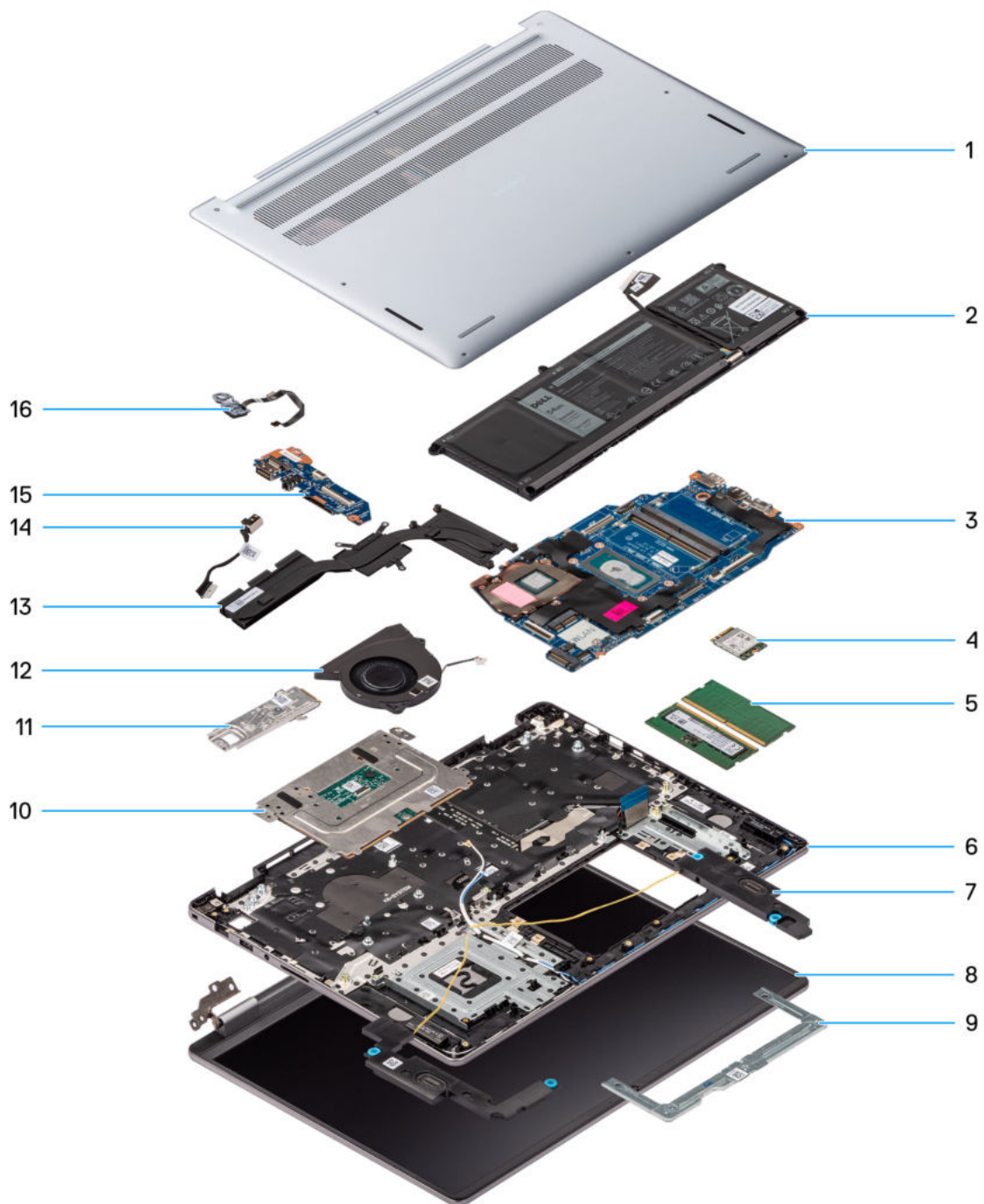
Abbildung 11. Hauptkomponenten des Dell 16 DC16250
