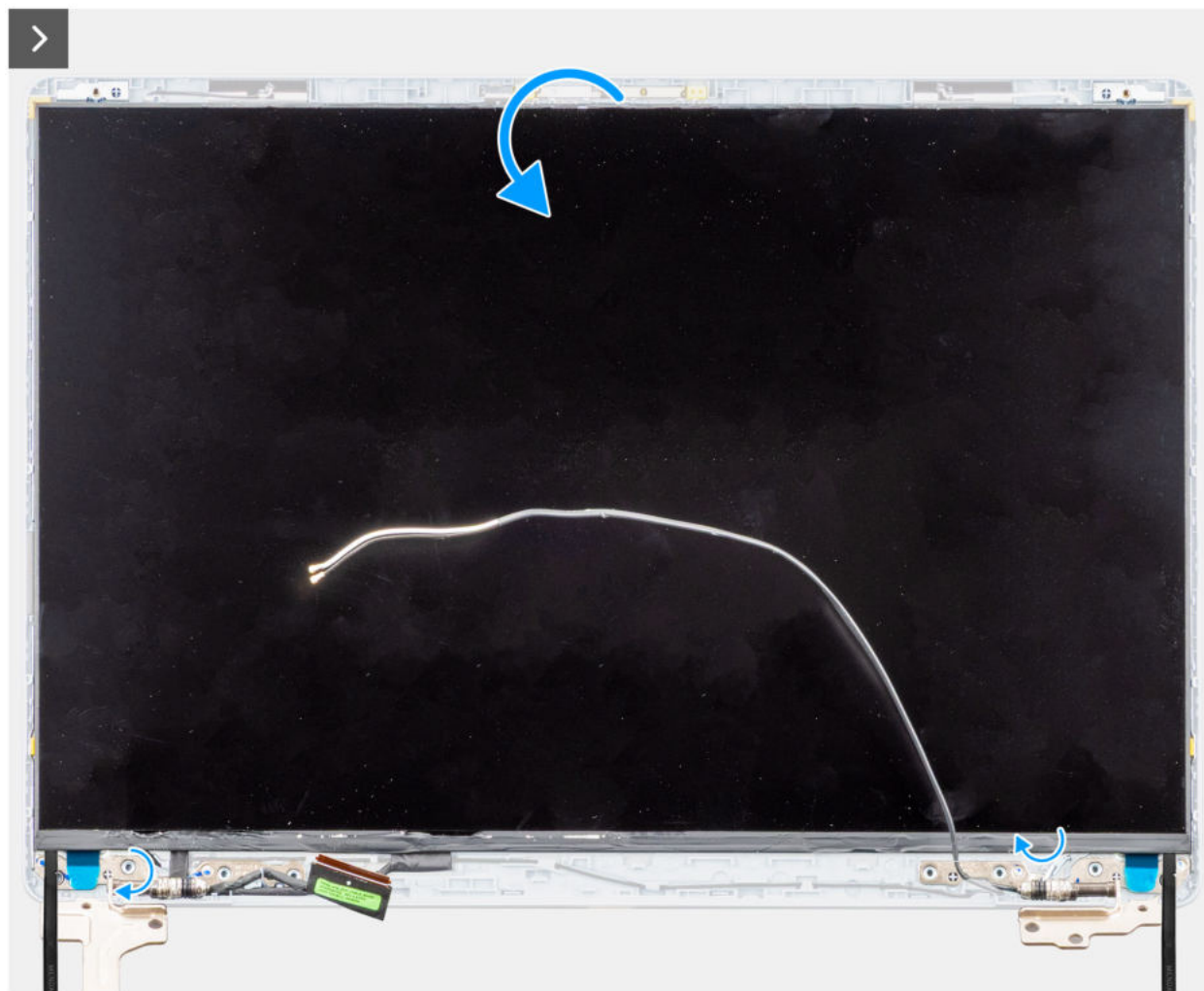
Abbildung 62. Entfernen des Bildschirms
