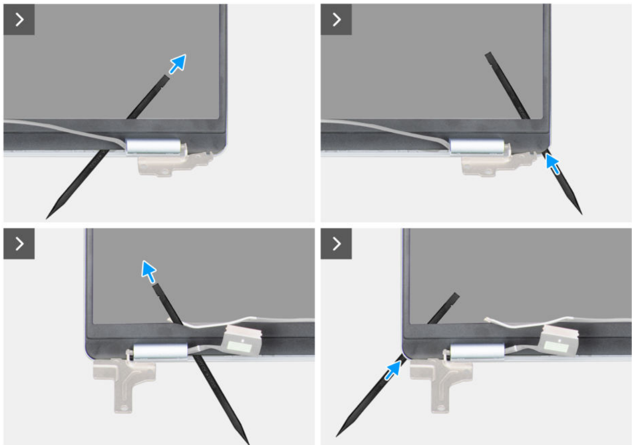
Abbildung 56. Entfernen der Bildschirmblende
