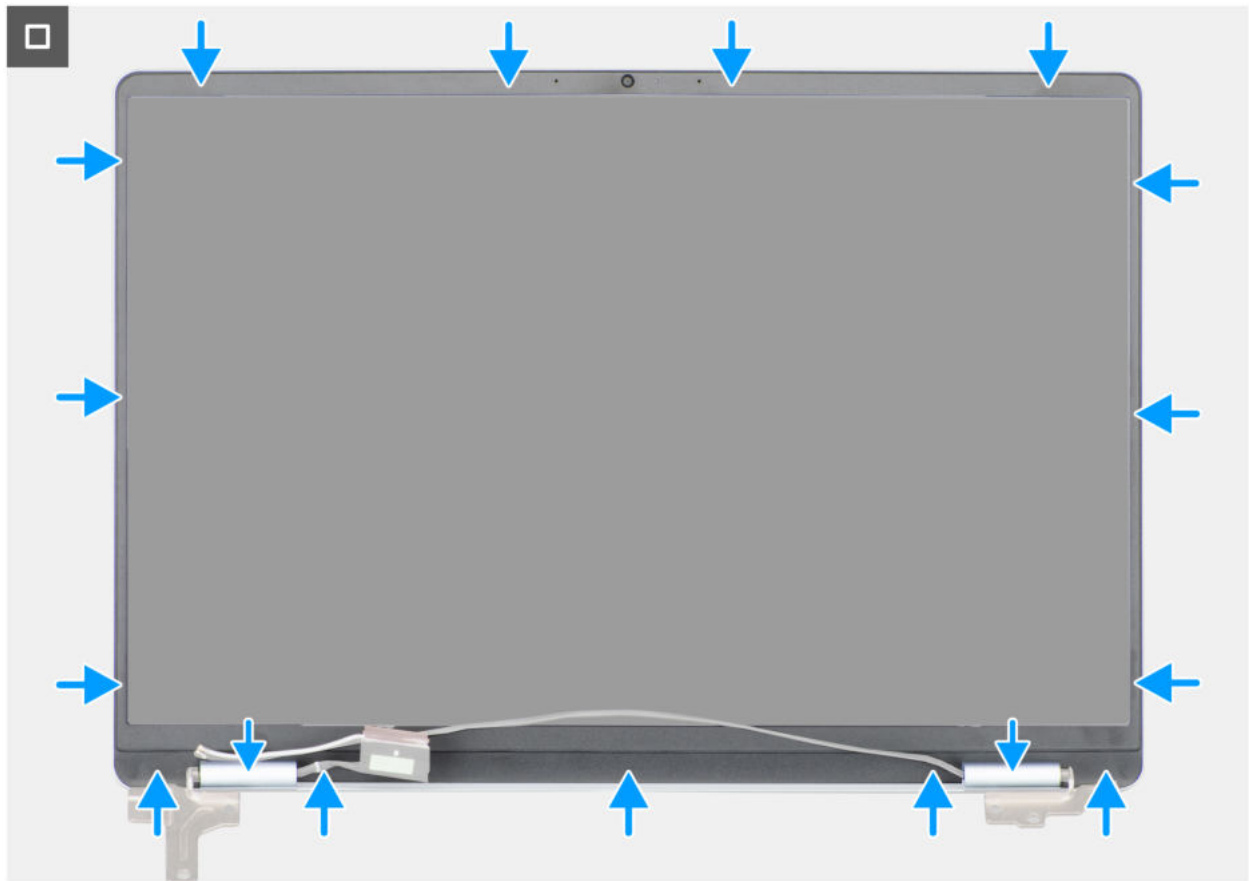
Abbildung 60. Einbauen der Bildschirmblende
