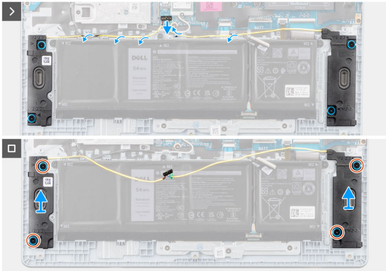
Abbildung 33. Entfernen der Lautsprecher
