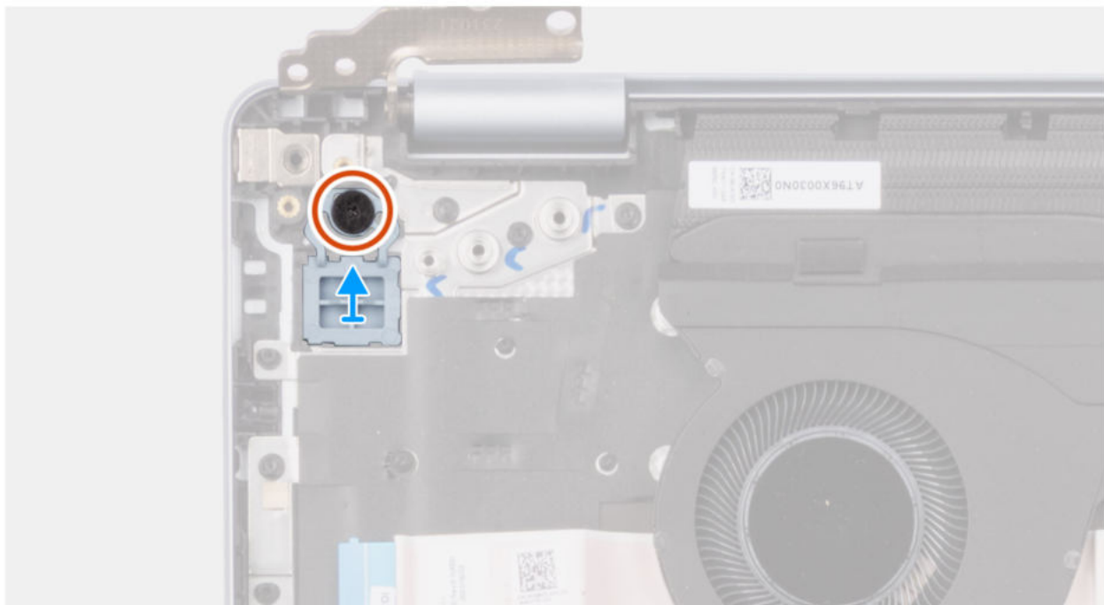
Abbildung 72. Entfernen des Netzschalters
