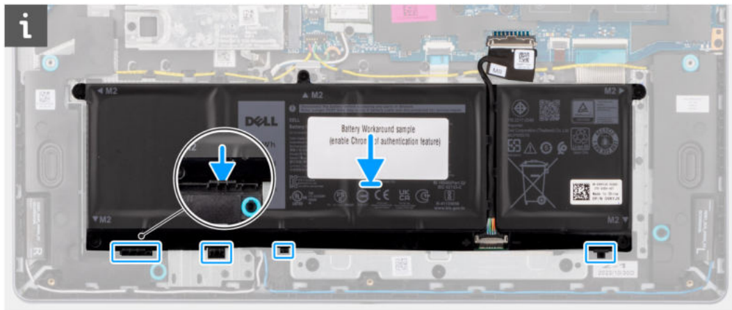
Abbildung 18. Einsetzen des Akkus – Einführen der Laschen in die Haken
