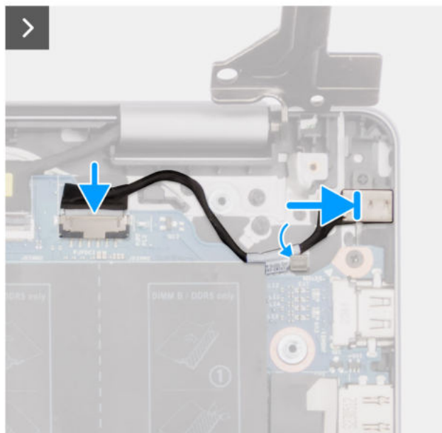
Abbildung 78. Einbauen des Netzadapteranschlusses
