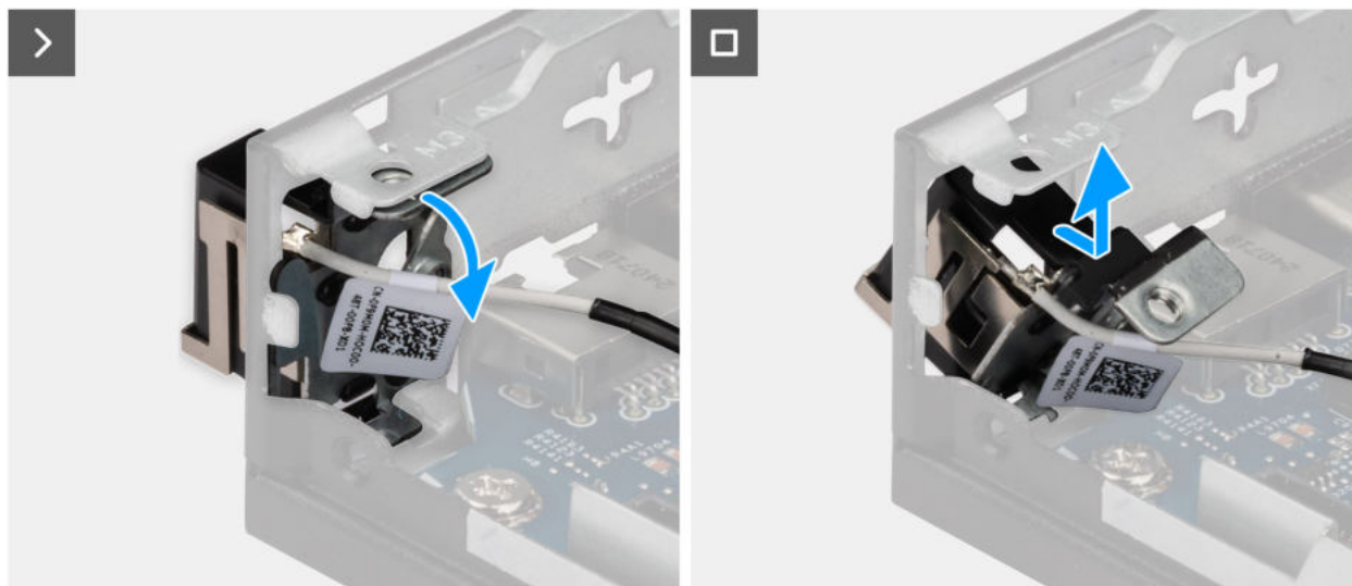
Abbildung 67. Entfernen des Antennenmoduls (weißes Kabel)
