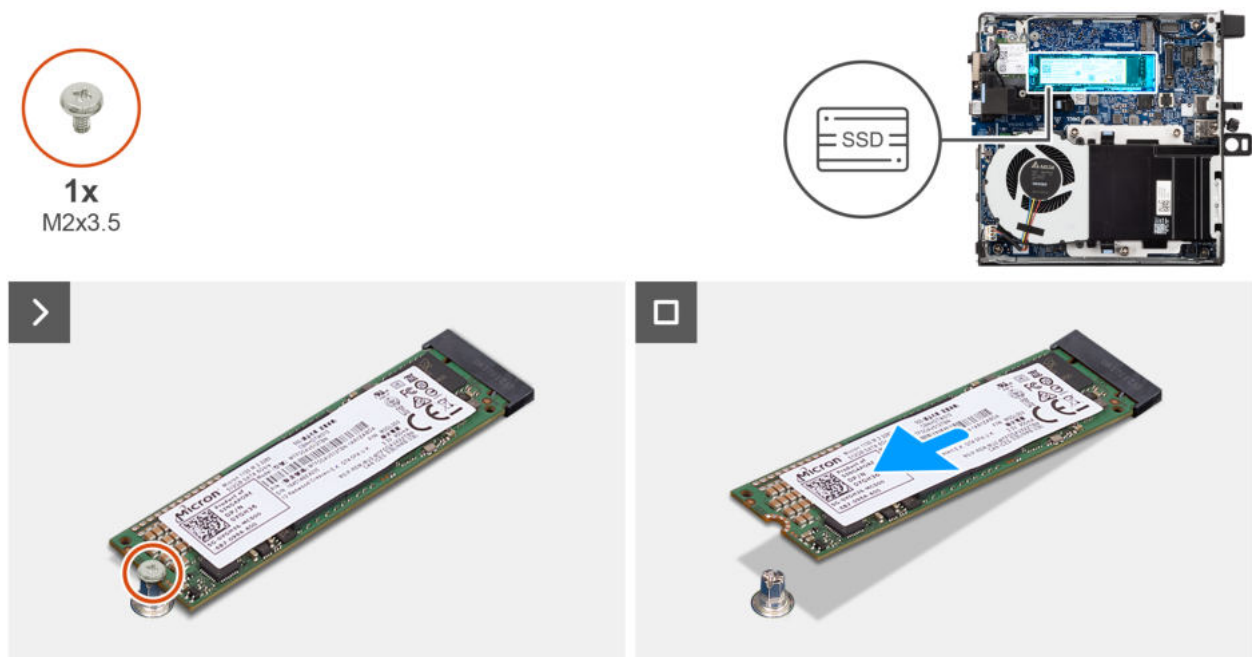
Abbildung 19. Entfernen des M.2-2280-Solid-State-Laufwerks
