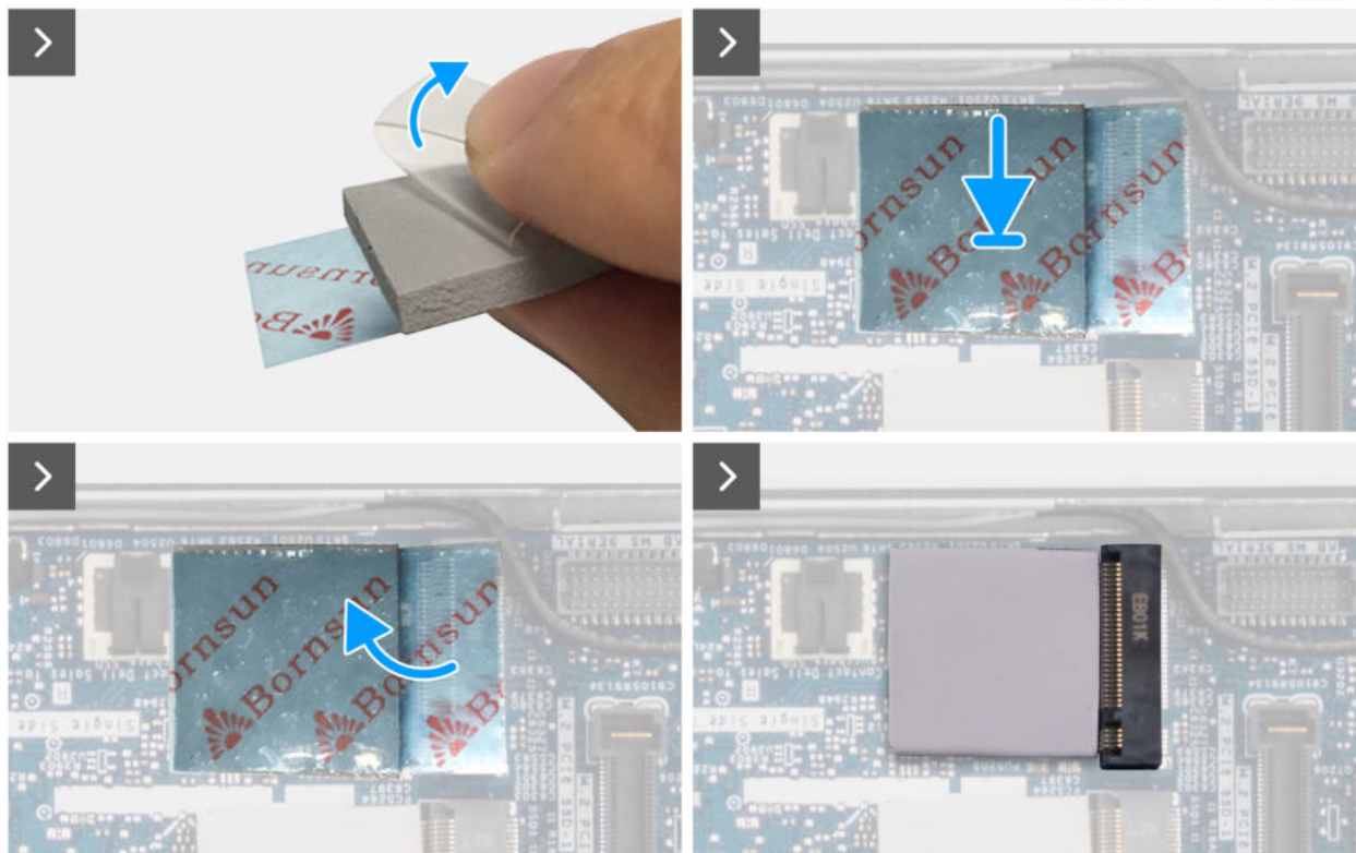
Abbildung 20. Einbauen des M.2-2280-Solid-State-Laufwerks
