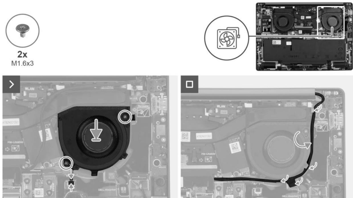
Abbildung 29. Installieren des linken Lüfters
