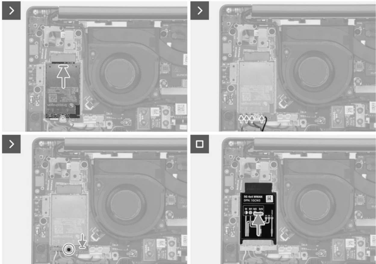
Abbildung 27. Einbauen der WWAN-Karte
