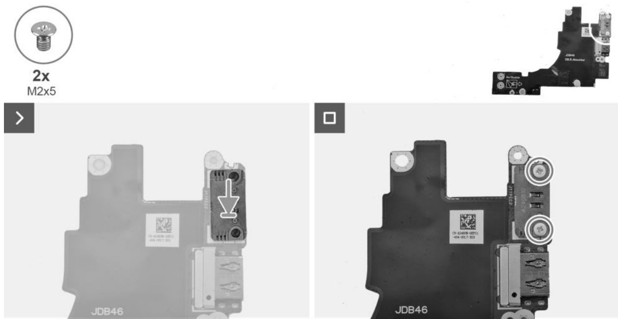
Abbildung 51. Installieren des linken USB Typ-C-Moduls
