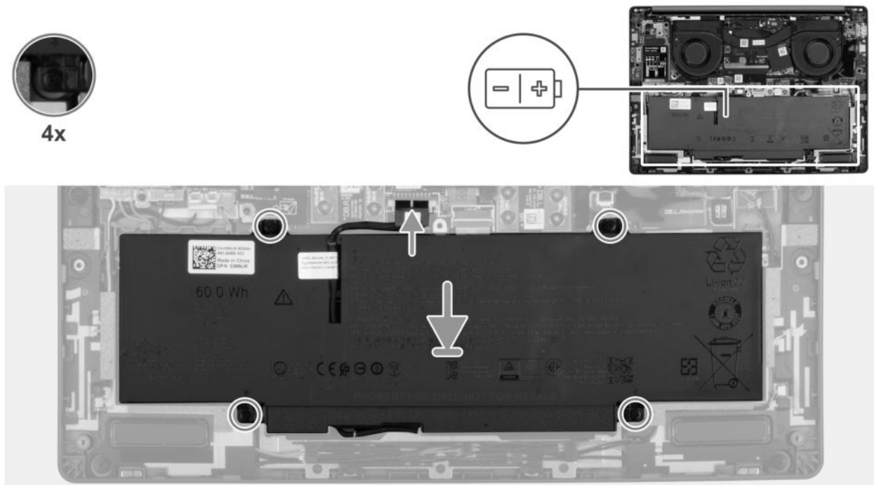
Abbildung 21. Einsetzen des Akkus
