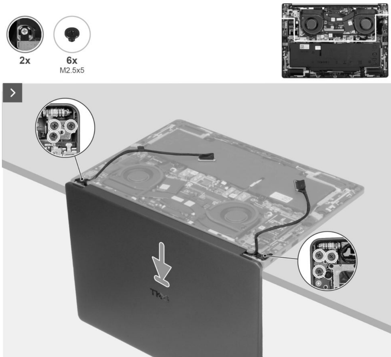
Abbildung 59. Einbauen der Displaybaugruppe
