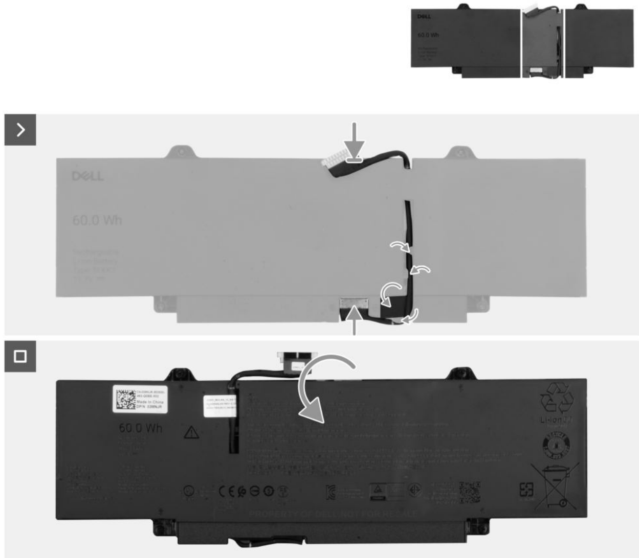
Abbildung 23. Anschließen und Installieren des Akkukabels
