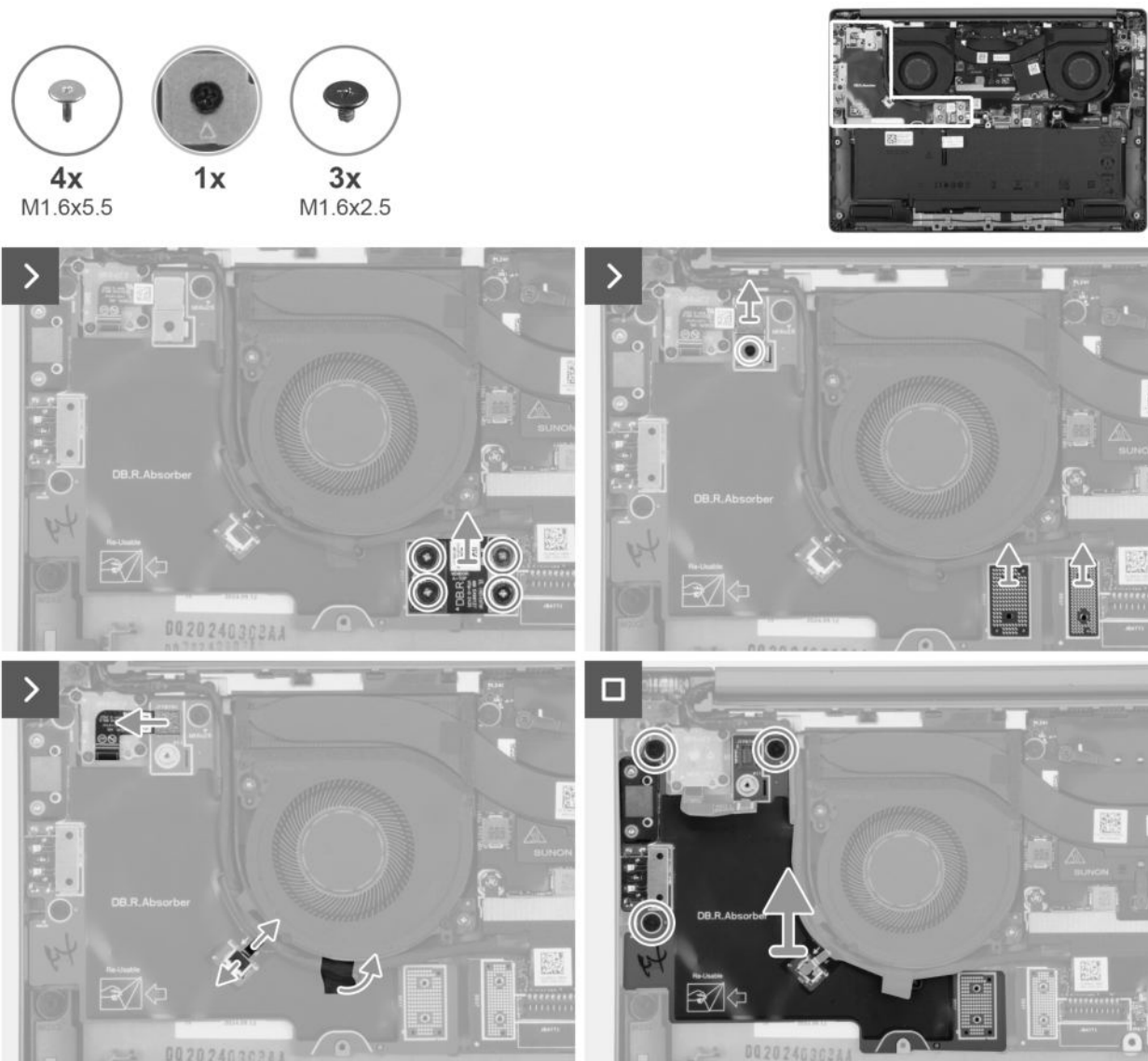
Abbildung 42. Entfernen der rechten I/O-Platine (ohne WWAN-Antennen)
