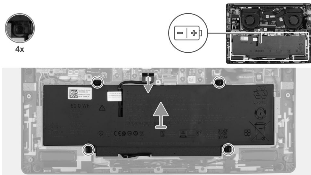
Abbildung 20. Lösen der unverlierbaren Schrauben
