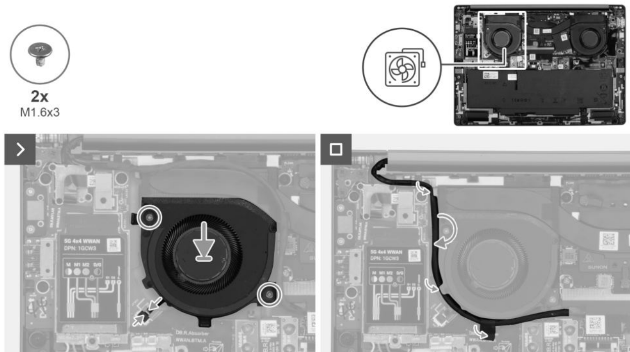
Abbildung 31. Installieren des rechten Lüfters
