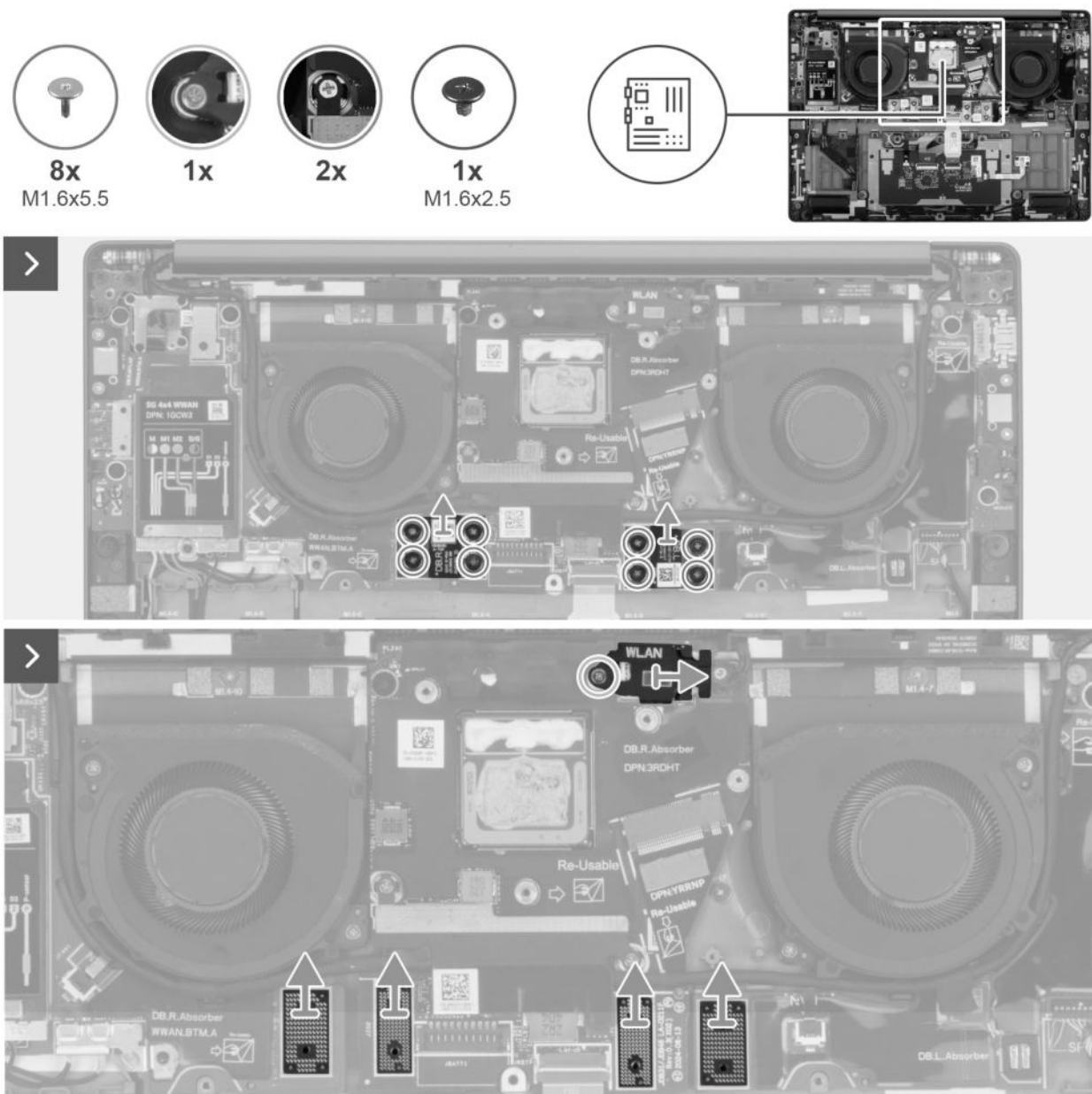
Abbildung 62. Entfernen der Systemplatte
