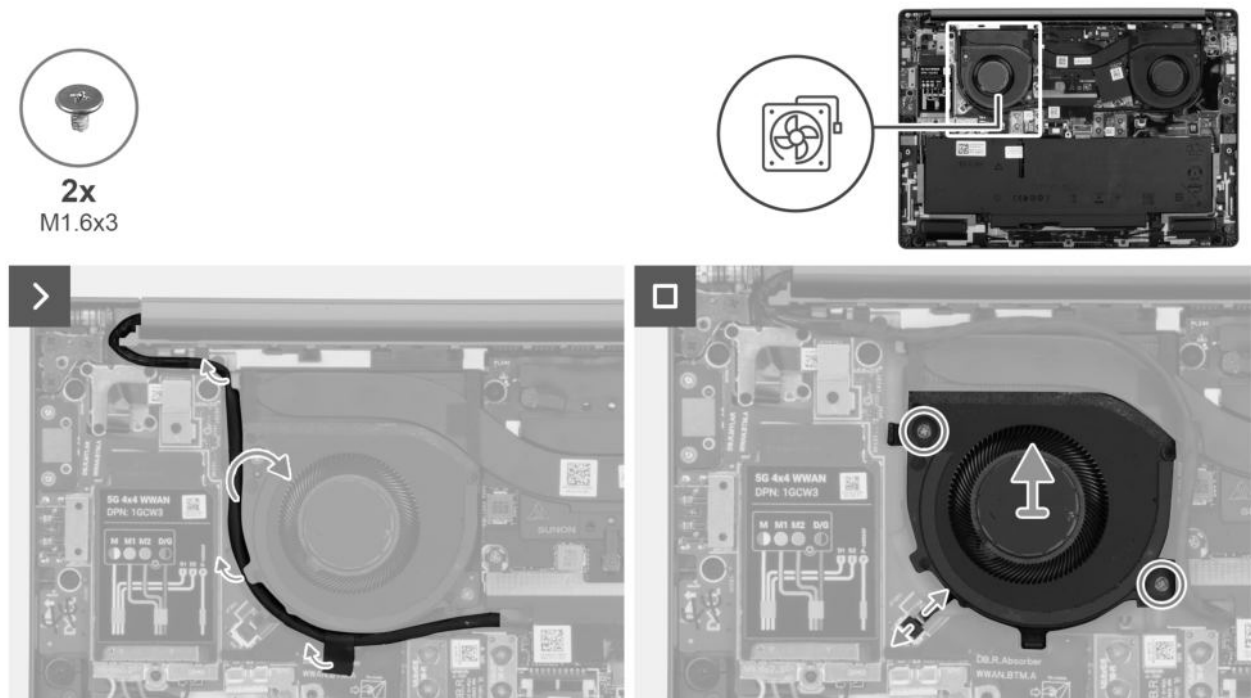
Abbildung 30. Entfernen des rechten Lüfters
