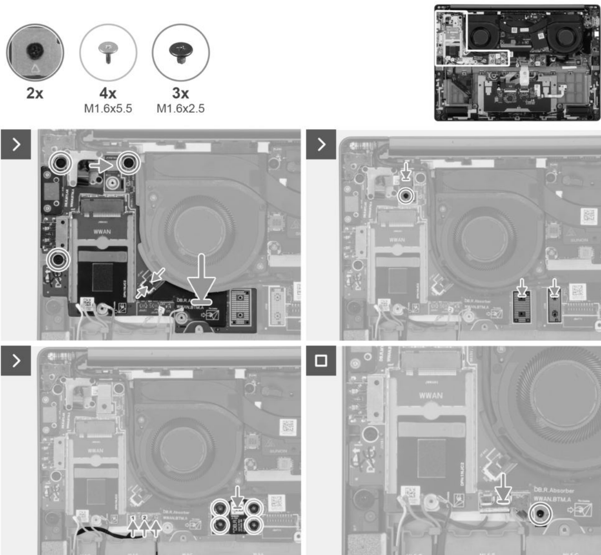
Abbildung 48. Installieren der rechten I/O-Platine (mit WWAN)
