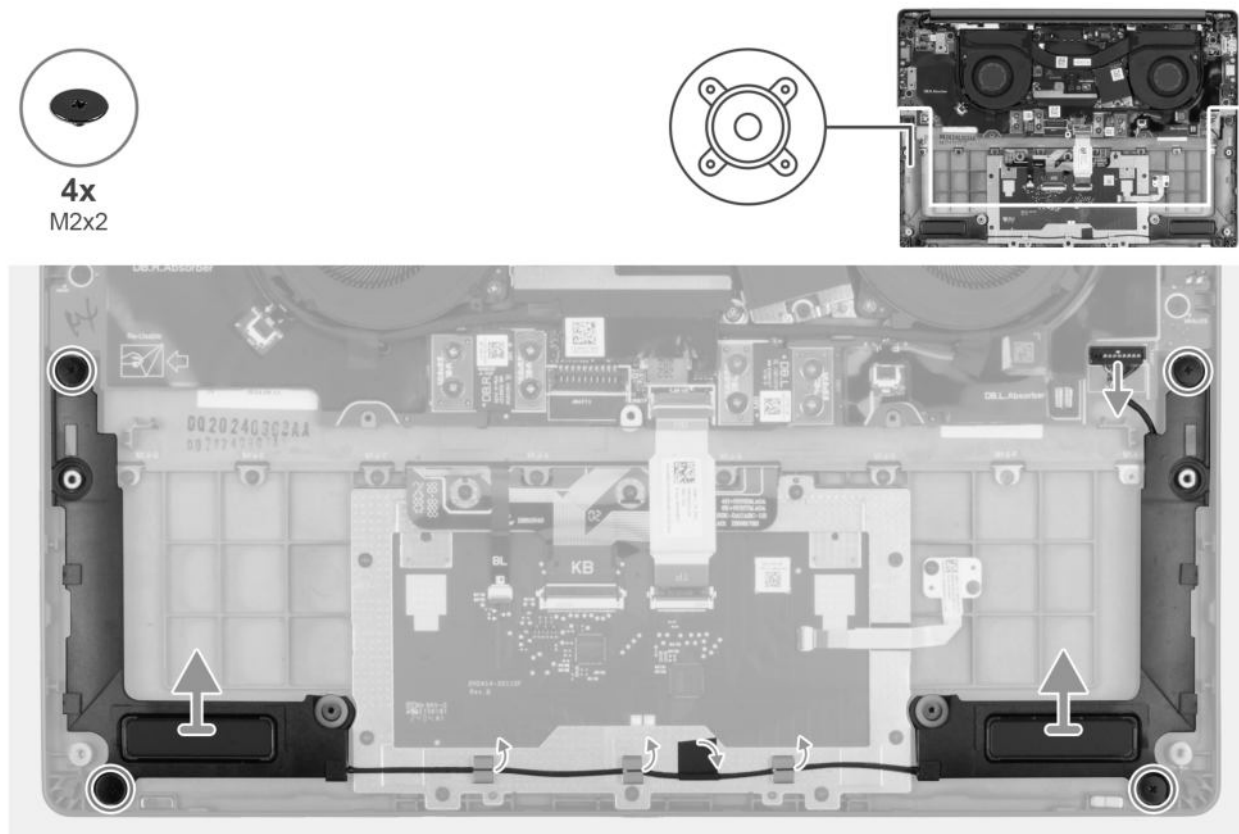
Abbildung 32. Entfernen der Lautsprecher ohne Antenne (WLAN-Konfiguration)
