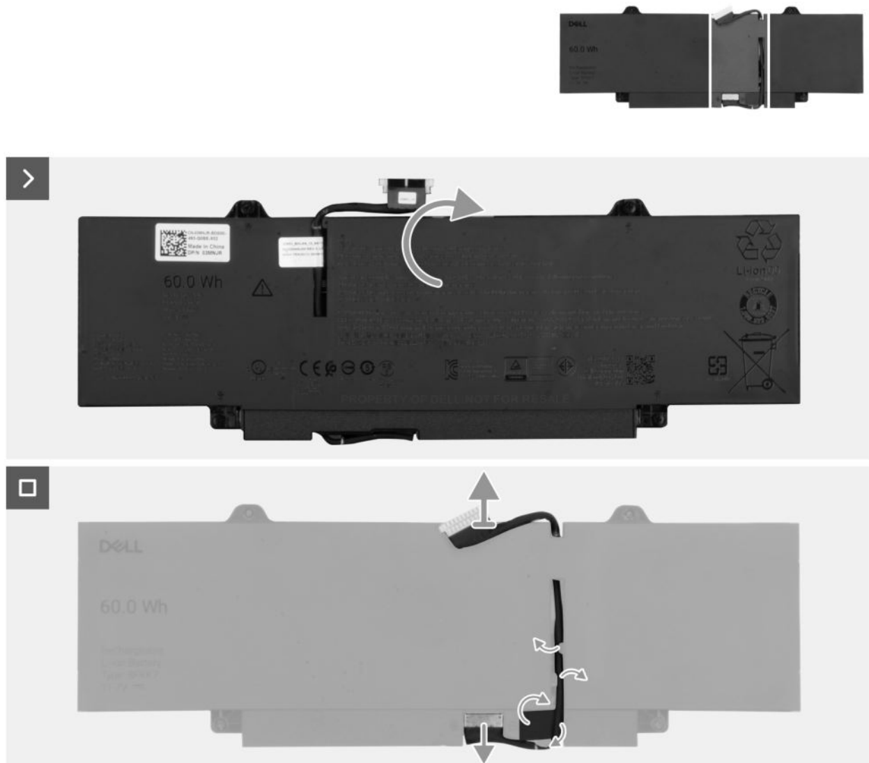
Abbildung 22. Entfernen und Trennen des Akkukabels
