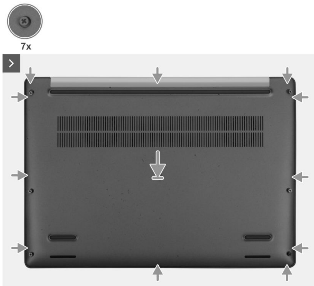
Abbildung 18. der Bodenabdeckung
