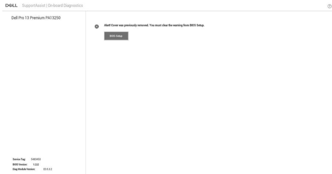
Abbildung 78. BIOS-Setup
