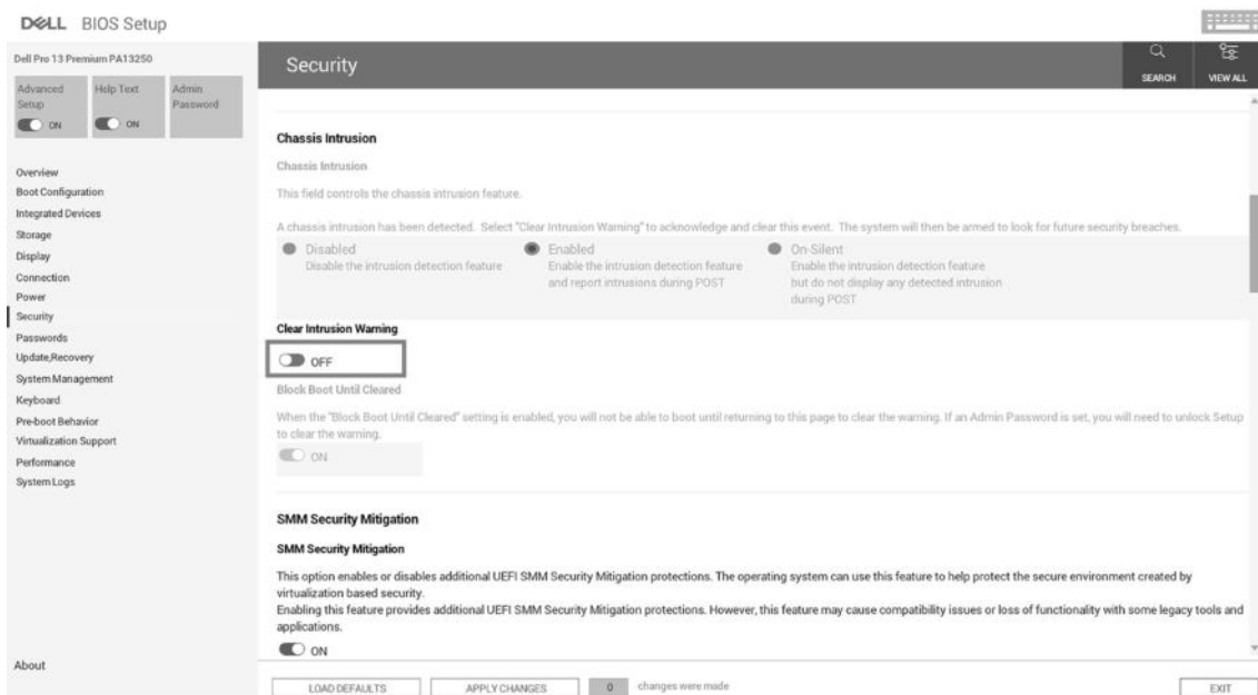
Abbildung 80. Gehäuseeingriffswarnung löschen
