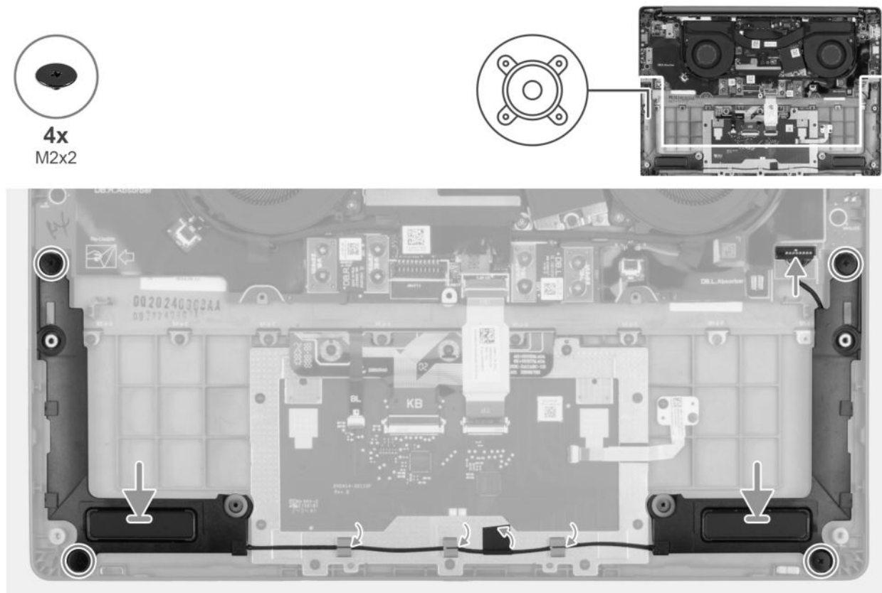
Abbildung 33. Installieren der Lautsprecher (ohne WWAN)
