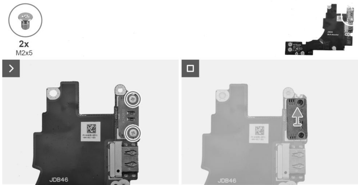
Abbildung 50. Entfernen des linken USB-Typ-C-Moduls
