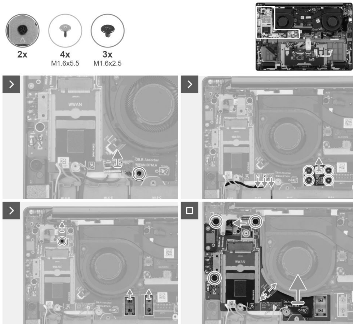
Abbildung 46. Entfernen der rechten I/O-Platine (mit WWAN)
