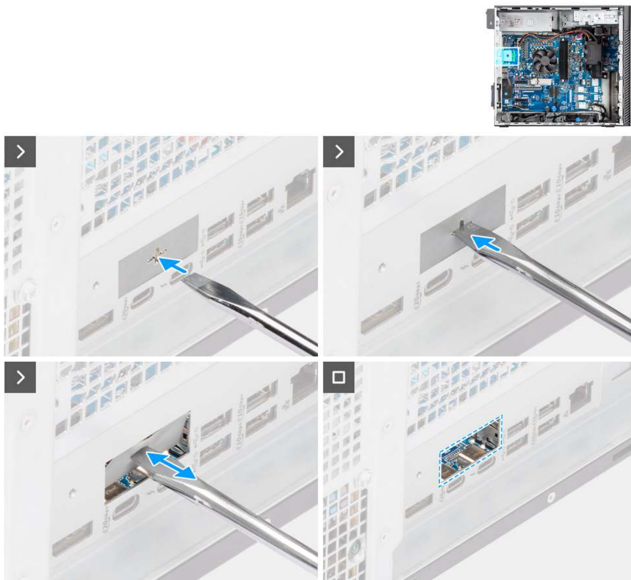
Afbeelding 68. De optionele DisplayPort-module installeren
