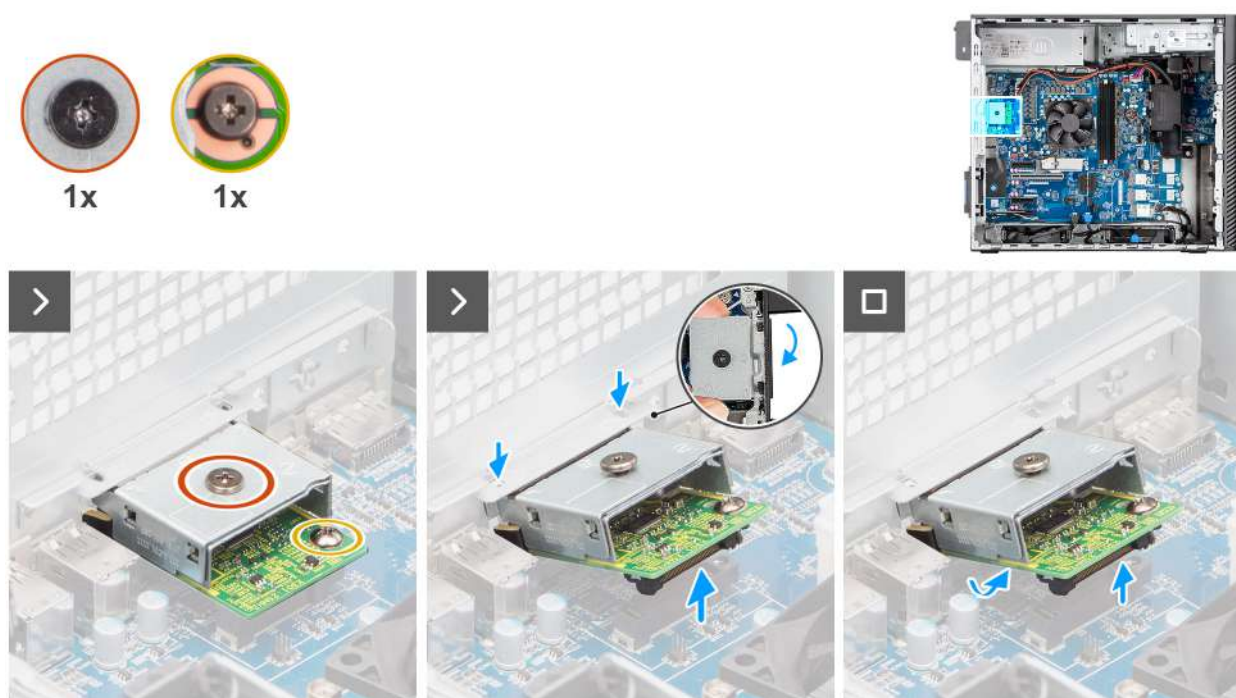
Afbeelding 67. De optionele DisplayPort-module verwijderen
