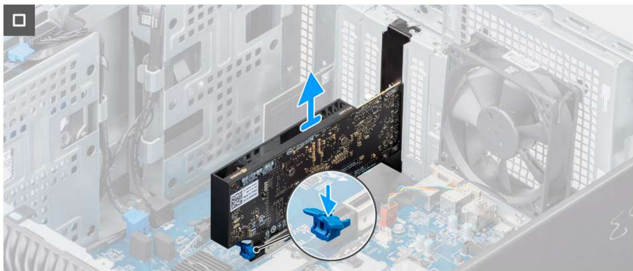
Afbeelding 37. De grafische kaart verwijderen
