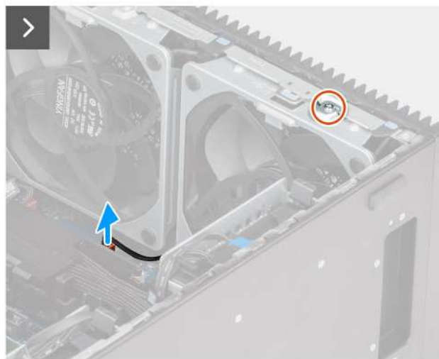
Afbeelding 46. Voorste ventilator 2
