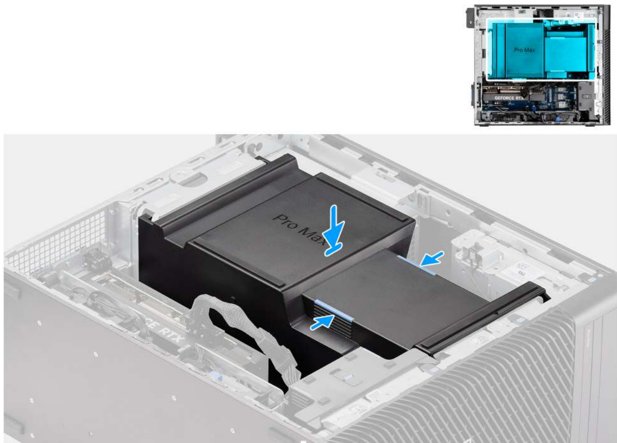
Afbeelding 14. De luchtkap plaatsen
