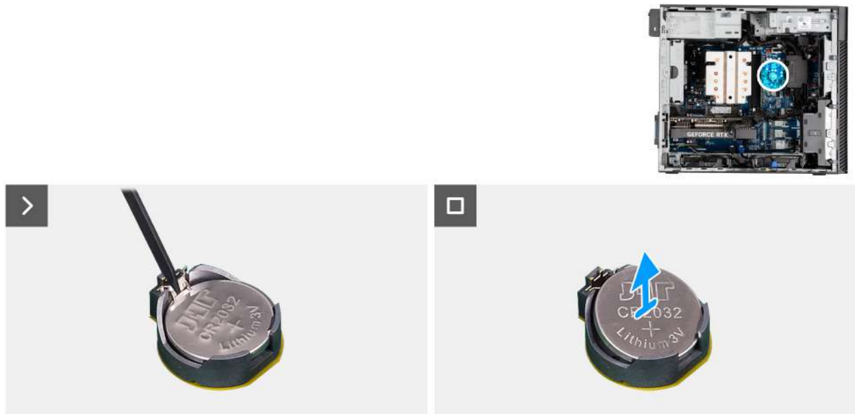
Afbeelding 15. De knoopcelbatterij verwijderen
