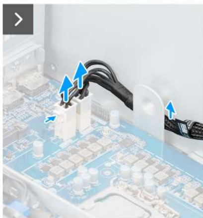
Afbeelding 53. De voedingseenheid van 1500 W verwijderen
