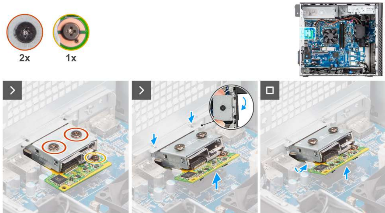
Afbeelding 73. De optionele optische 5 GbE-module verwijderen
