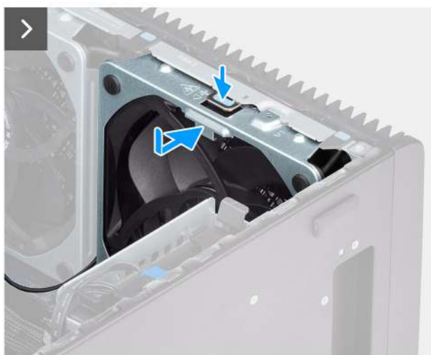
Afbeelding 48. Voorste ventilator 2
