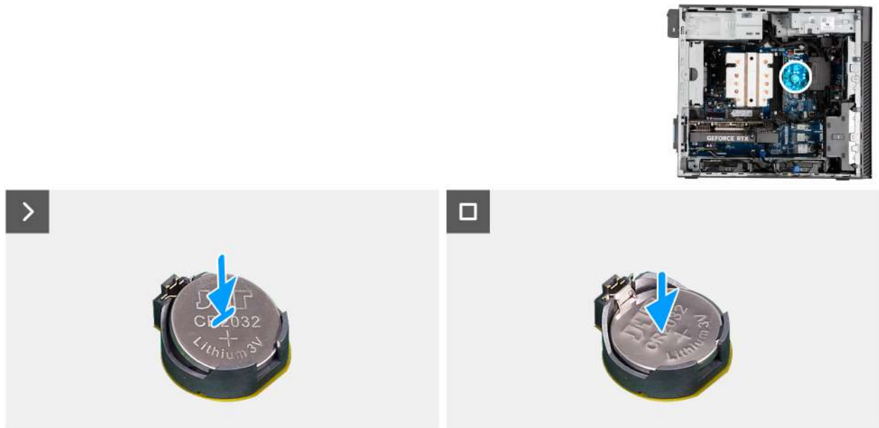
Afbeelding 16. De knoopcelbatterij plaatsen
