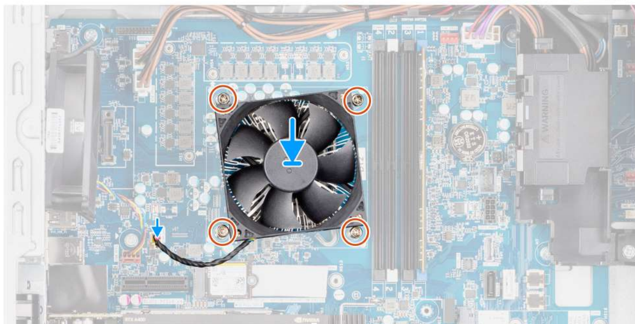
Afbeelding 62. De processorventilator en 65 W koelplaateneenheid plaatsen
