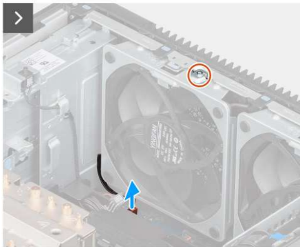
Afbeelding 45. Voorste ventilator 1
