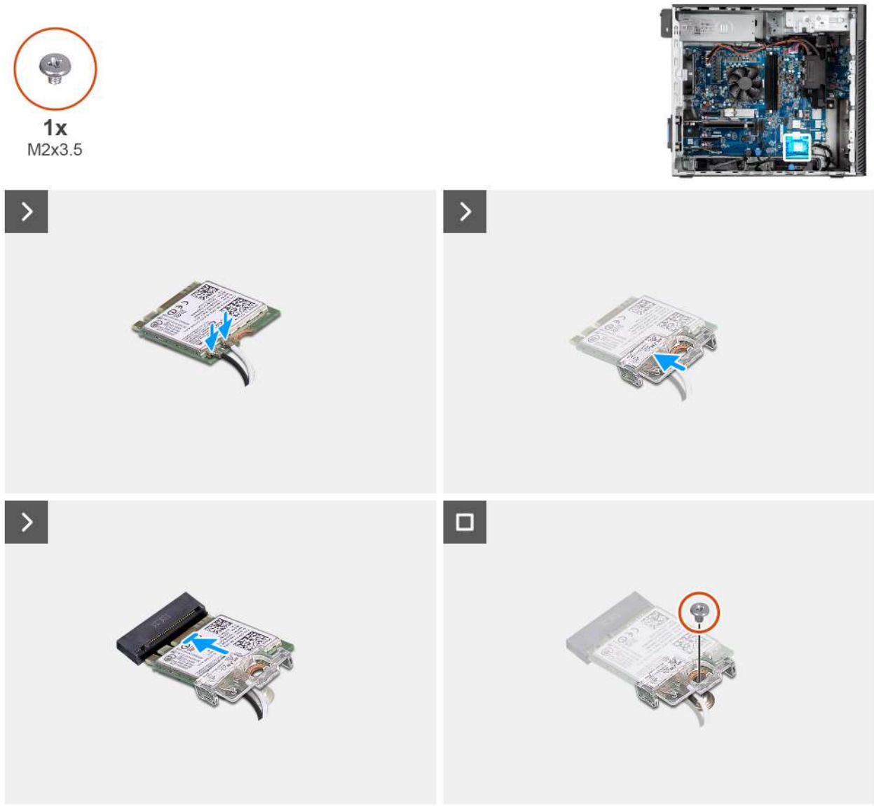
Afbeelding 42. De draadloze kaart plaatsen
