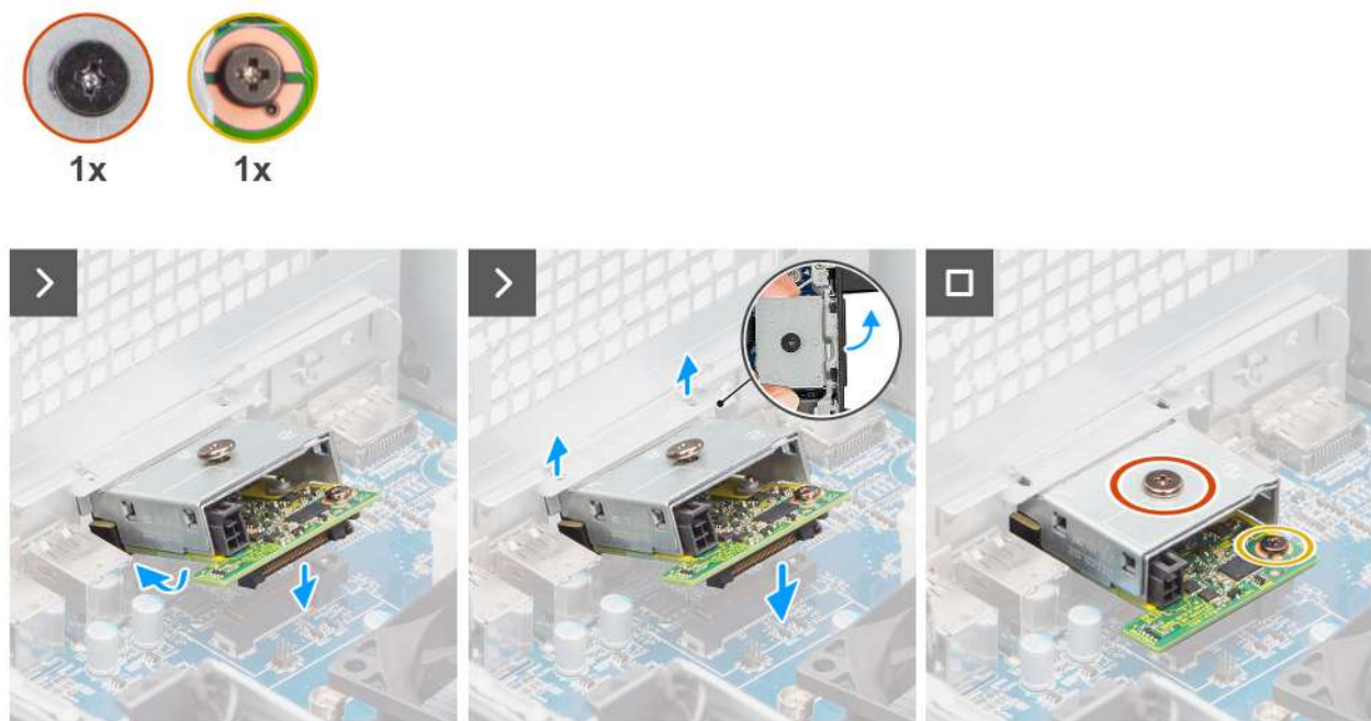
Afbeelding 84. De optionele USB-module installeren.
