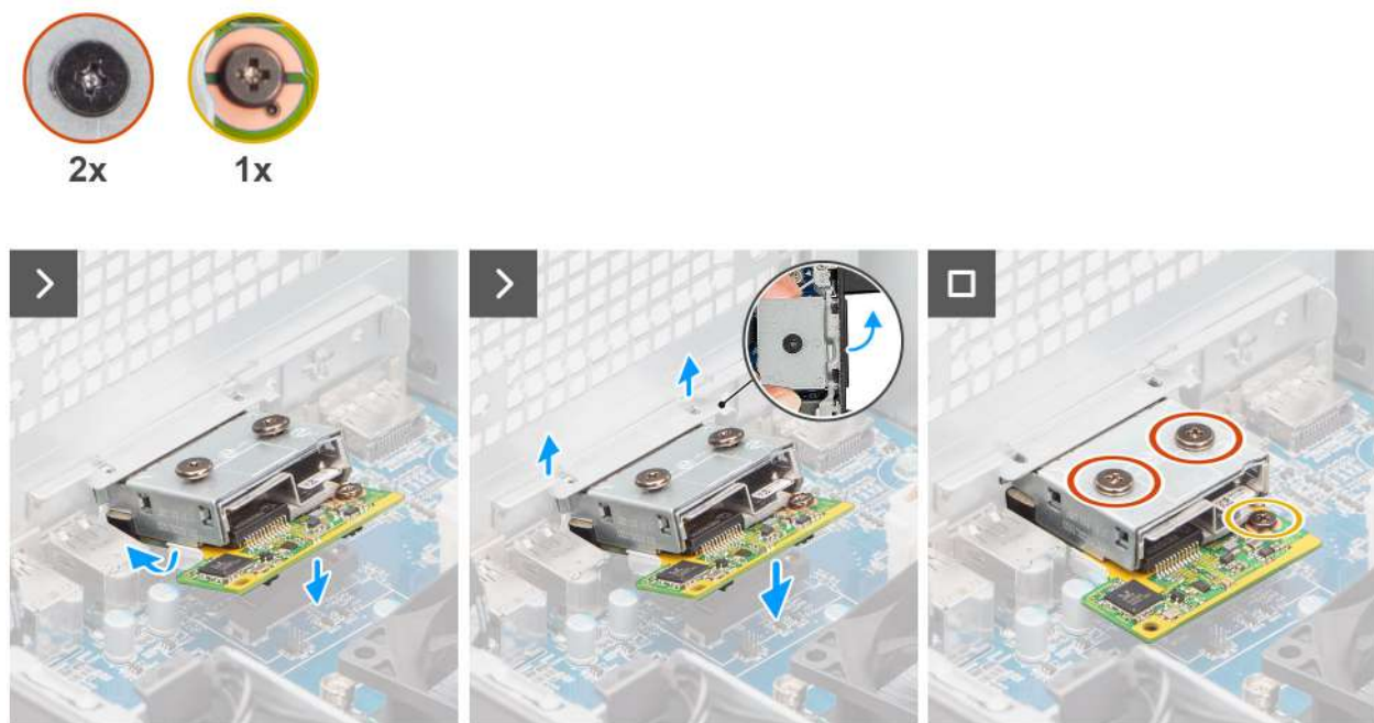
Afbeelding 75. De optionele optische 5 GbE-module installeren
