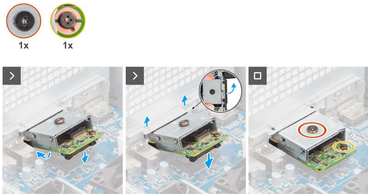
Afbeelding 78. De optionele LAN-module installeren.
