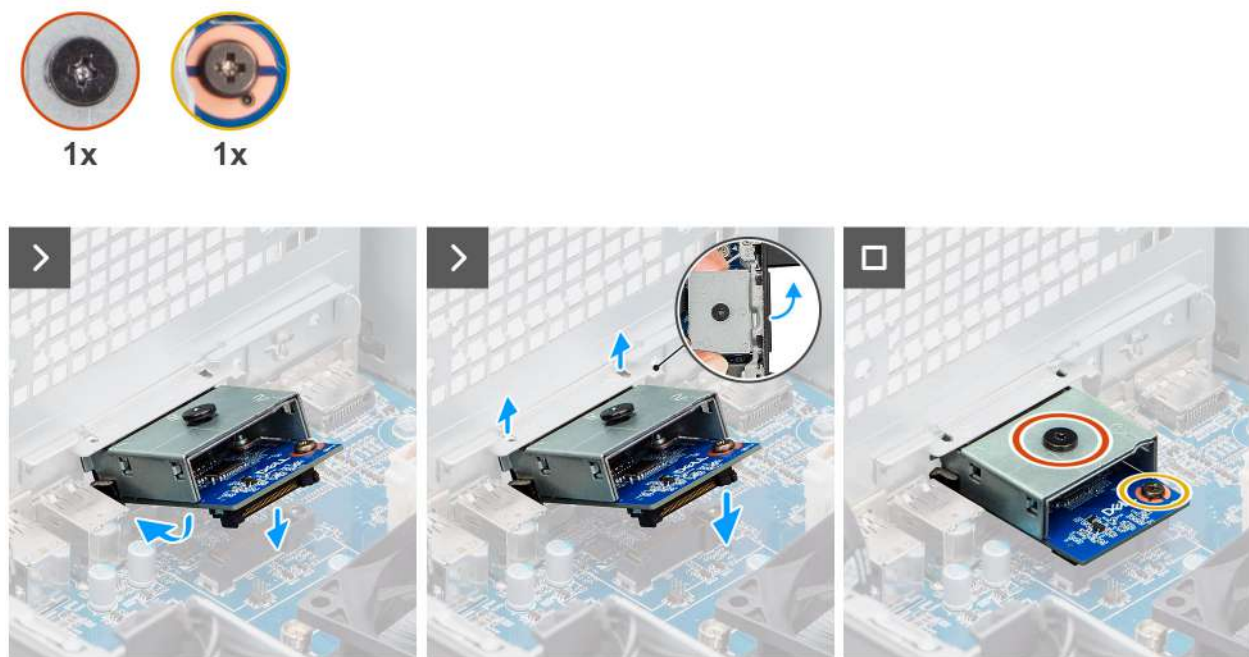
Afbeelding 72. De optionele HDMI-module installeren.
