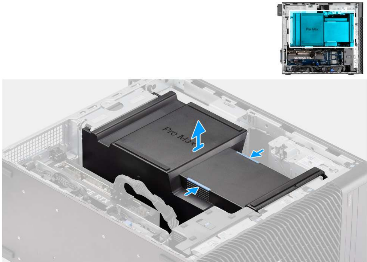
Afbeelding 13. De luchtkap verwijderen
