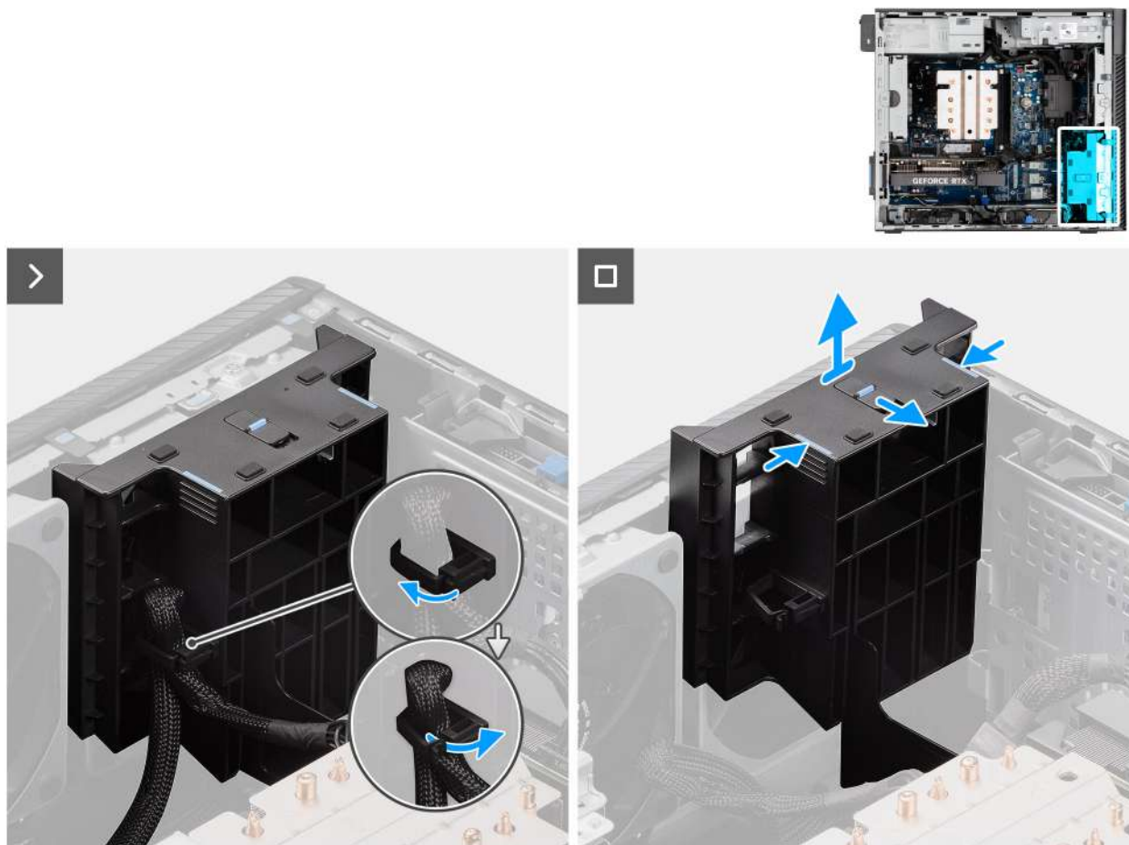
Afbeelding 35. De GPU-eindhouders verwijderen
