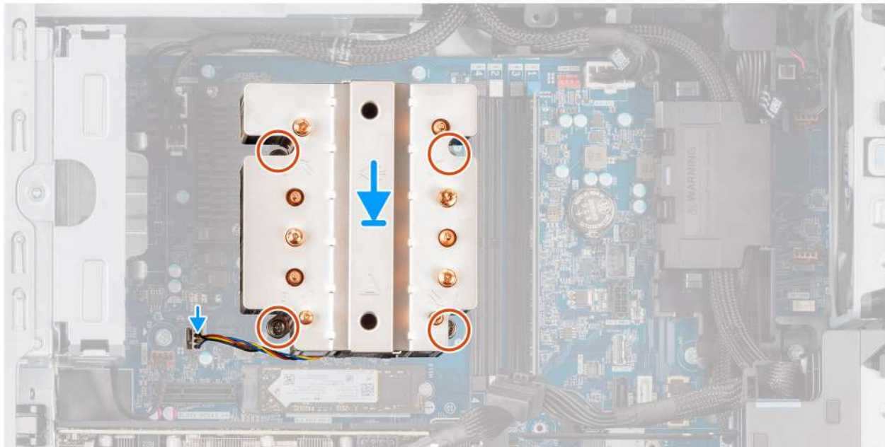
Afbeelding 60. De processorventilator en 125 W koelplaat eenheid plaatsen
