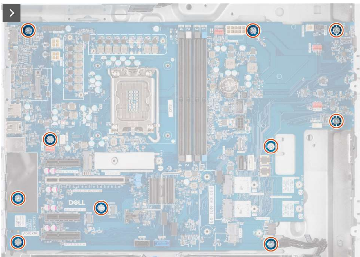
Afbeelding 91. De systeemkaart verwijderen
