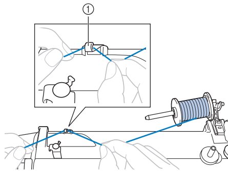
① Fadenführung
