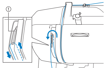
① Fadenhebel
