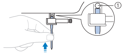
① Nadelanschlag
