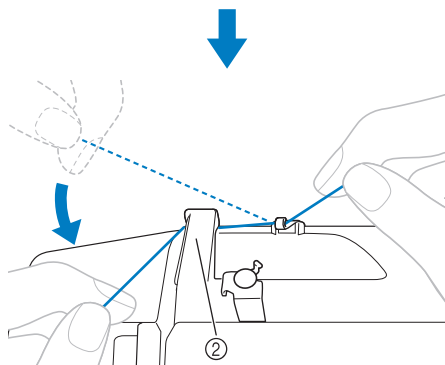
② Fadenführungsdeckel
