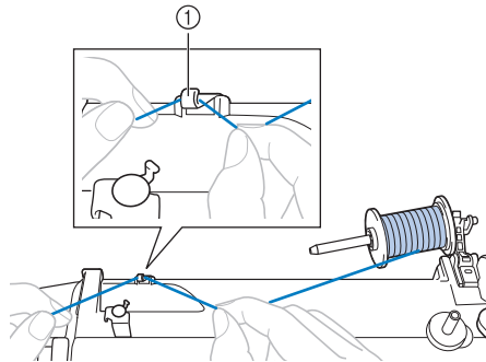
① Fadenführung
