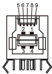
Afbeelding 10. USB Type-B 5 Gbps upstream-poort
