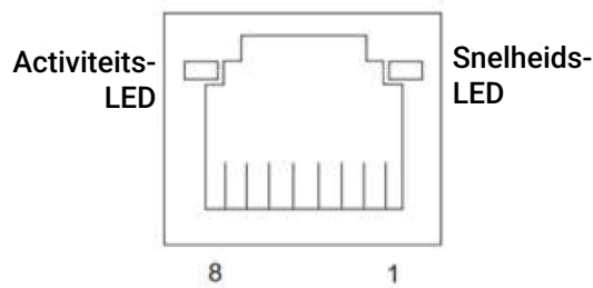
Afbeelding 13. RJ45-poort (connectorzijde)
