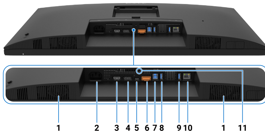
Afbeelding 3. Onderaanzicht van het beeldscherm
