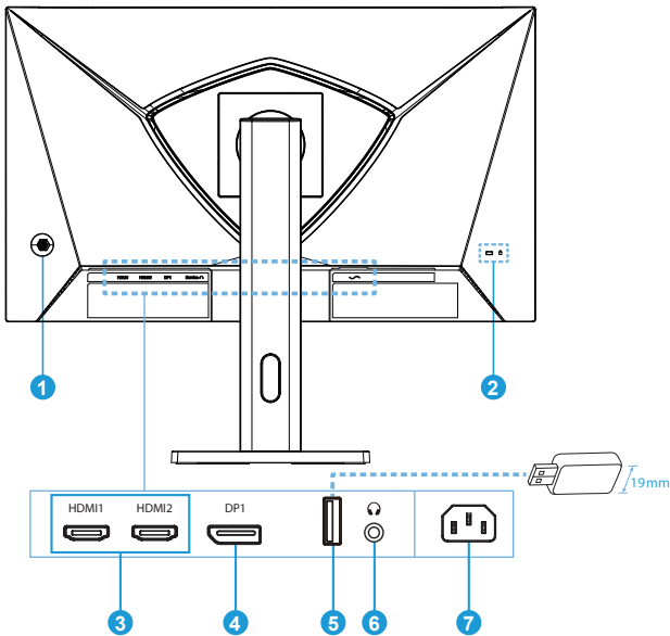
1 Betriebs-LED
