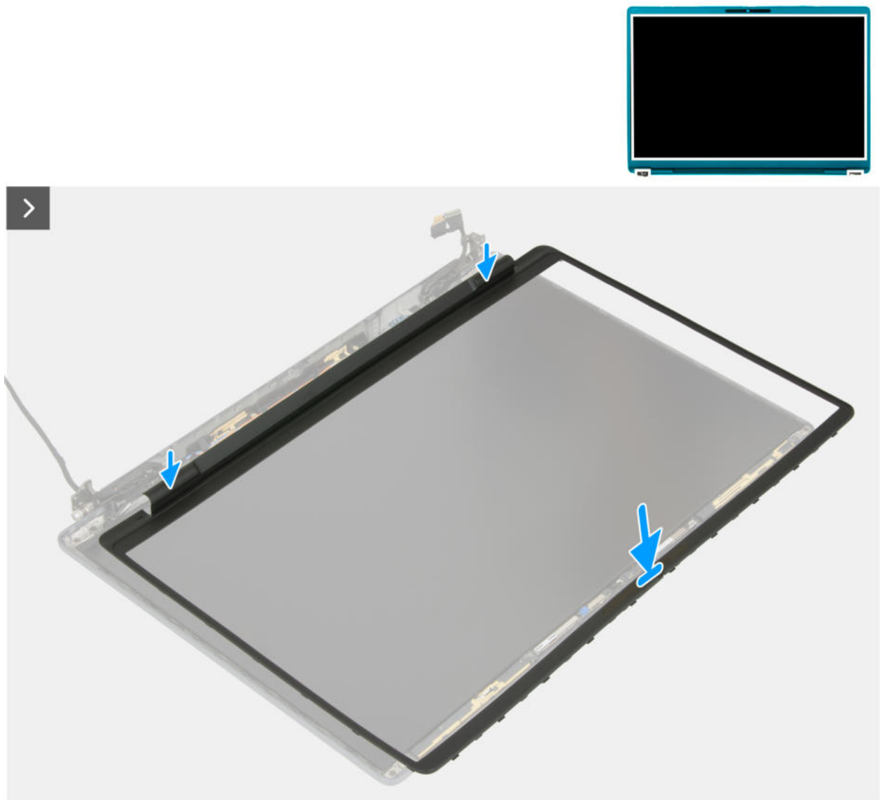
Abbildung 89. Einbauen der Bildschirmblende
