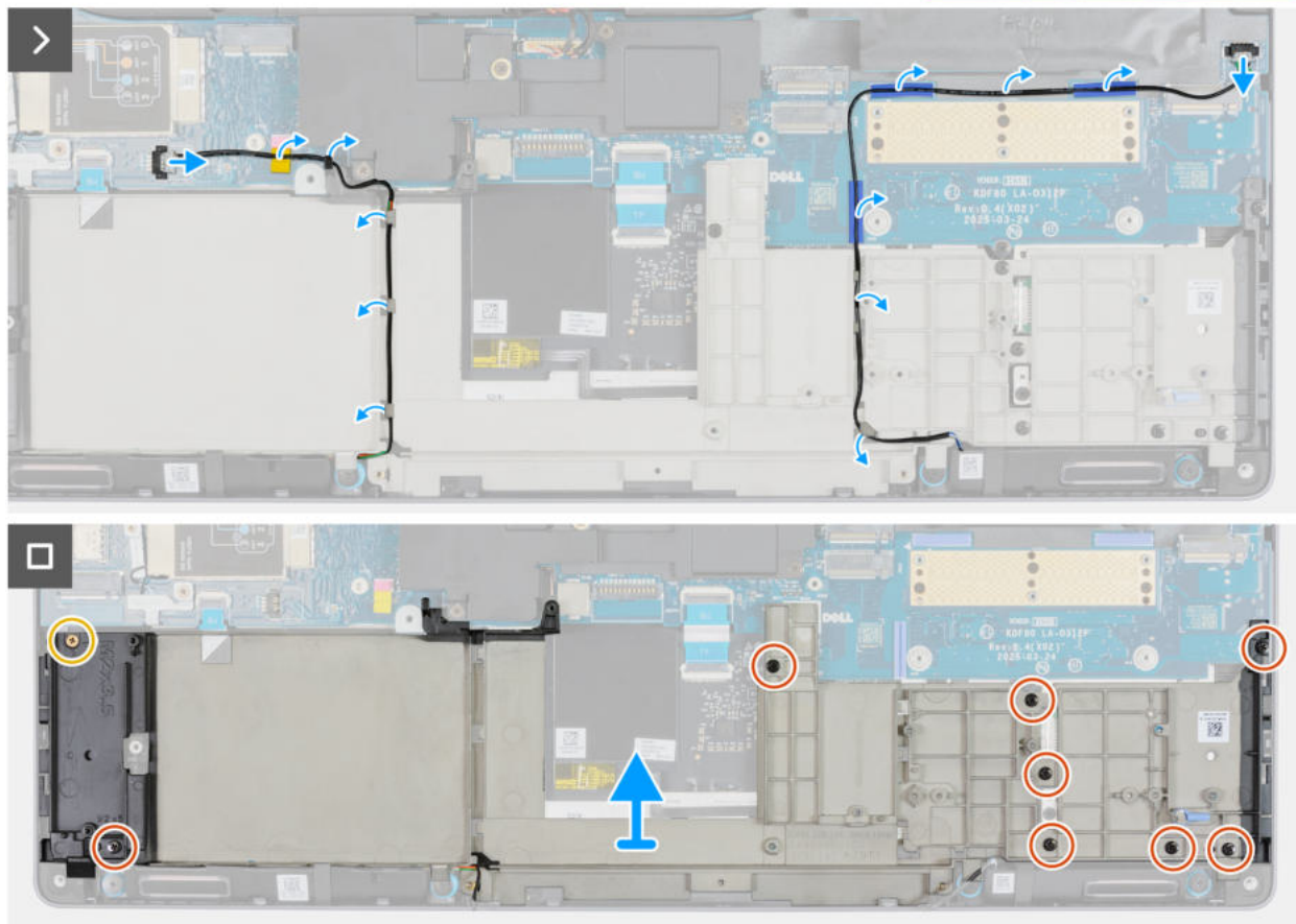
Abbildung 79. Entfernen des inneren Rahmens
