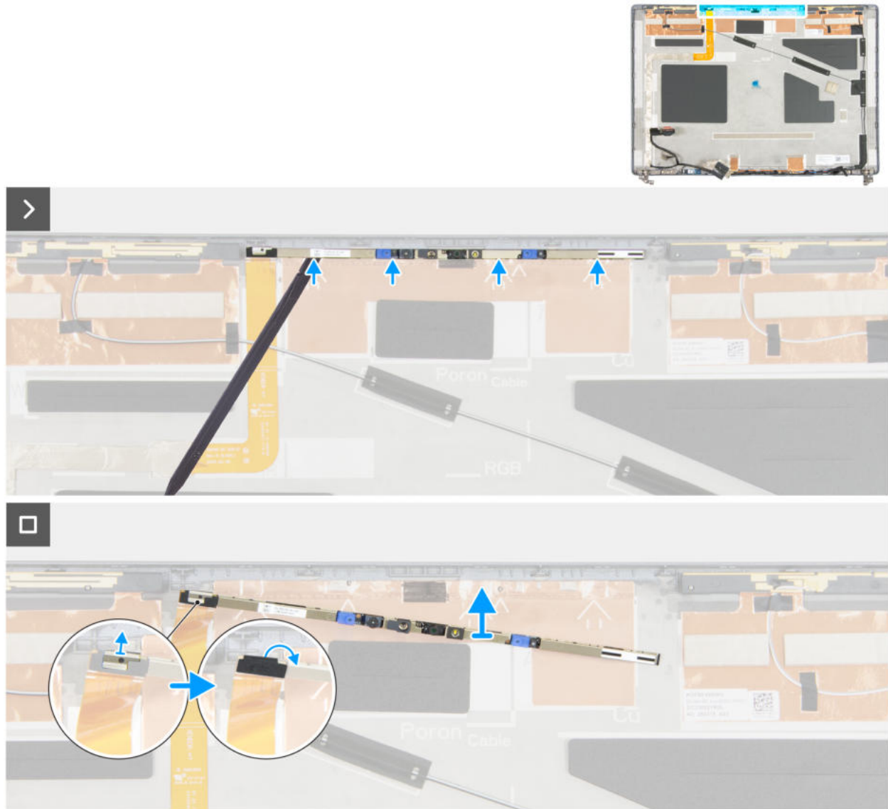
Abbildung 103. Entfernen des Kameramoduls
