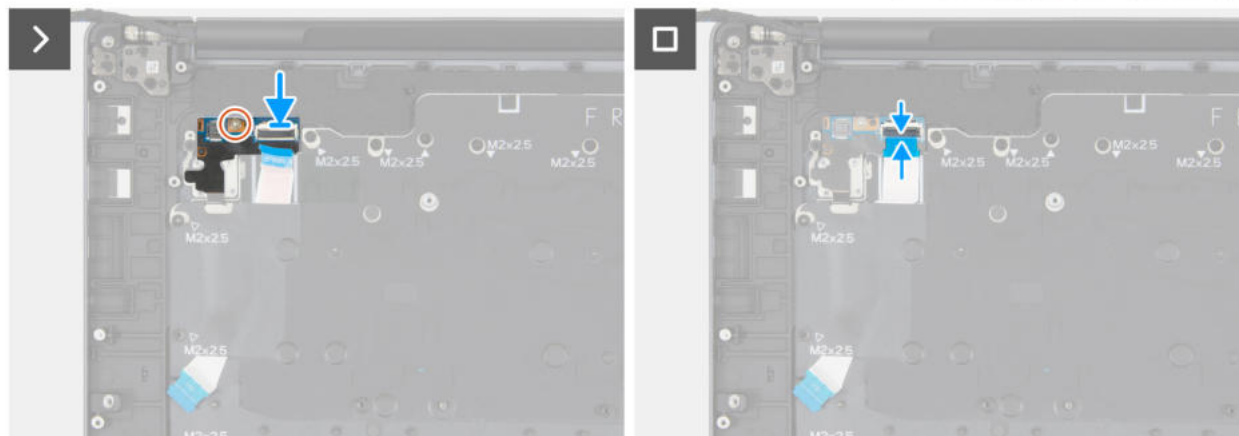
Abbildung 128. Einbauen der Netzschalterplatine
