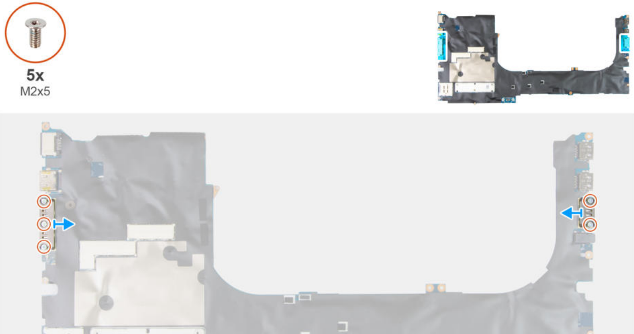
Abbildung 115. Entfernen des USB-Typ-C-Anschlussmoduls
