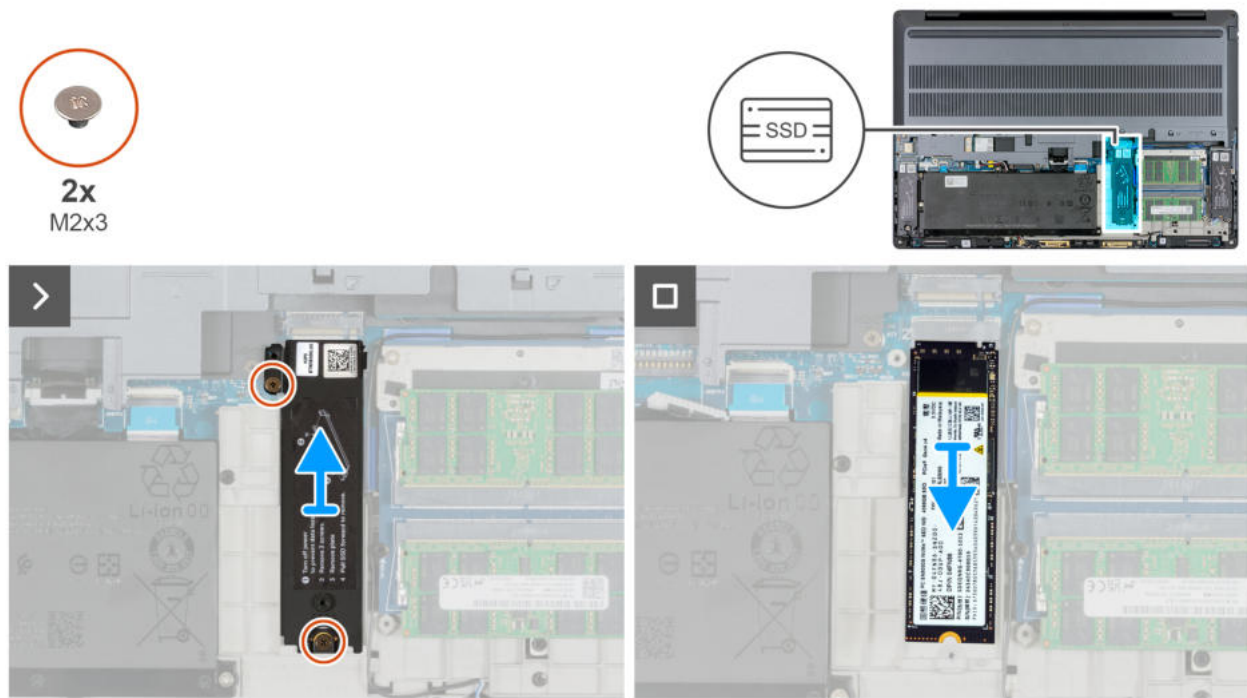
Abbildung 36. Entfernen der M.2-2280-SSD aus Steckplatz 3 (SSD3)
