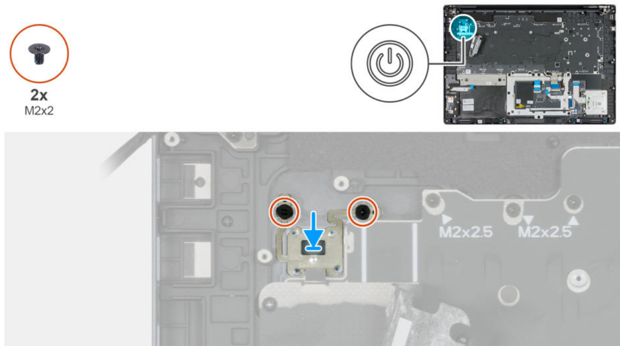
Abbildung 130. Installieren des Netzschalters
