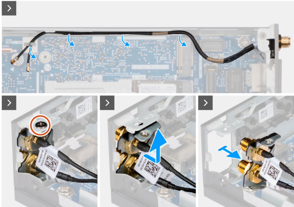
Abbildung 36. Entfernen der SMA-Antenne
