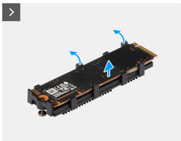
Abbildung 24. Entfernen des M.2 2280-PCIe-SSD-Laufwerks
