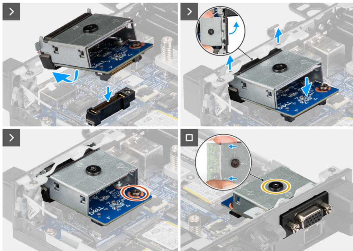
Abbildung 52. Installieren des VGA-Anschlussmoduls
