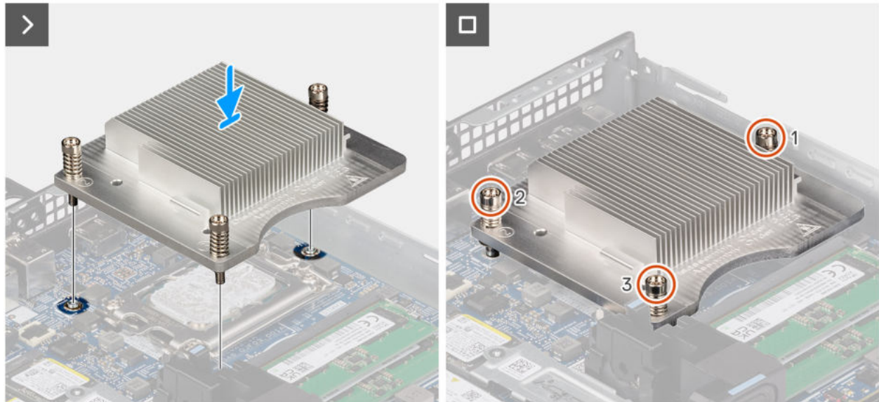
Abbildung 63. Einsetzen des Kühlkörpers
