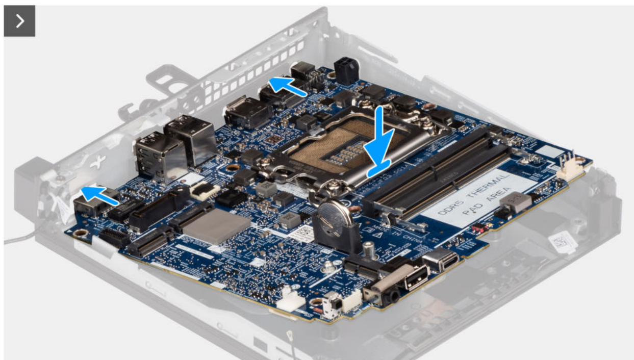
Abbildung 78. Einbauen der Systemplatine
