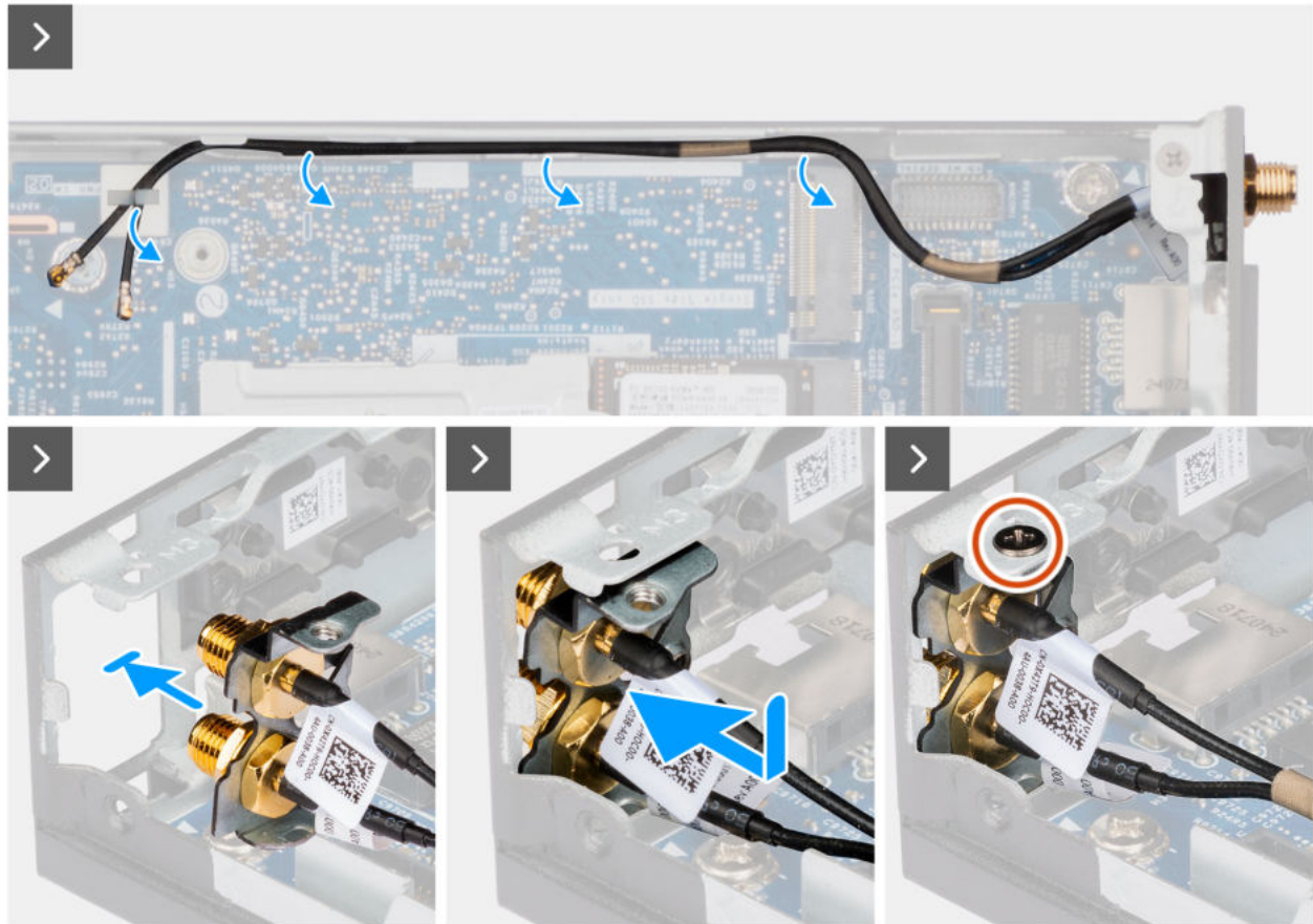
Abbildung 37. Installieren des SMA-Antennenmoduls
