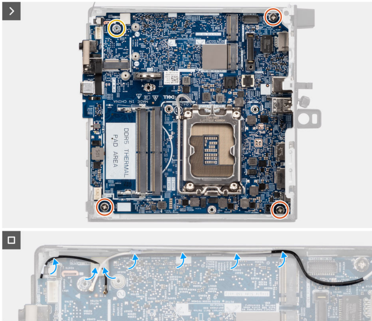
Abbildung 79. Einbauen der Systemplatine
