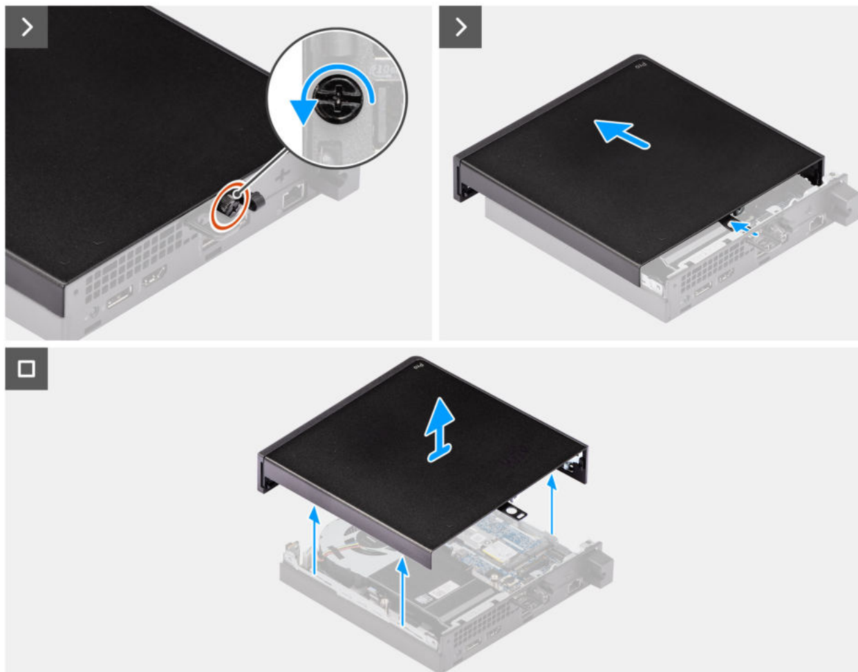
Abbildung 10. Entfernen der Seitenabdeckung
