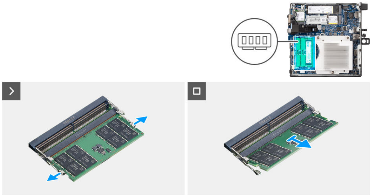
Abbildung 32. Entfernen des Arbeitsspeichersmoduls
