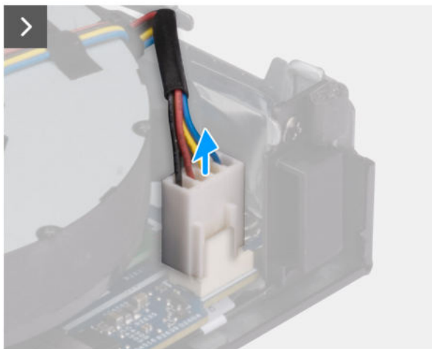
Abbildung 28. Entfernen des Lüfters
