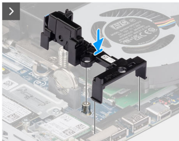
Abbildung 73. Installieren der Lautsprecherhalterung
