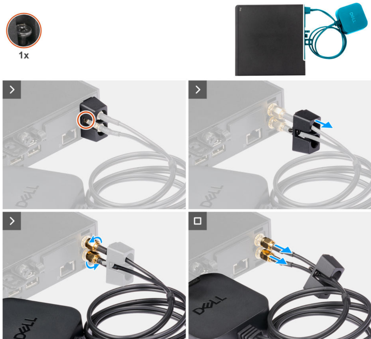
Abbildung 34. Entfernen der externen Puck-Antenne
