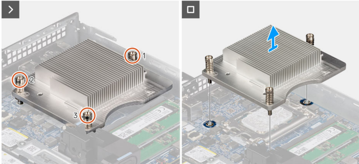
Abbildung 62. Kühlkörper entfernen
