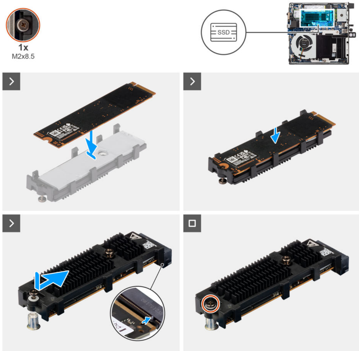
Abbildung 25. Einbauen des M.2 2280-PCIe-SSD-Laufwerks
