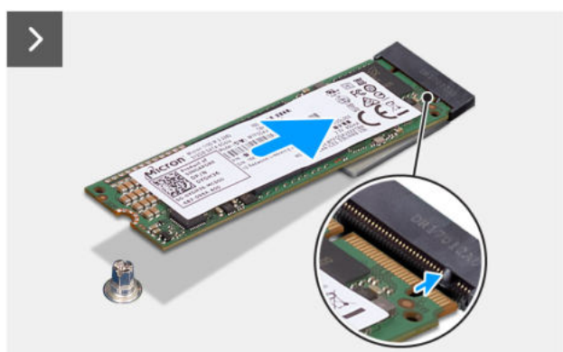
Abbildung 21. Einbauen des M.2-2280-Solid-State-Laufwerks
