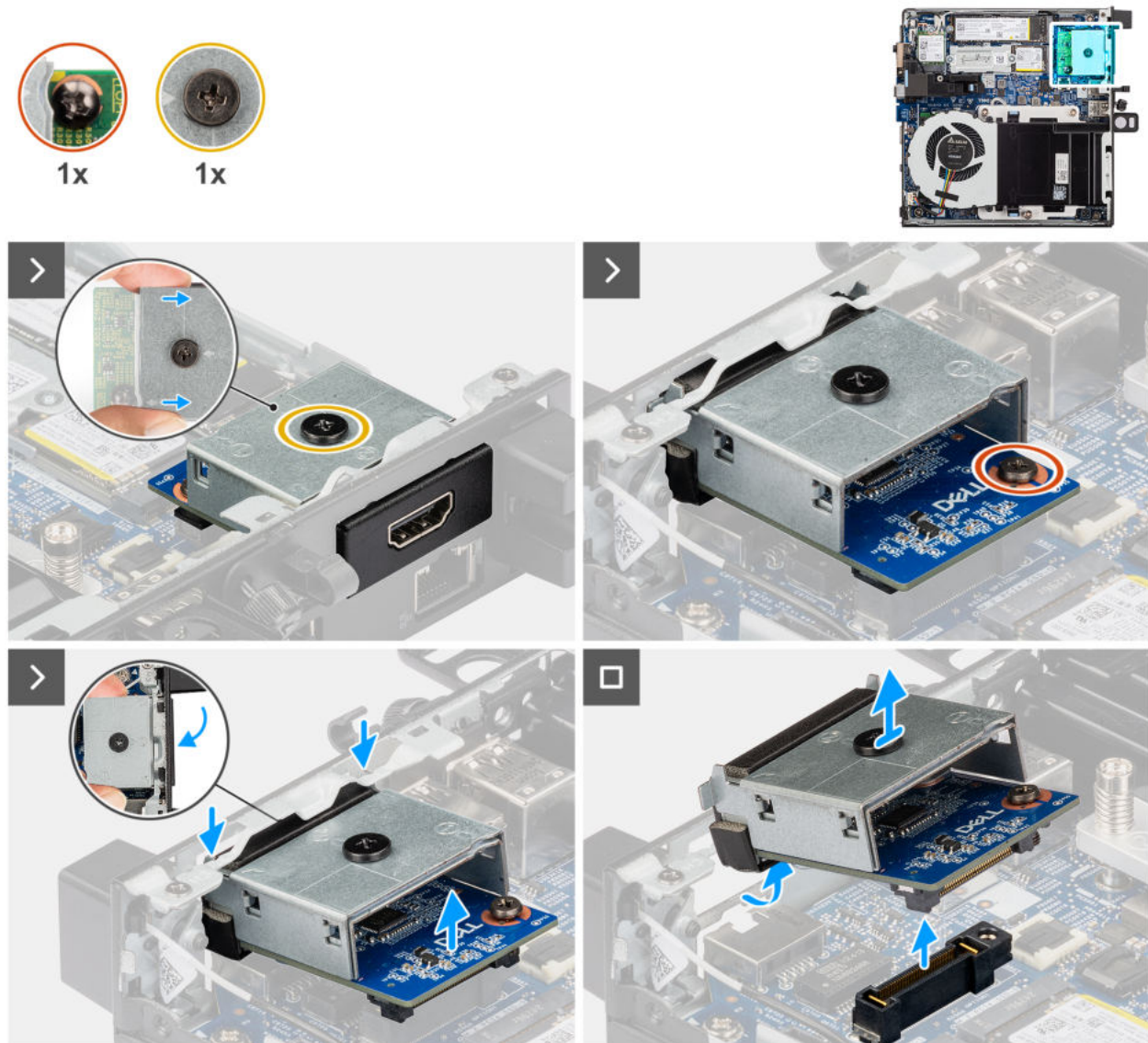
Abbildung 47. Entfernen des HDMI-Anschlussmoduls
