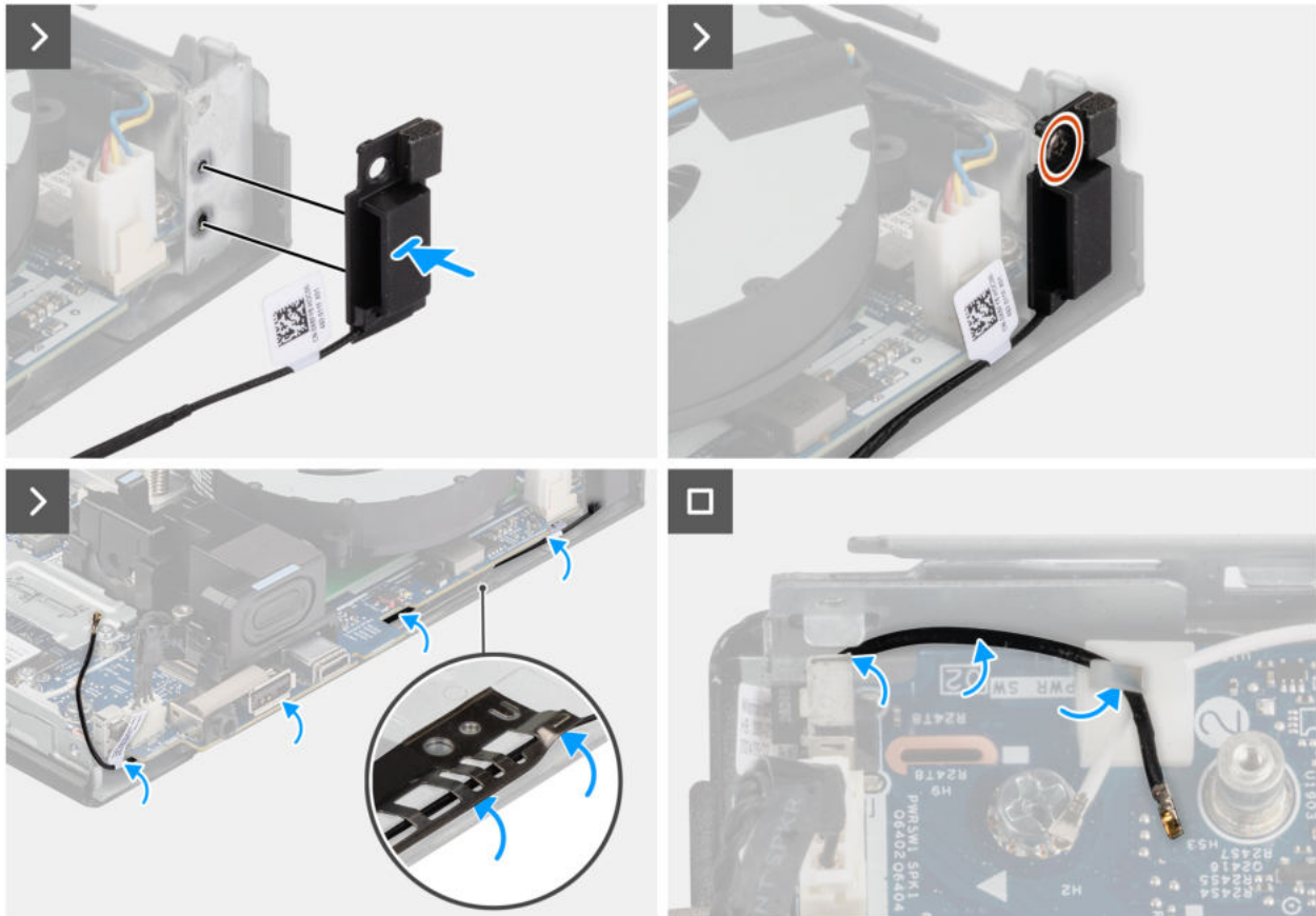
Abbildung 65. Einbauen des Antennenmoduls (schwarzes Kabel)
