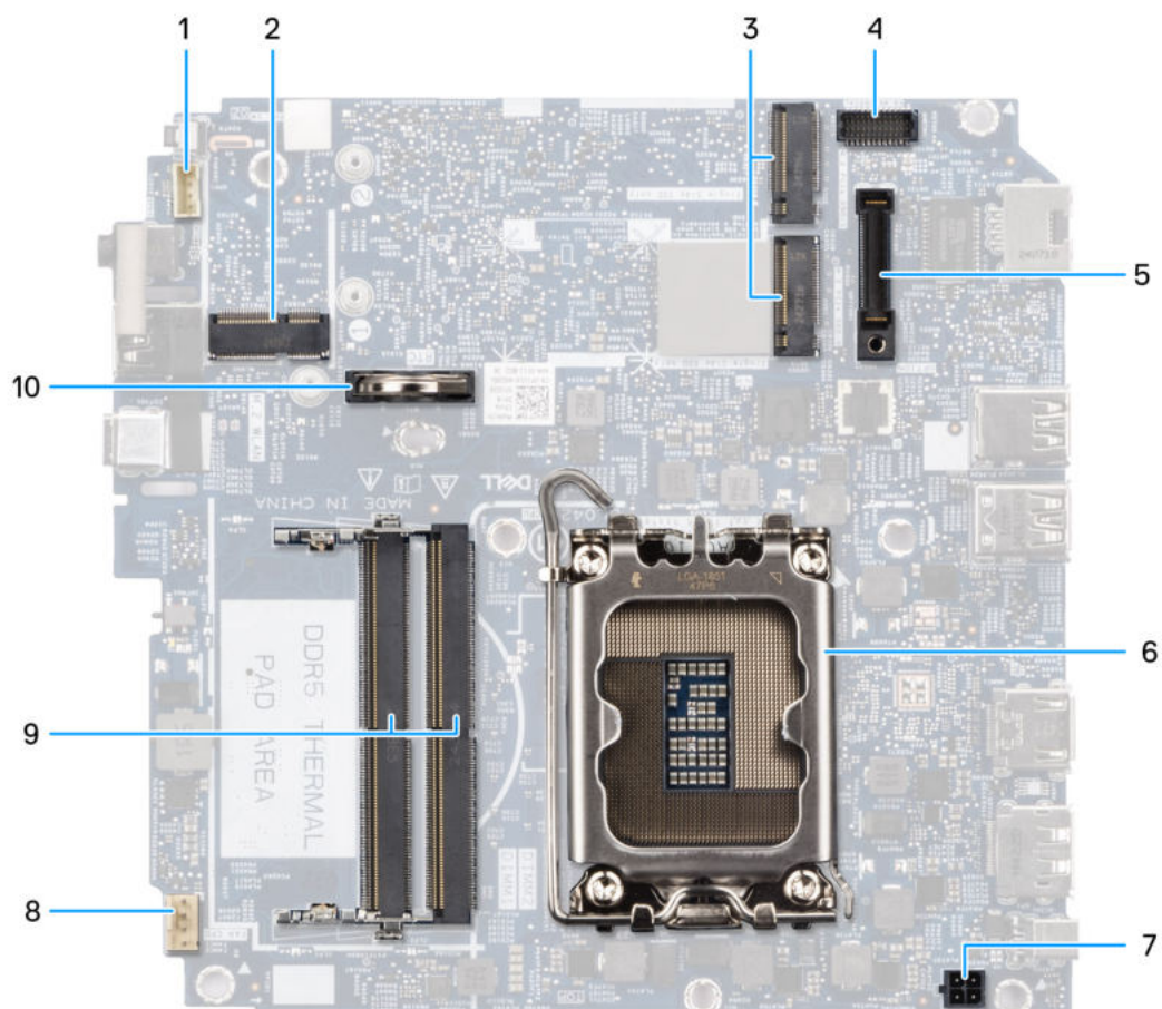
Abbildung 74. Anschlüsse auf der Hauptplatine
