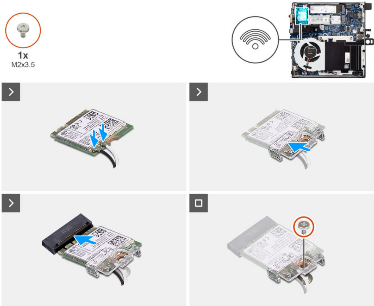
Abbildung 27. Installieren der Wireless-Karte
