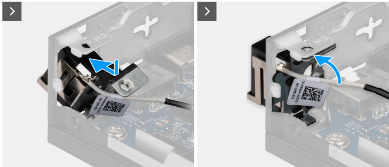
Abbildung 68. Einbauen des Antennenmoduls (weißes Kabel)
