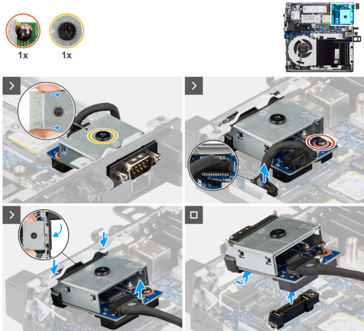
Abbildung 56. Entfernen des seriellen Anschlussmoduls
