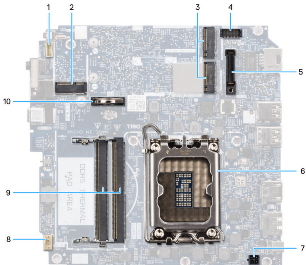
Abbildung 77. Anschlüsse auf der Hauptplatine
