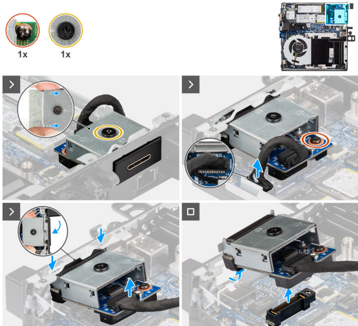
Abbildung 53. Entfernen des PS2-Anschlussmoduls
