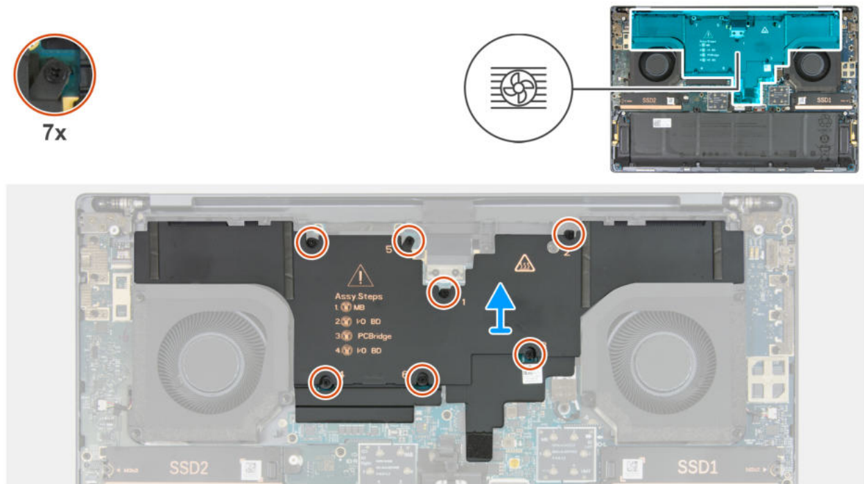
Abbildung 48. Kühlkörper entfernen
