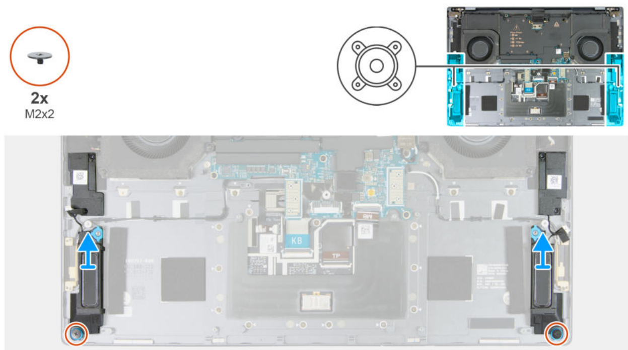
Abbildung 74. Entfernen der Lautsprecher
