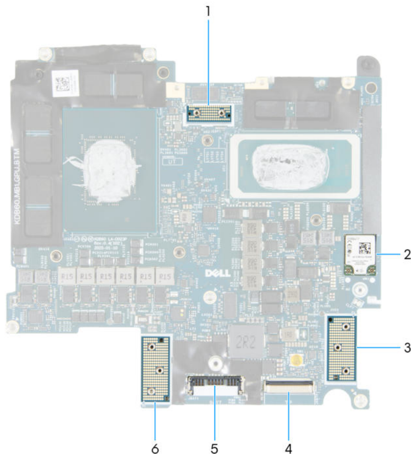
Abbildung 63. Anschlüsse auf der Hauptplatine
