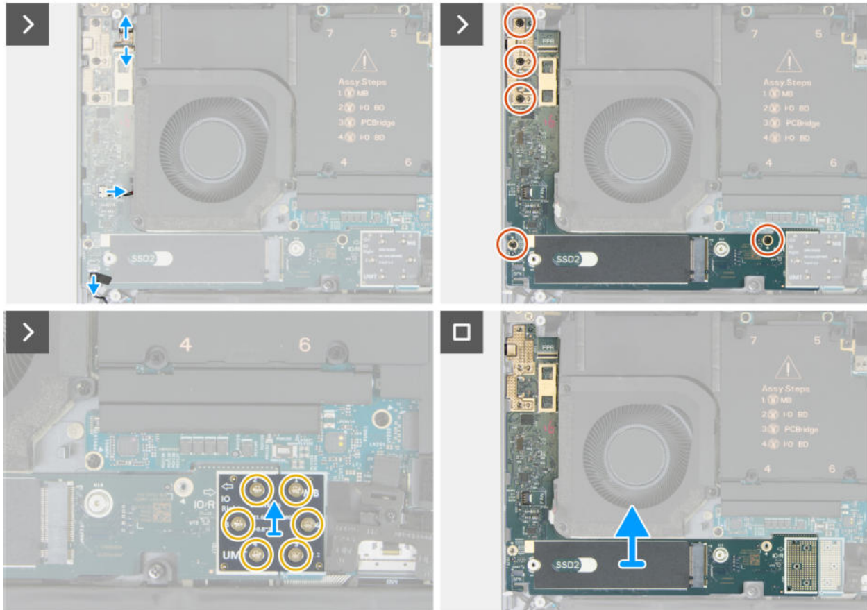
Abbildung 52. Entfernen der rechten E/A-Platine
