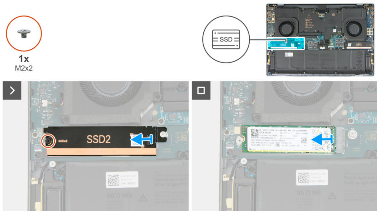
Abbildung 23. Entfernen des M.2 2280-Solid-State-Laufwerks (SSD2)
