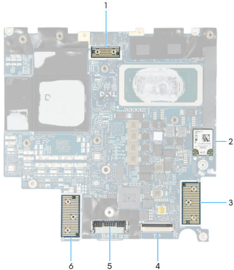
Abbildung 58. Anschlüsse auf der Hauptplatine
