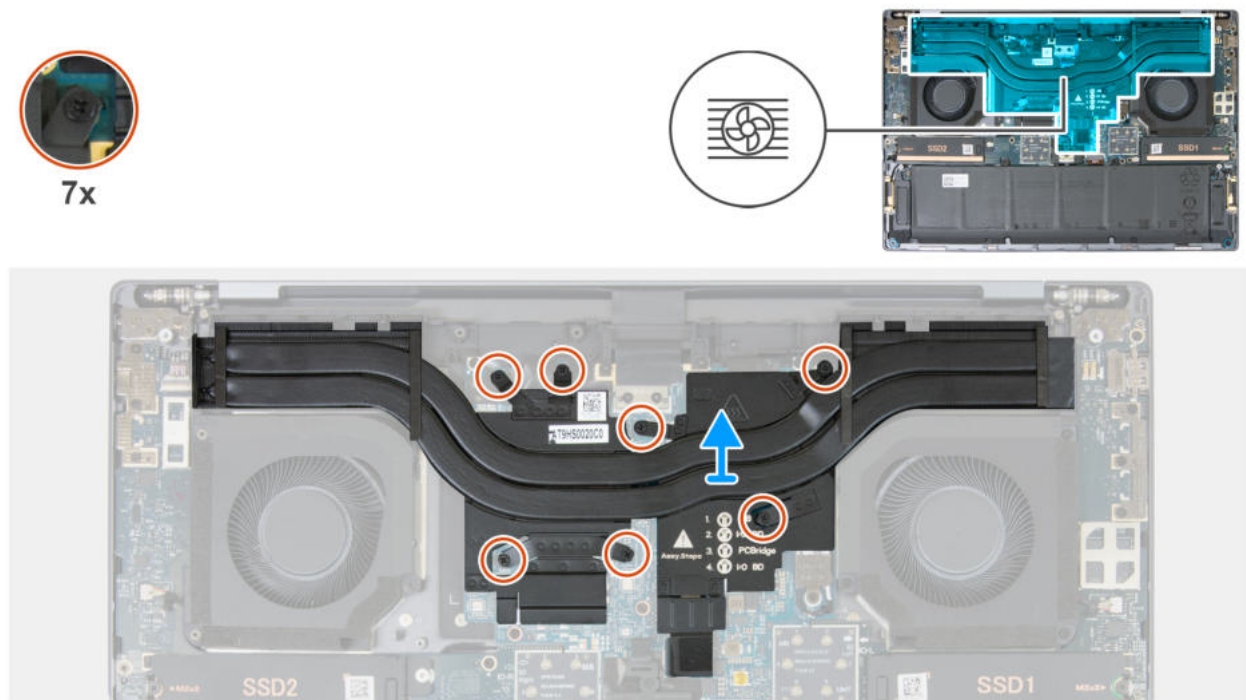
Abbildung 46. Kühlkörper entfernen
