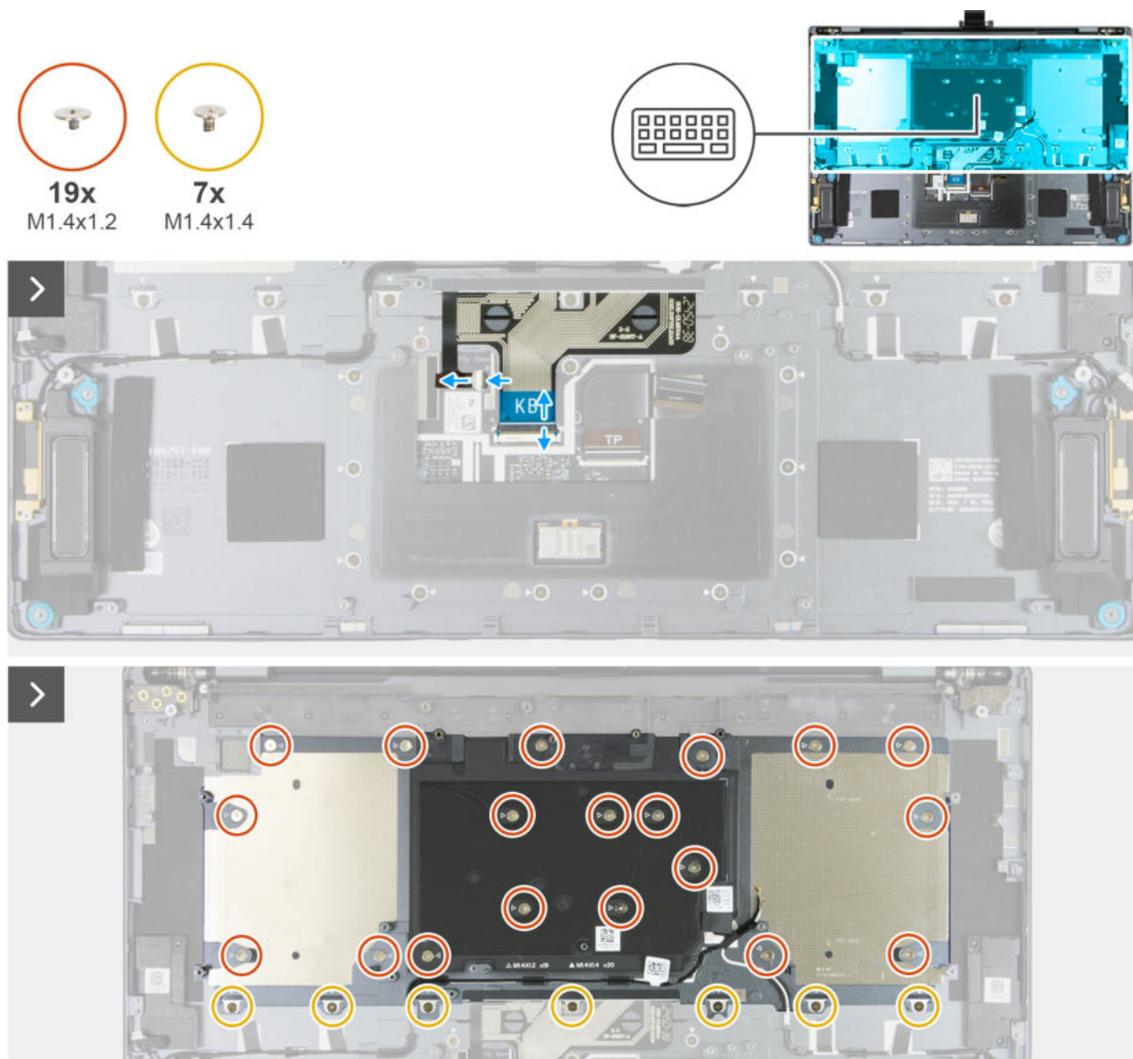
Abbildung 76. Entfernen der Tastatur
