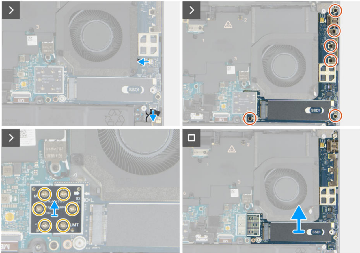
Abbildung 50. Entfernen der linken E/A-Platine
