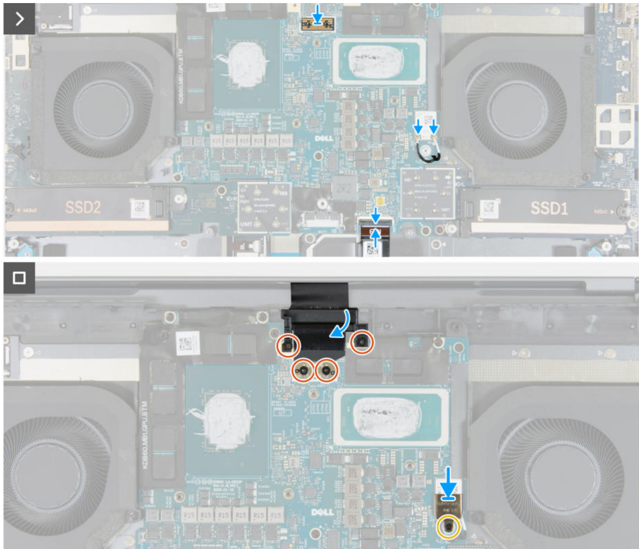
Abbildung 69. Einbauen der Hauptplatine (separate Grafikkarte)
