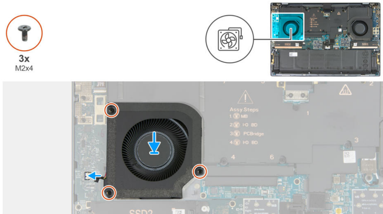
Abbildung 33. Installieren des rechten Lüfters
