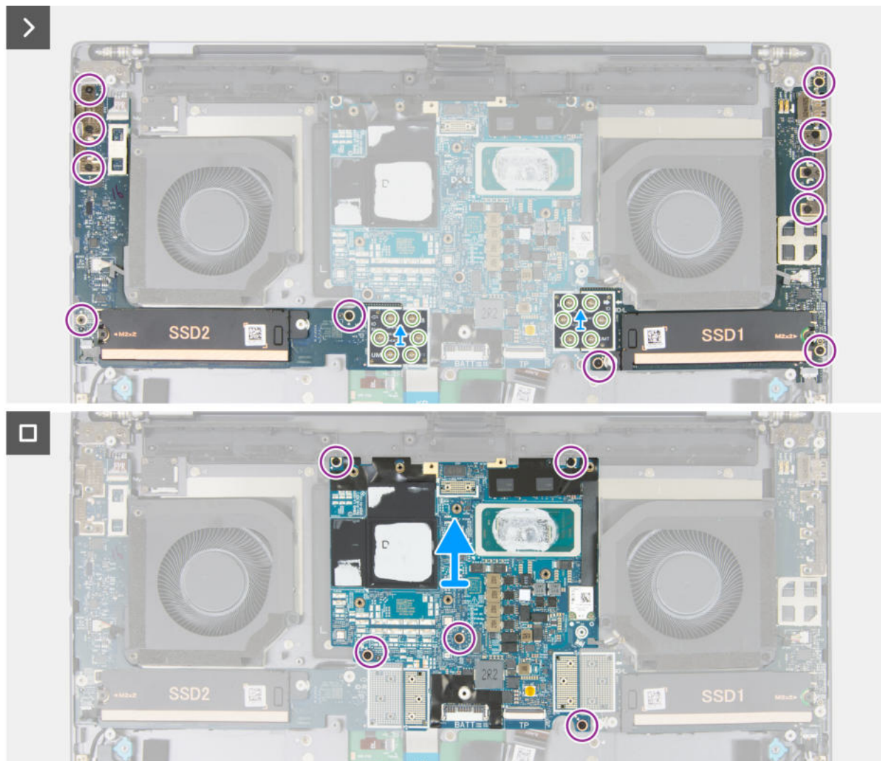
Abbildung 56. Entfernen der Hauptplatine (integrierte Grafikkarte)
