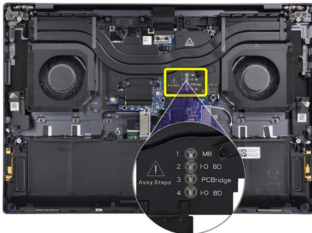
Abbildung 62. Auf dem Kühlkörper aufgedruckte Montageschritte
