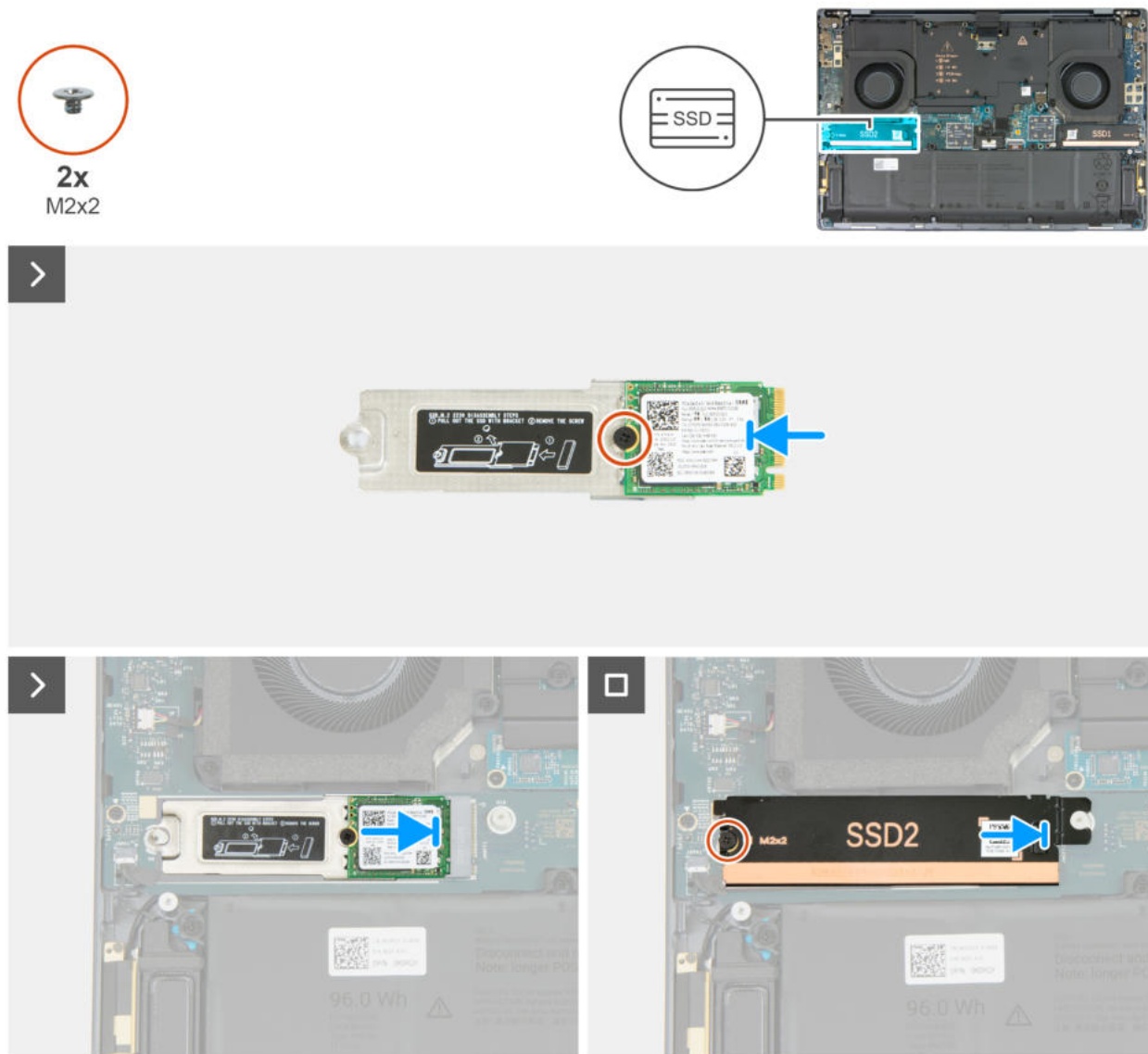
Abbildung 29. Einbauen des M.2 2230-Solid-State-Laufwerks (SSD2)
