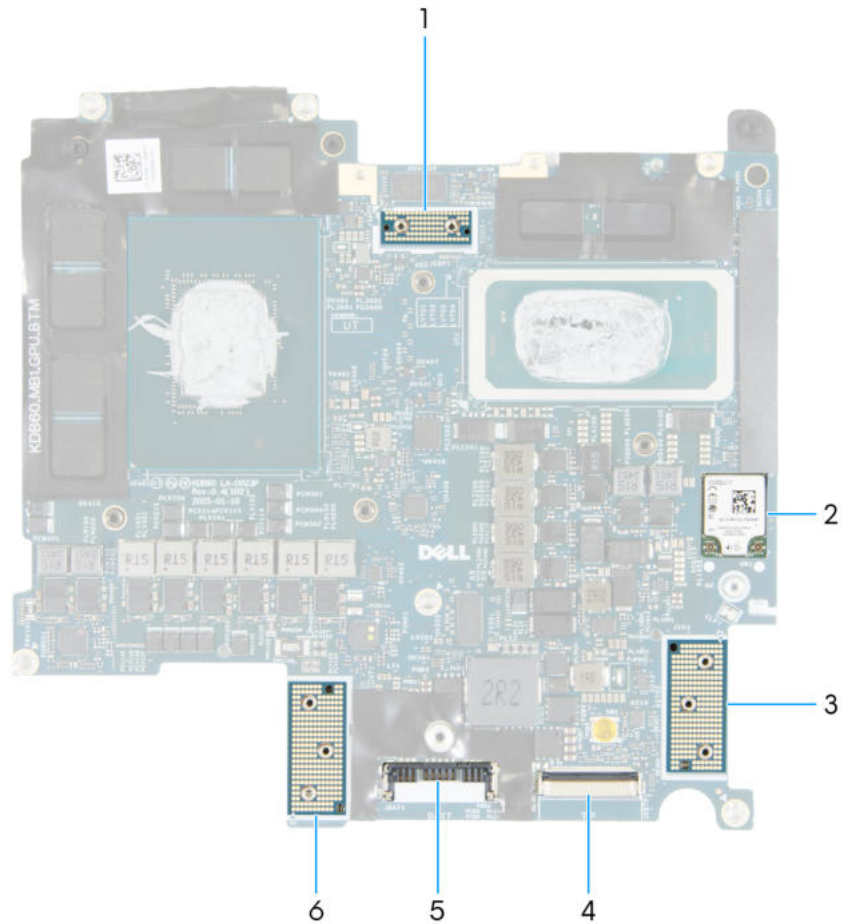
Abbildung 67. Anschlüsse auf der Hauptplatine
