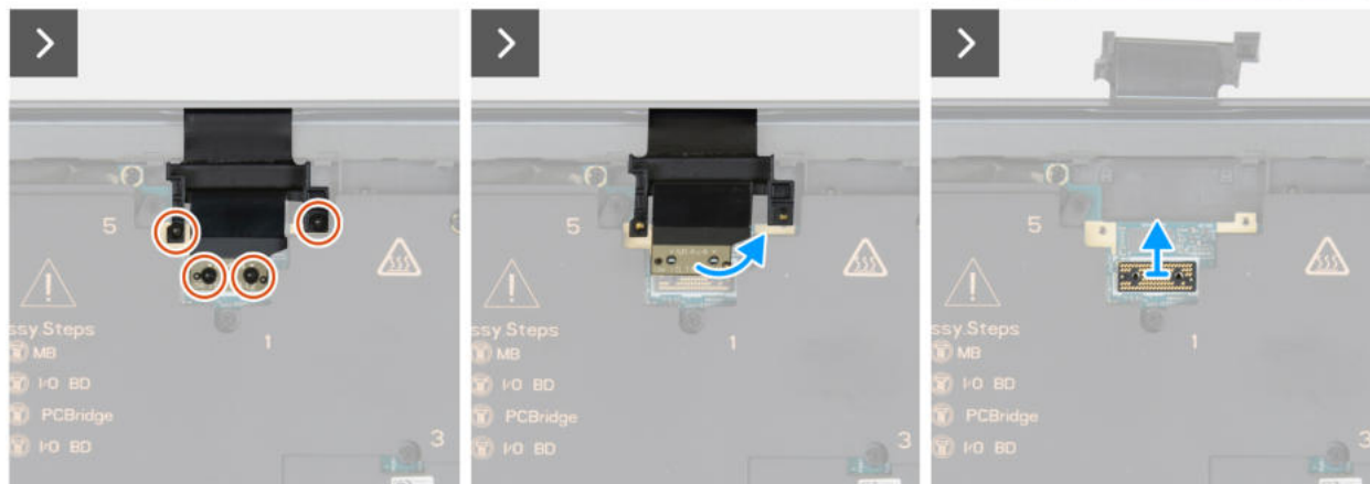
Abbildung 34. Entfernen der Bildschirmbaugruppe
