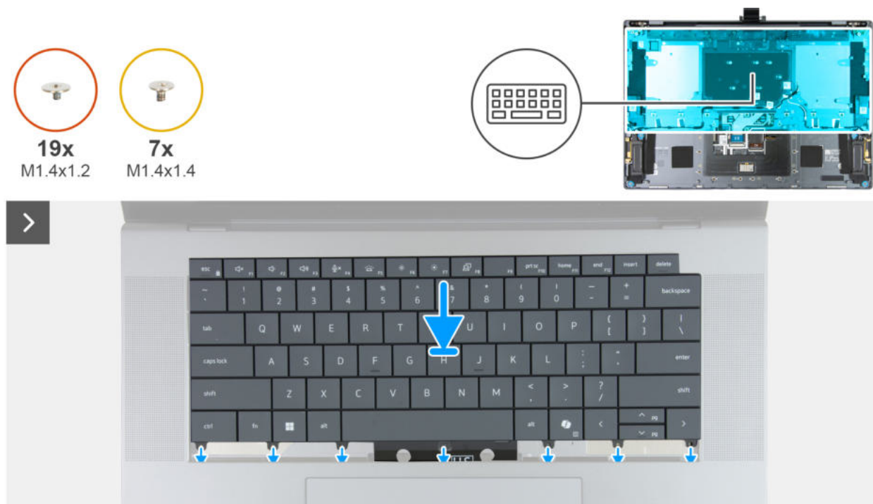
Abbildung 79. Einbauen der Tastatur
