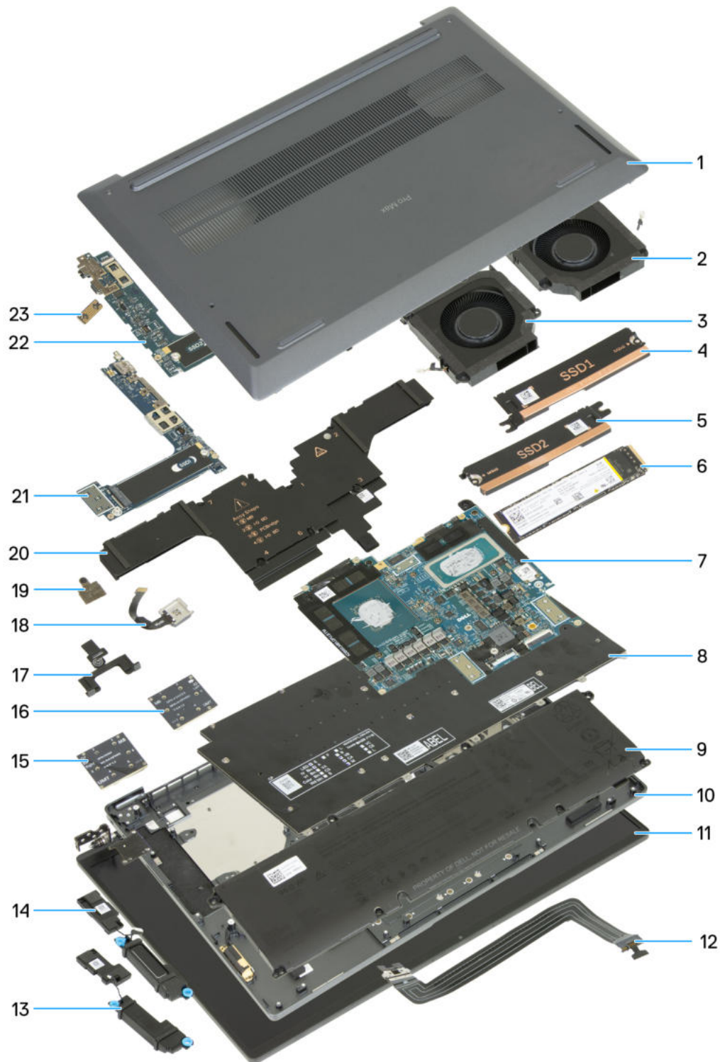
Abbildung 10. Hauptkomponenten Ihres Dell Pro Max 16 Premium-MA16250
