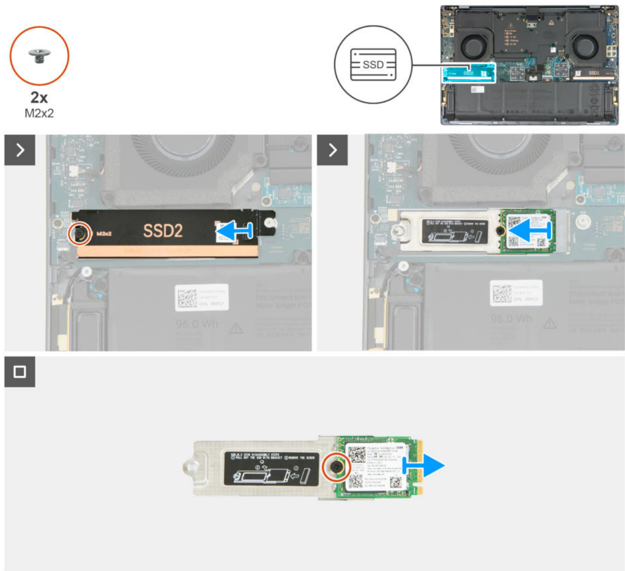
Abbildung 27. Entfernen des M.2 2230-Solid-State-Laufwerks (SSD2)
