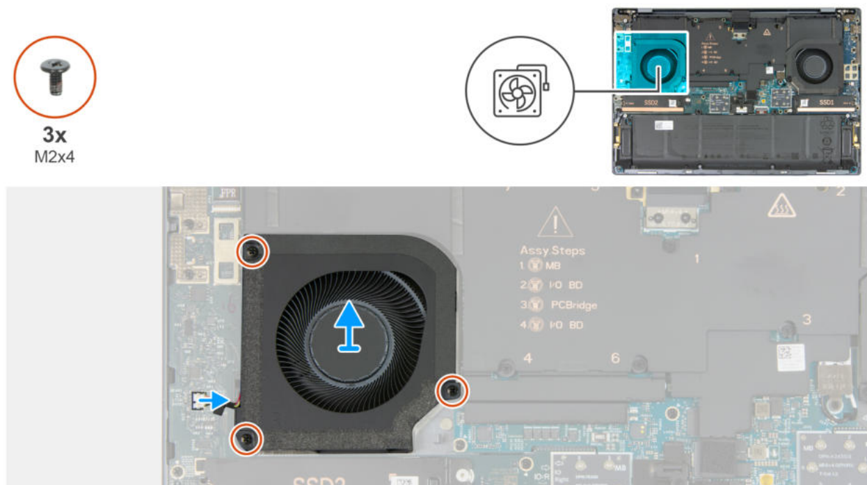
Abbildung 32. Entfernen des rechten Lüfters
