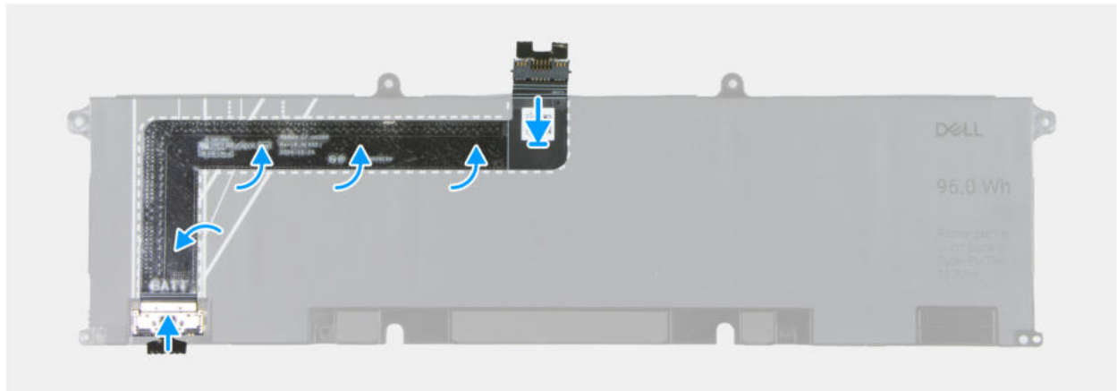
Abbildung 21. Einsetzen des Akkukabels
