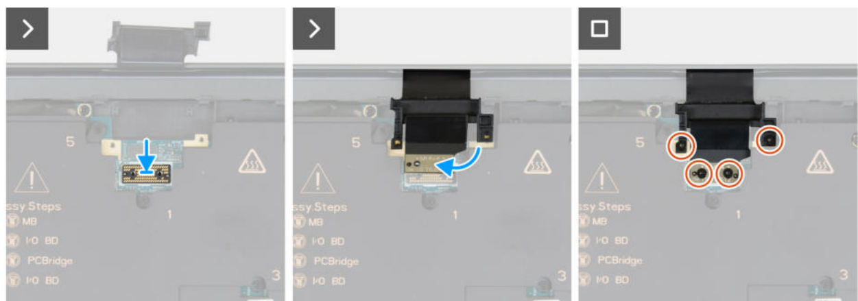
Abbildung 43. Einbauen der Bildschirmbaugruppe
