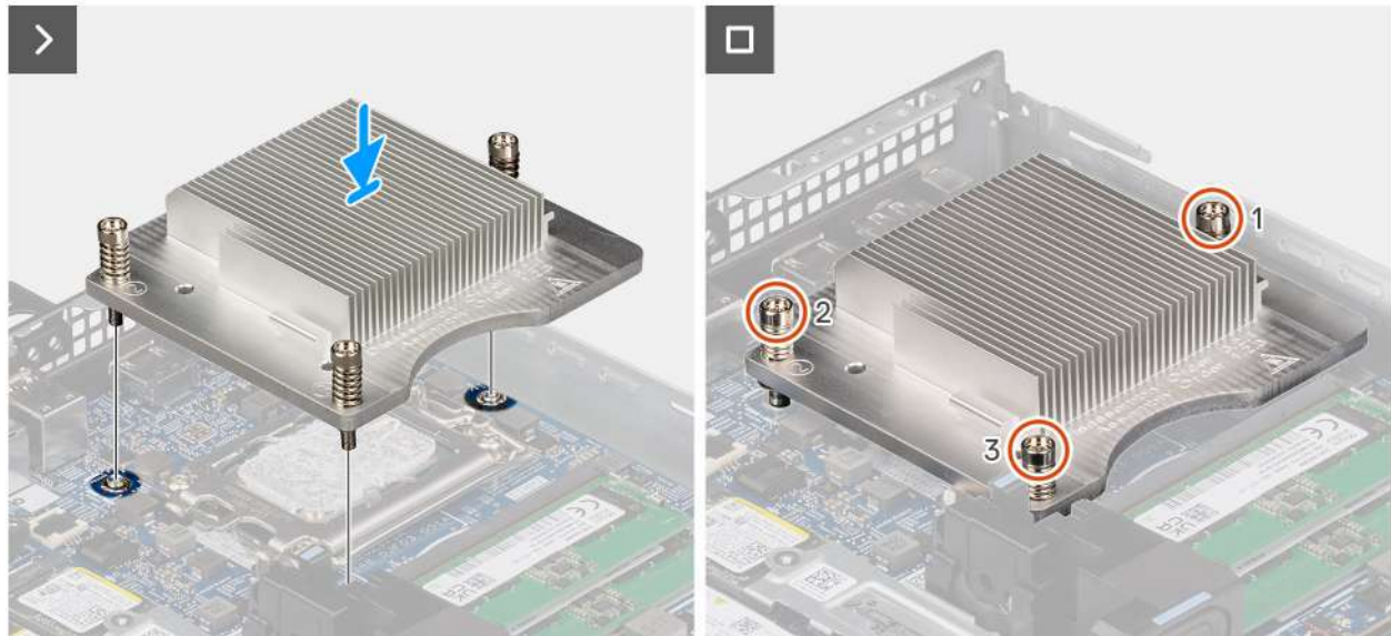
Afbeelding 63. De koelplaat plaatsen
