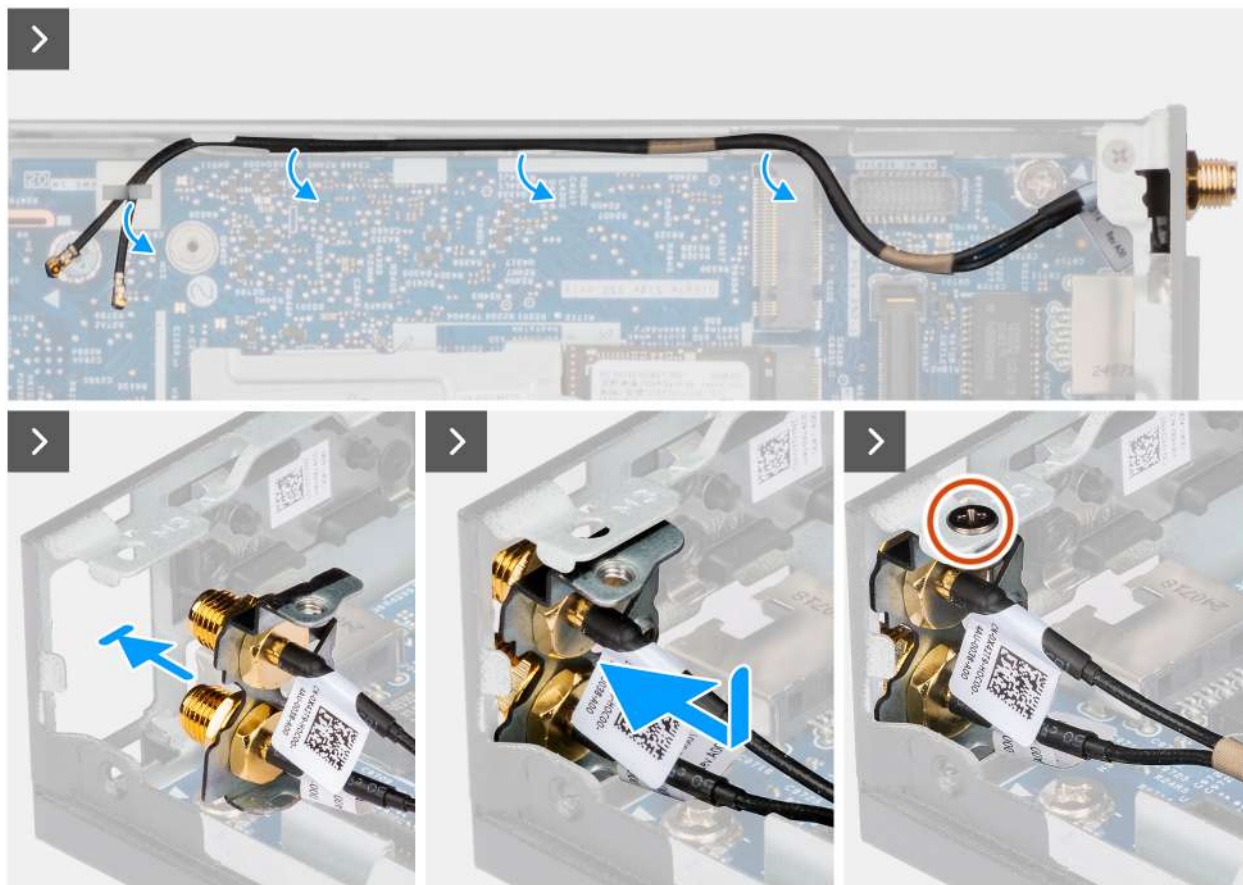
Afbeelding 37. De SMA-antennemodule plaatsen
