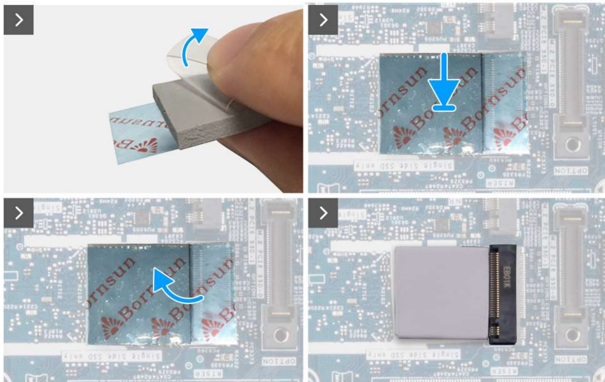
Afbeelding 17. De 2230 SSD installeren
