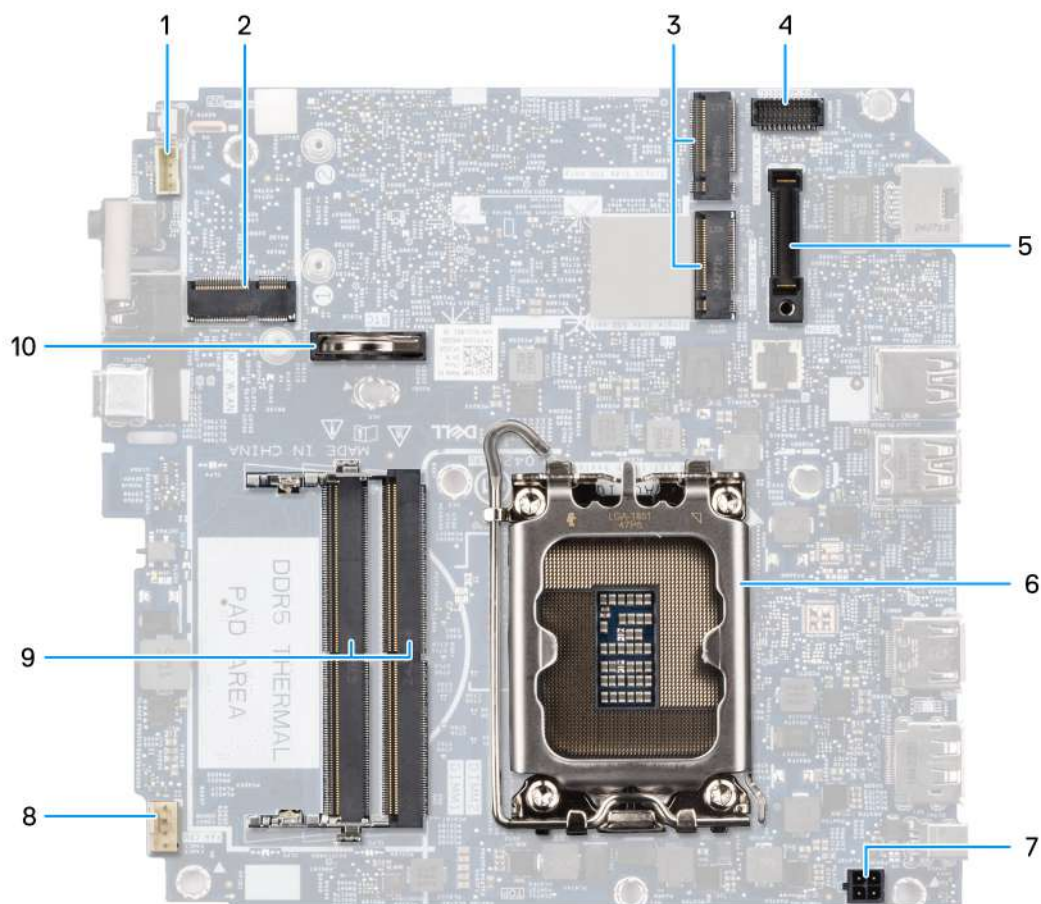
Afbeelding 77. Systeemkaartconnectoren
