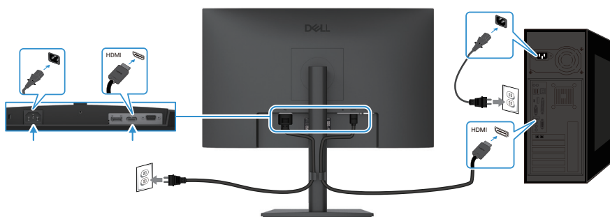
Afbeelding 16. HDMI-kabel aansluiten
