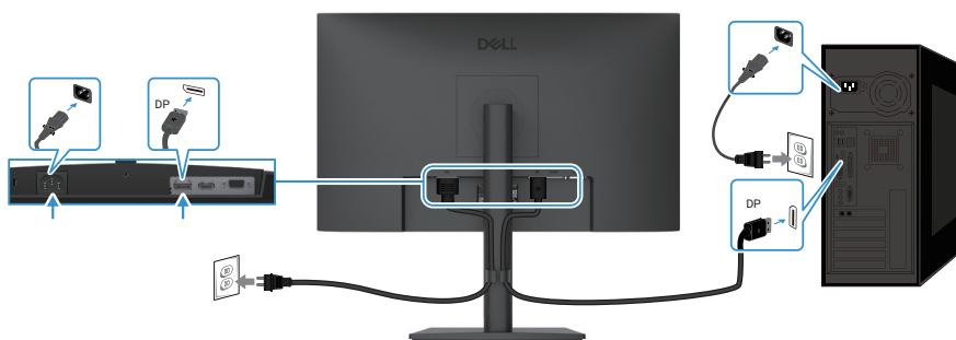
Afbeelding 15. DP-kabel aansluiten
