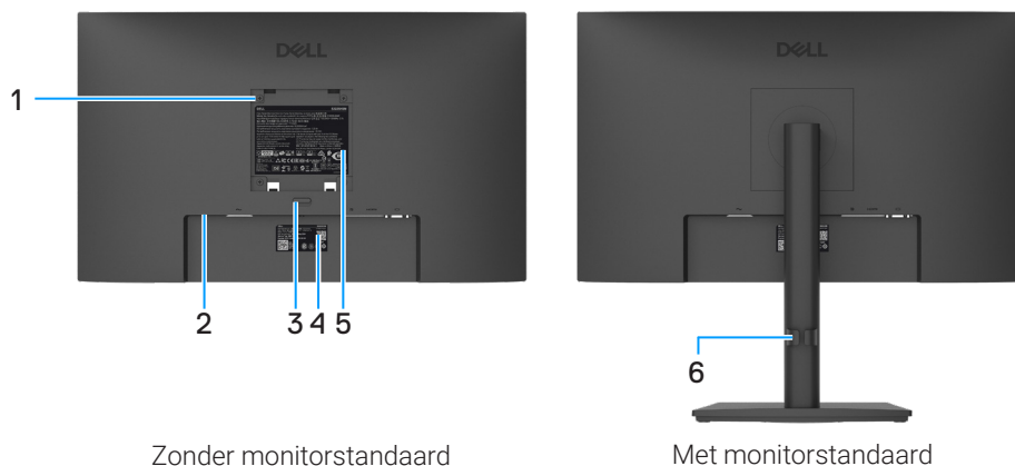
Afbeelding 2. Achteraanzicht
