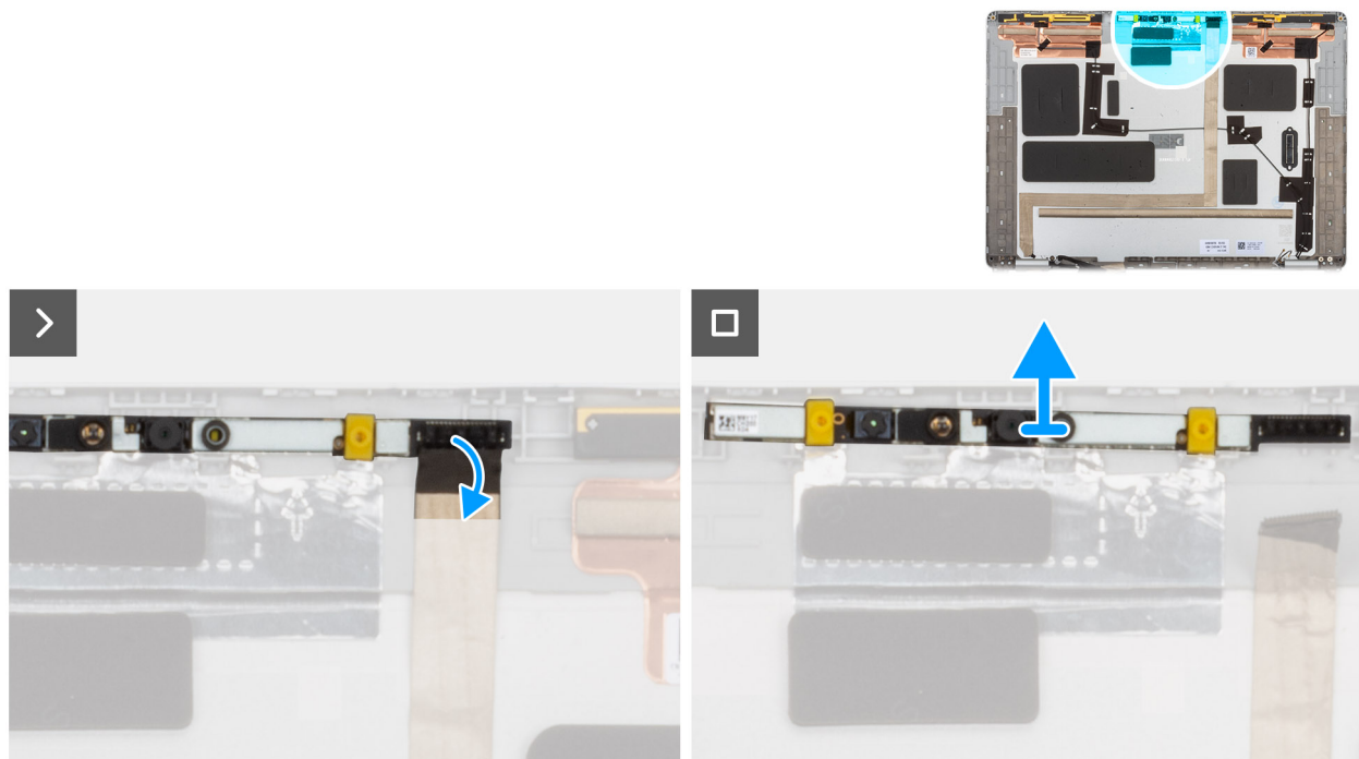
Abbildung 81. Entfernen der RGB/IR-Kamera
