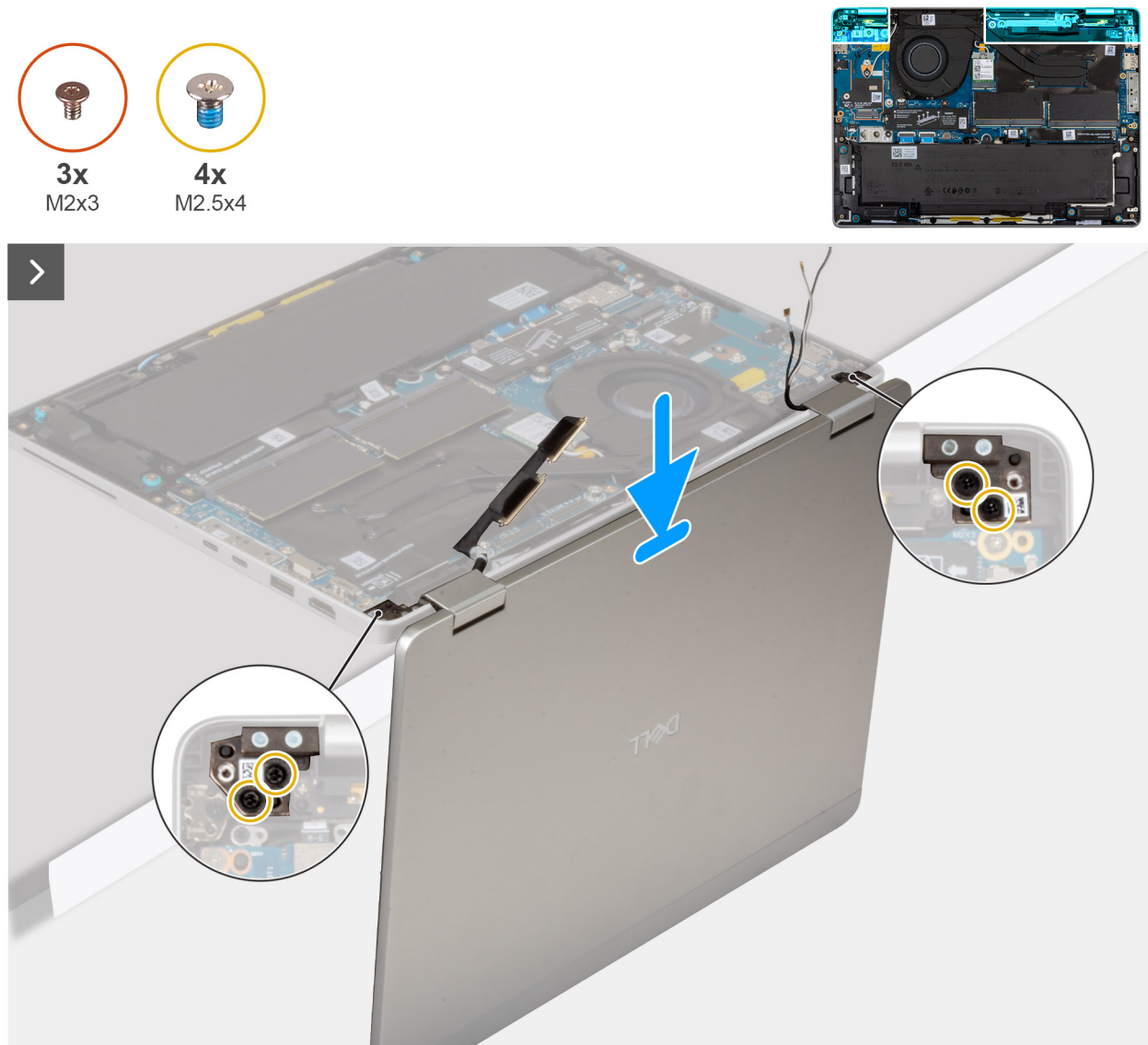
Abbildung 65. Einbauen der Displaybaugruppe
