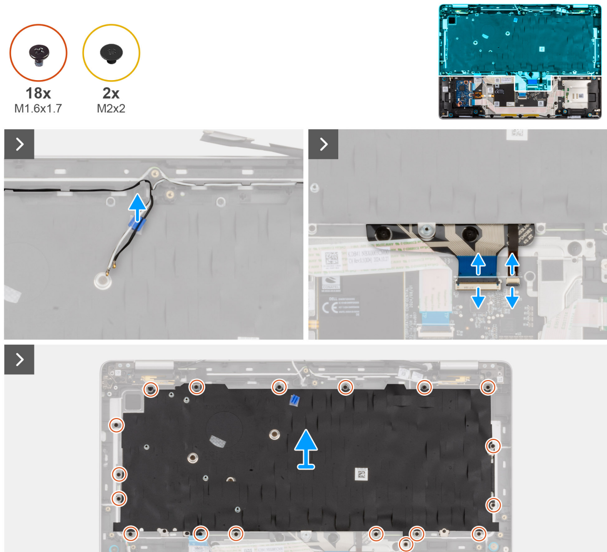
Abbildung 97. Entfernen der Tastatur
