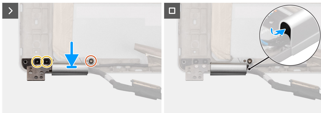
Abbildung 86. Einbauen des Bildschirmkabels
