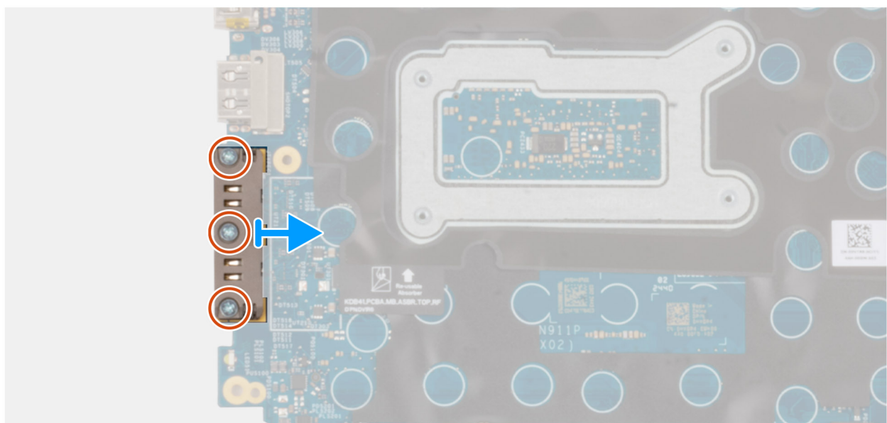
Abbildung 57. Entfernen des USB-Type-C-Anschlussmoduls
