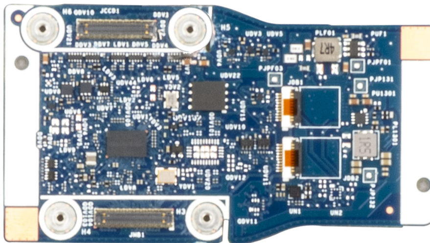
Abbildung 93. Mittlere Zusatzplatine
