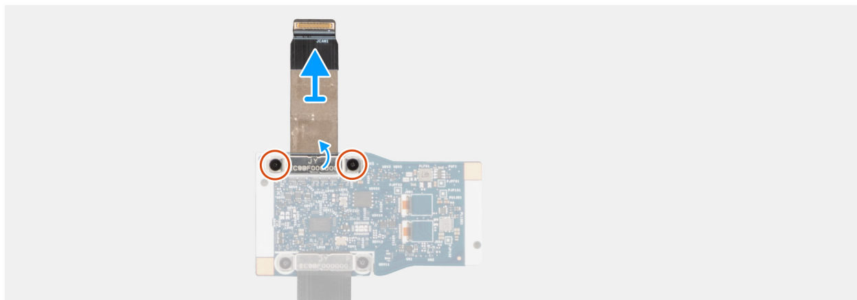
Abbildung 91. Entfernen des Kabels der mittleren Zusatzplatine
