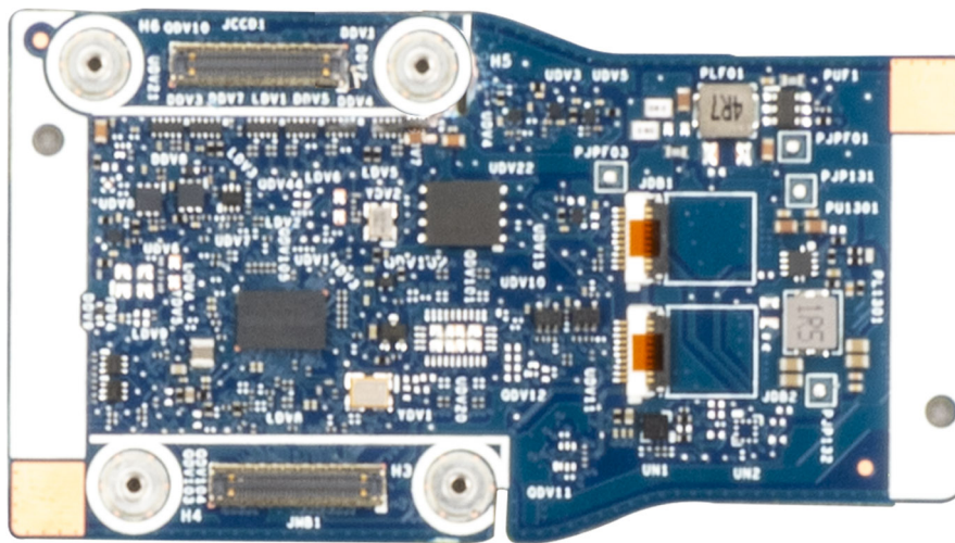
Abbildung 94. Mittlere Zusatzplatine
