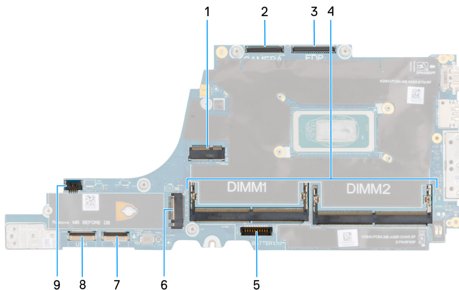
Abbildung 51. Anschlüsse auf der Hauptplatine
