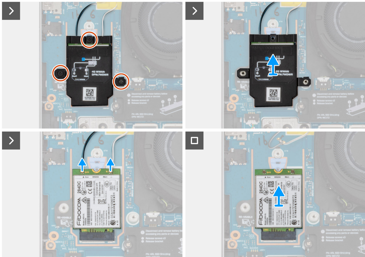
Abbildung 33. Entfernen der WWAN-Karte
