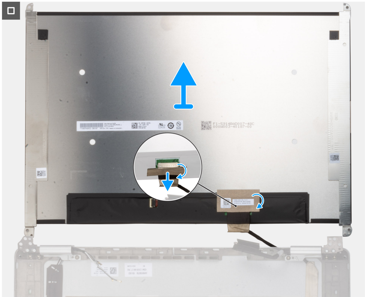
Abbildung 75. Entfernen des Bildschirms
