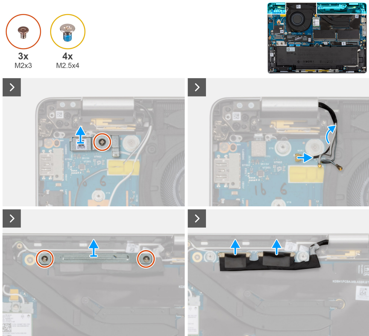
Abbildung 63. Entfernen der Bildschirmbaugruppe
