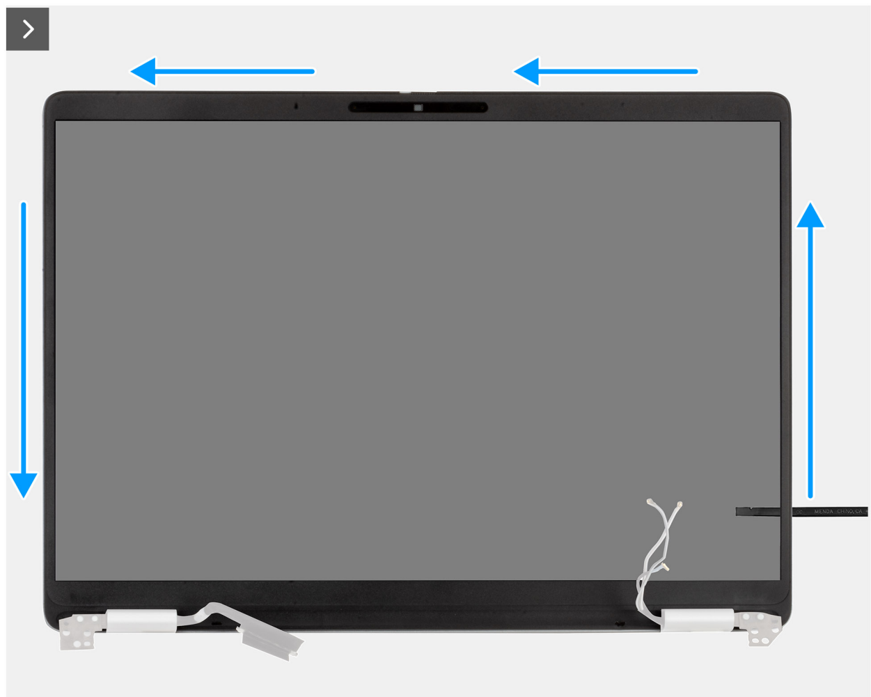
Abbildung 70. Entfernen der Bildschirmblende
