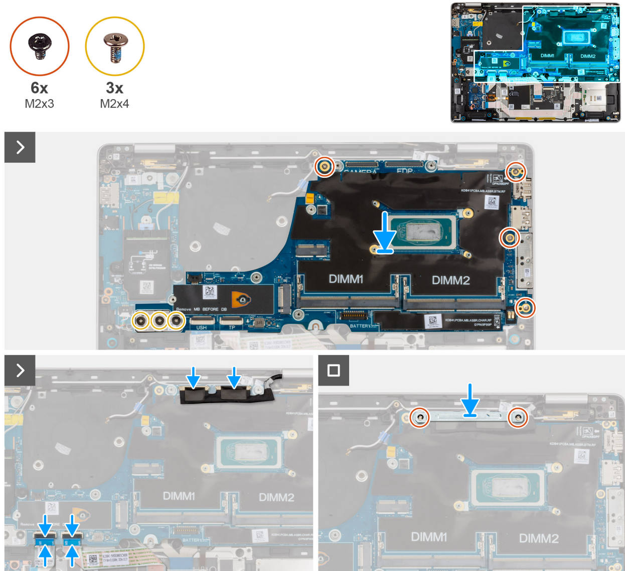
Abbildung 52. Einbauen der Systemplatine
