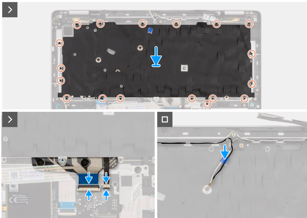
Abbildung 100. Einbauen der Tastatur
