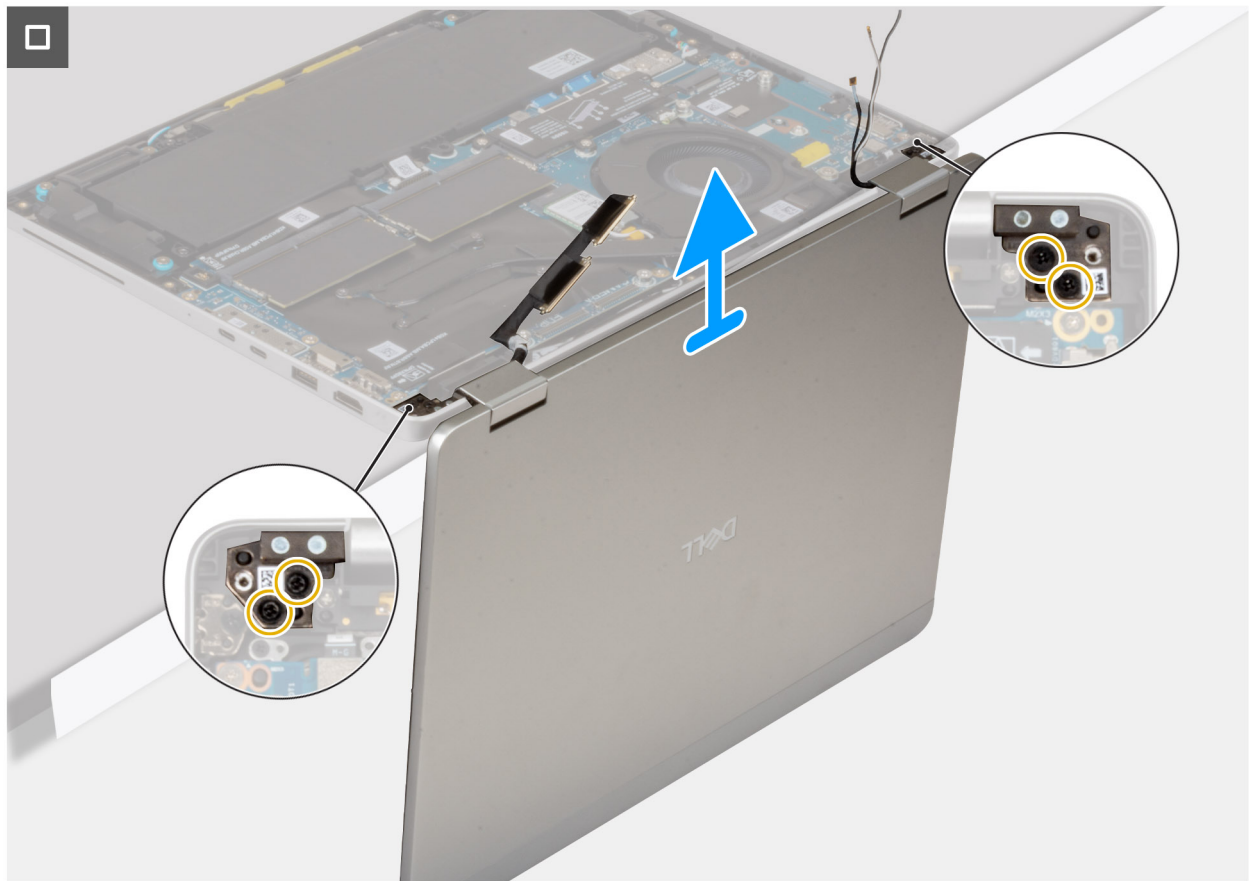
Abbildung 64. Entfernen der Bildschirmbaugruppe
