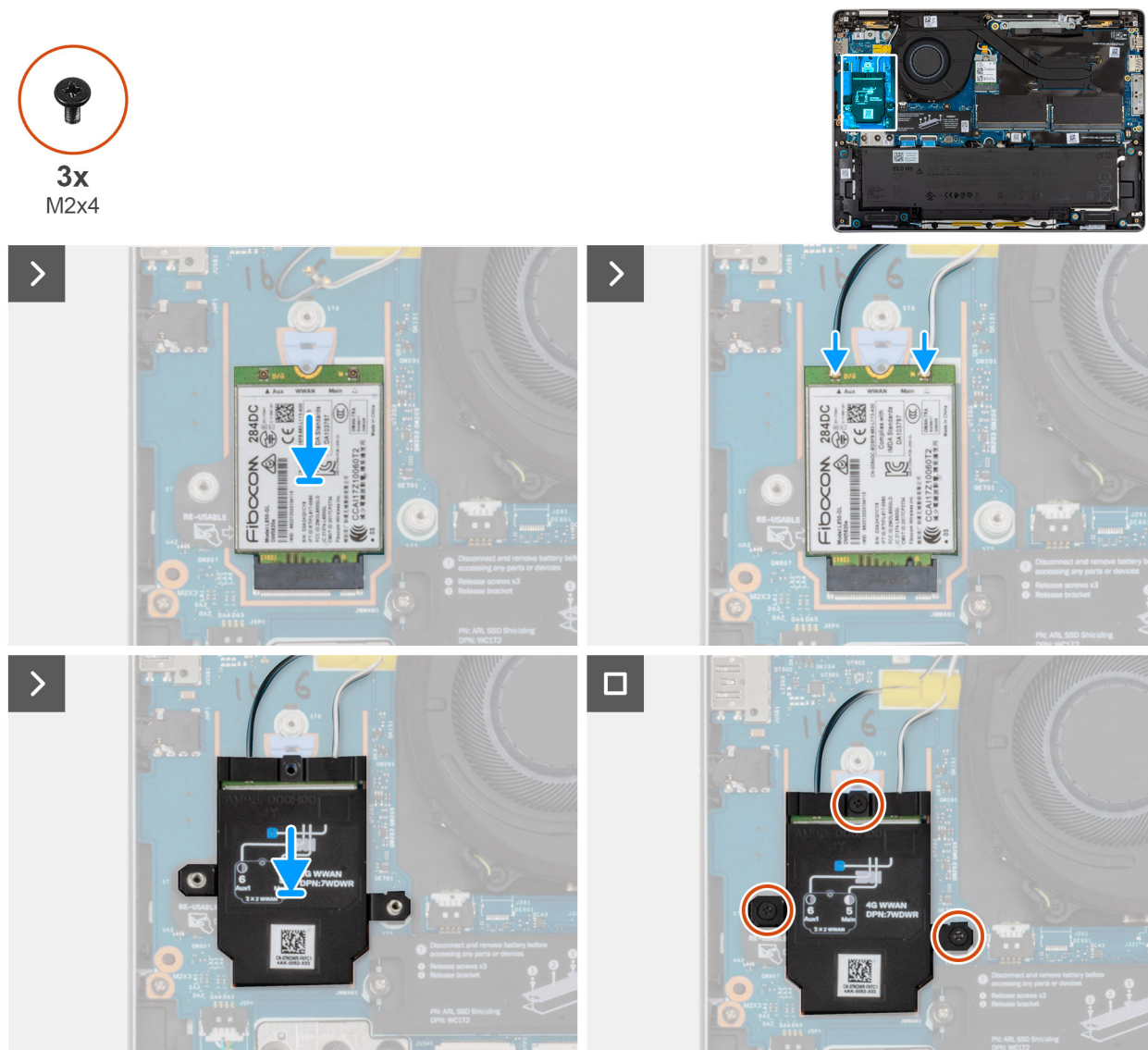
Abbildung 34. Einbauen der WWAN-Karte
