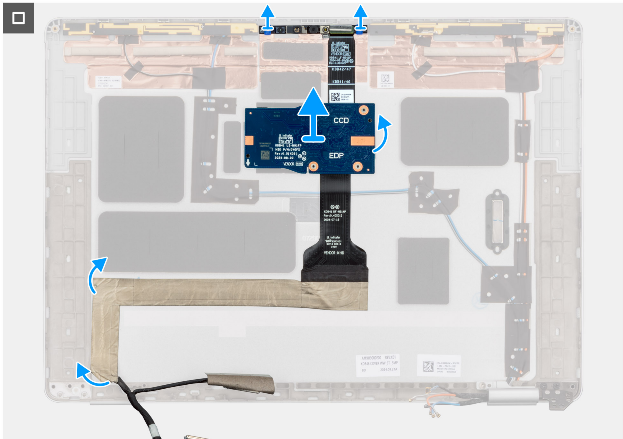
Abbildung 84. Entfernen des Bildschirmkabels
