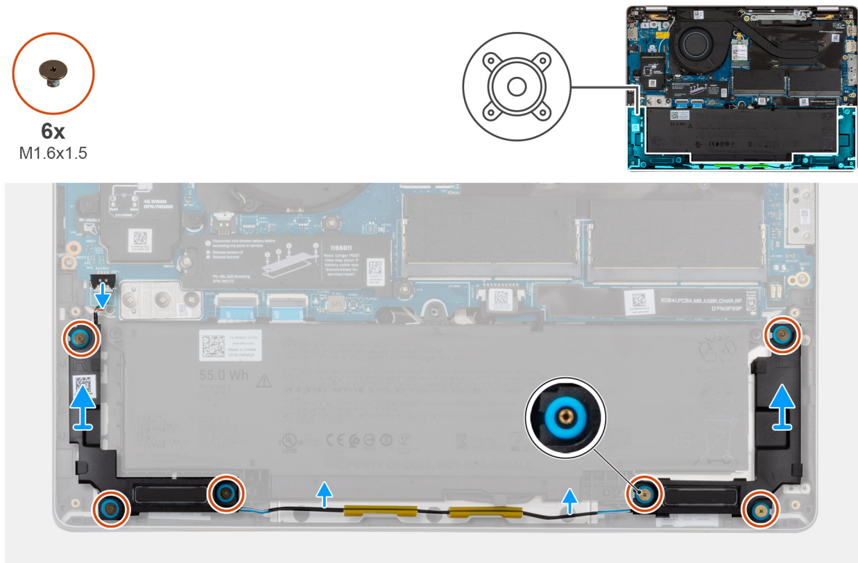
Abbildung 41. Entfernen der Lautsprecher
