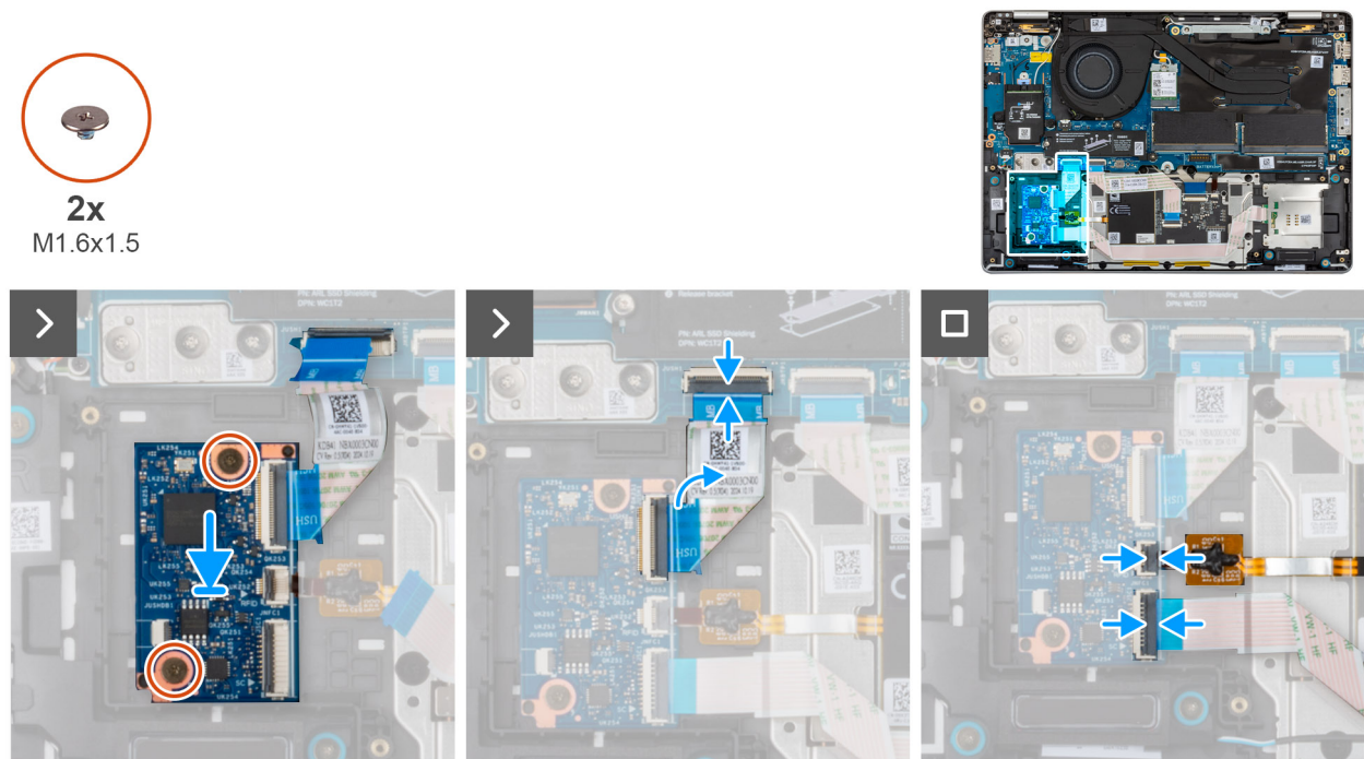
Abbildung 46. Installieren der USH-Zusatzplatine
