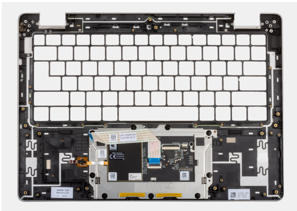
Abbildung 102. Handauflagenbaugruppe
