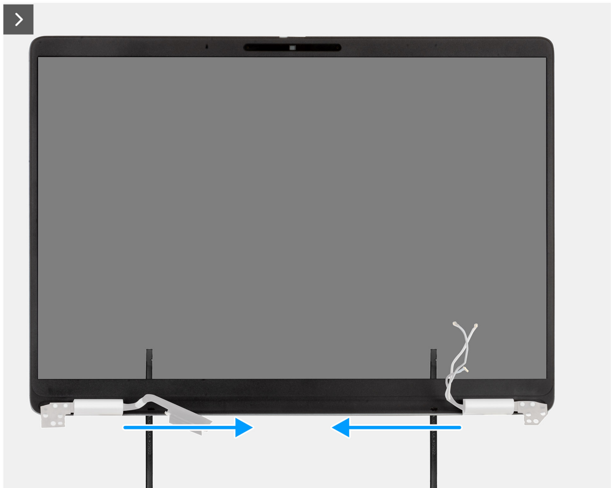
Abbildung 68. Entfernen der Bildschirmblende
