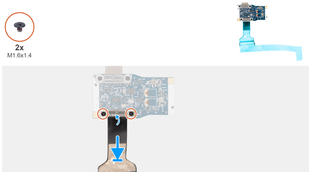
Abbildung 90. Installieren des Bildschirmkabels für die MIPI-Kamera
