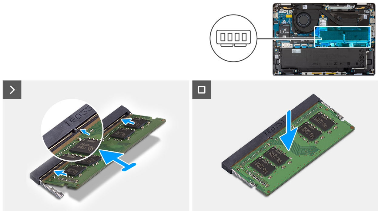
Abbildung 32. Einsetzen des Speichermoduls
