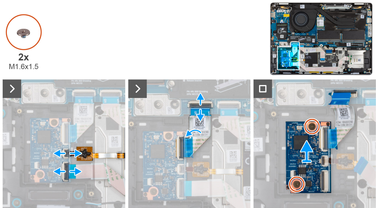
Abbildung 45. Entfernen der USH-Zusatzplatine
