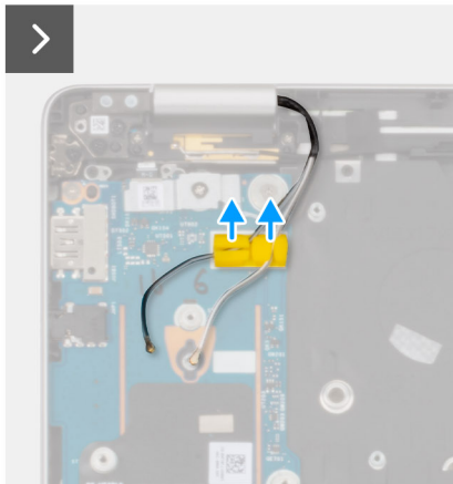
Abbildung 53. Entfernen des WLAN-Antennenmoduls
