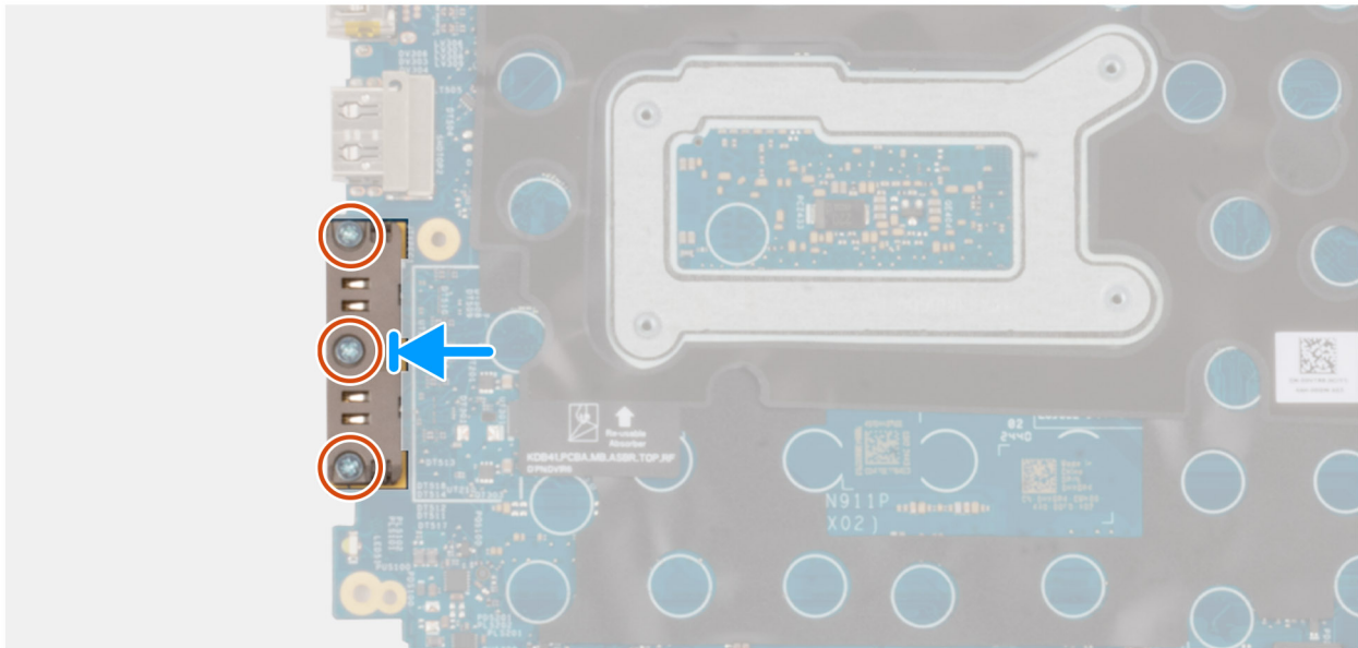
Abbildung 58. Installieren des USB-Type-C-Anschlussmoduls
