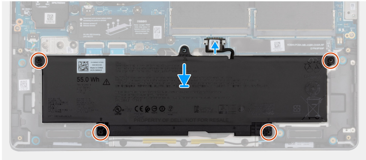
Abbildung 28. Einsetzen des Akkus
