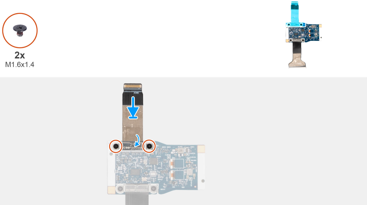
Abbildung 92. Installieren des Kabels der mittleren Zusatzplatine
