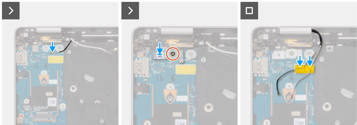
Abbildung 56. Einbauen des WLAN-Antennenmoduls
