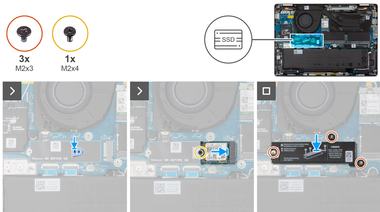
Abbildung 36. Einbauen des M.2-2280-SSD
