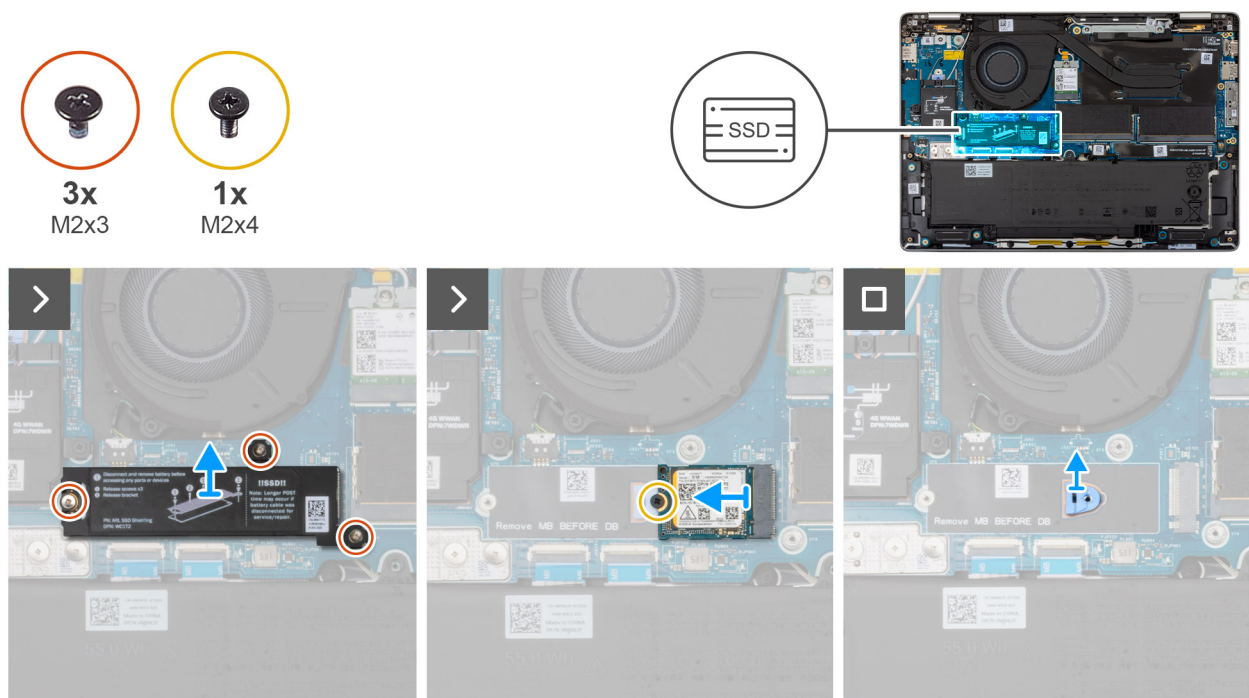
Abbildung 35. Entfernen des M.2-2230-Solid-State-Laufwerks
