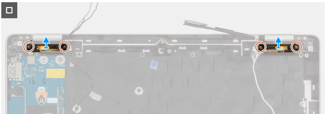
Abbildung 54. Entfernen des WLAN-Antennenmoduls
