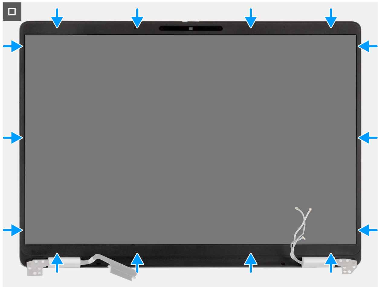
Abbildung 73. Einbauen der Bildschirmblende
