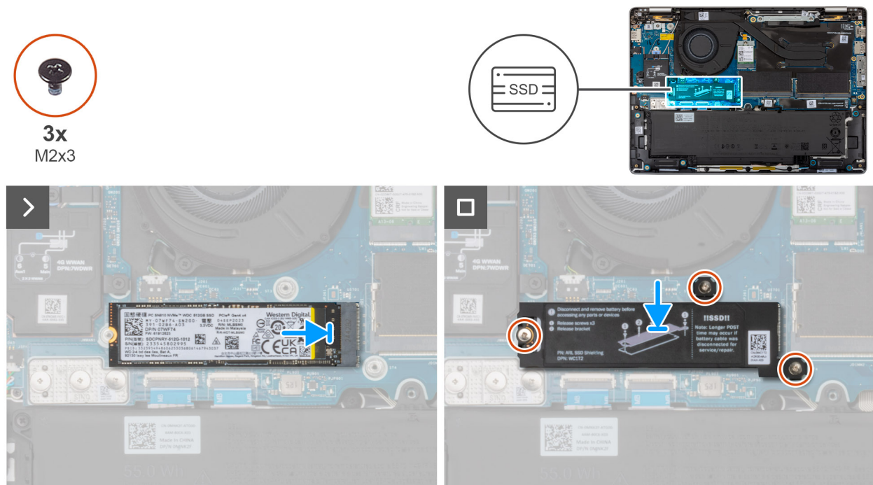
Abbildung 38. Installieren der M.2-2280-SSD
