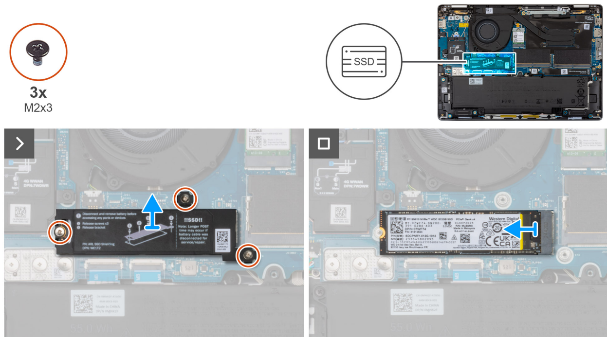
Abbildung 37. Entfernen der M.2-2280-SSD
